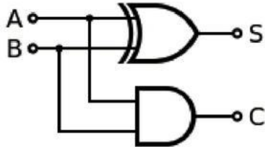
FIGURE 5.5 : Un demi-additionneur.
