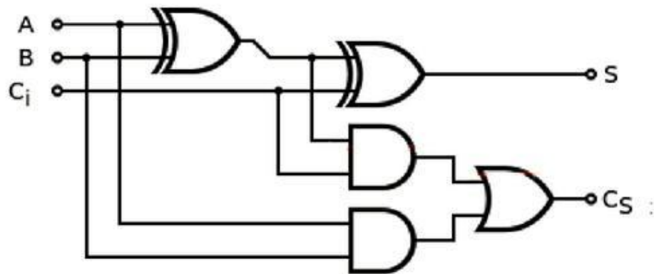
FIGURE 5.6 : Un additionneur complet (full-adder).
