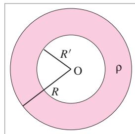
Fig. 3.10. Coquille sphérique uniformément chargée.
