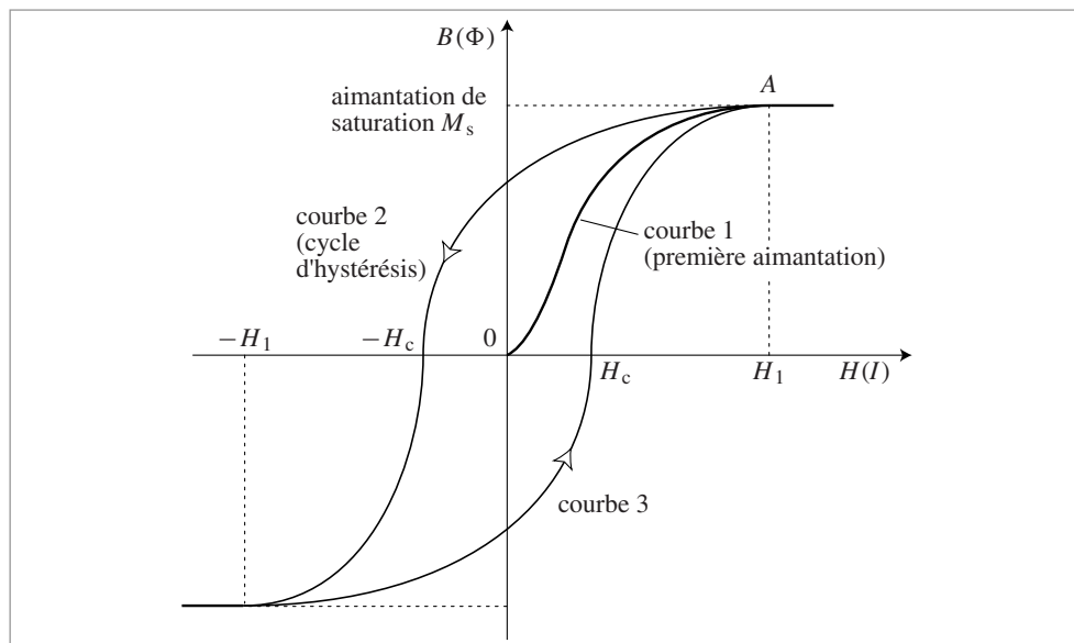
Fig. 12.6. Courbes d'hystérésis.
