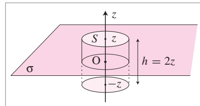
Fig. 3.14. Surface de Gauss permettant de calculer le champ électrostatique créé par un plan infini uniformément chargé.
