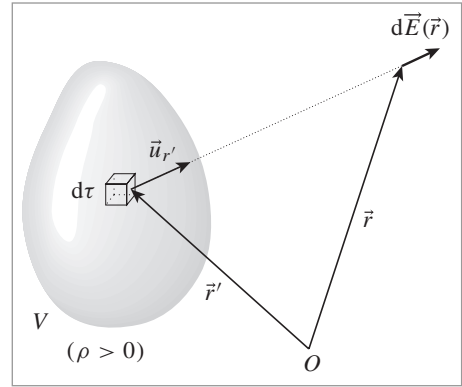
Fig. 2.5. Champ électrostatique créé par un élément infinitésimal de charge électrique dq .
