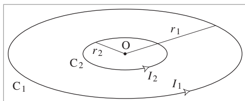
Fig. 11.5. Calcul de l'inductance mutuelle de deux spires.
