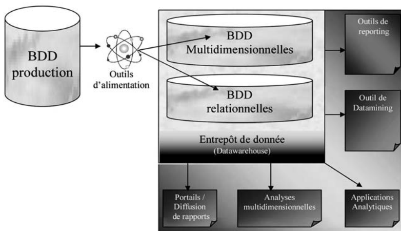
Figure 53. Architecture décisionnelle
