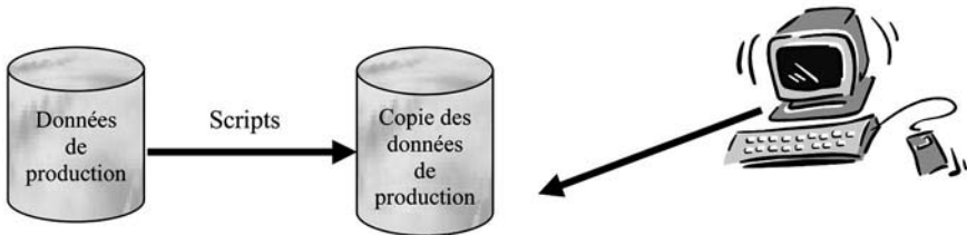
Figure 50. Architecture « infocentre »
