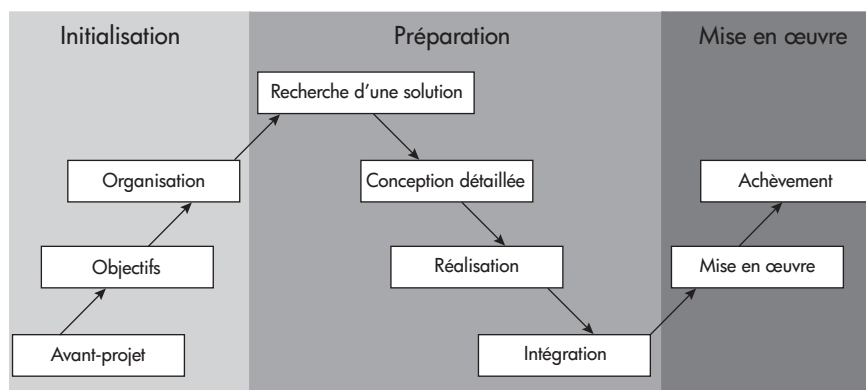
Figure 13. Cycle d'intégration
