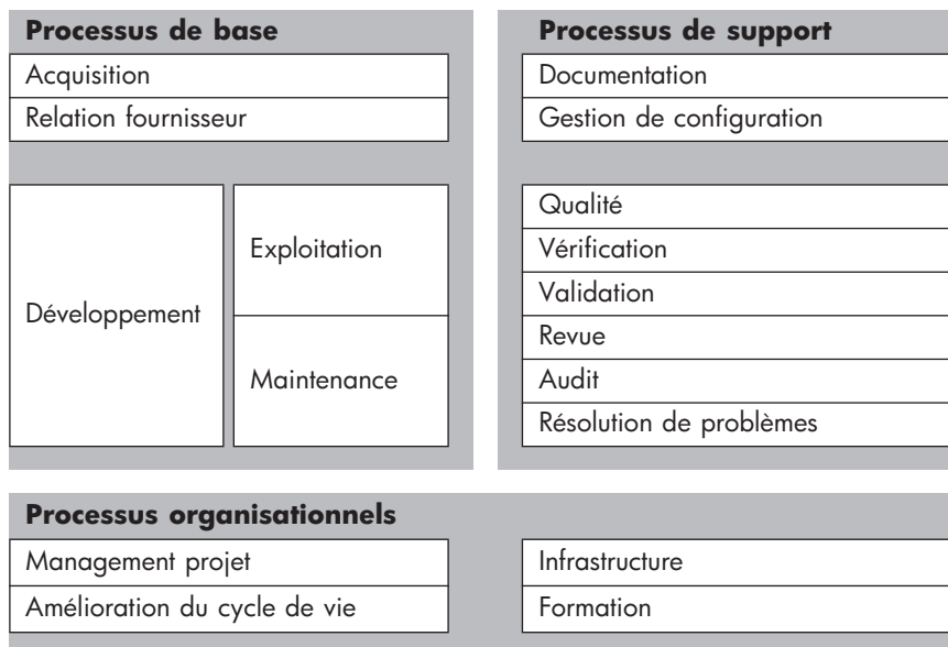
Figure 11. Modèle ISO 12207
