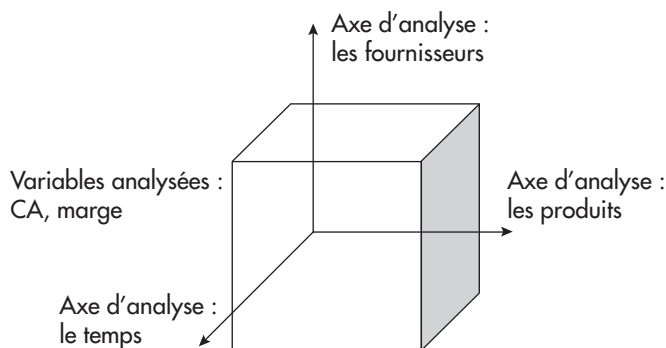
Figure 60. Cube multidimensionnel
