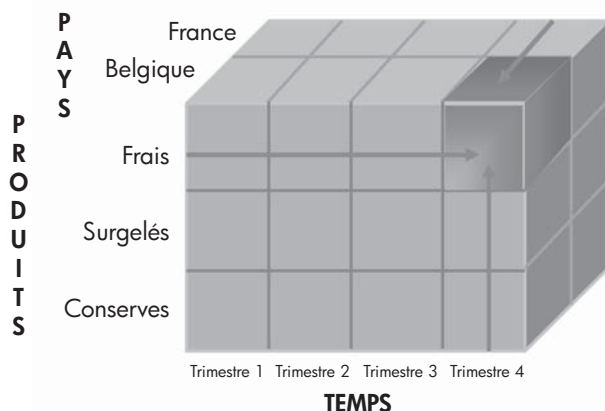
Figure 55. Cube multidimensionnel
