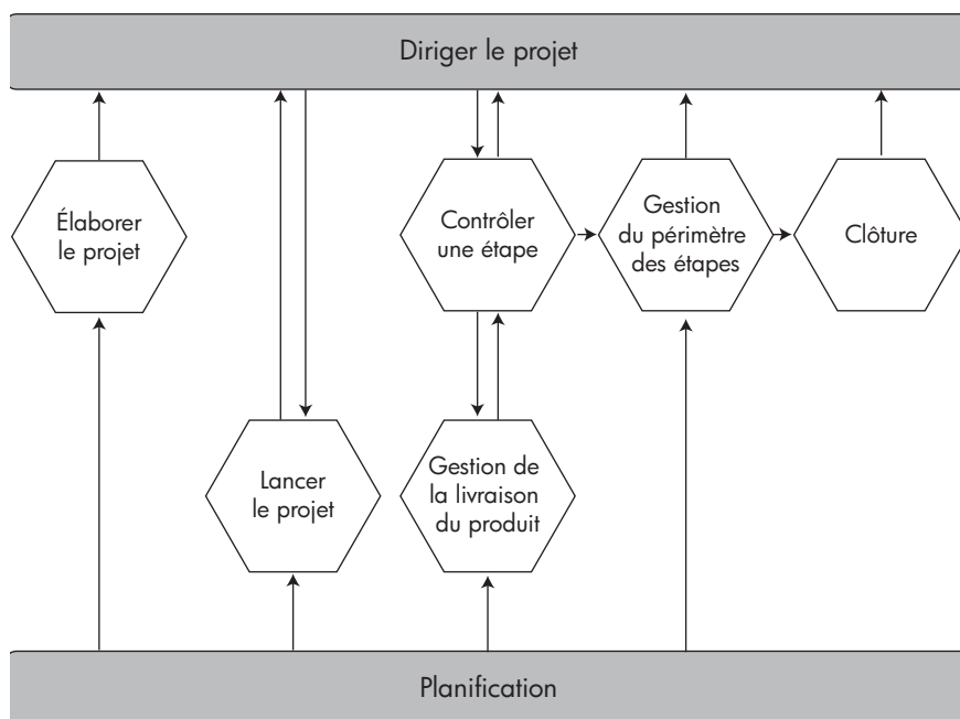
Figure 28. Méthodologie PRINCE2
