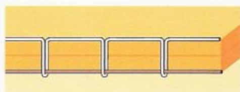
Tension du fil de la canette trop forte
