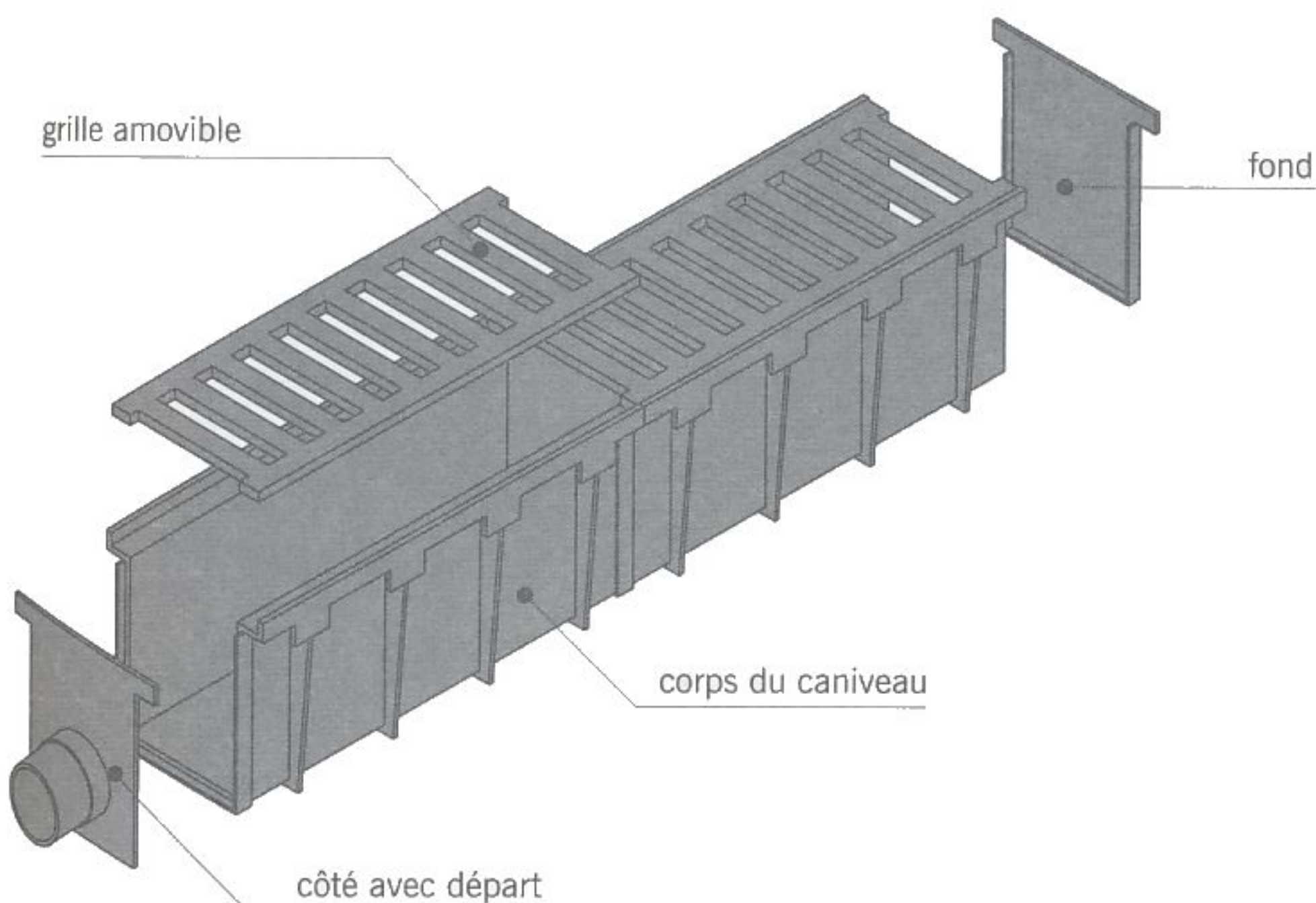
fig. 7.71 caniveau en plastique
