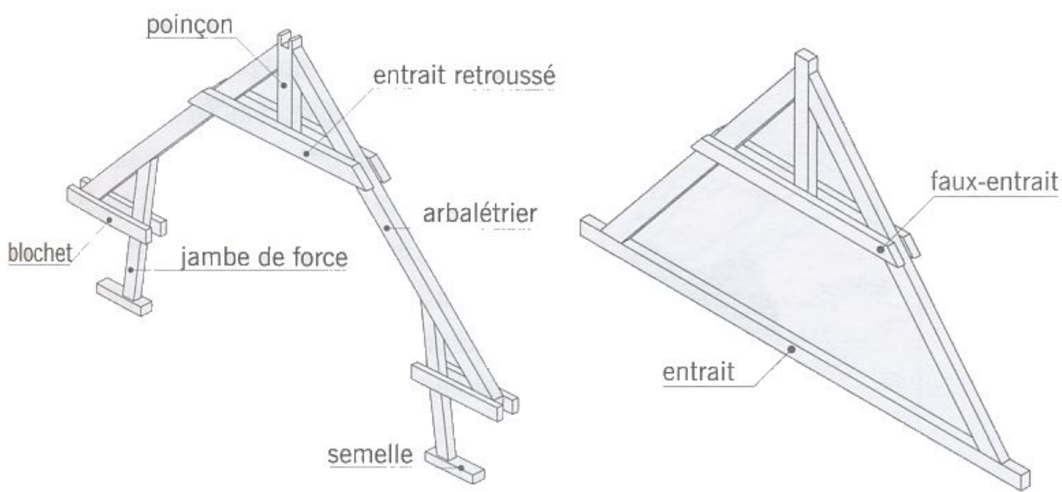
fig. 5.7 ferme à entrain retroussé
