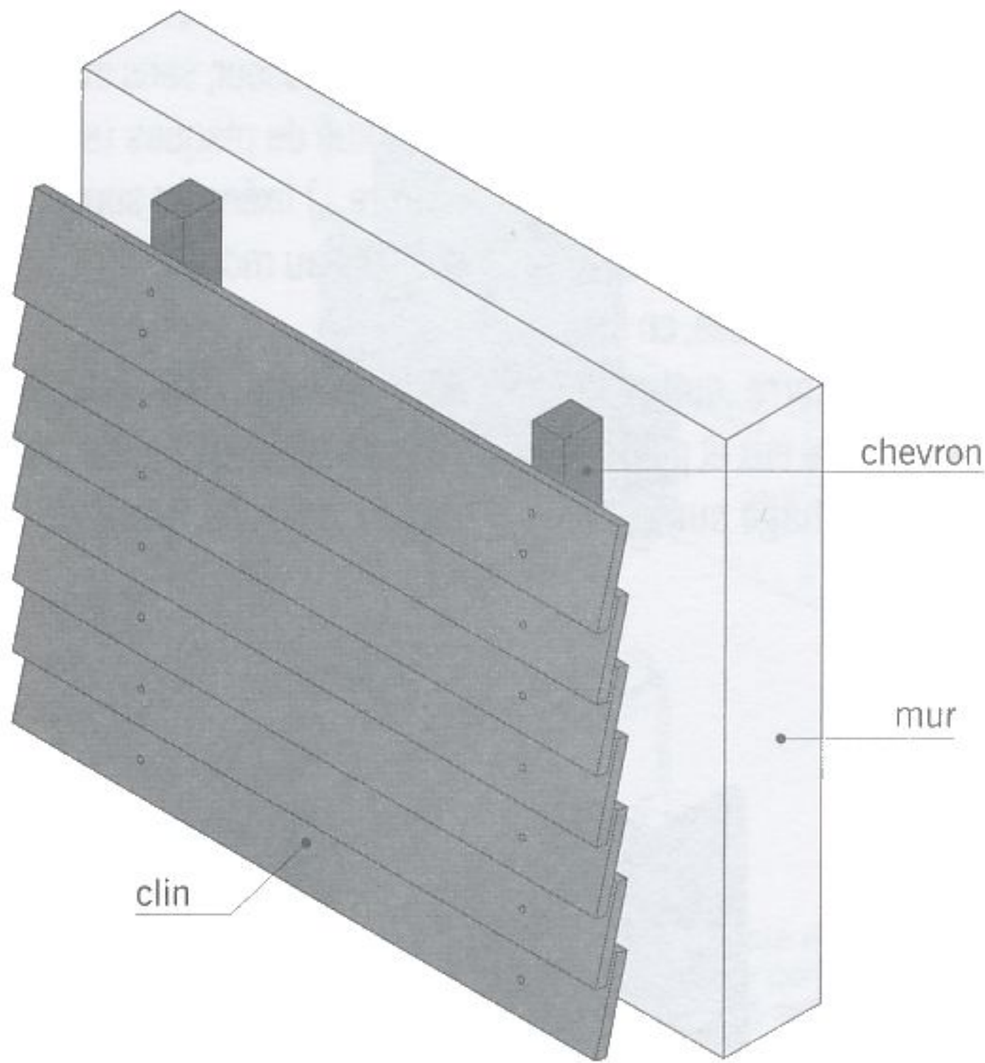
bardage en clin
