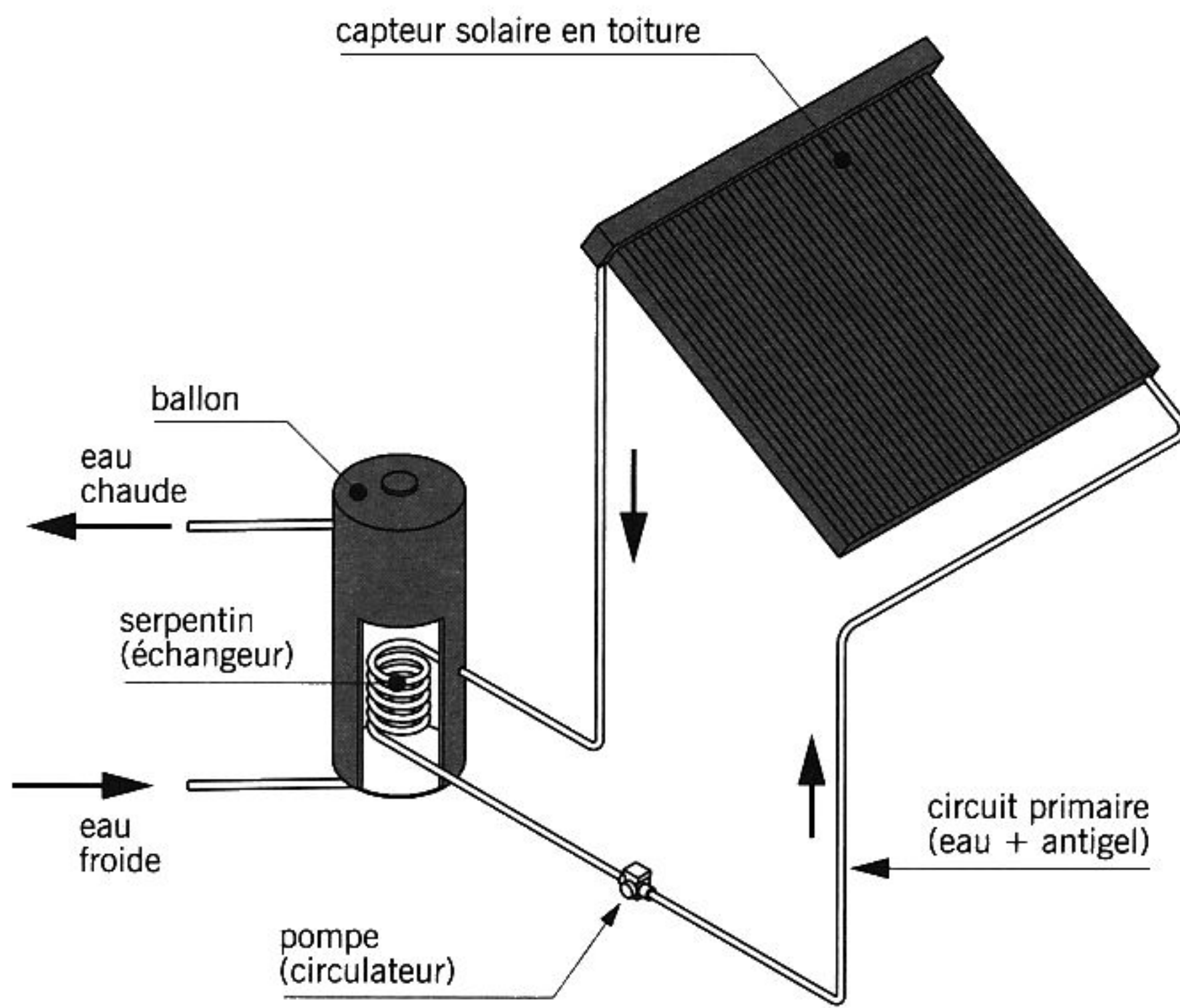
fig. 14.13 chauffe-eau solaire à éléments séparés (schéma d'installation)
