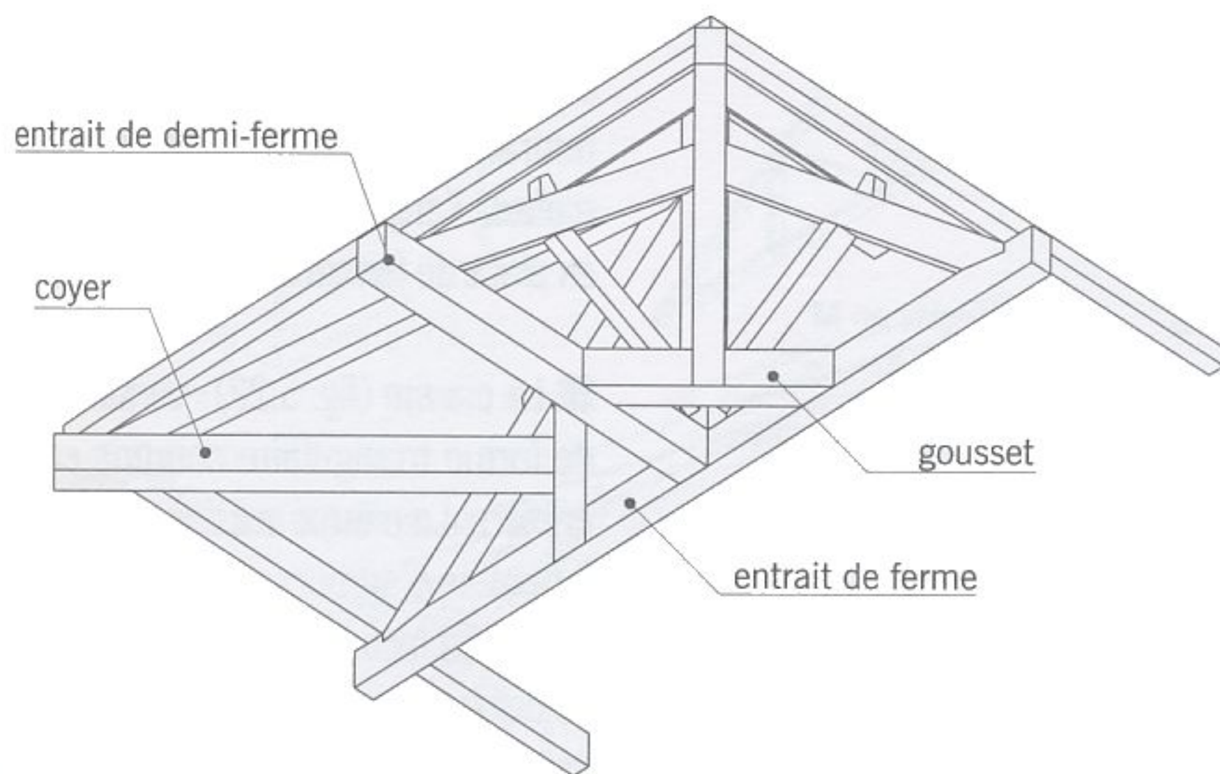
fig. 5.14 enrayure observée par dessous
