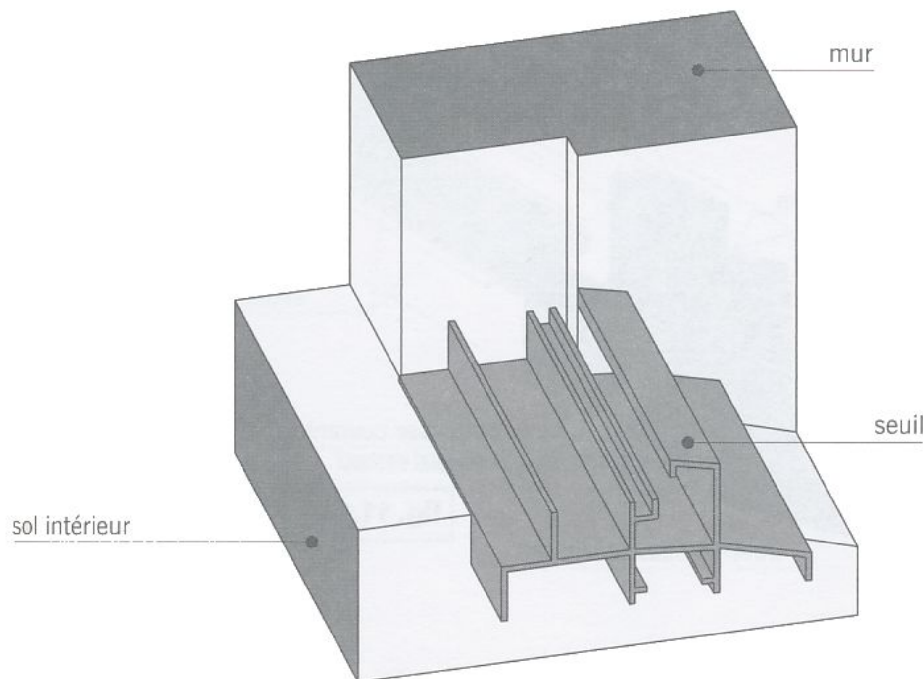
fig. 11.9 seuil de porte-fenêtre en aluminium
