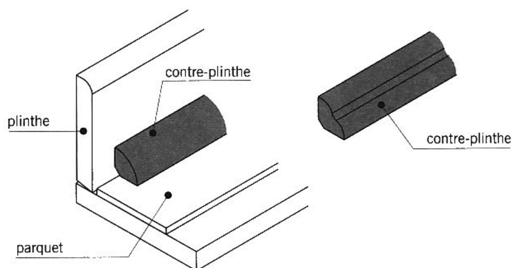
fig. 12.30 contre-plinthes
