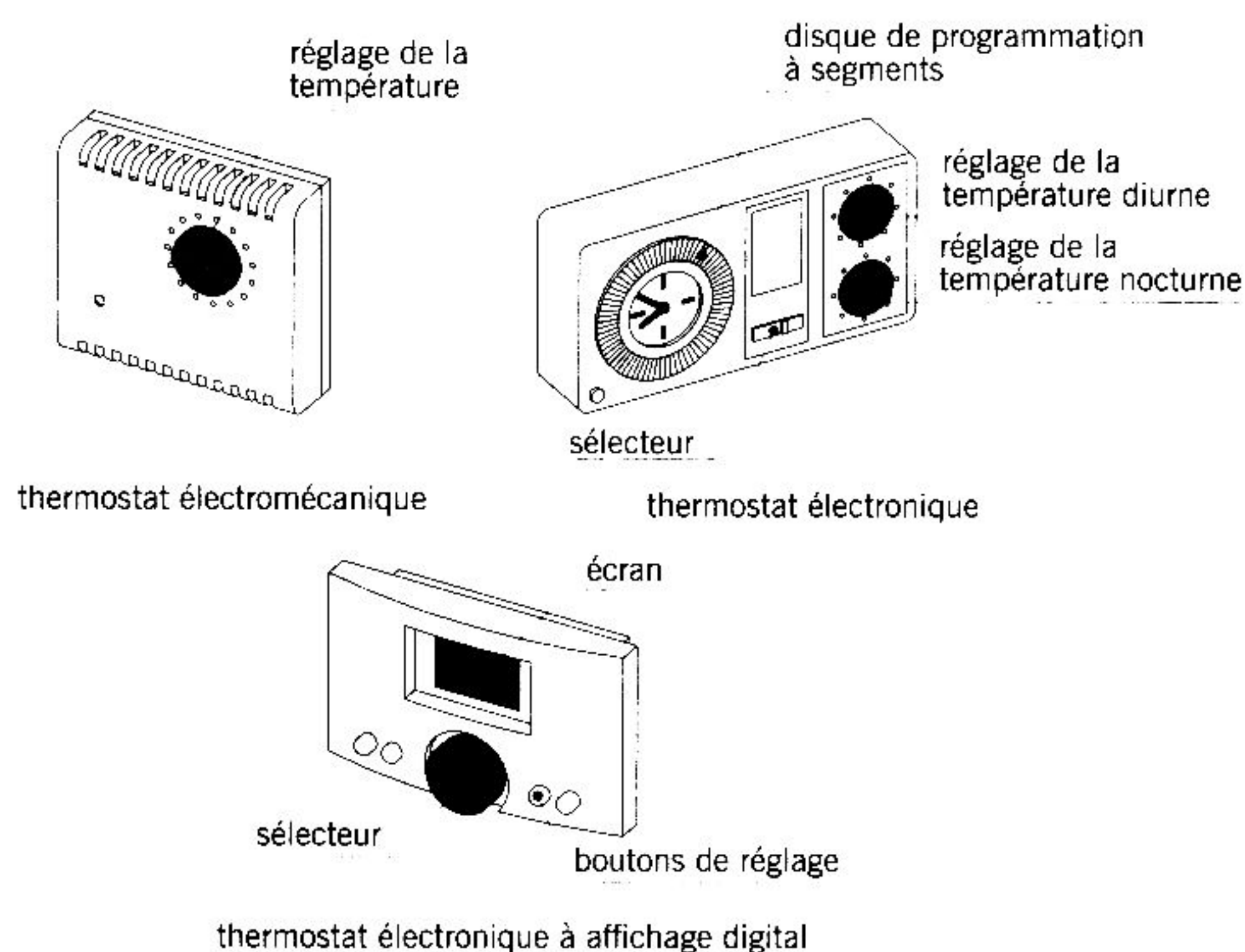
fig. 17.1 thermostats d'ambiance
