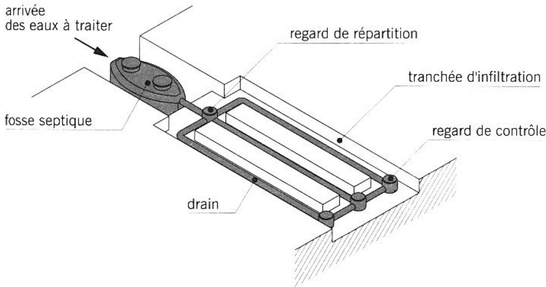
fig. 15.15 tranchées d'épandage à faible profondeur
