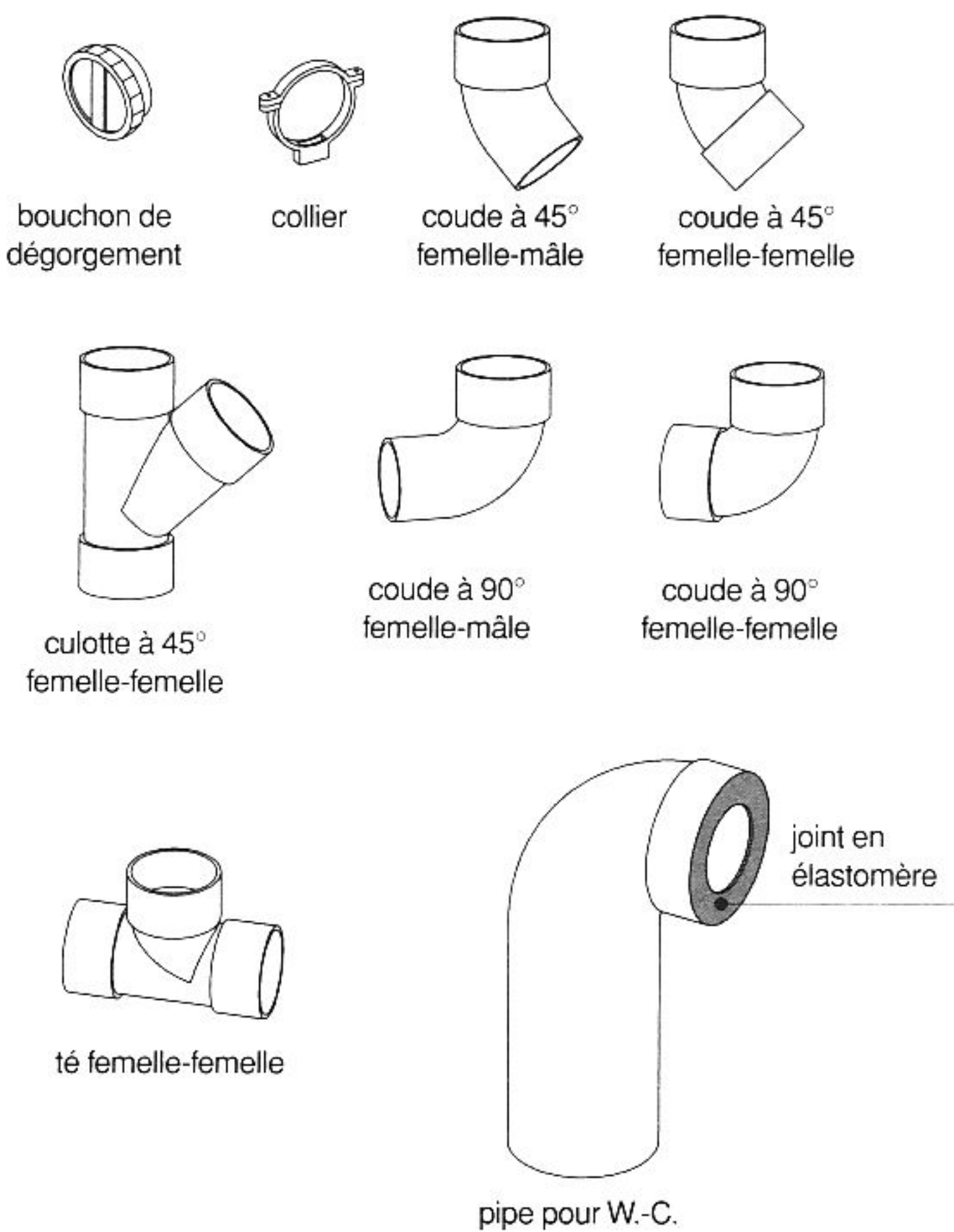
fig. 15.2 accessoires et raccords en PVC
