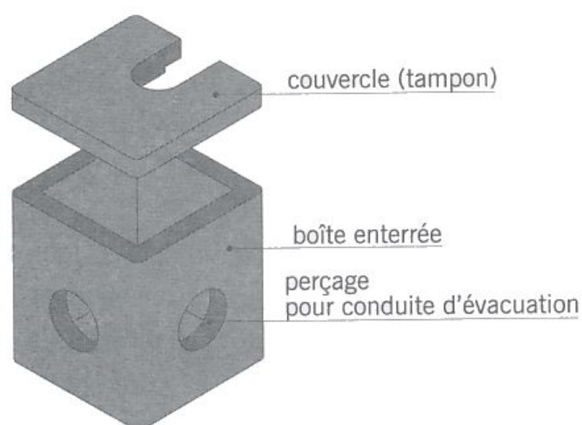
fig. 7.62 regard pour eaux pluviales
