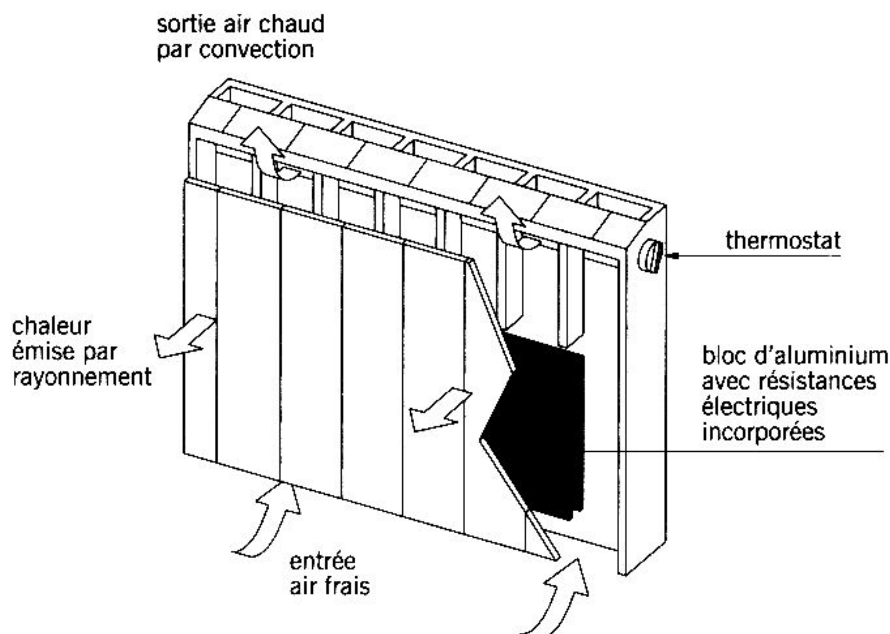
fig. 17.7 radiateur à deux modes de transmission
