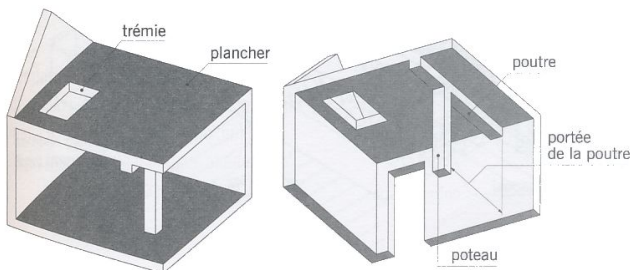
fig. 4.10 mots du plancher
