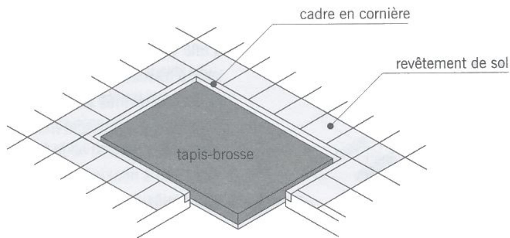
fig. 10.21 tapis brosse
