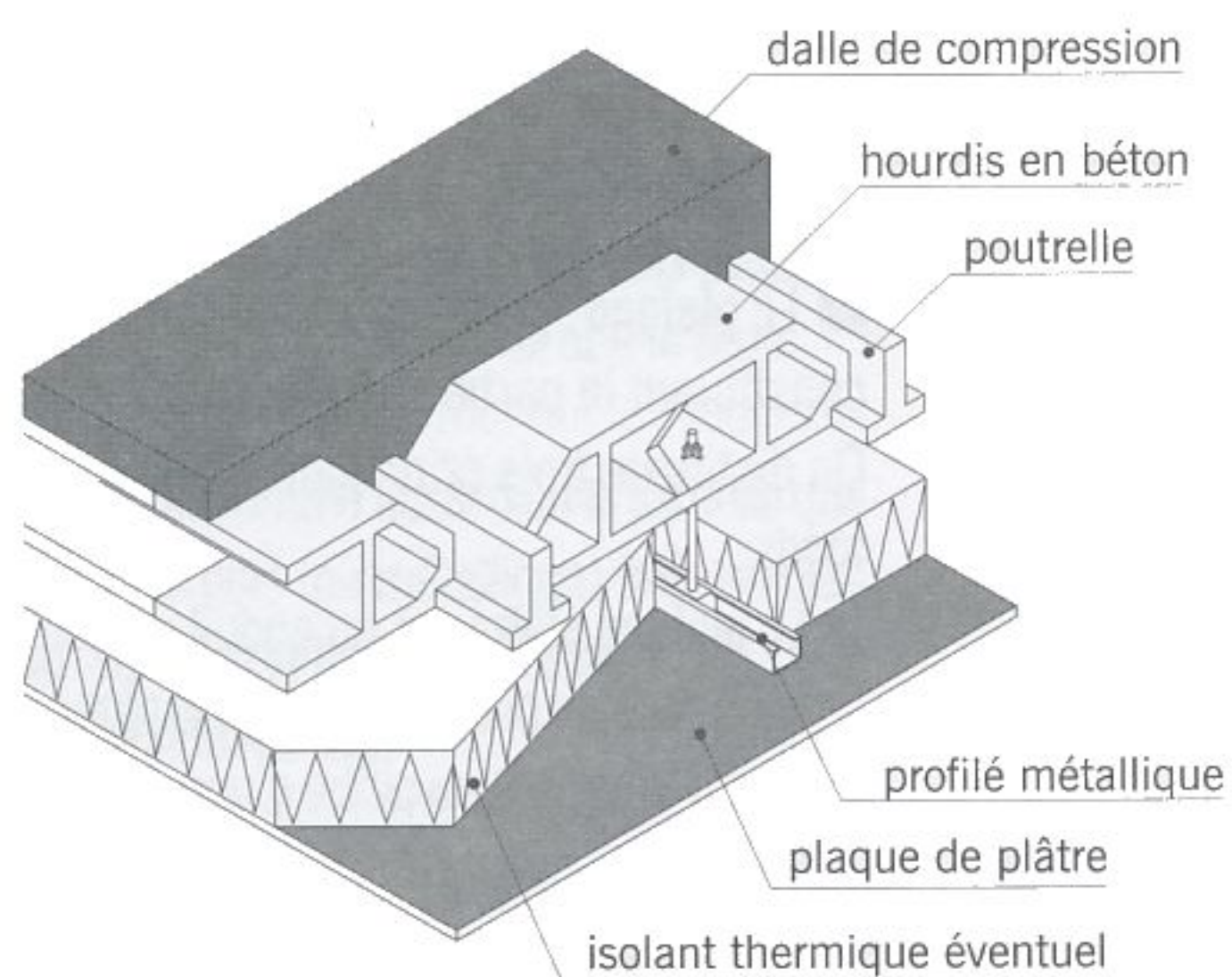
plafond suspendu sous plancher béton
