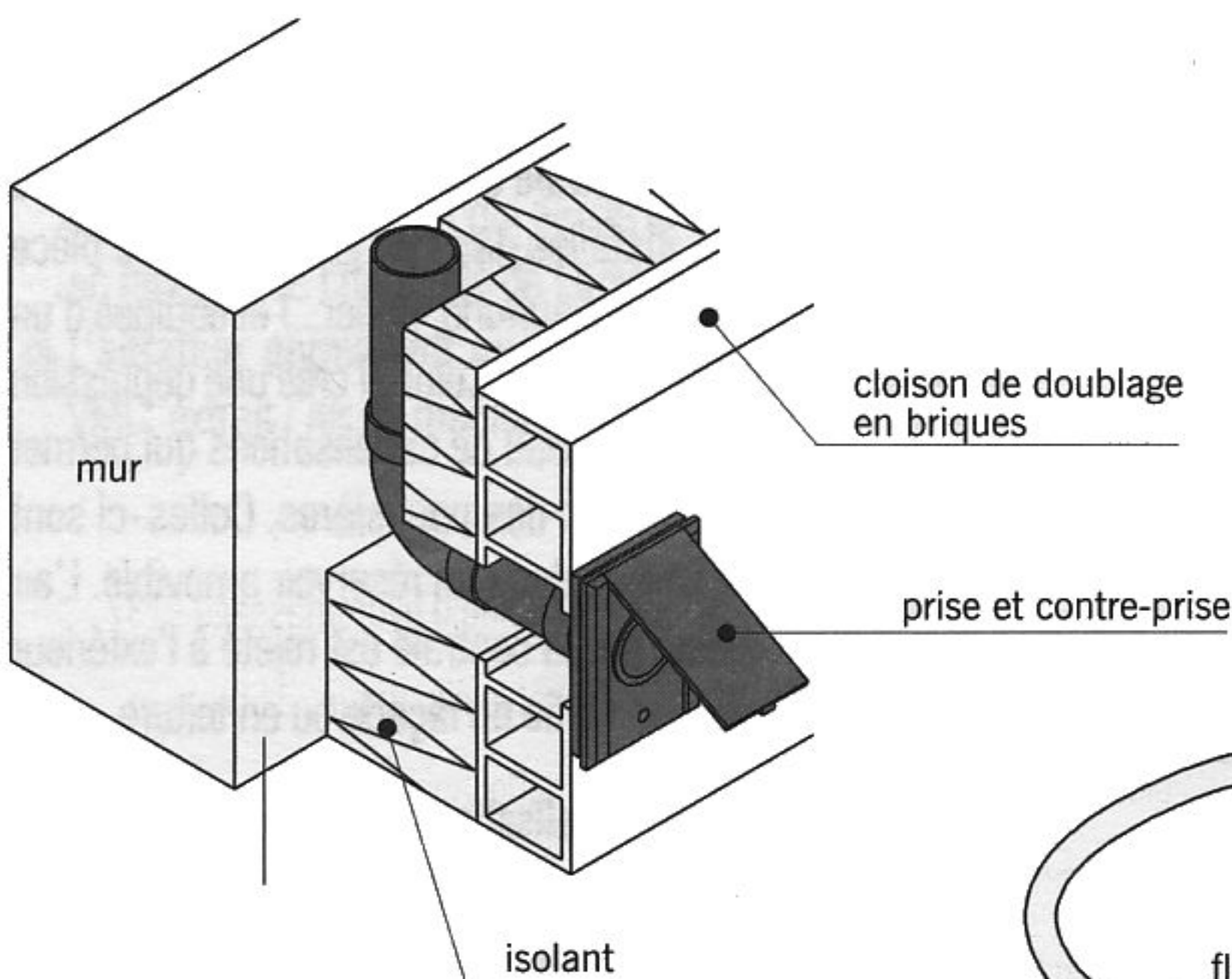
fig. 19.5 contre-prises
