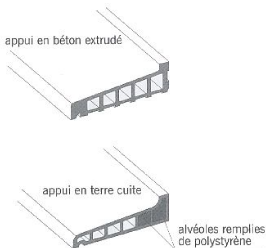
fig. 3.32 appuis de baie préfabriqués
