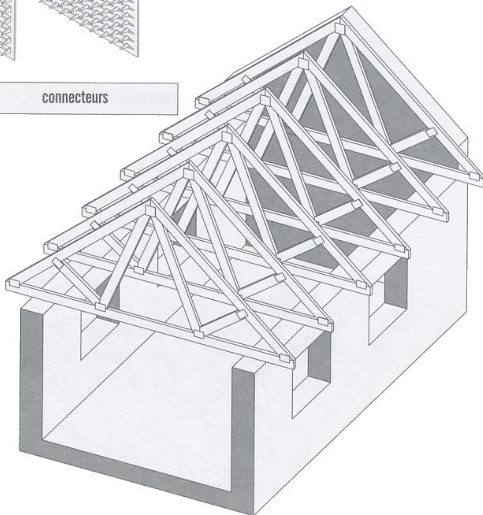
fig. 5.17 charpente en fermettes pour combles perdus
