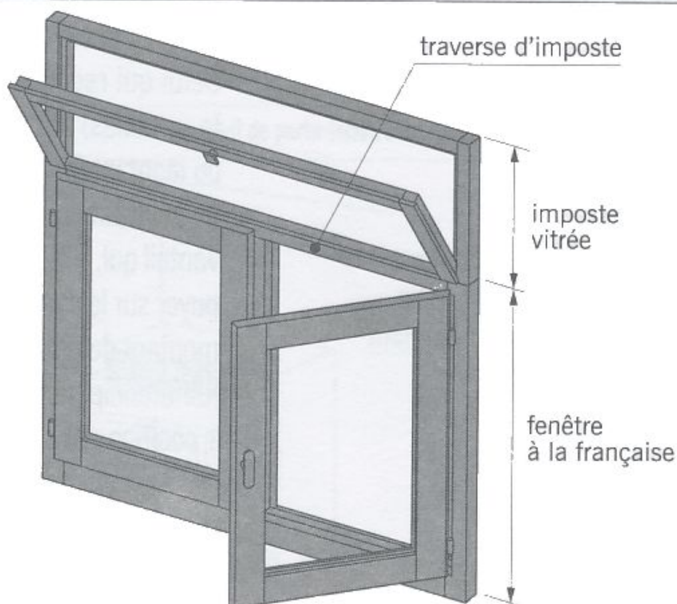
fig. 11.3 fenêtre composée en bois (fenêtre à la française + imposte)
