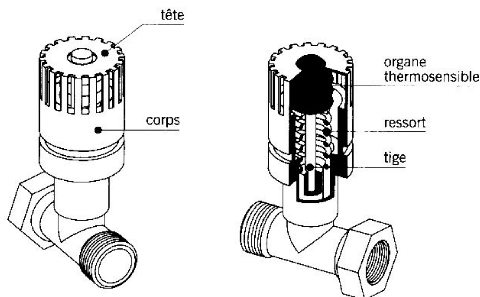
fig. 17.2 robinet thermostatique
