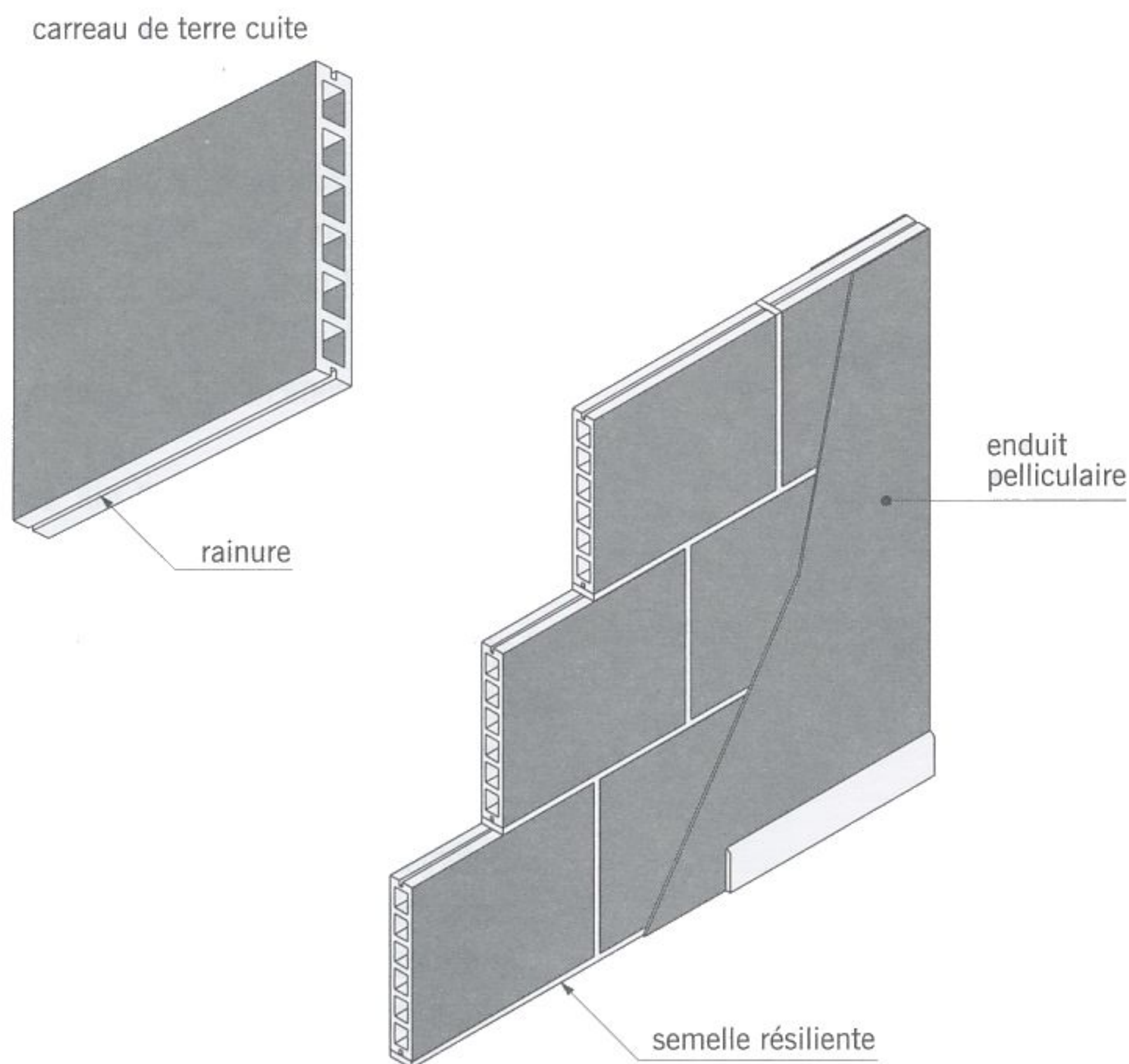
cloison pleine en carreaux de terre cuite
