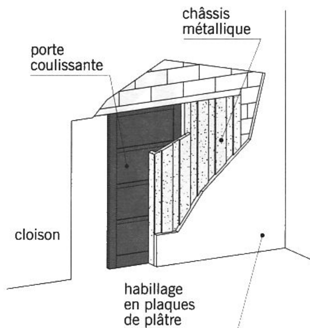
fig. 12.12 porte coulissante escamotable
