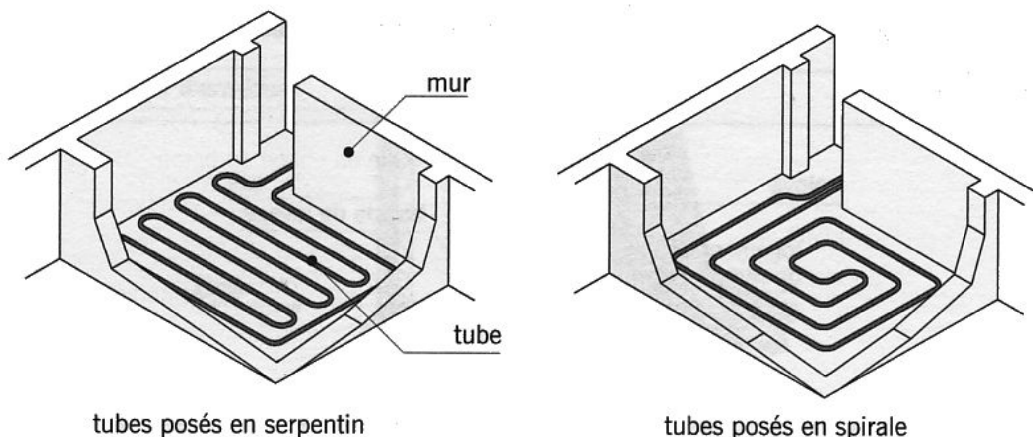
fig. 17.30 modes de pose des tubes
