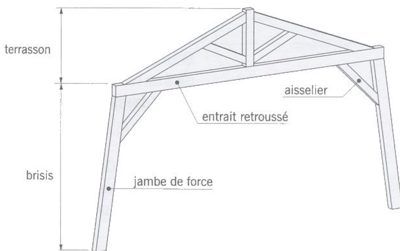
fig. 5.9 ferme à la Mansart
