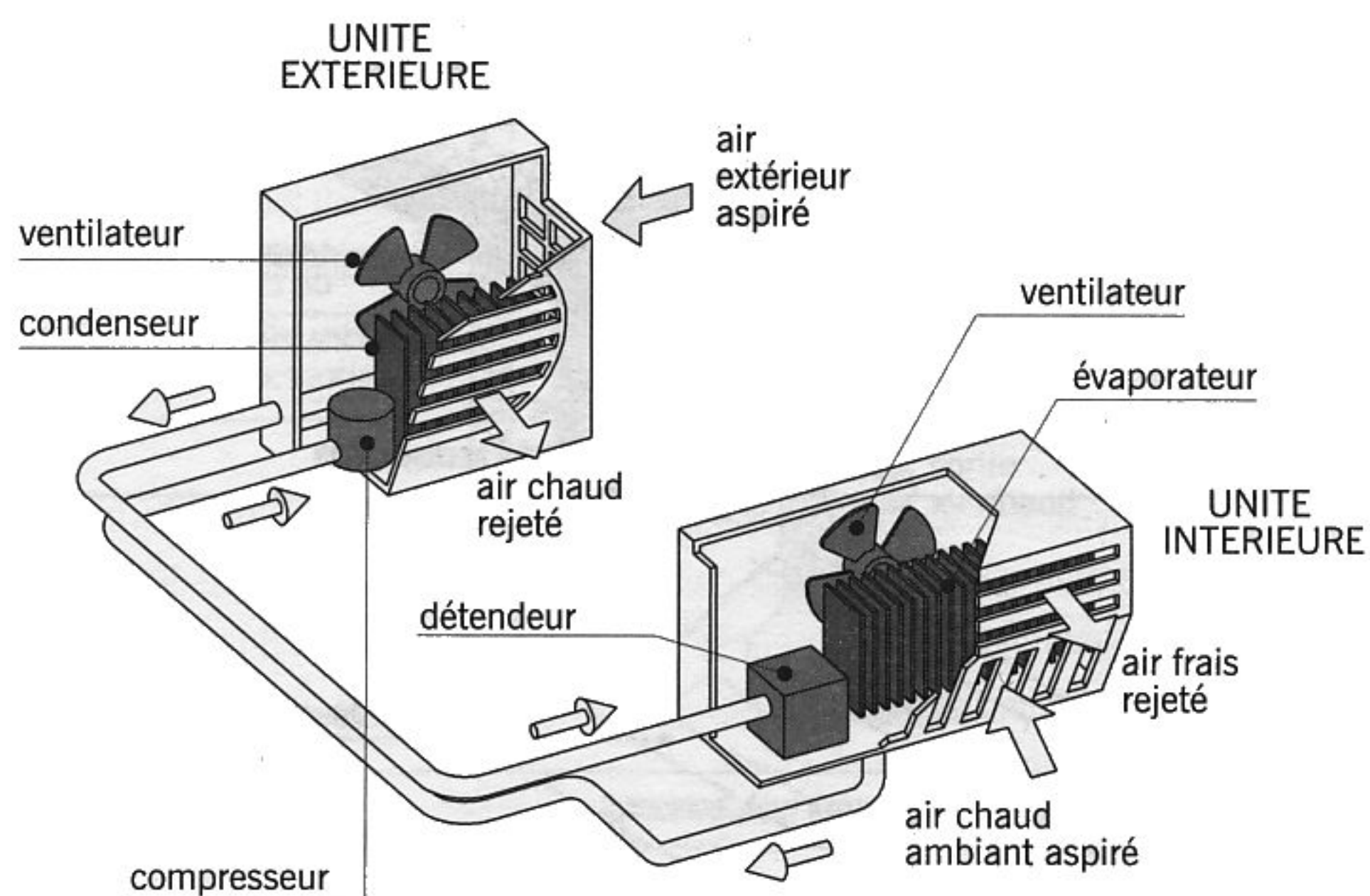
fig. 17.16 principe de fonctionnement d'un climatiseur bi-bloc
