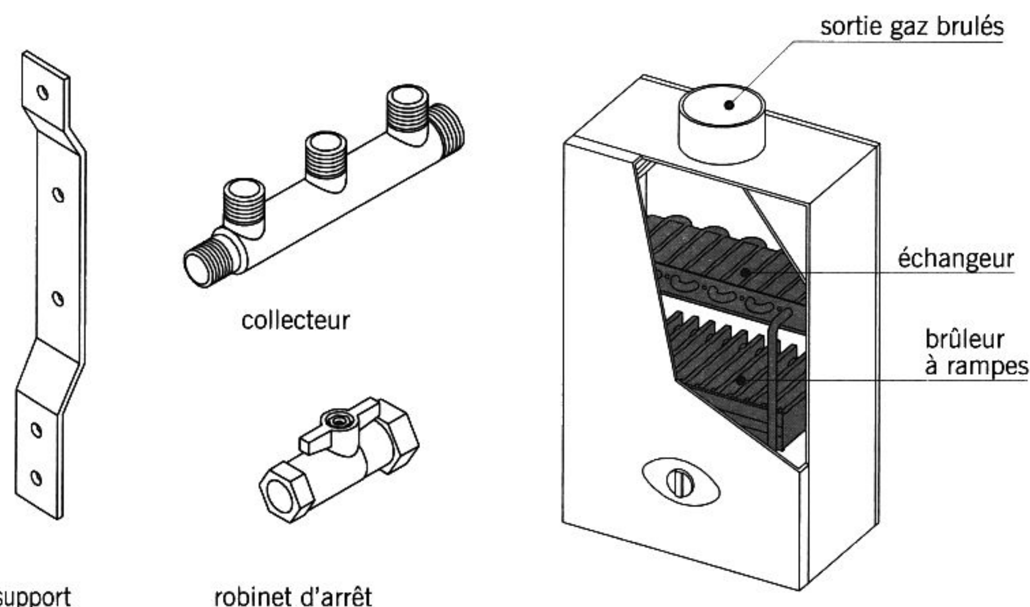
fig. 14.7 accessoires pour tubes PER
