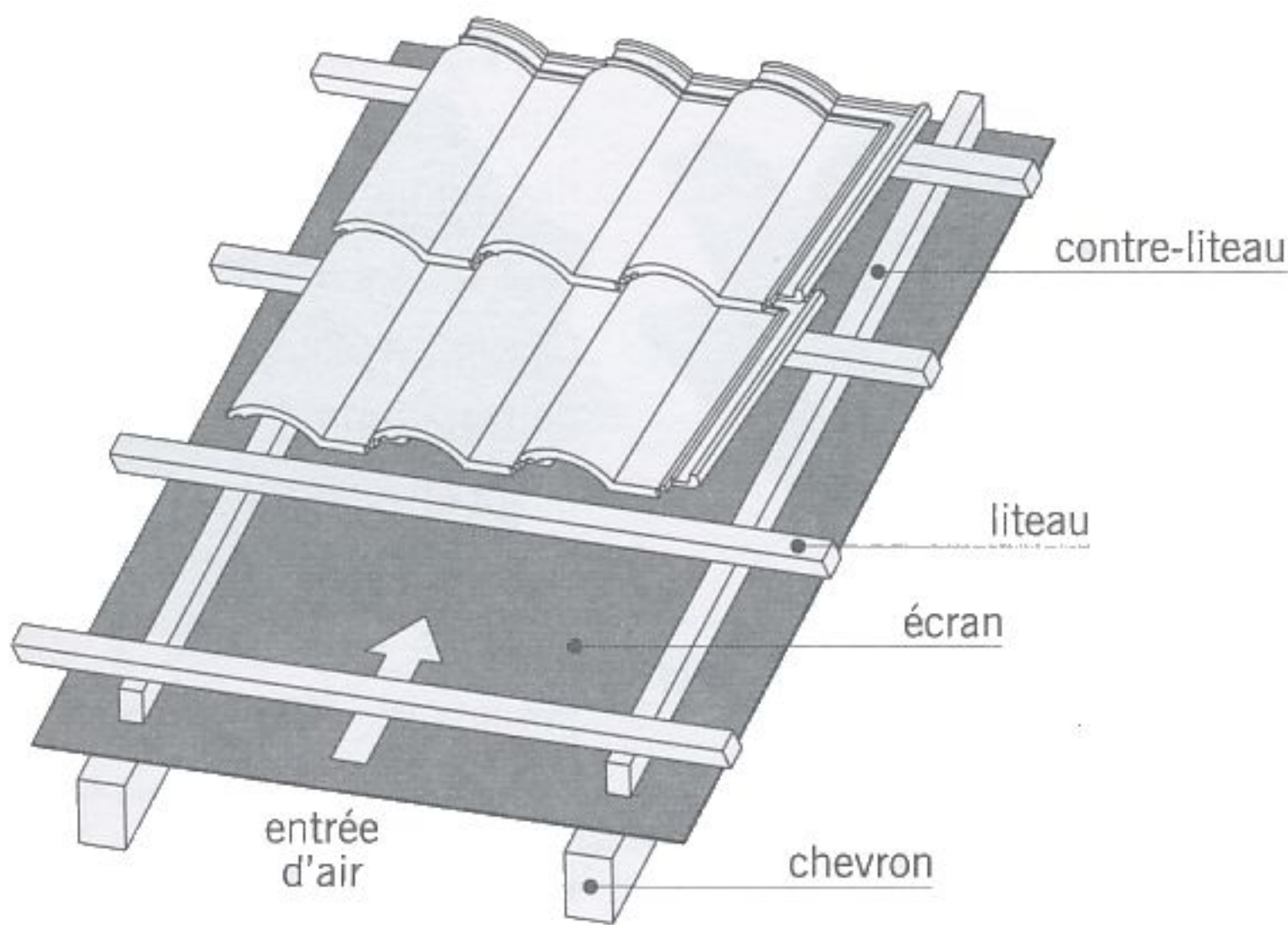
fig. 7.8 écran souple tendu
