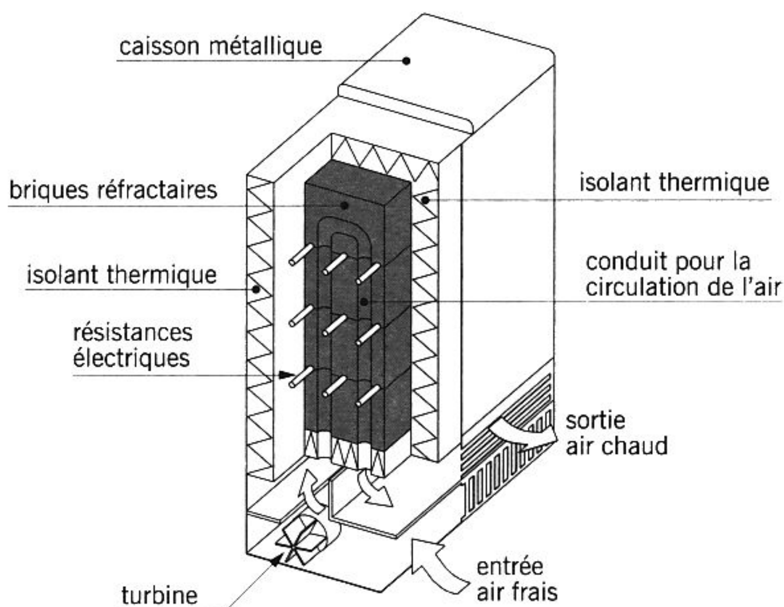
fig. 17.9 accumulateur dynamique
