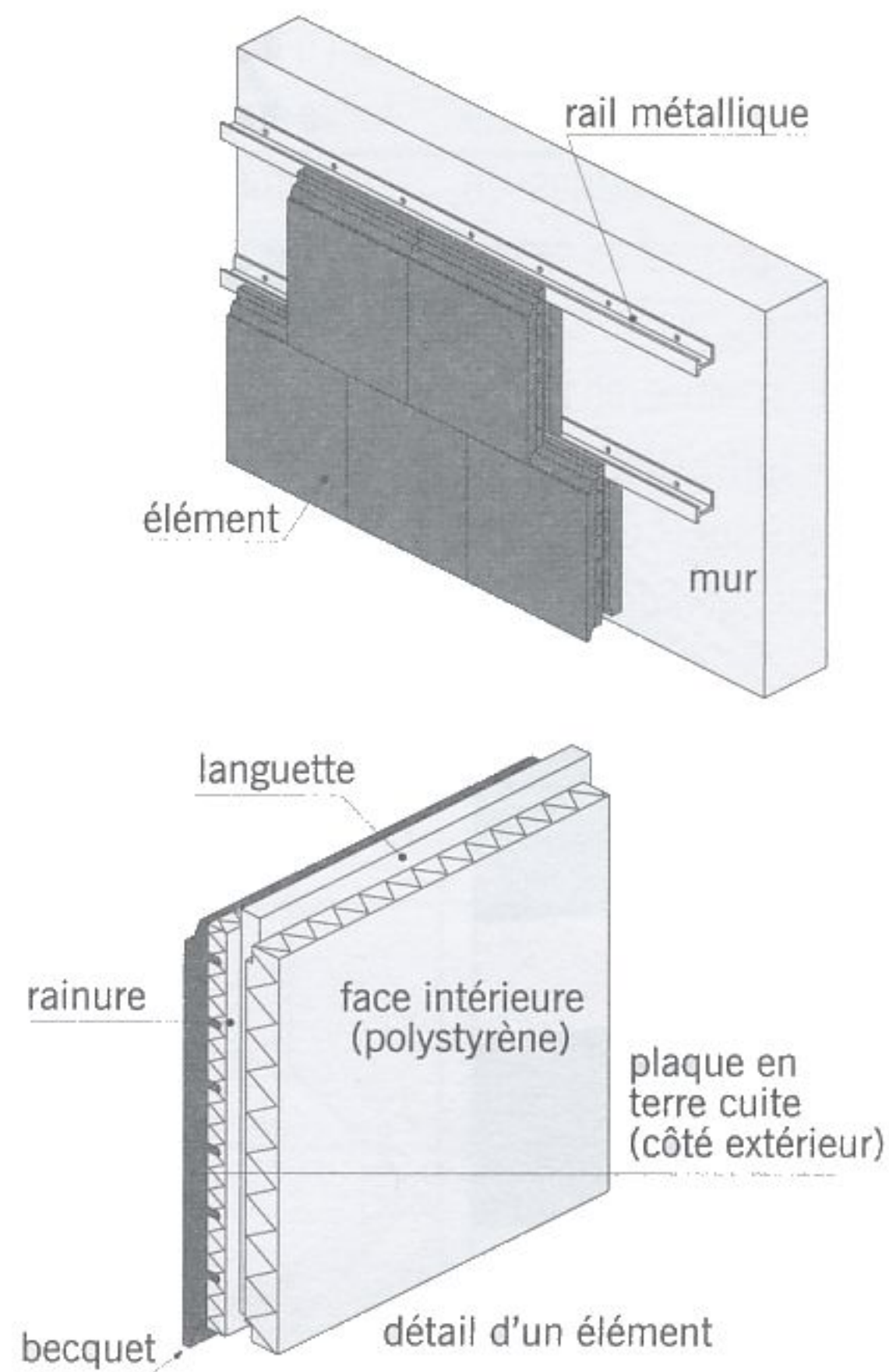
fig. 3.44 vêtture en terre cuite
