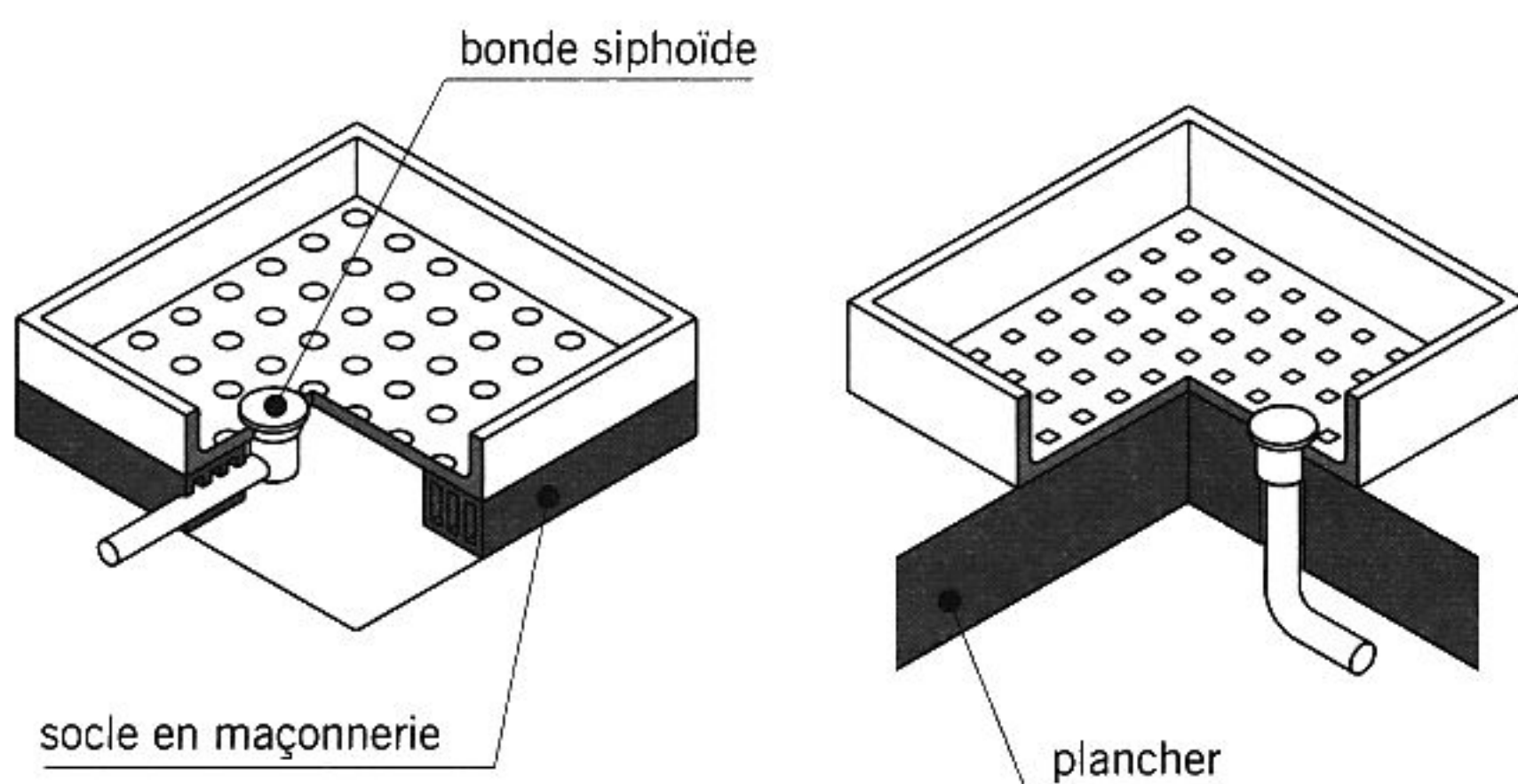
fig. 14.19 receveur à poser
