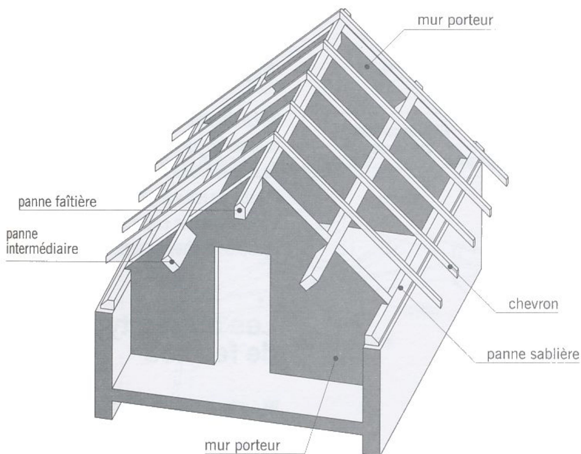
fig. 5.1 pannes reposant sur des murs porteurs
