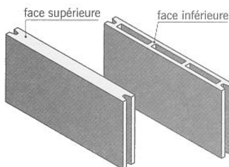
fig. 3.6 planelle
