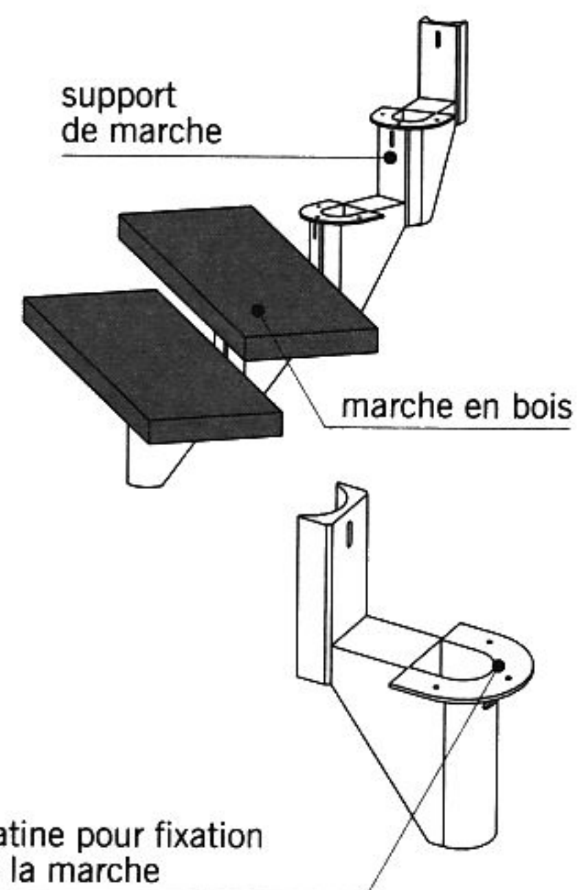
fig. 13.33 escalier à supports métalliques orientables
