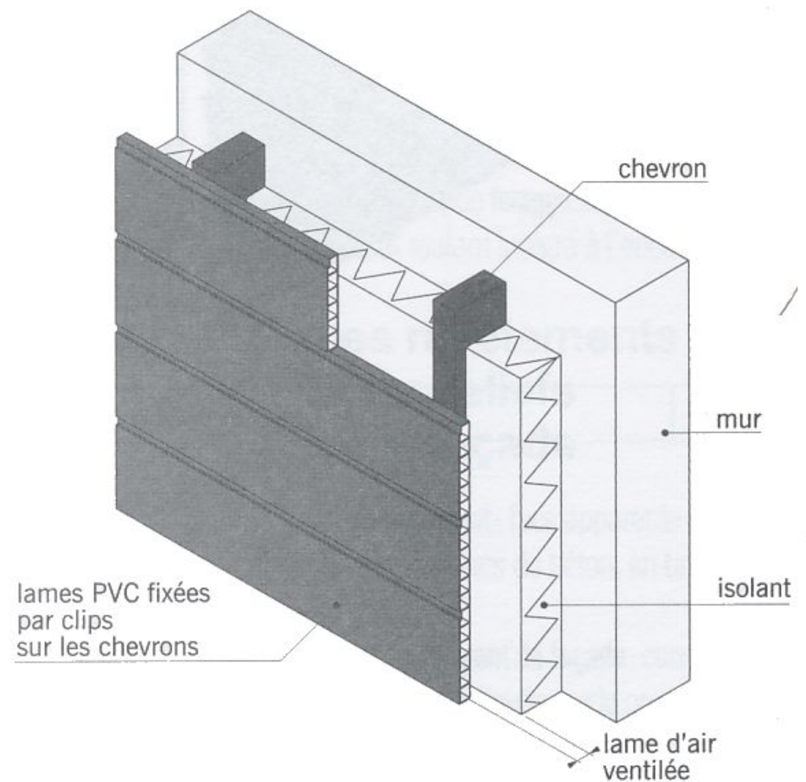
bardage en lames PVC
