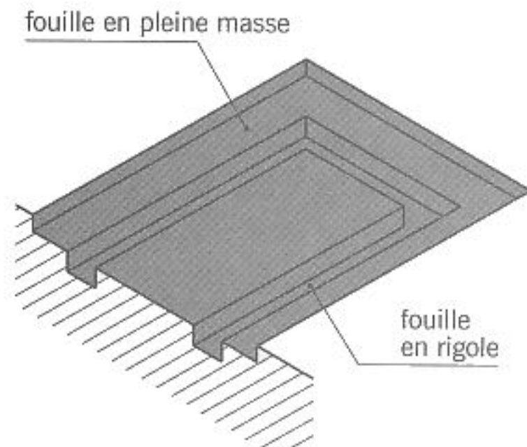
fig. 2.1 fouille
