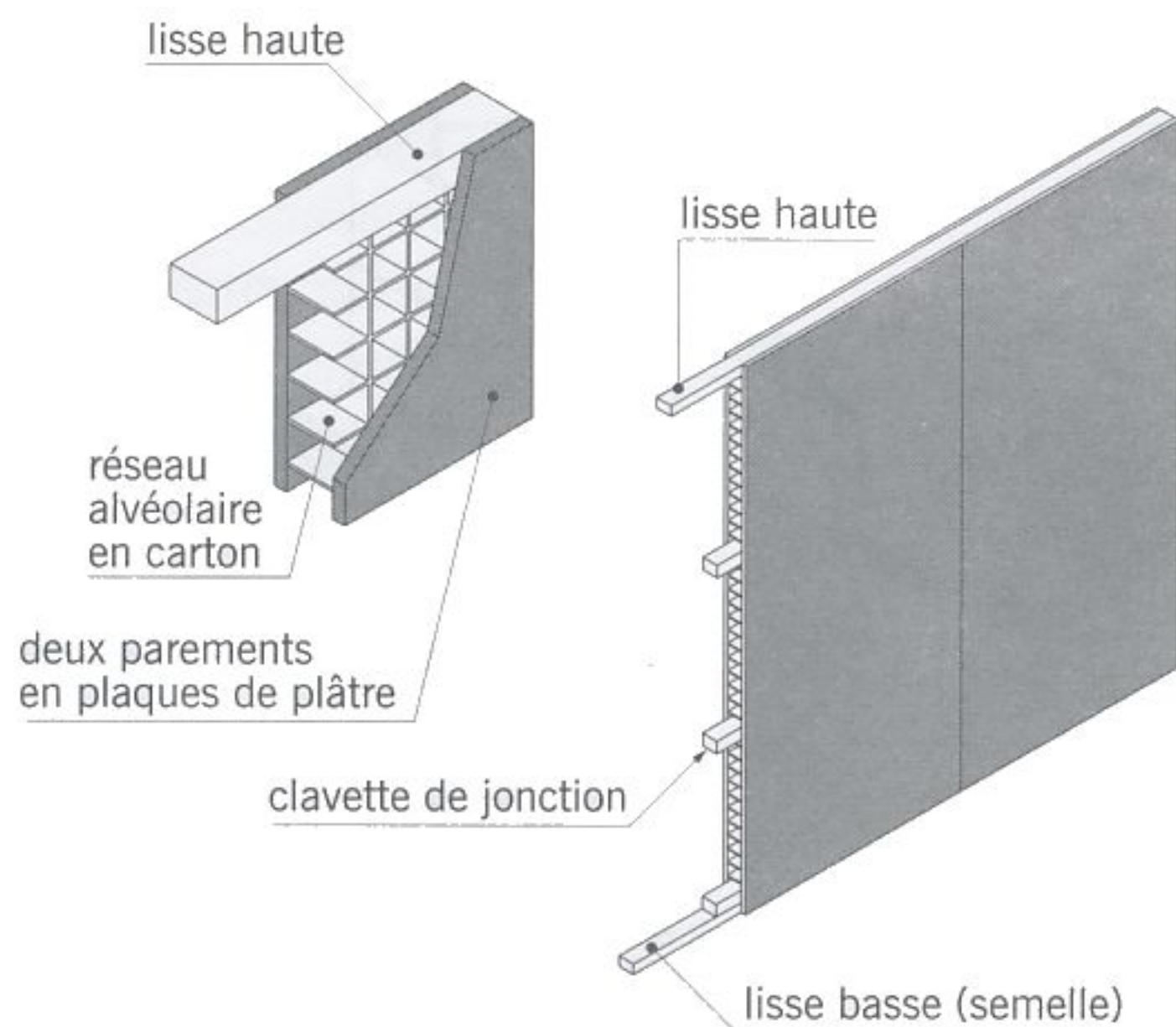
fig. 8.6 cloison sèche en panneaux à âme alvéolaire
