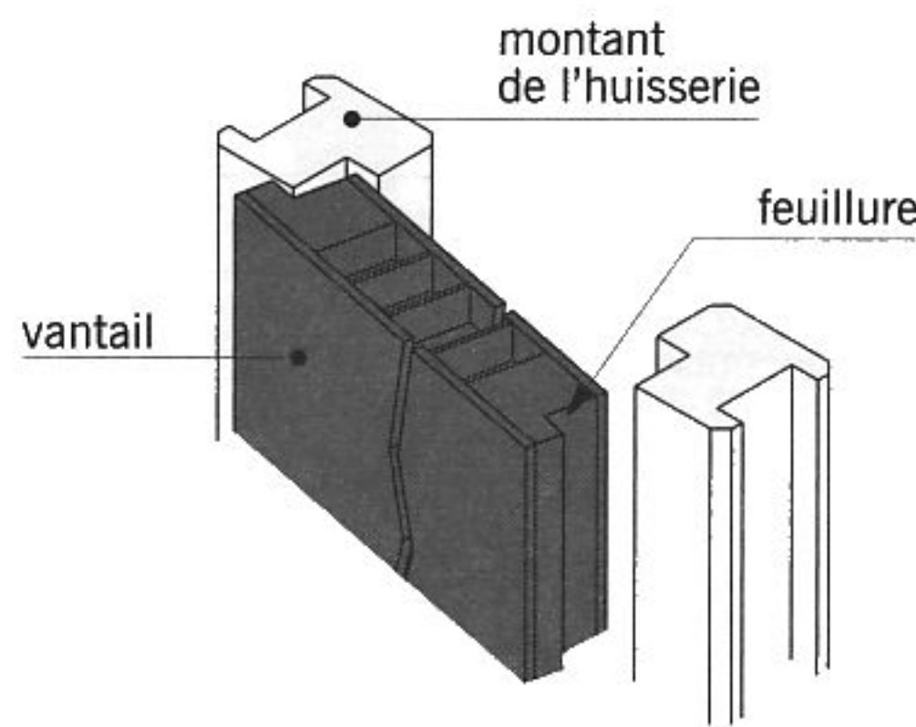
fig. 12.10 porte à recouvrement
