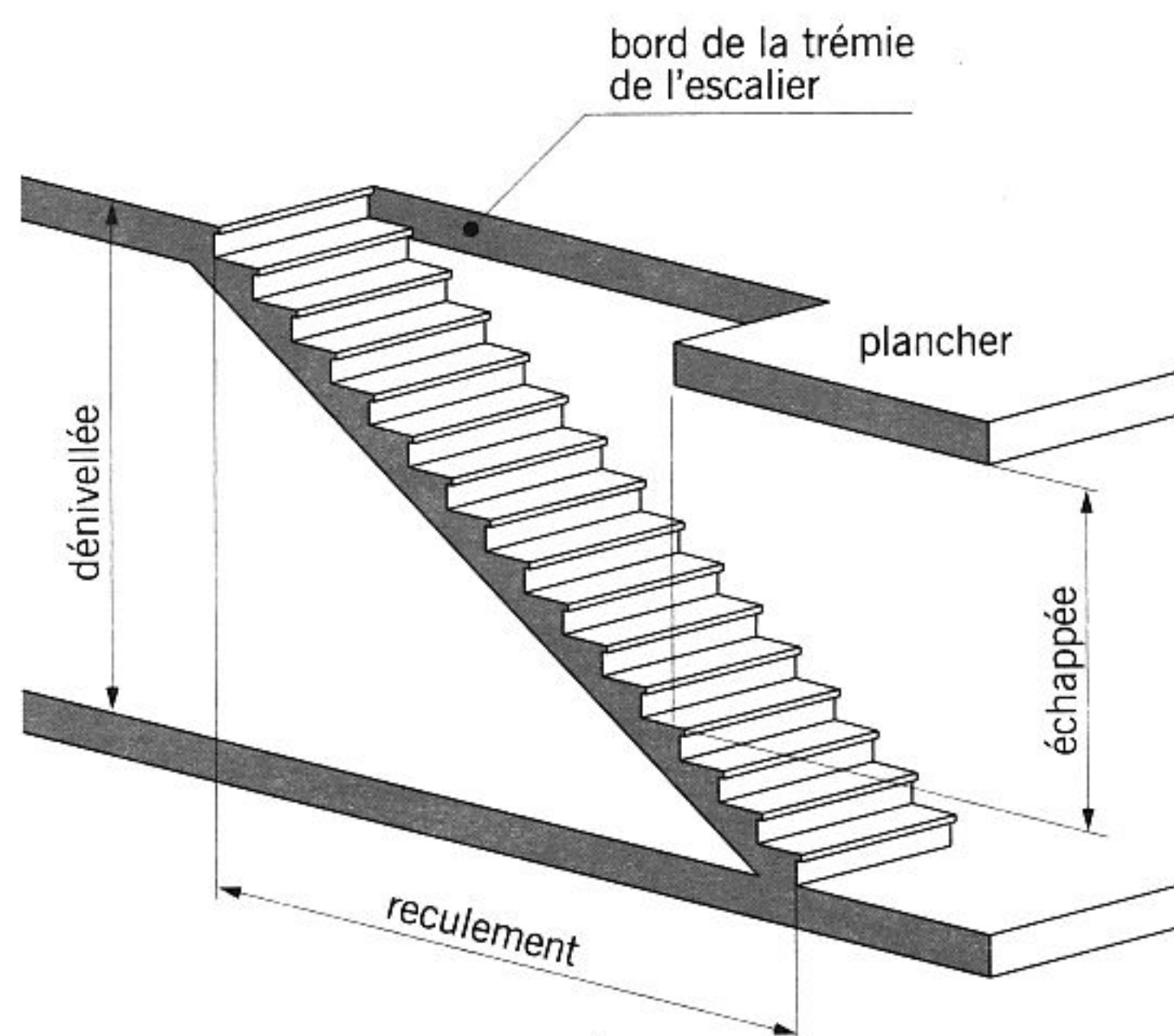
volée et trémie de l'escalier
