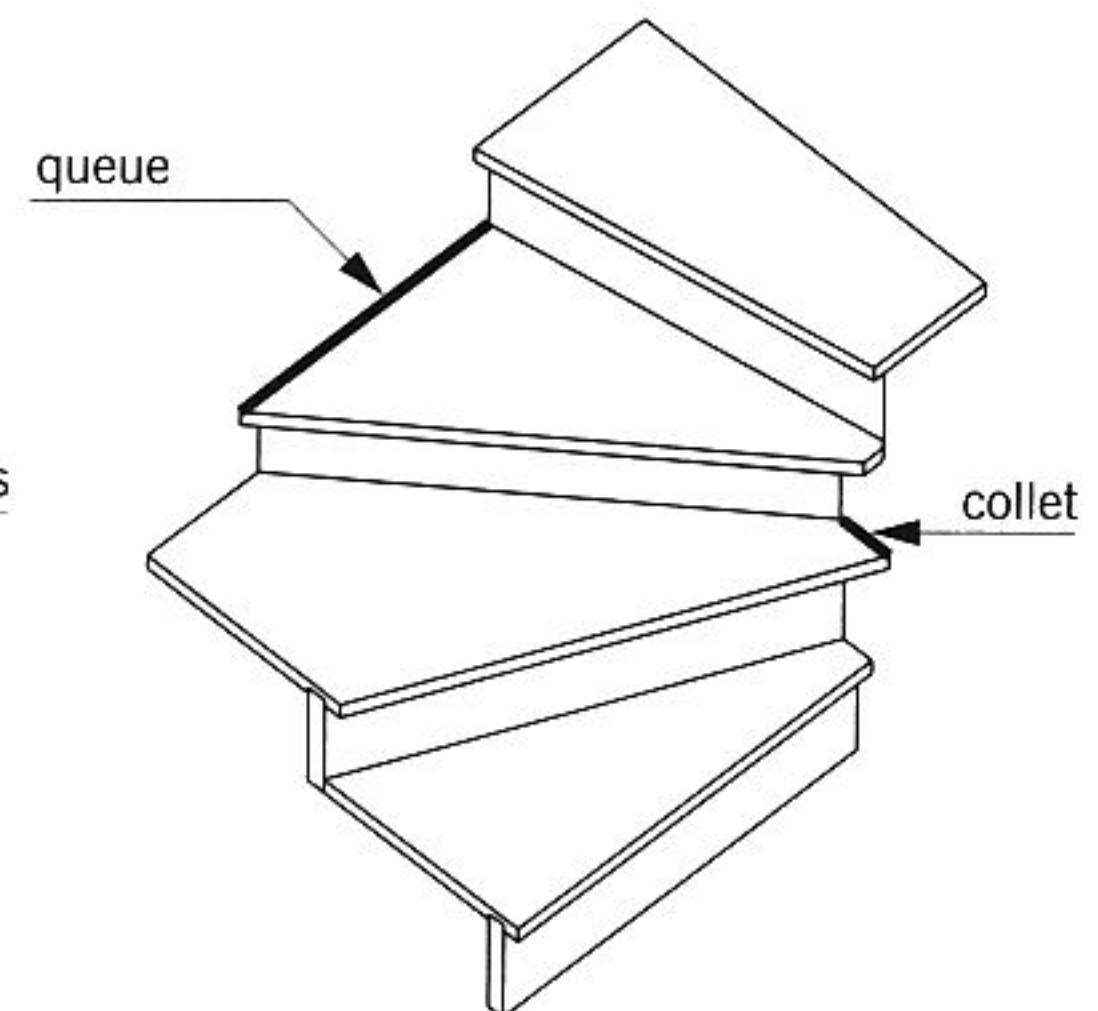
fig. 13.18 queue et collet
