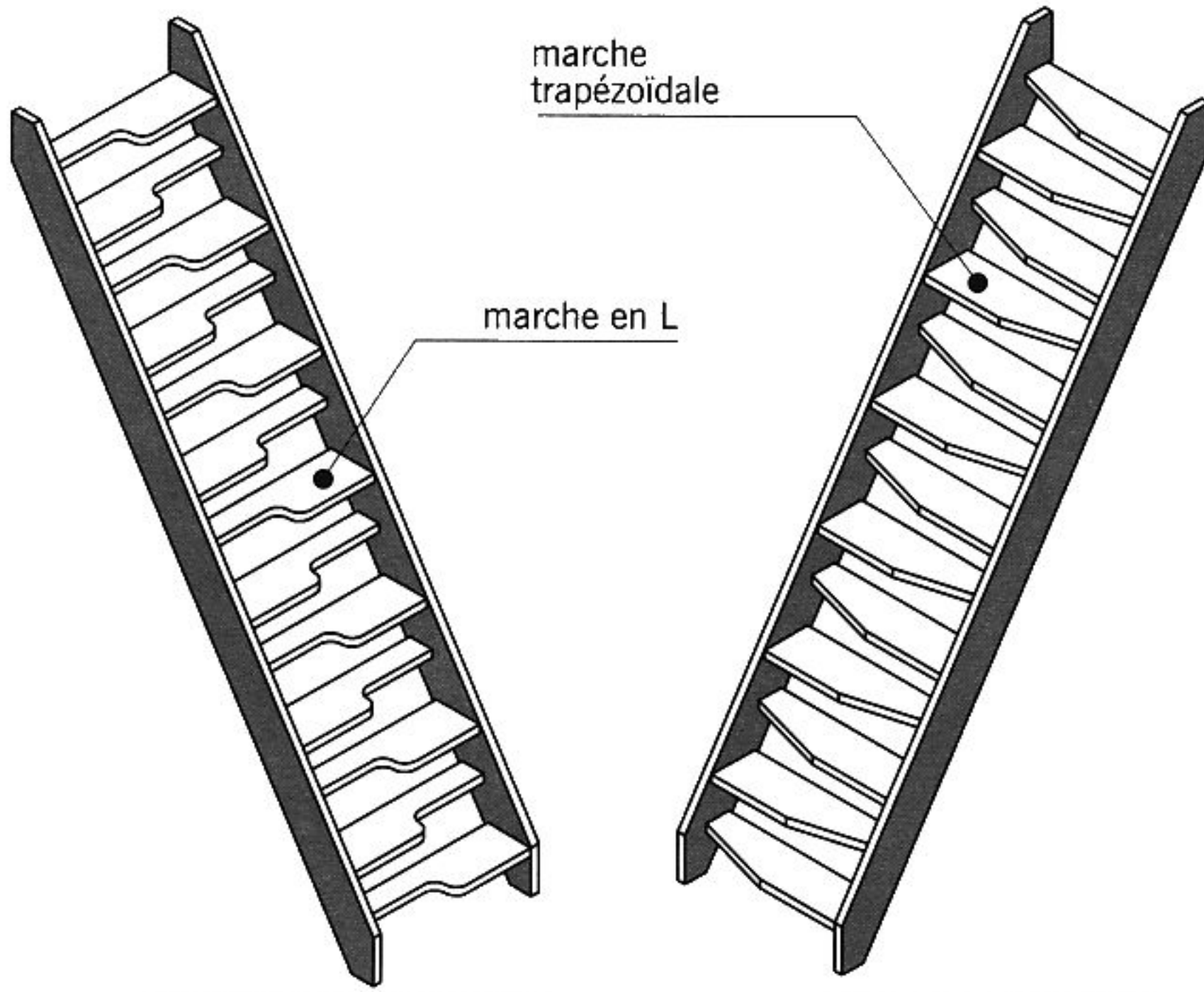
fig. 13.21 échelles à pas décalés
