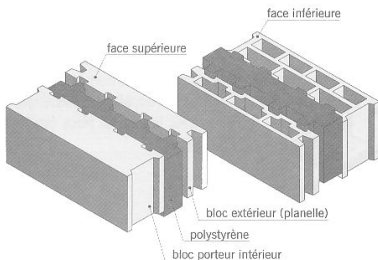
fig. 3.13 bloc à isolation intégrée
