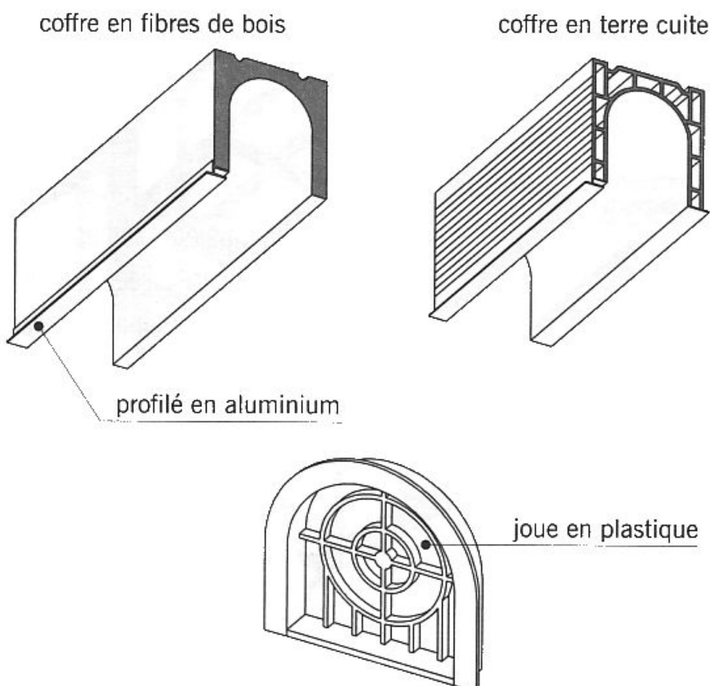
fig. 11.65 coffres de volet roulant
