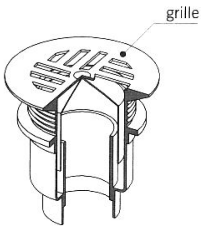
fig. 15.8 bonde siphonide pour receveur de douche
