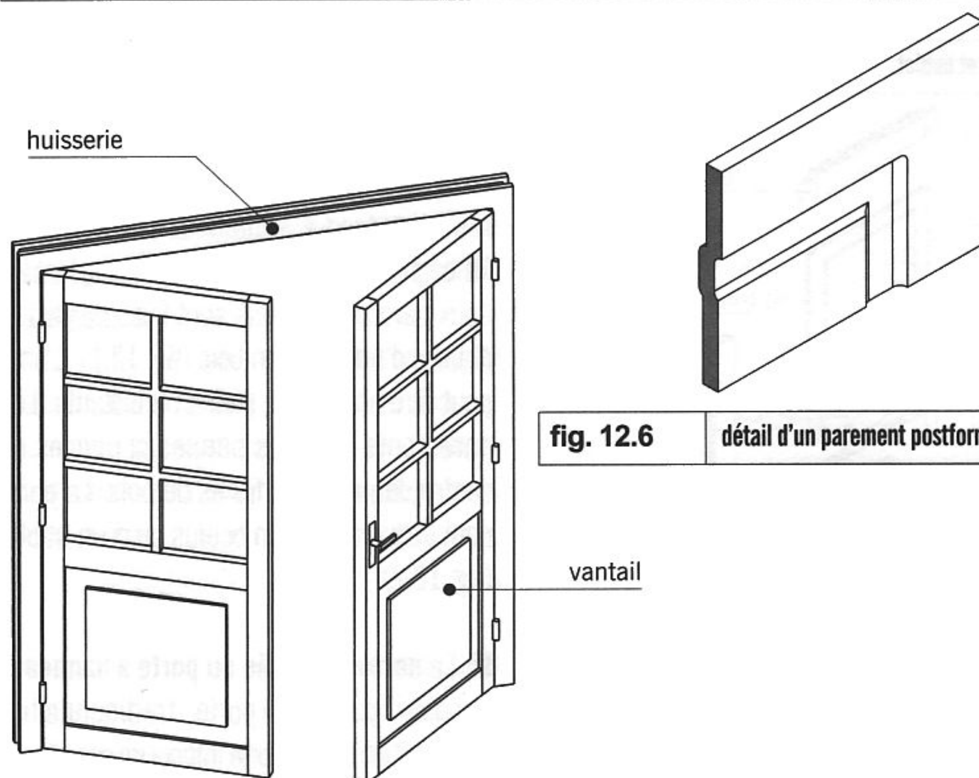
fig. 12.7 bloc-porte
