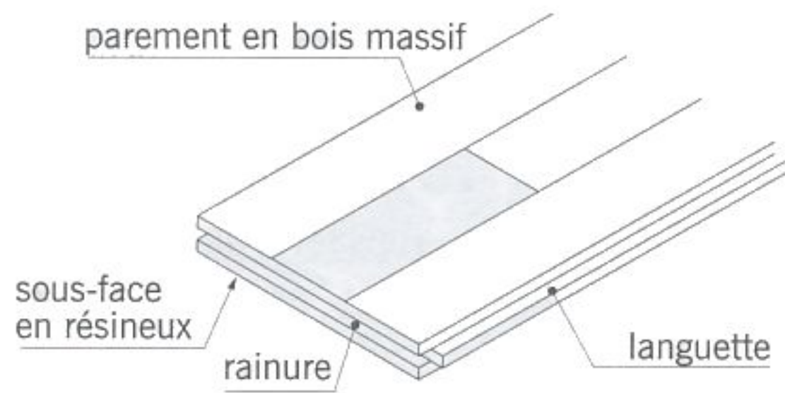
fig. 10.9 parquet en panneaux contre-collés (détail d'un élément)
