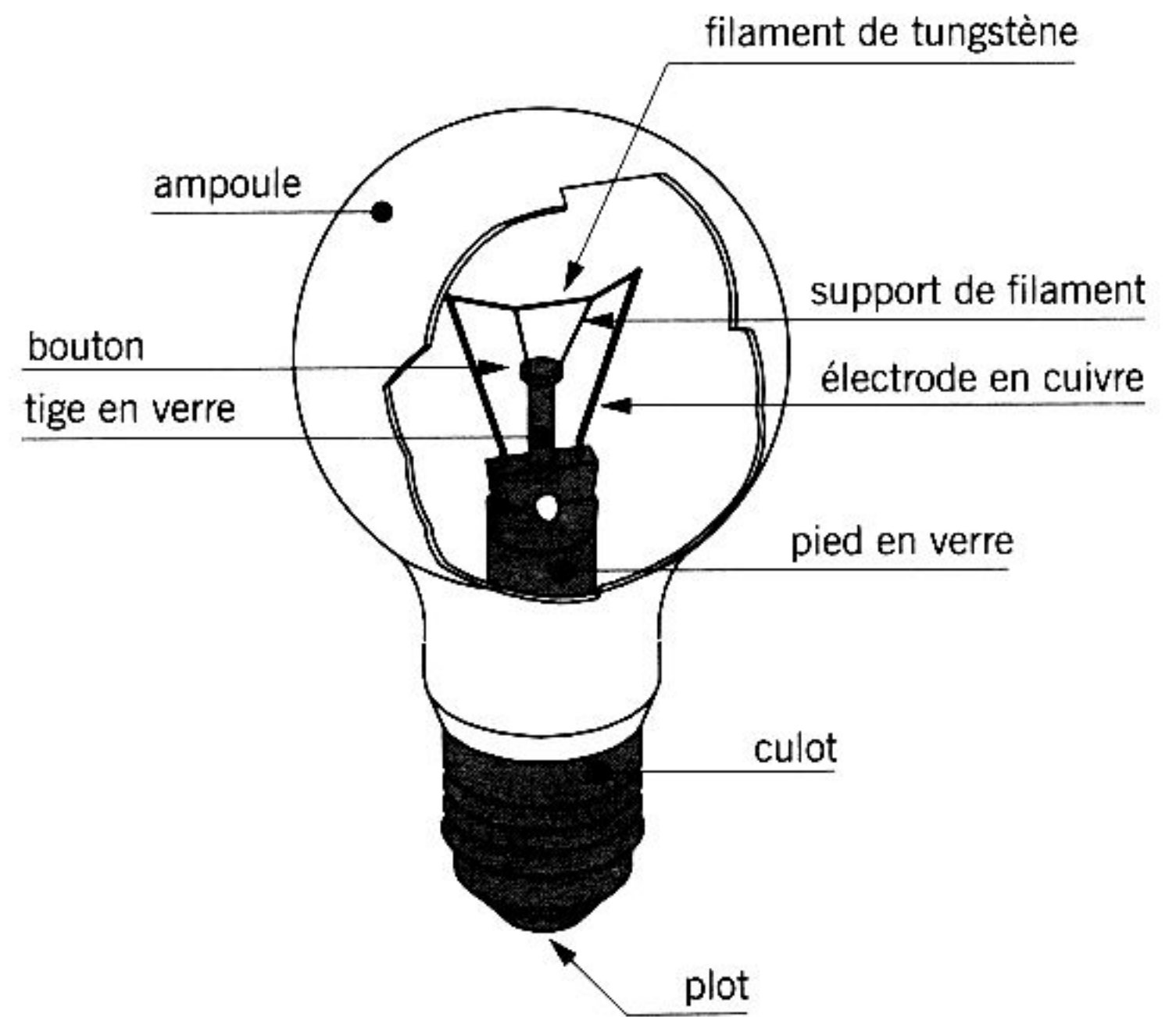
fig. 16.29 lampe à incandescence
