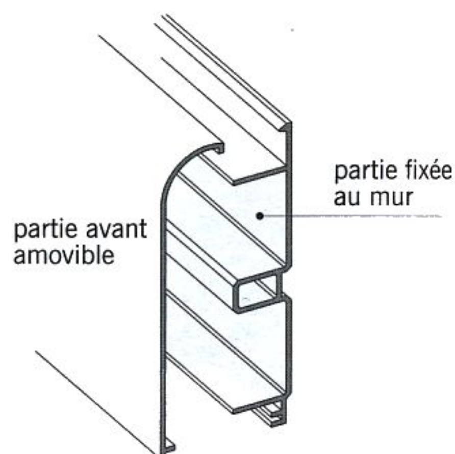
fig. 16.14 plinthe en PVC
