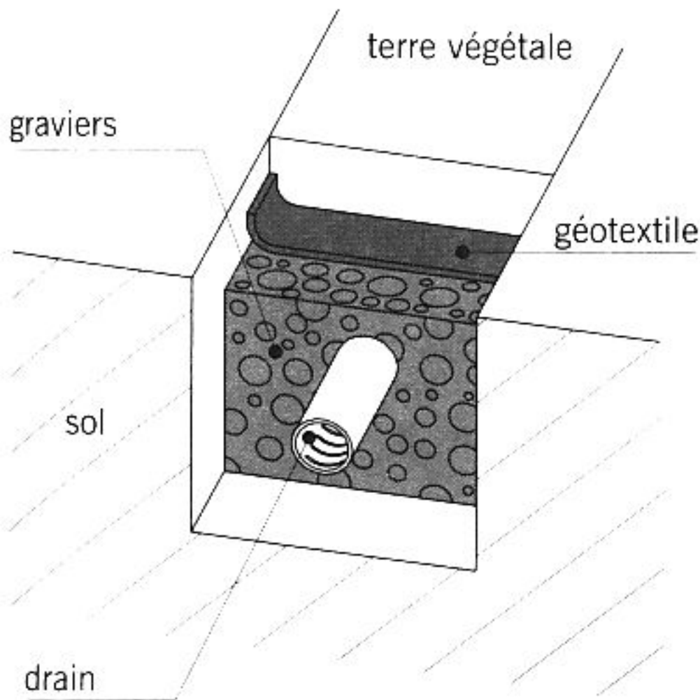
fig. 15.17 détail d'une tranchée d'infiltration
