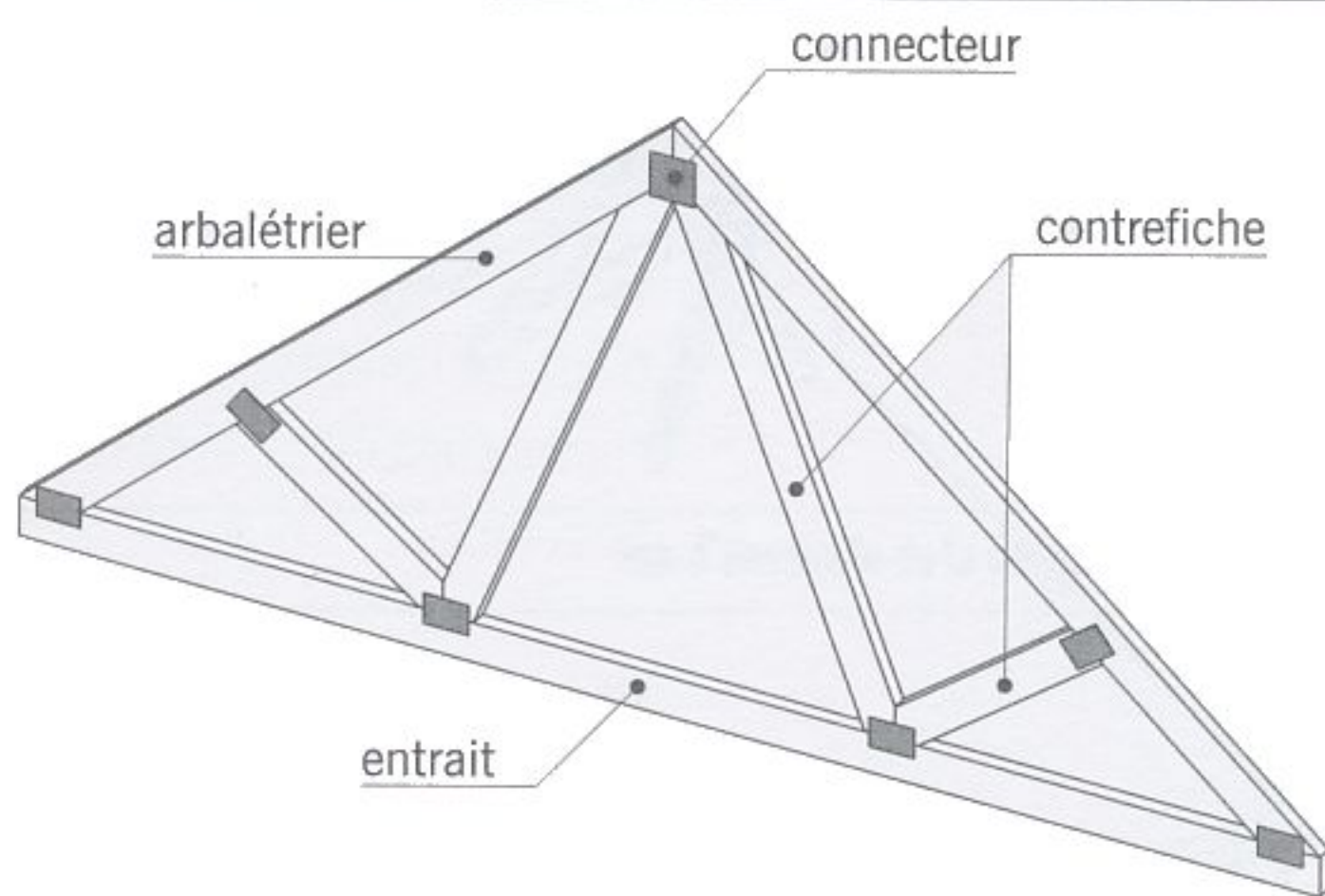
fig. 5.15 éléments constitutifs d'une ferme
