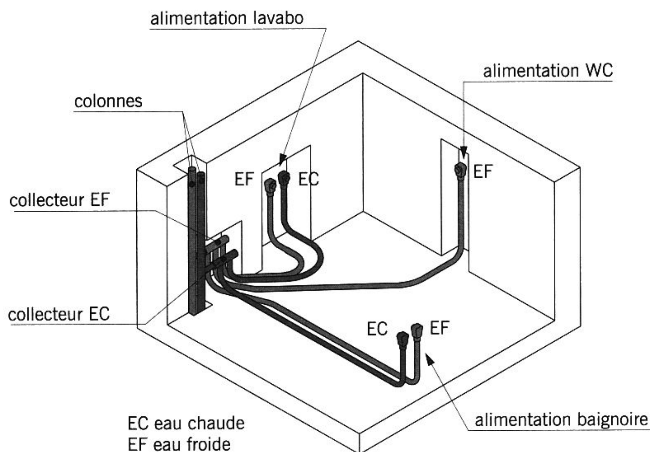
fig. 14.4 exemple d'hydrodistribution par piquages (robinetteries, appareils sanitaires non représentés)
