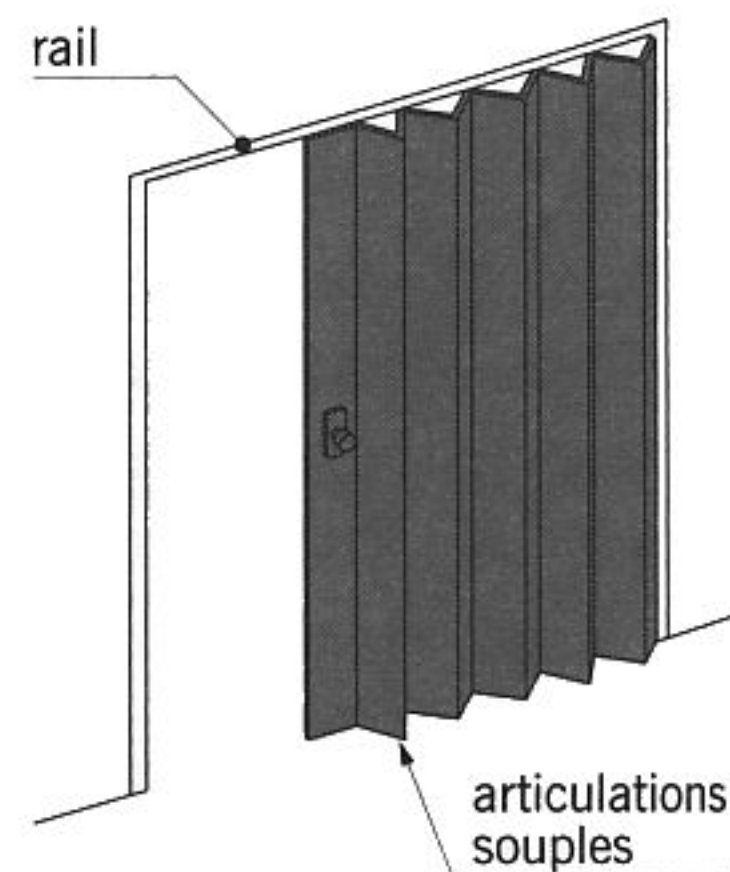
fig. 12.16 porte extensible
