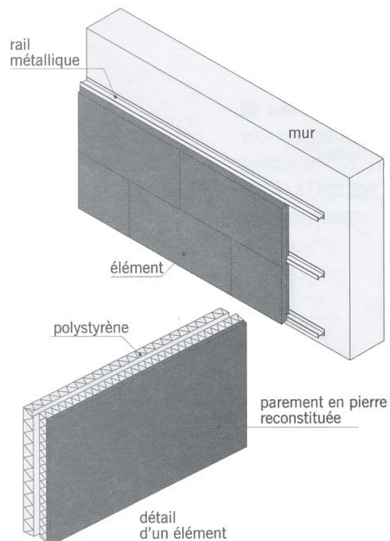
vêtture en pierre reconstituée
