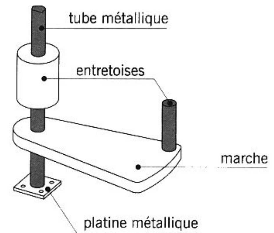
fig. 13.25 détail d'un escalier hélicoïdal
