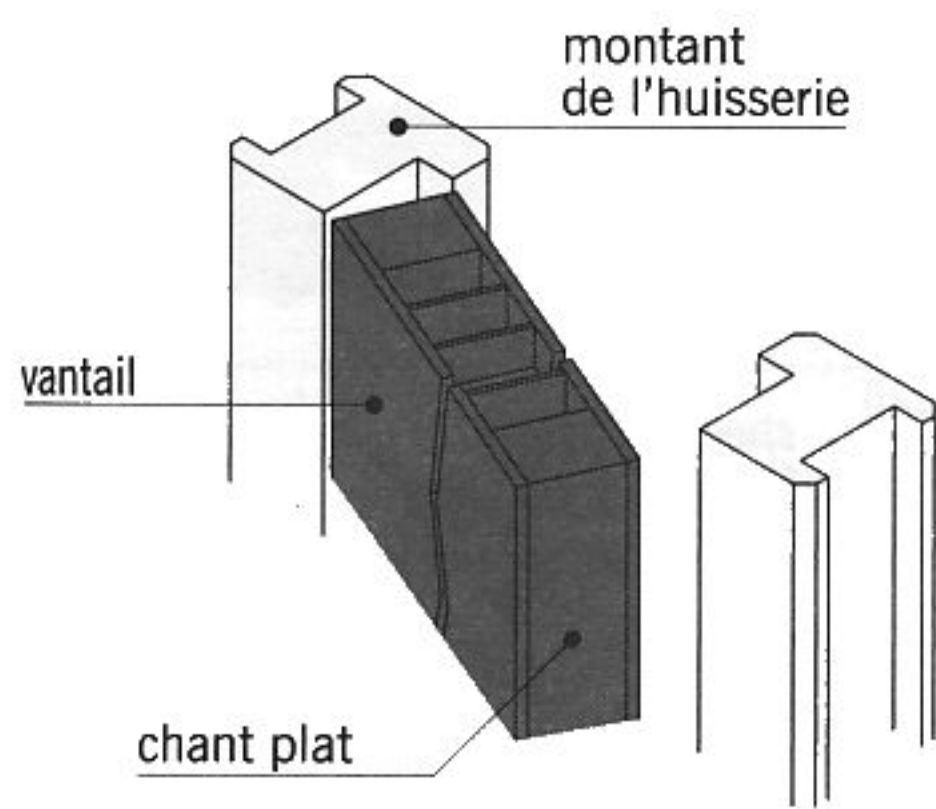
fig. 12.9 porte à chant plat
