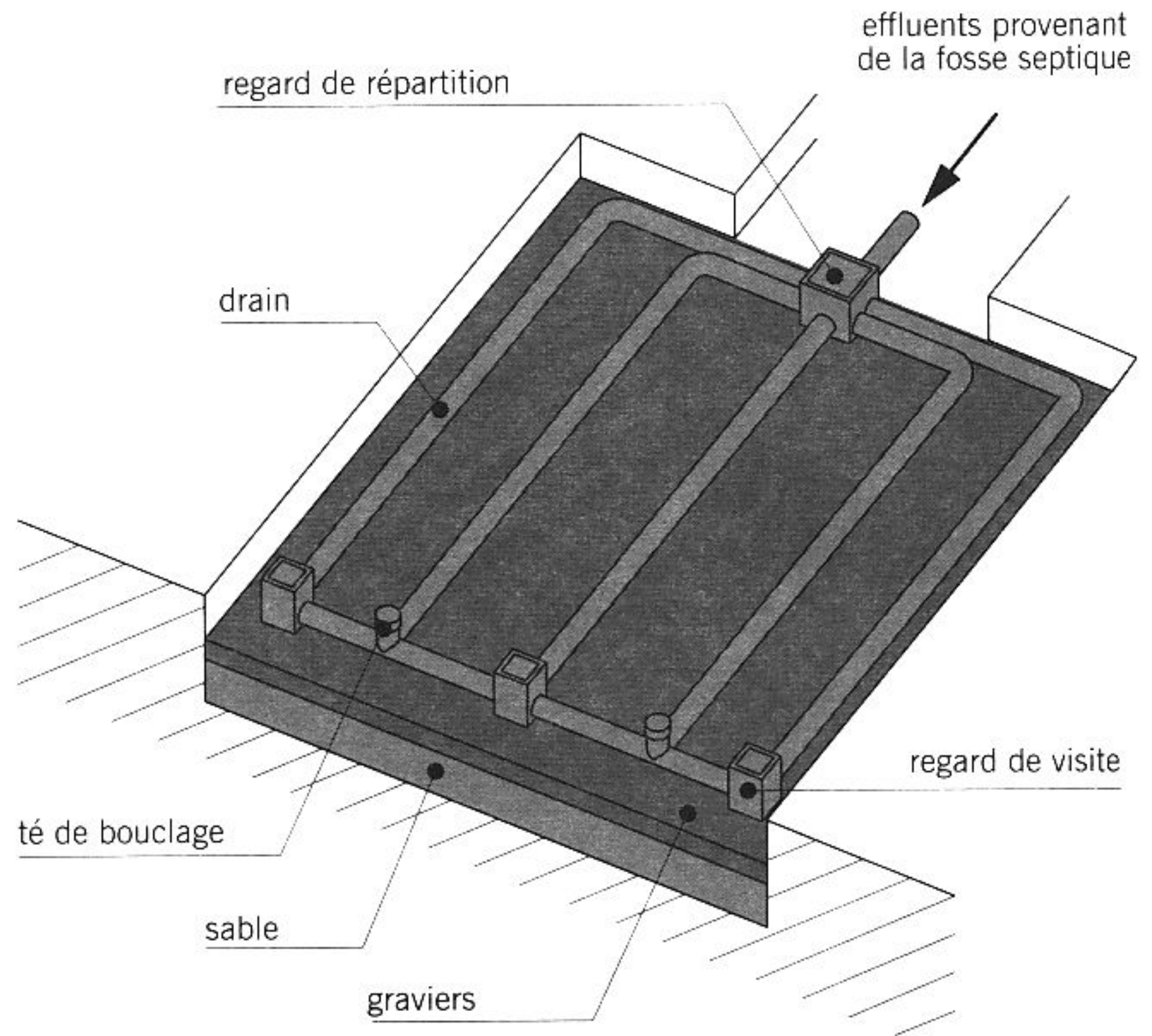
fig. 15.19 filtre à sable vertical non drainé
