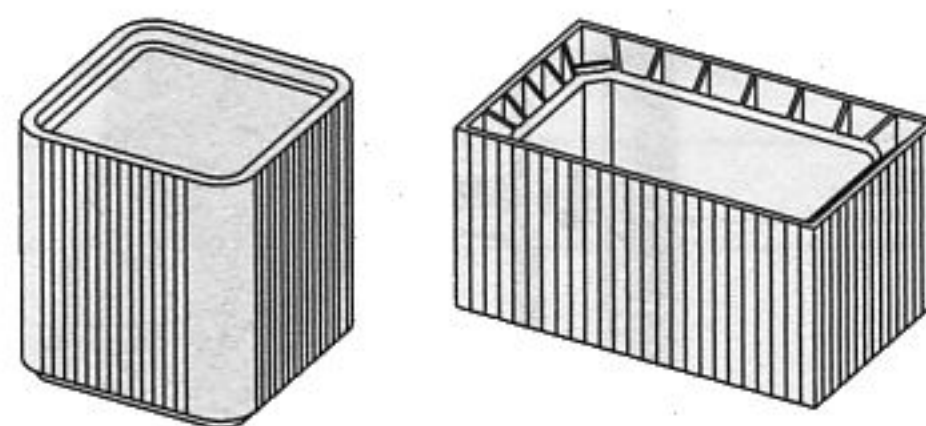
boisseau à parois pleines boisseau à parois alvéolées
