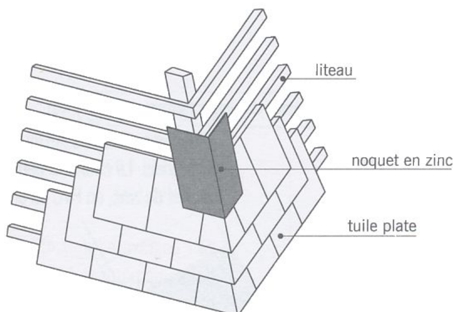
fig. 7.49 noquet sur arêtier en tuiles plates
