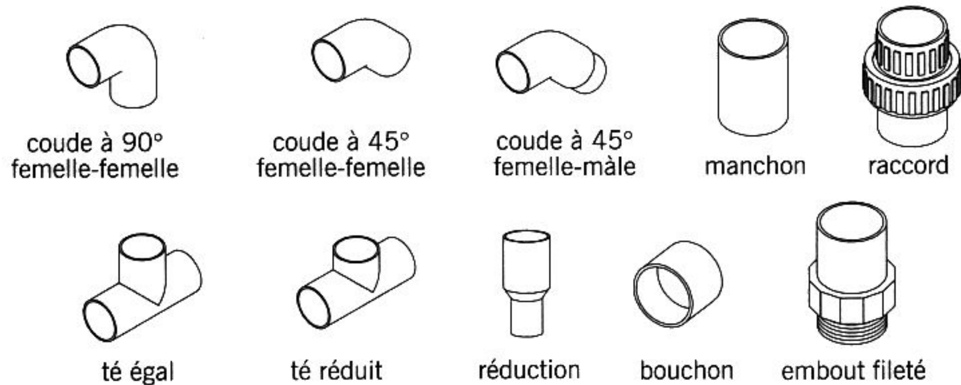
fig. 14.3 raccords et accessoires en PVC
