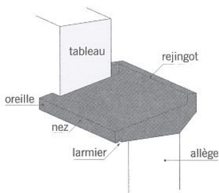
fig. 3.31 appui de baie
