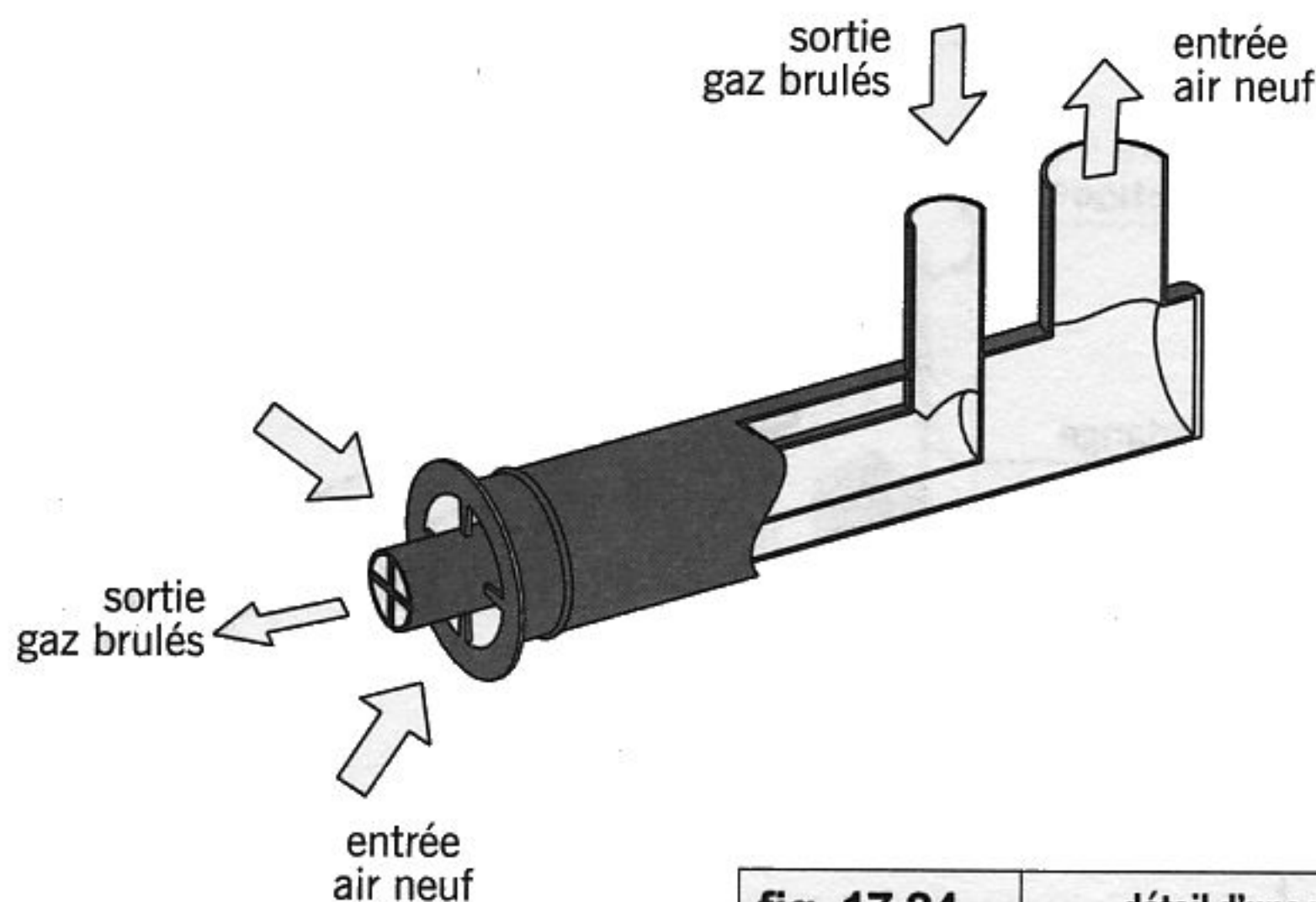
fig. 17.24 détail d'une ventouse
