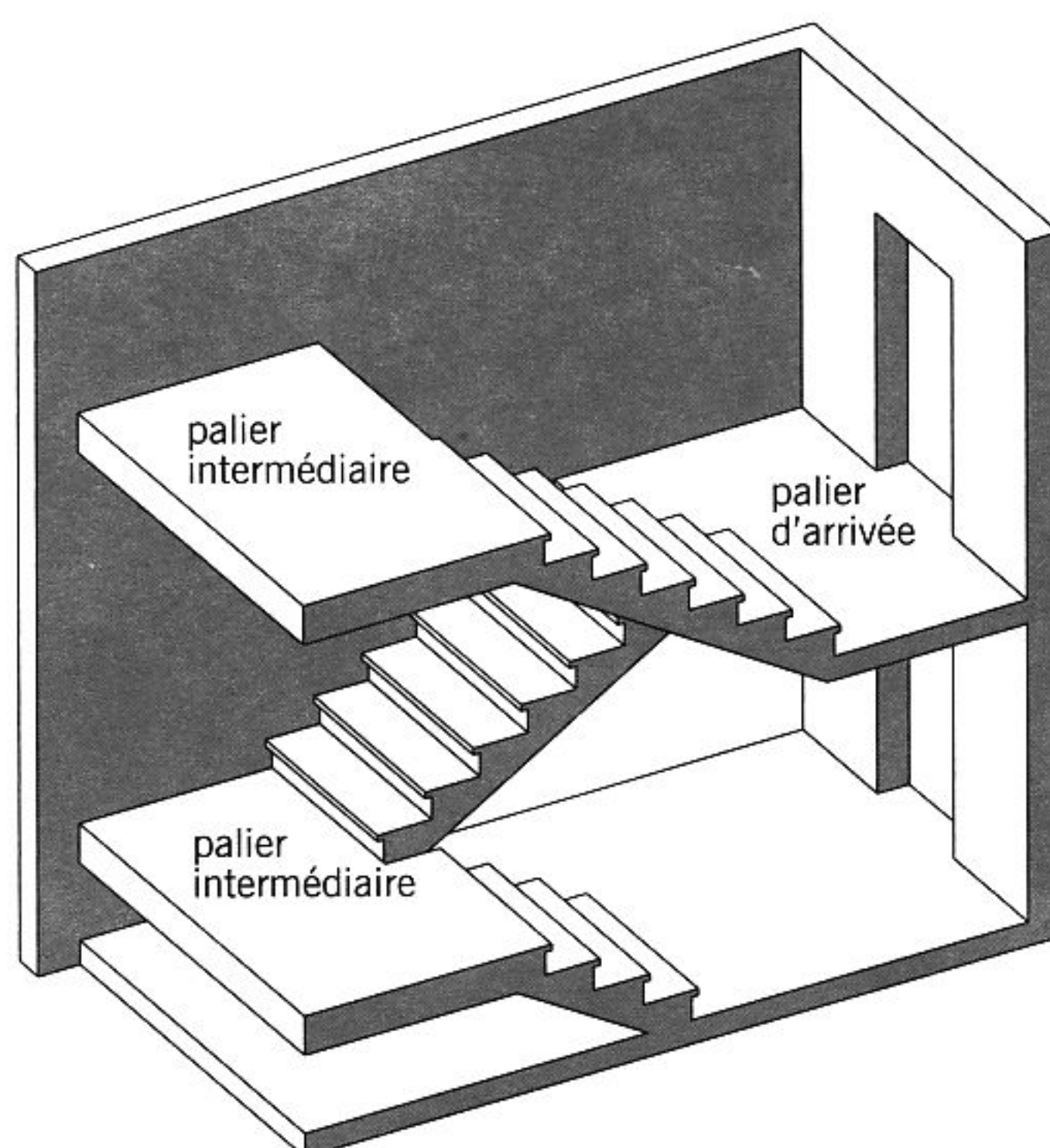
volées et paliers
