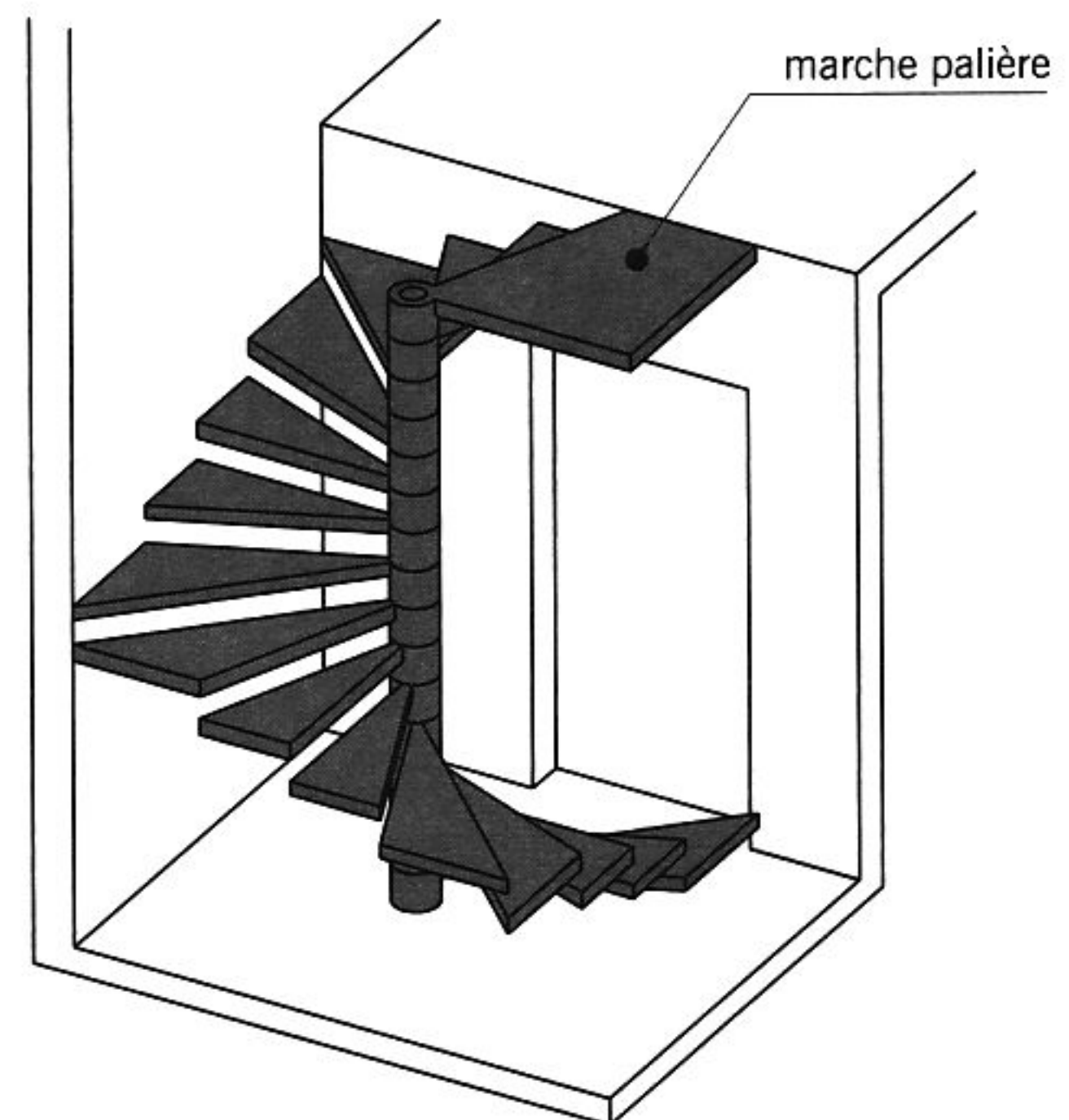
escalier hélicoïdal avec marches préfabriquées
