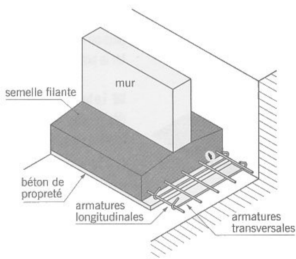
semelle filante fortement armée
