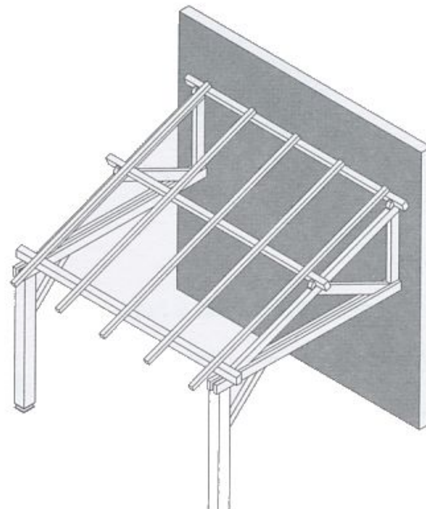
fig. 5.33 charpente d'appentis reposant sur un mur et deux poteaux
