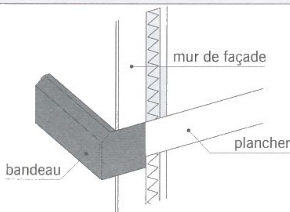
bandeau préfabriqué à agraffer
