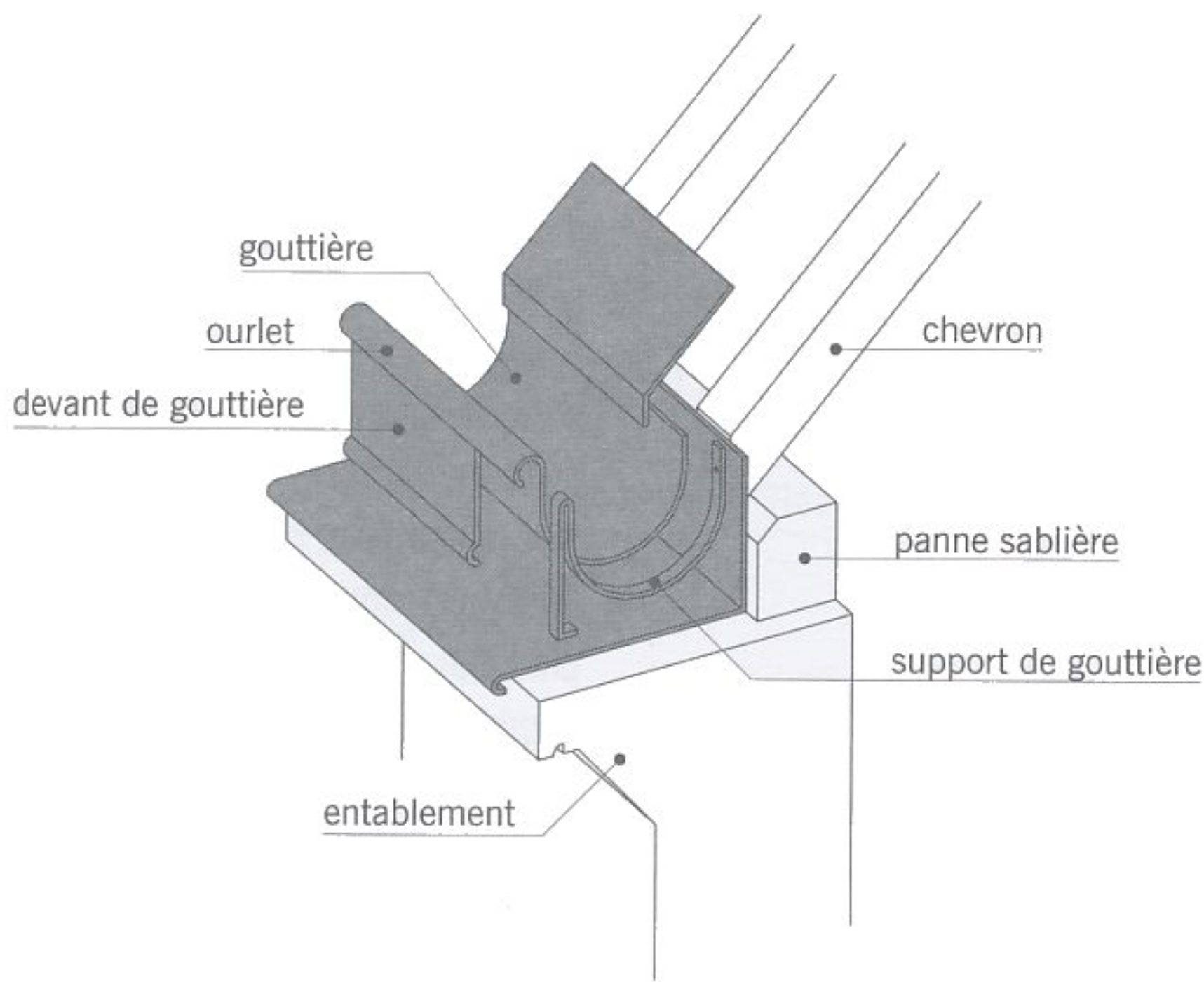
fig. 7.58 gouttière à l'anglaise (représentation simplifiée)
