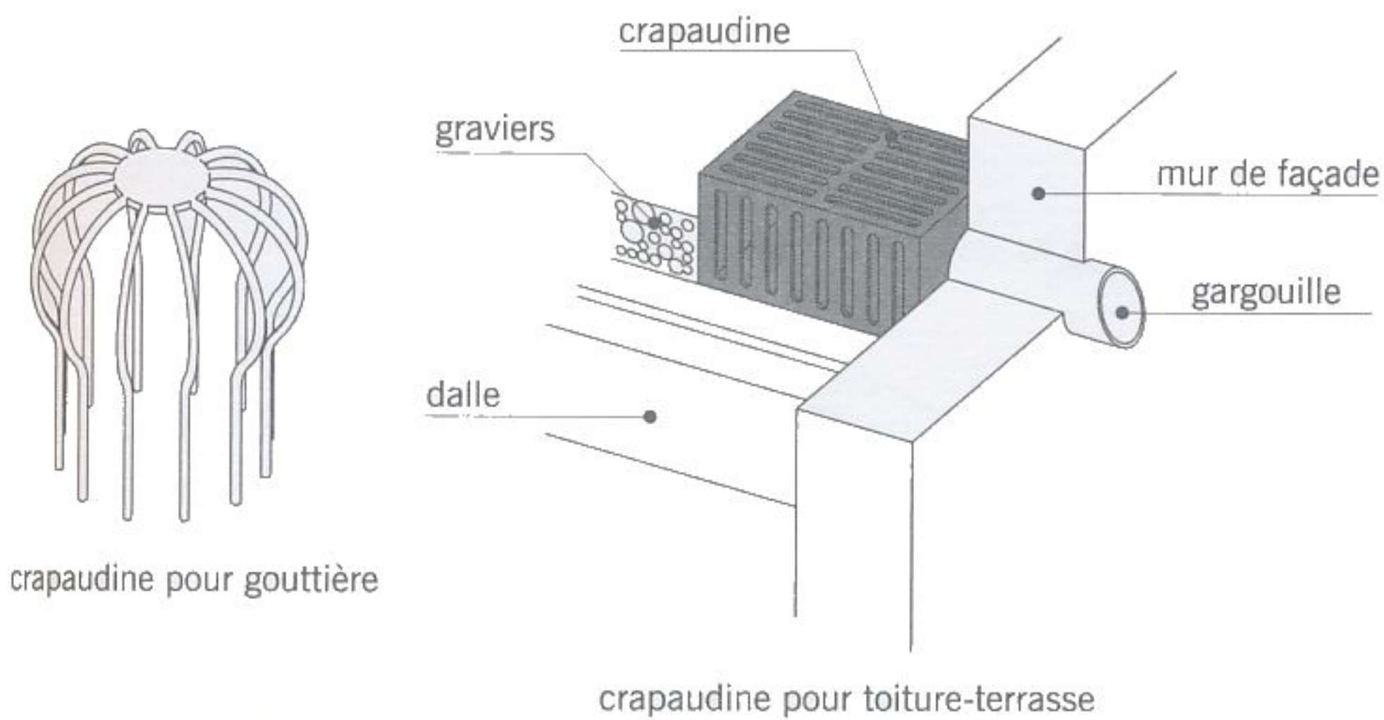
fig. 7.70 crapaudines
