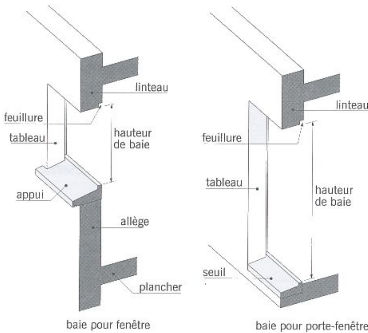
fig. 3.27 baies (1)
