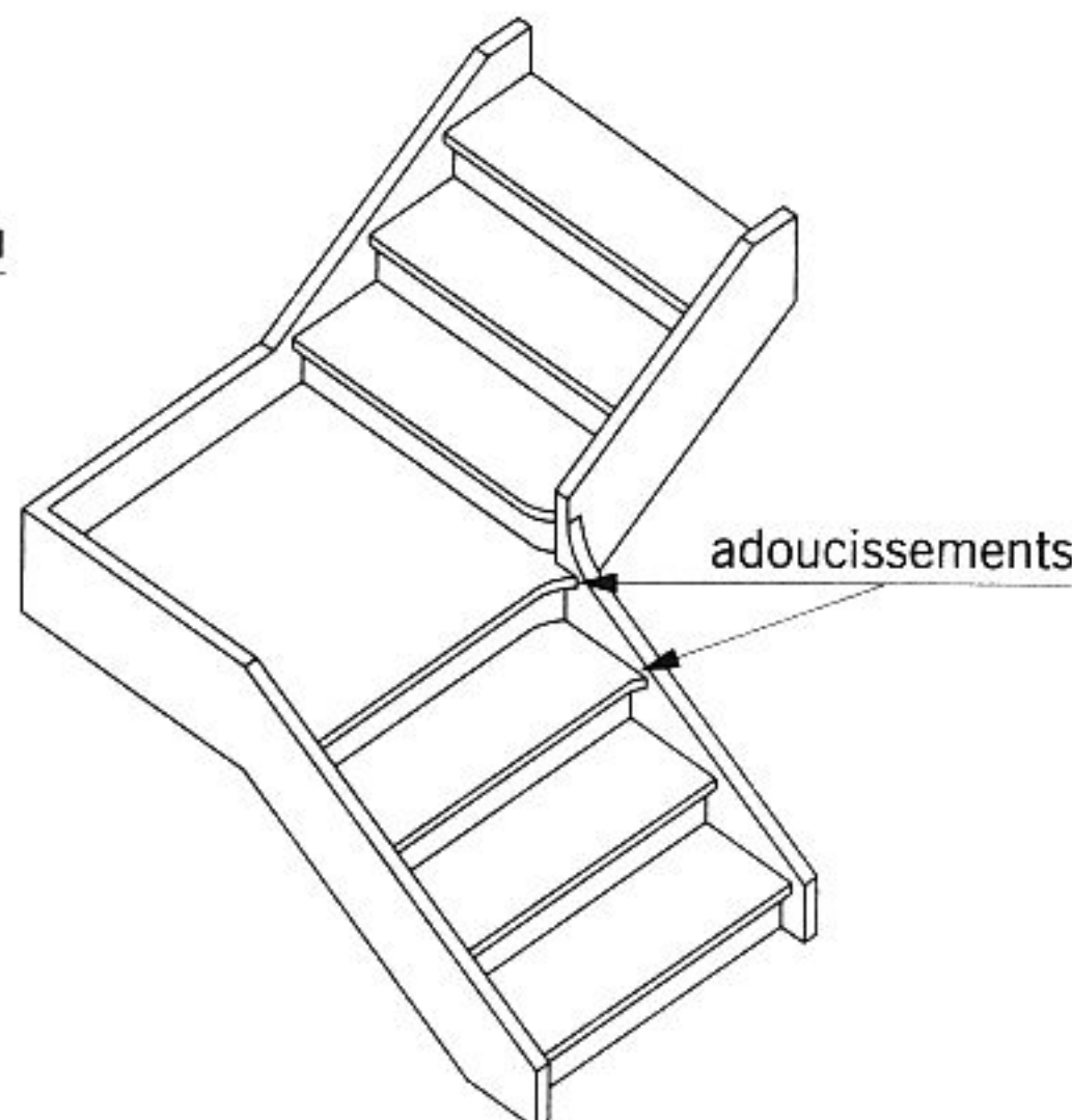
fig. 13.17 adoucissement
