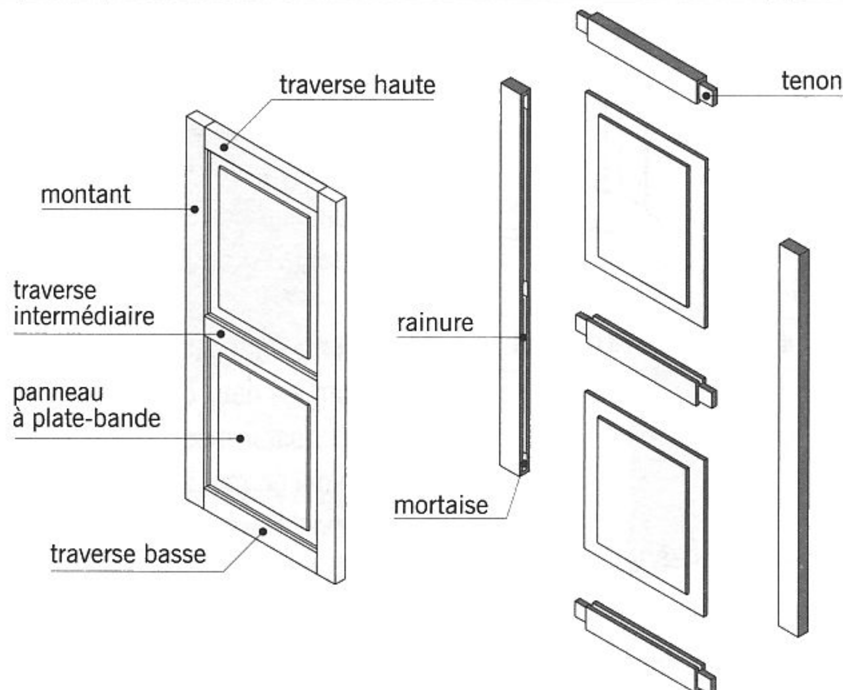
fig. 12.3 porte menuisée pleine
