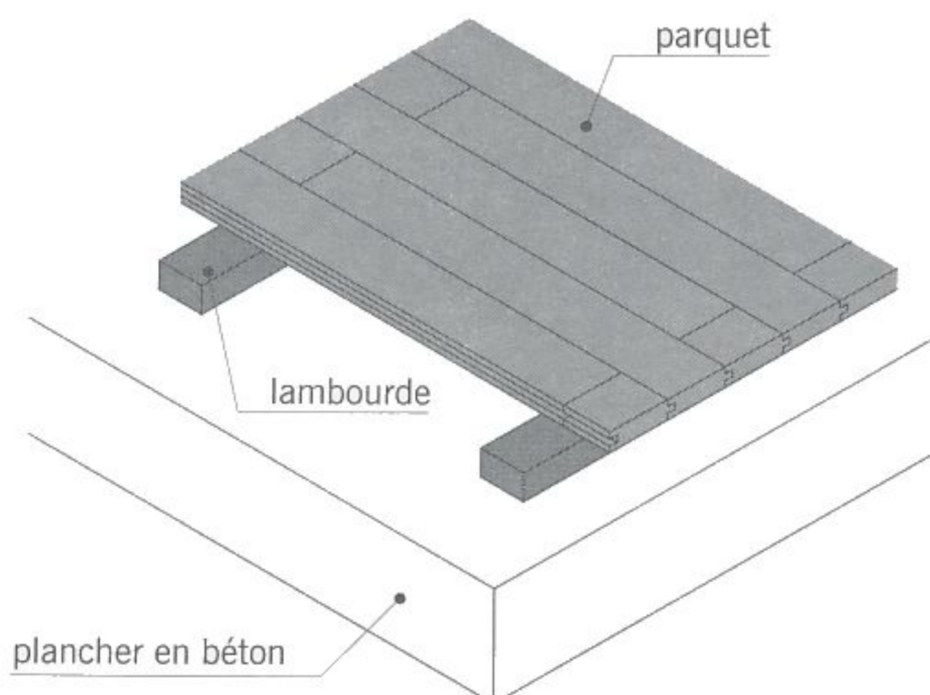
fig. 10.4 la pose sur lambourdes (2)
