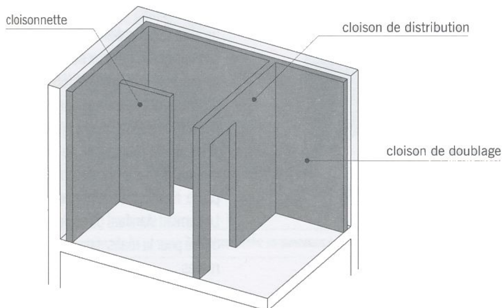
fig. 8.1 différentes cloisons
