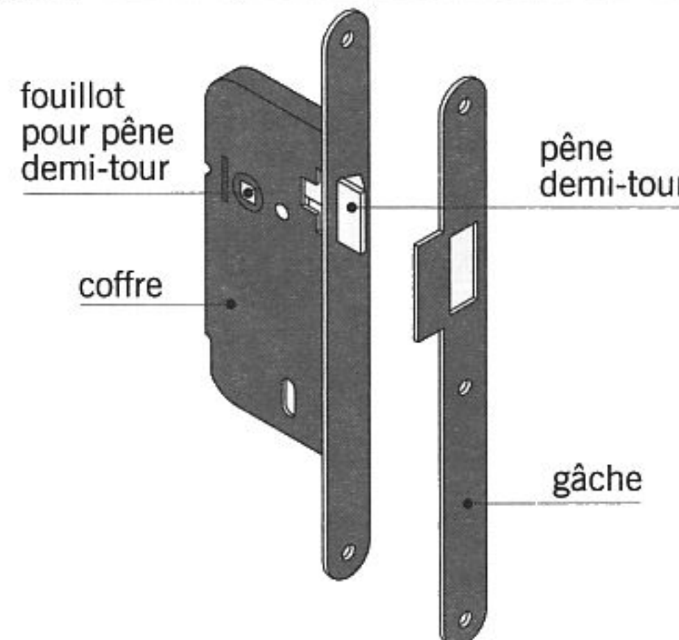
fig. 12.18 serrure à larder à bec de cane
