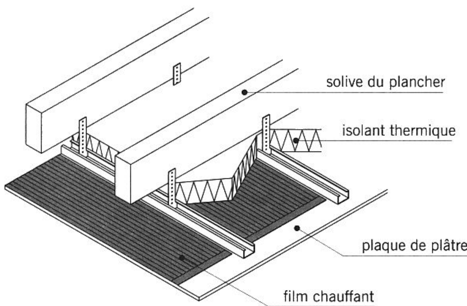
fig. 17.12 plafond avec film chauffant
