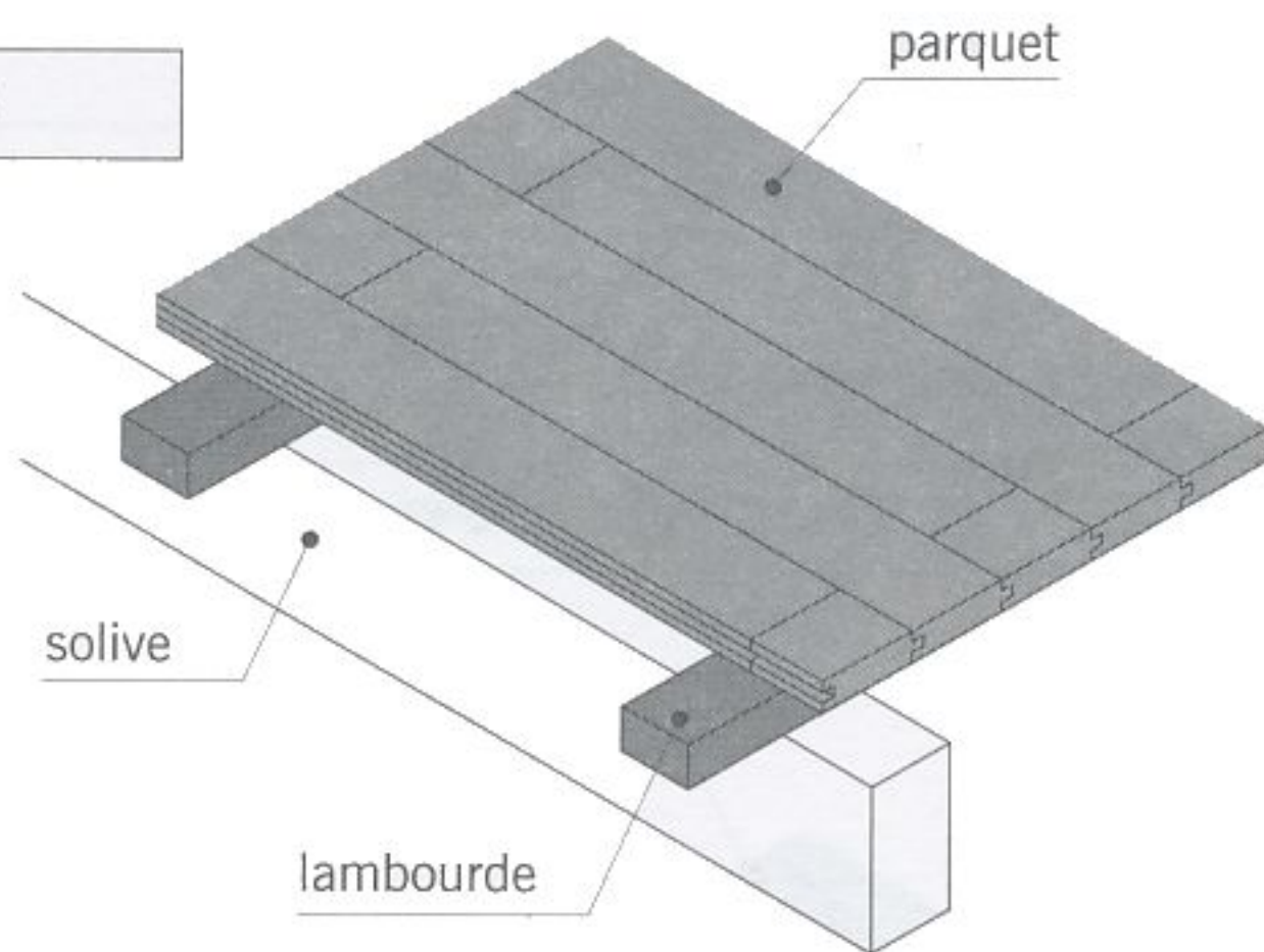
fig. 10.3 la pose sur lambourdes (1)
