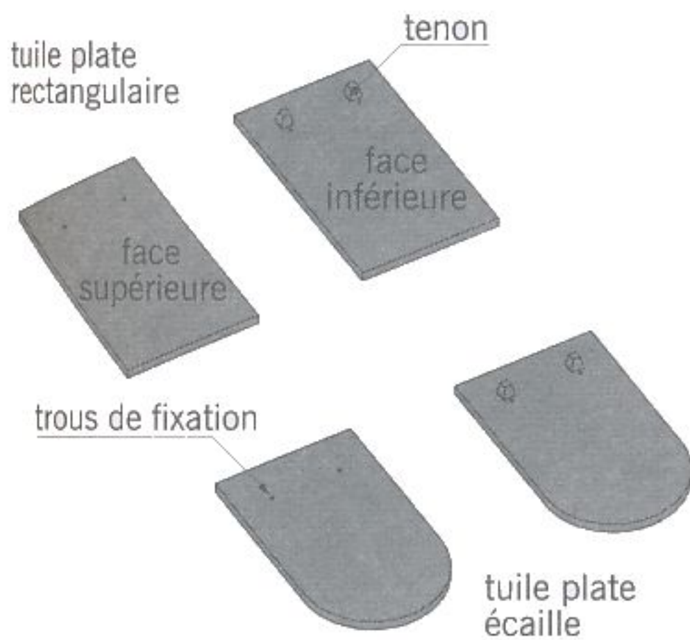
fig. 7.10 tuiles plates
