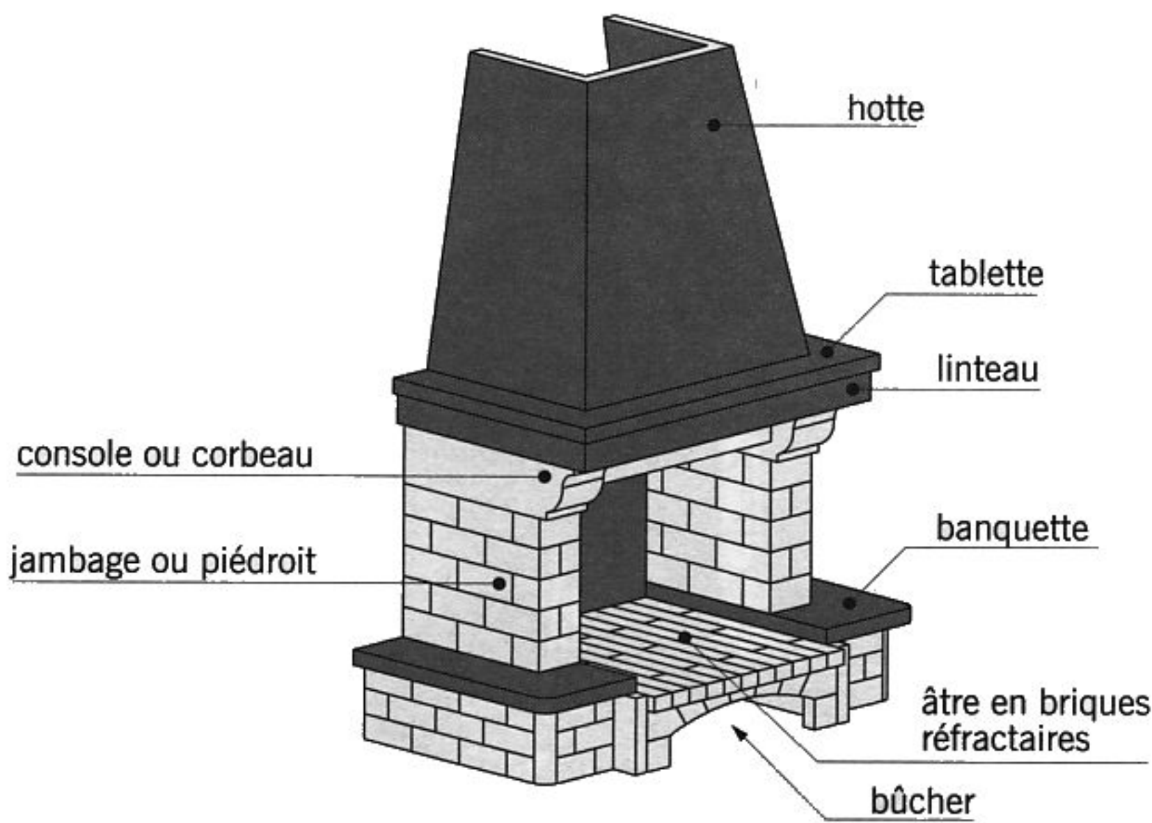
fig. 17.36 cheminée (1)
