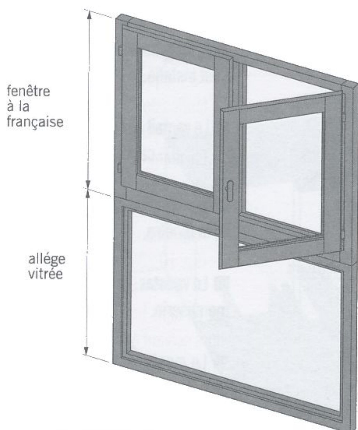
fig. 11.2 fenêtre composée en bois (fenêtre à la française + allège)
