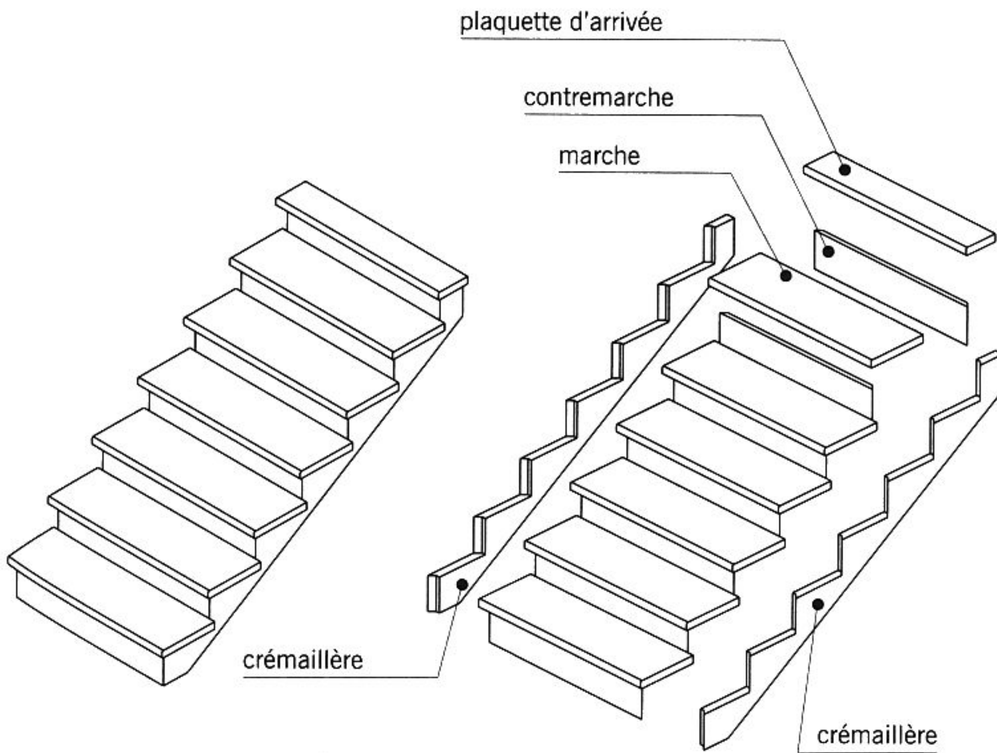
fig. 13.15 escaler à l'anglaise
