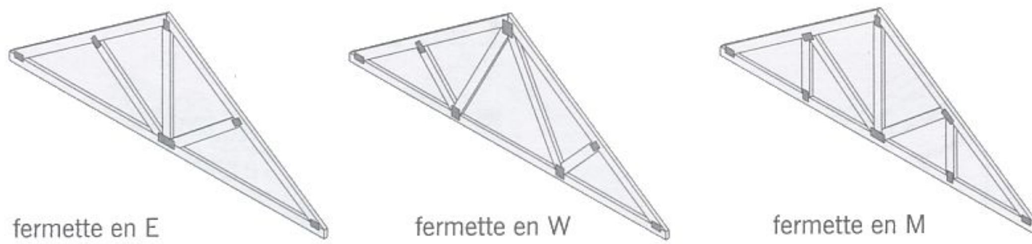
fig. 5.18 fermettes pour combles perdus
