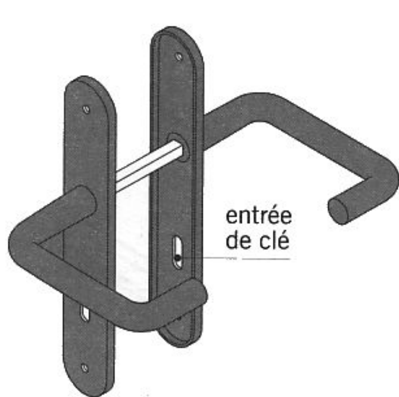
fig. 12.22 ensemble de porte pour serrure à deux pênes
