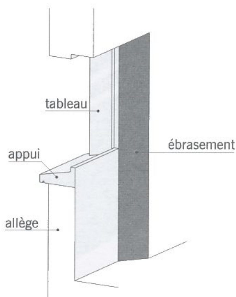
fig. 3.37 ébrasement
