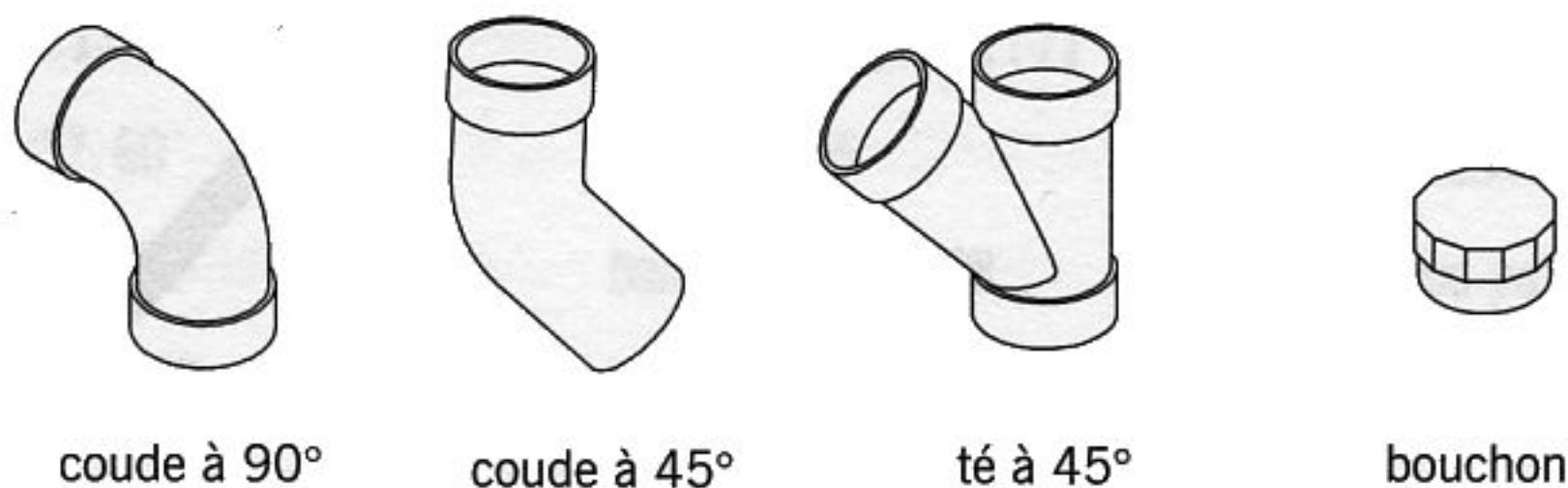
fig. 19.3 raccords
