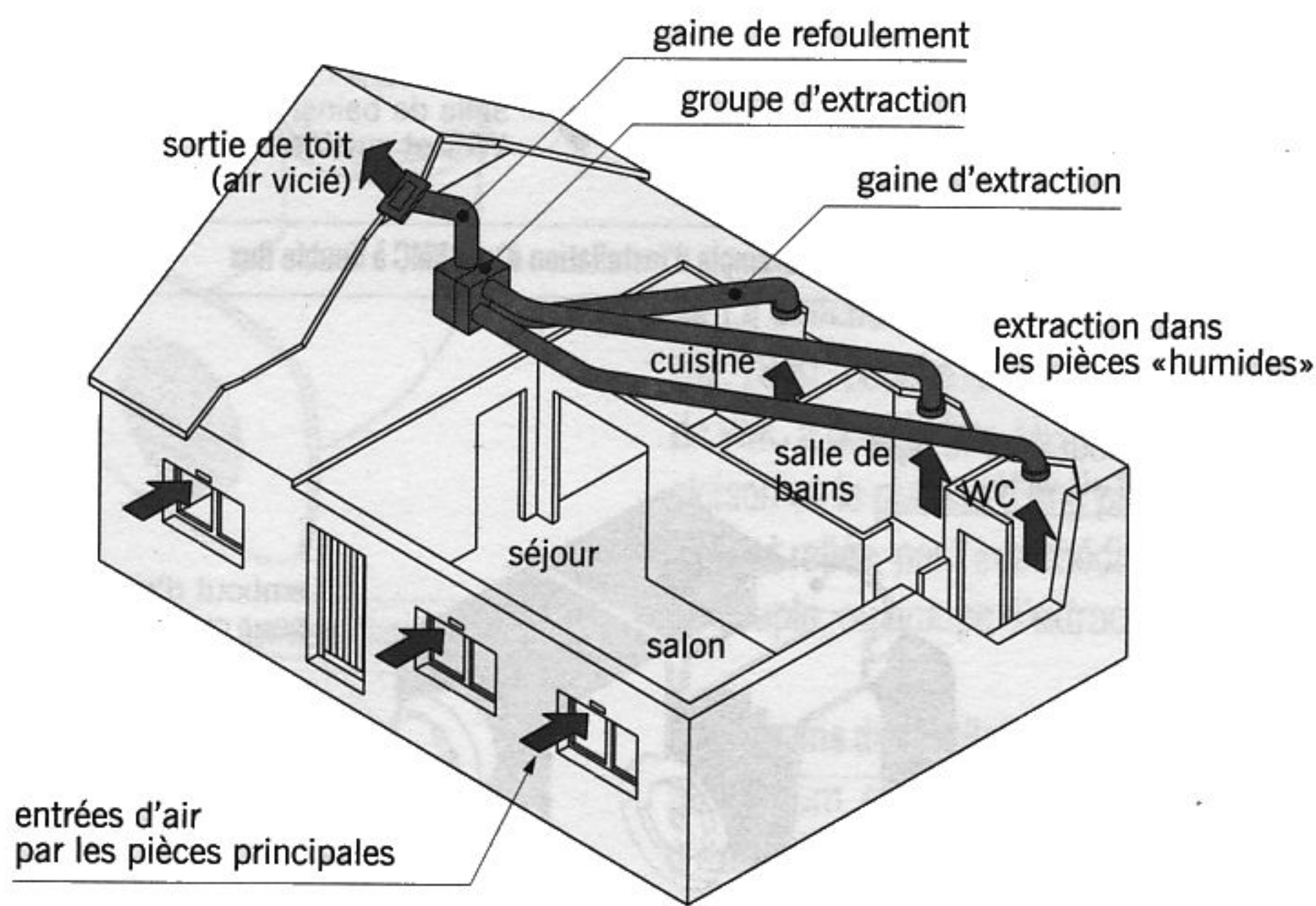
fig. 18.2 VMC à simple flux
