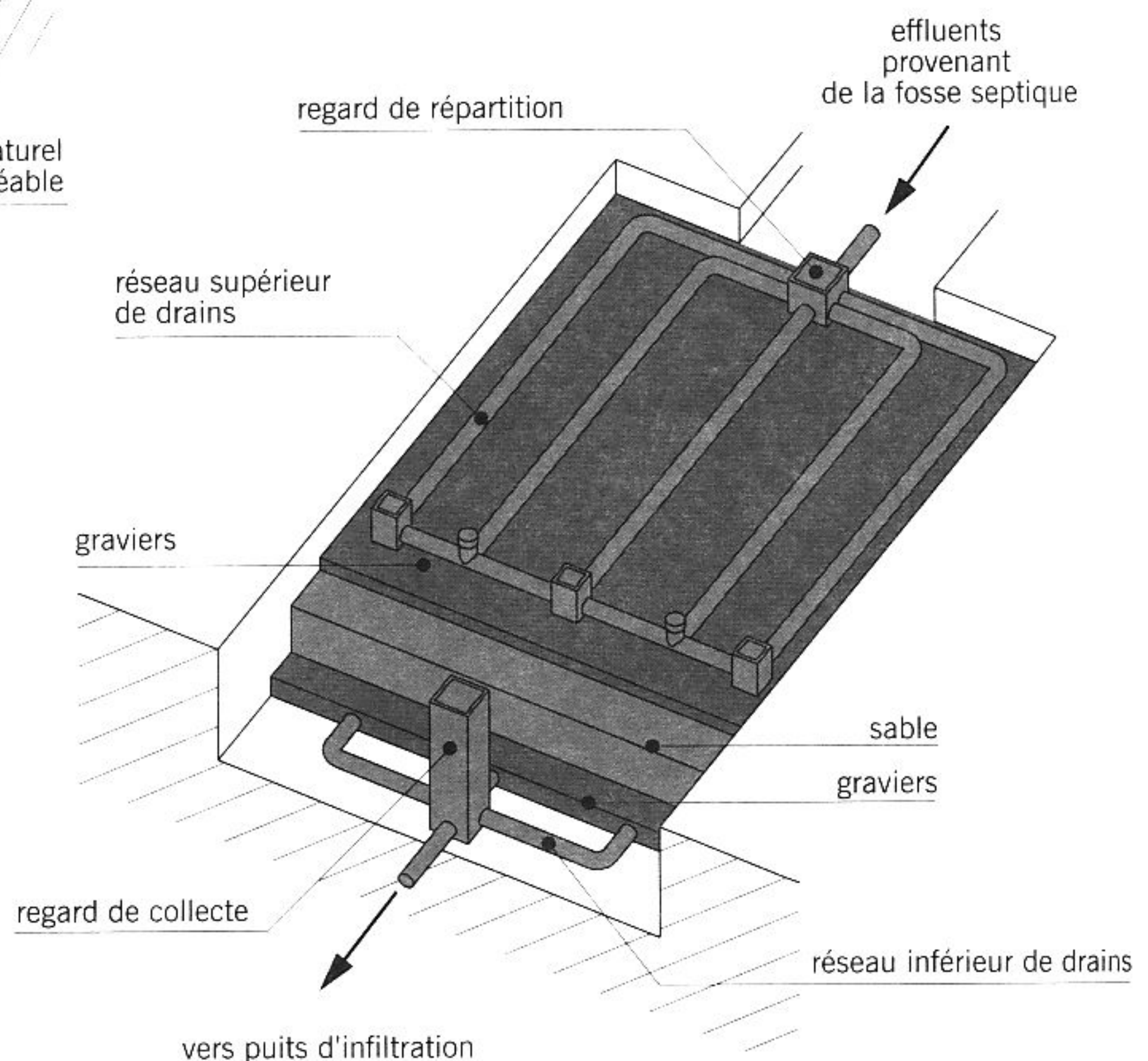
fig. 15.21 filtre à sable vertical drainé
