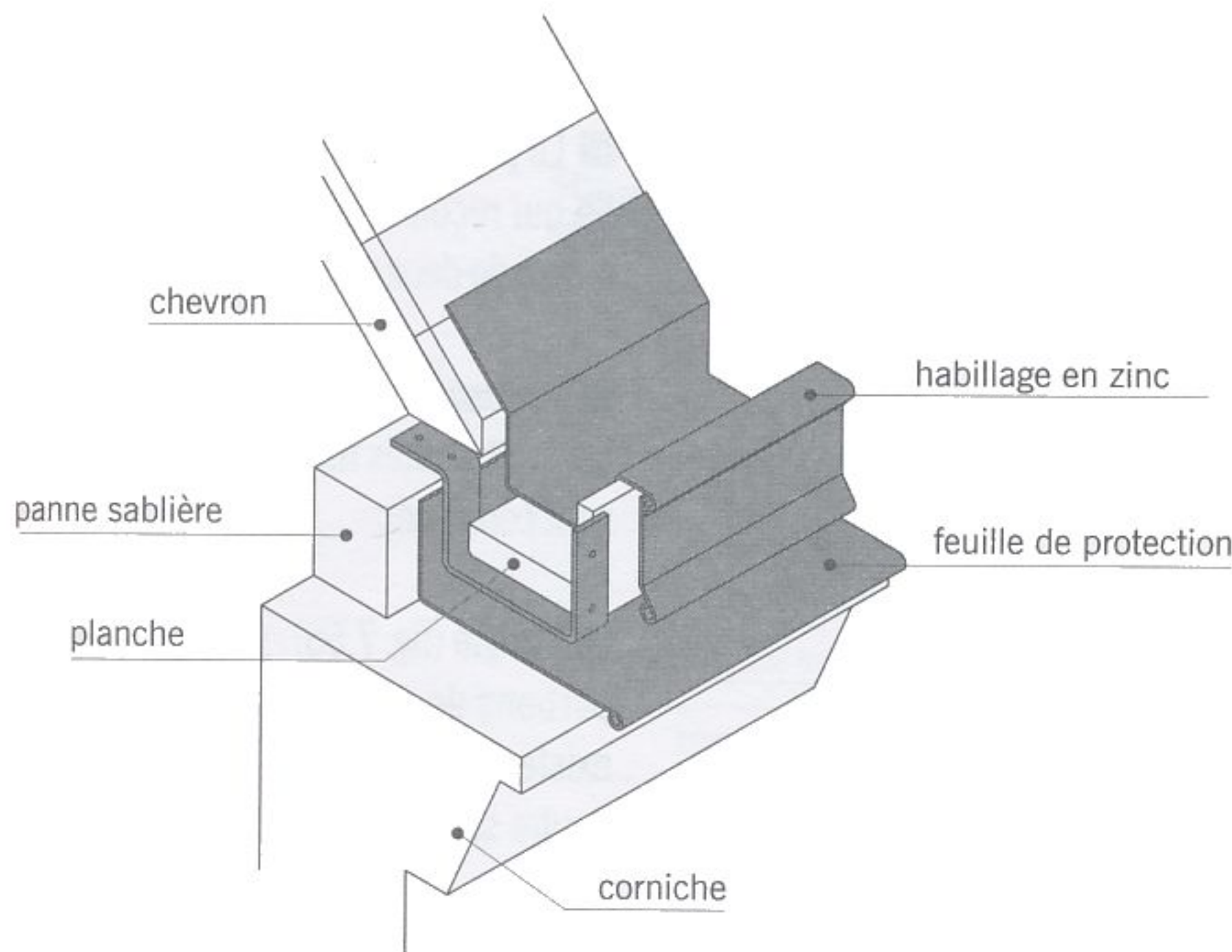
fig. 7.59 chéneau à l'anglaise (couverture non représentée)
