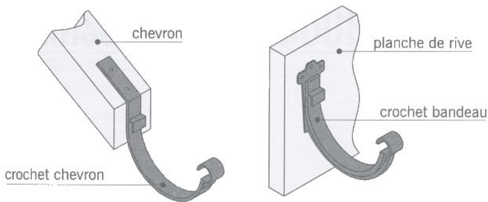
fig. 7.68 crochets pour gouttières pendantes
