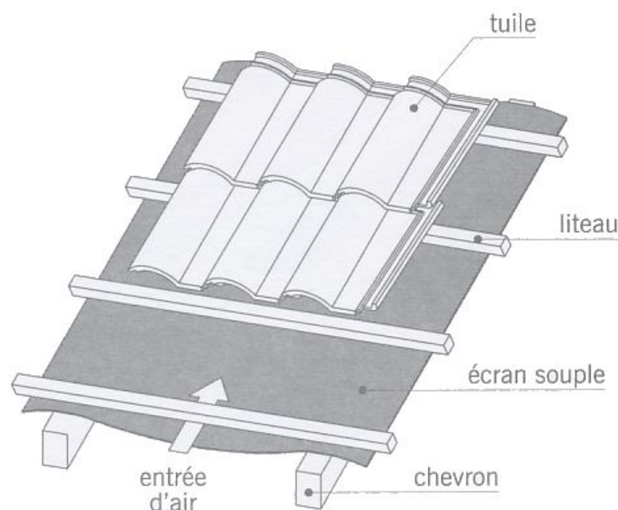
fig. 7.7 écran souple non tendu
