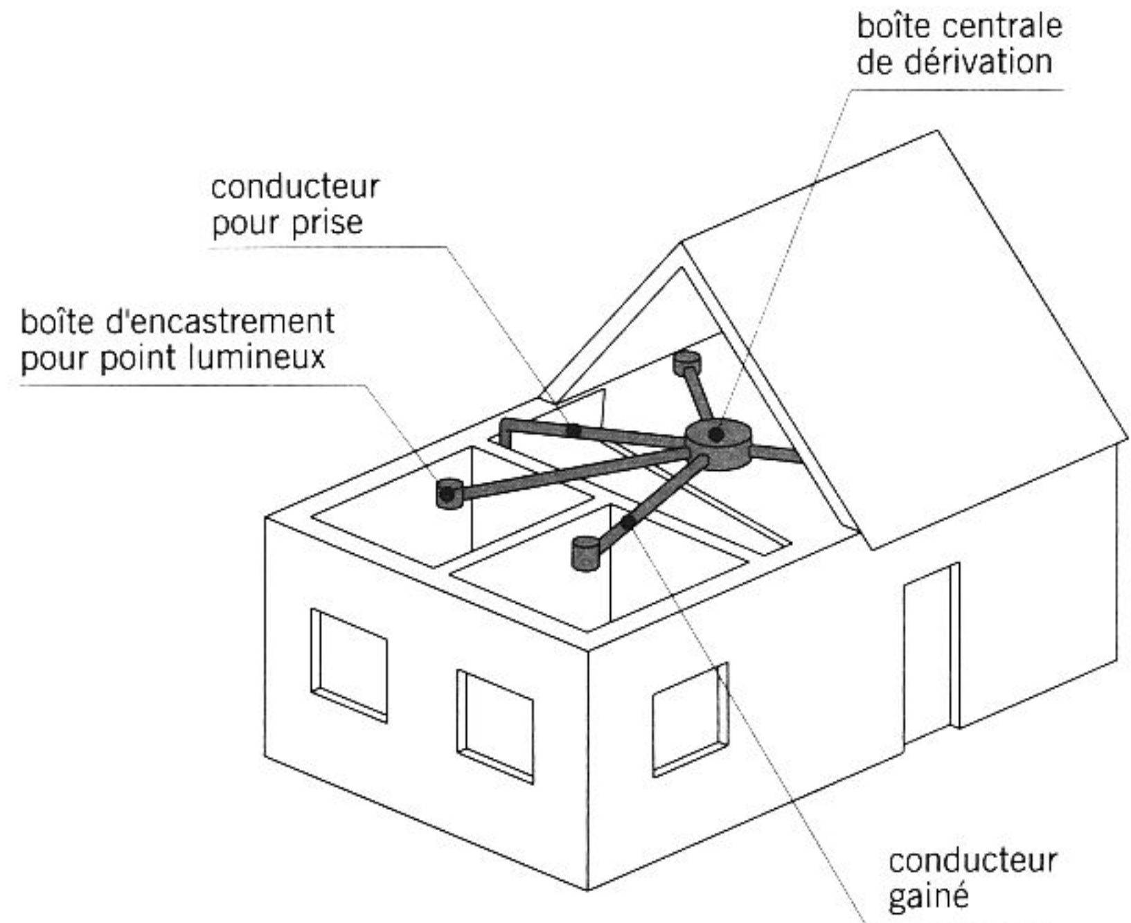
schéma d'installation d'un montage pieuvre
