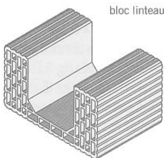
fig. 3.11 blocs spéciaux en terre cuite
