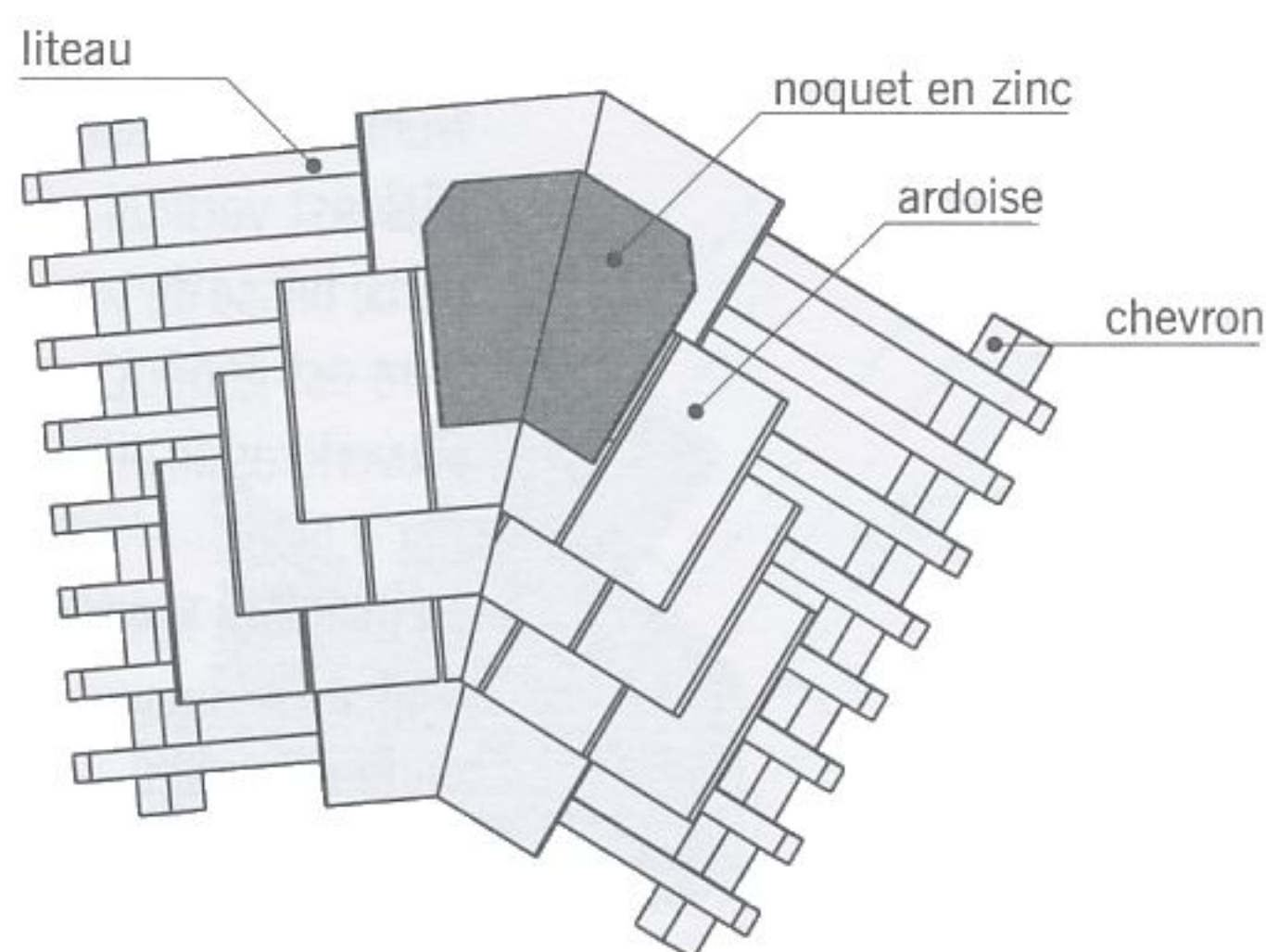
fig. 7.48 noquet sur noue en ardoises
