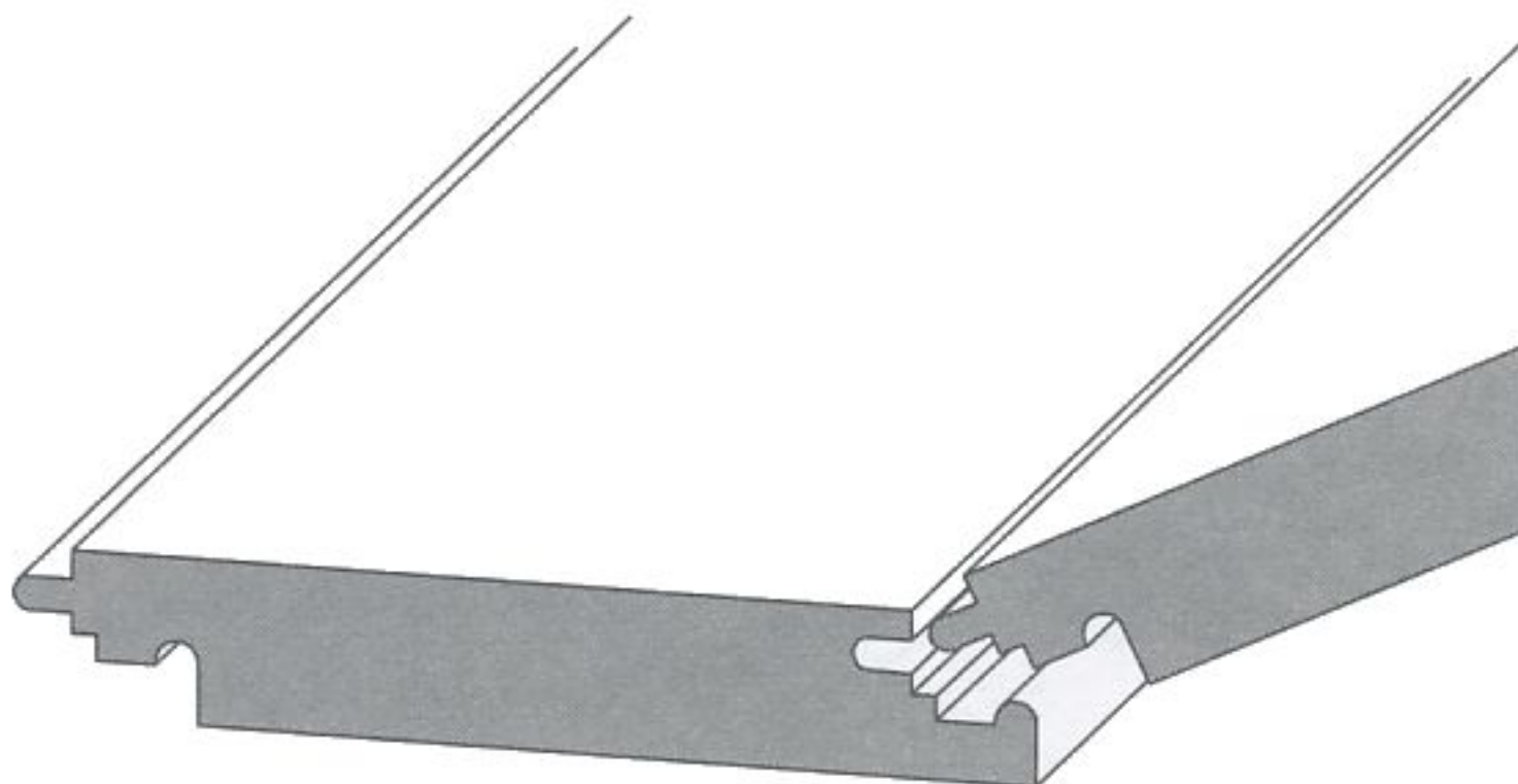
fig. 10.11 lames stratifiées (exemple d'un système d'emboîtement)
