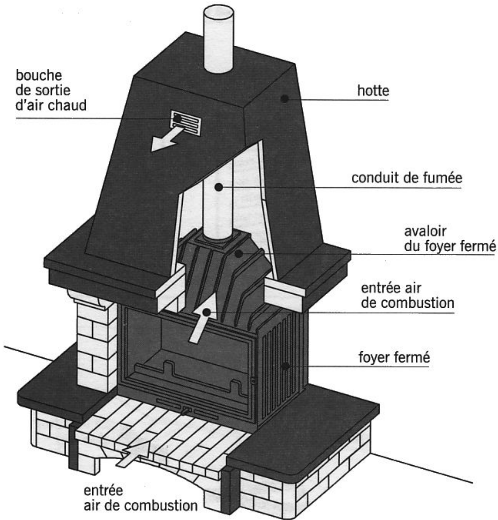
principe de fonctionnement du foyer fermé
