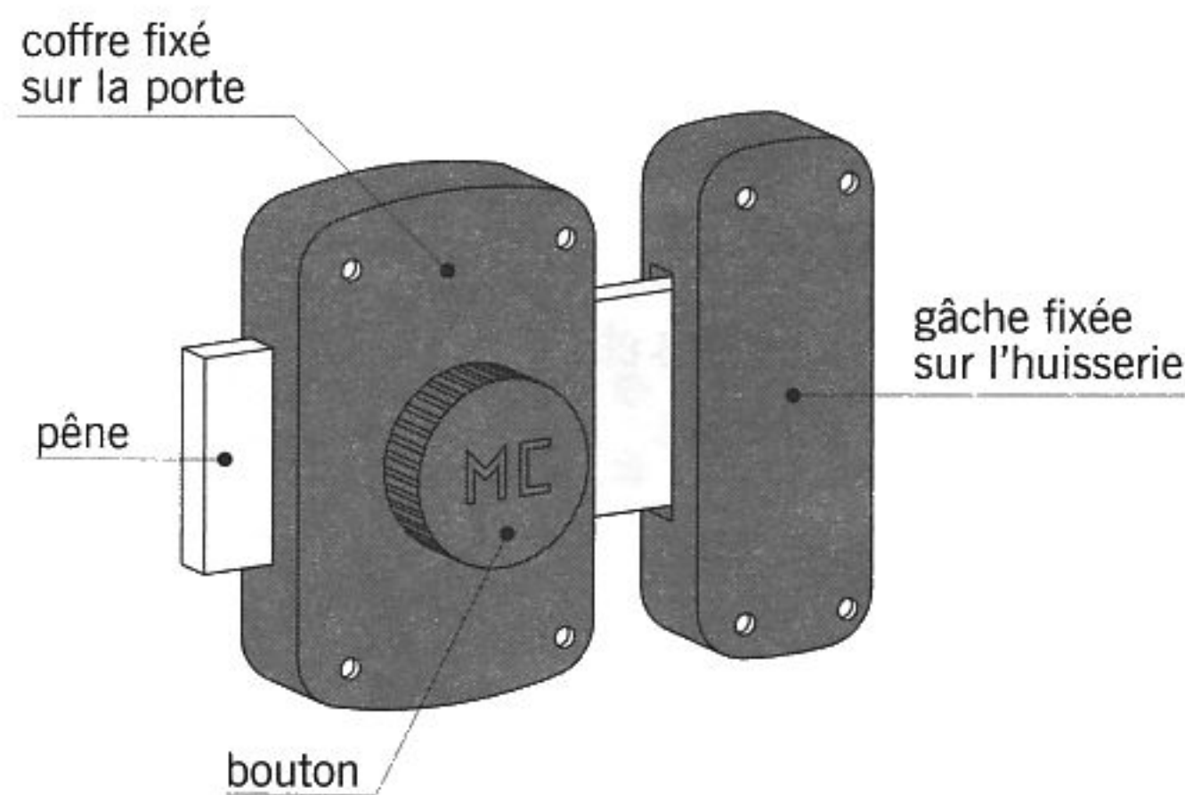
fig. 11.49 verrou de sûreté
