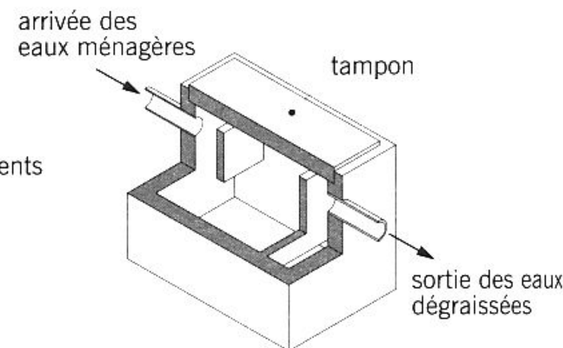
fig. 15.13 bac à graisses en béton
