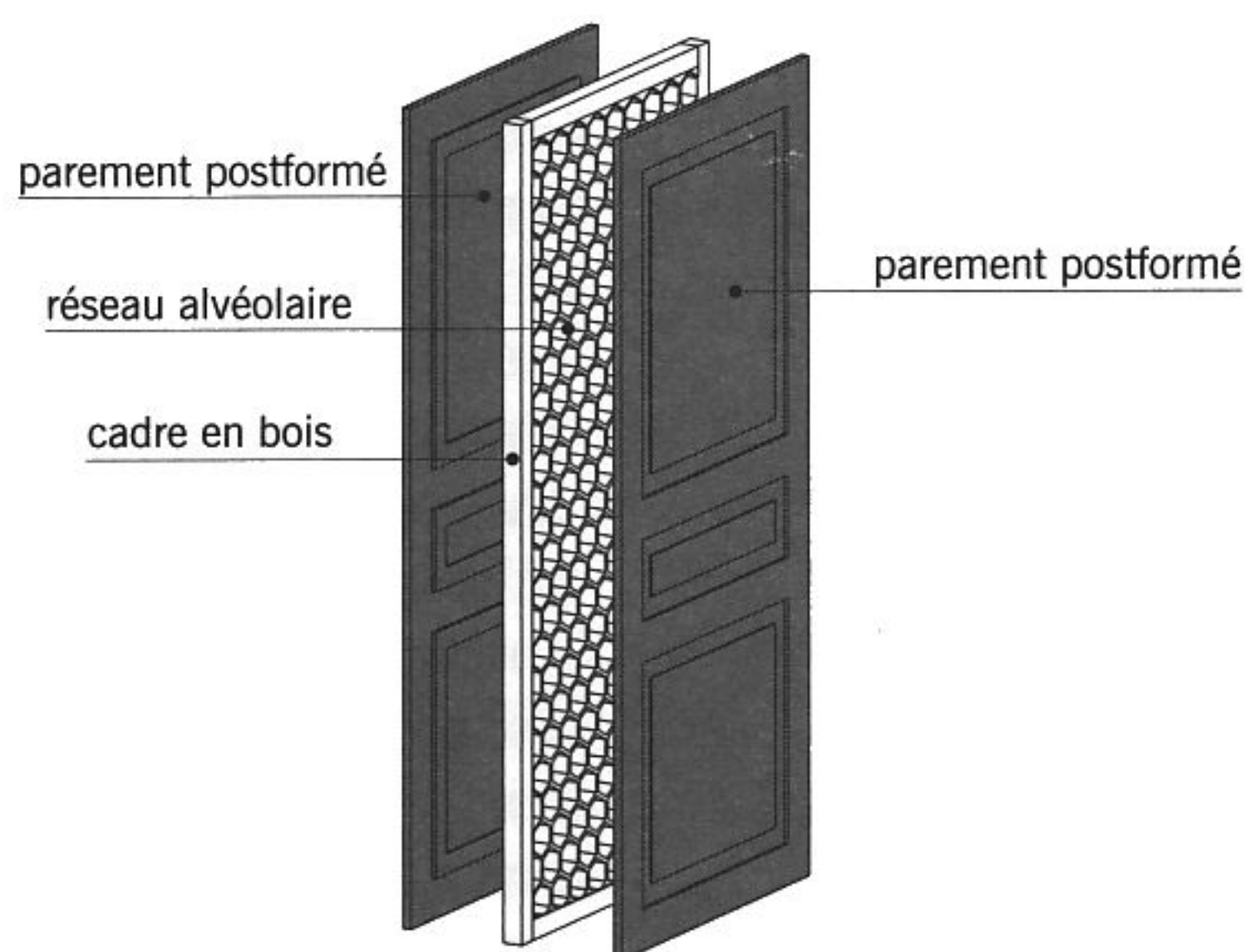
fig. 12.5 porte postformée
