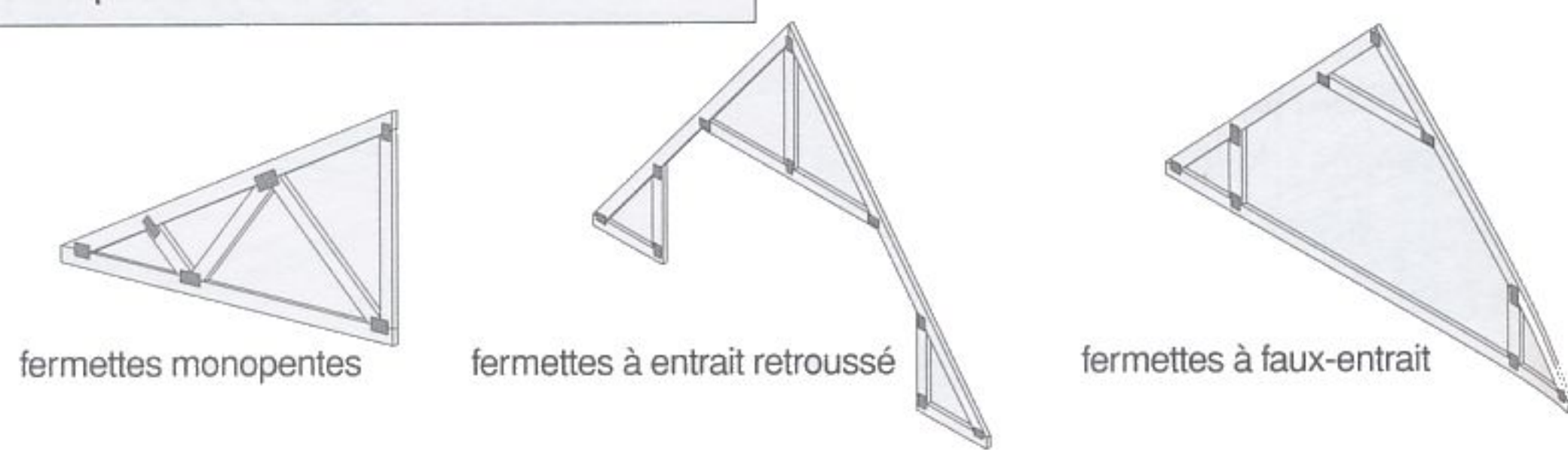
fig. 5.19 charpente en fermettes pour combles habitables
