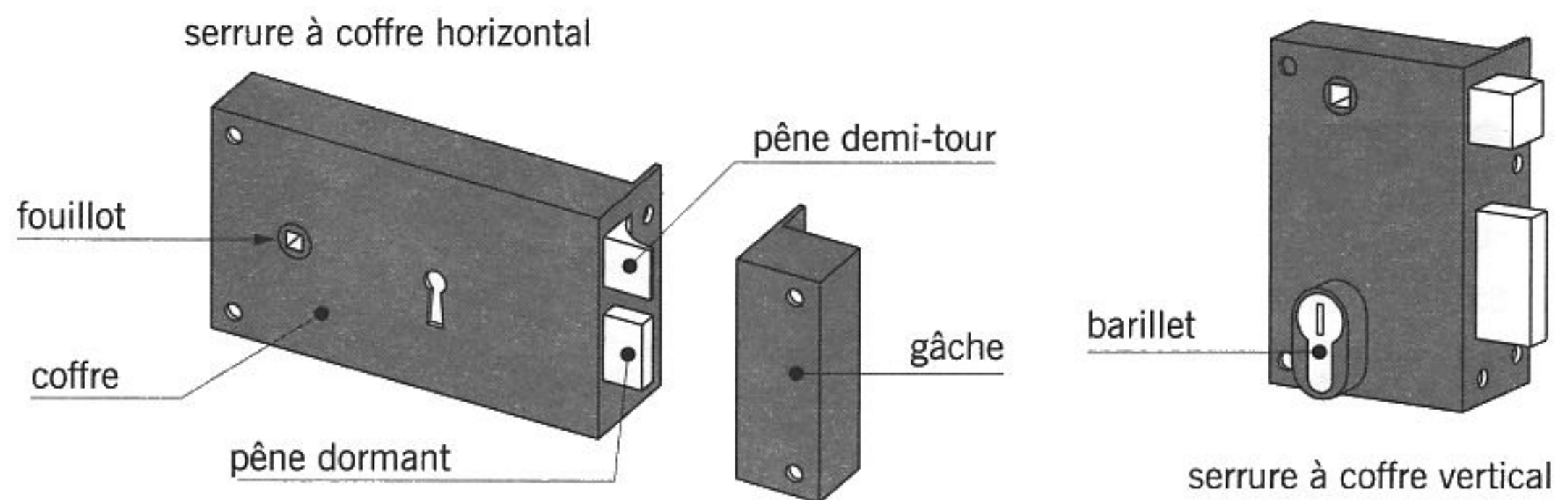
fig. 11.48 serrures en applique
