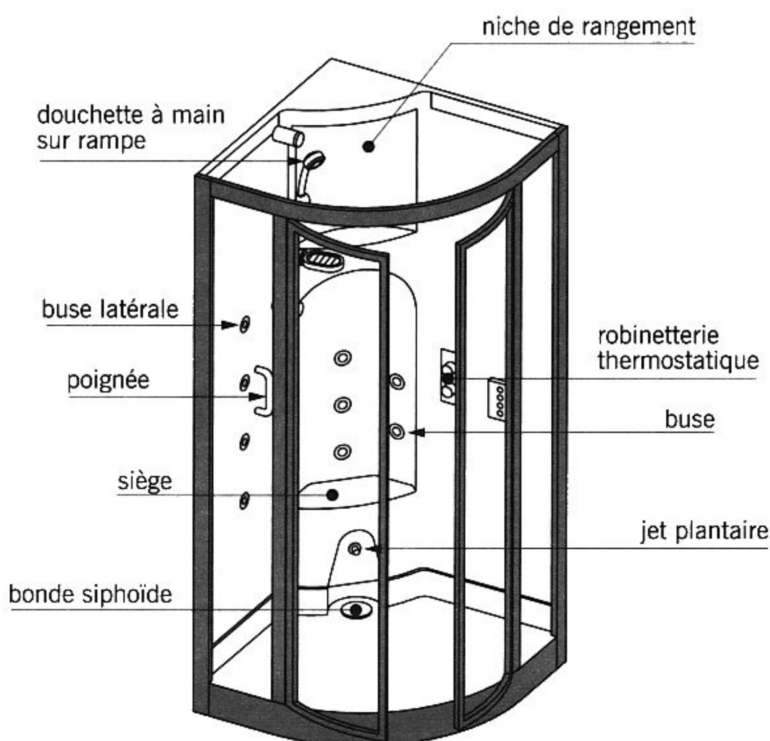
fig. 14.22 cabine d'hydromassage
