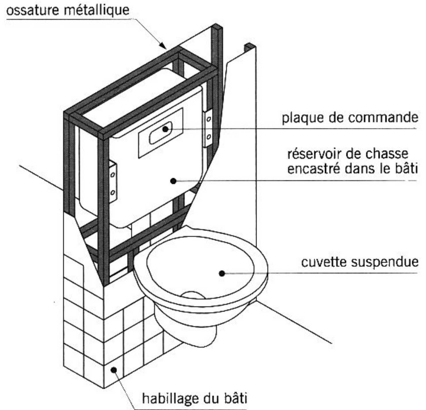
W.-C. fixé sur un bâti support
