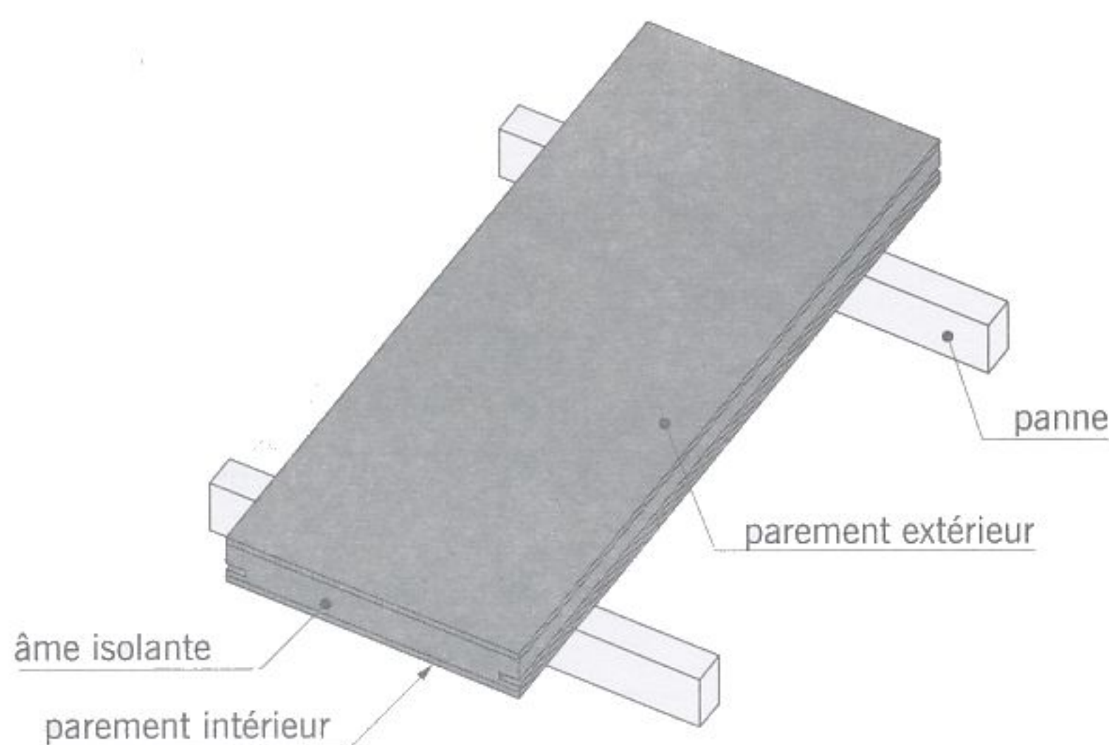
fig. 7.4 panneau sandwich
