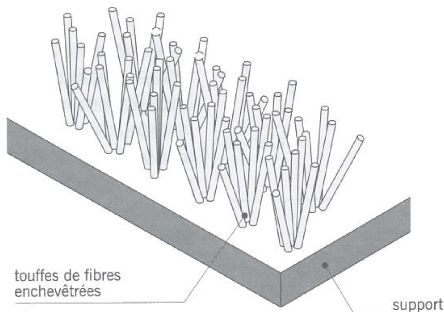
fig. 10.19 moquette aiguilletée
