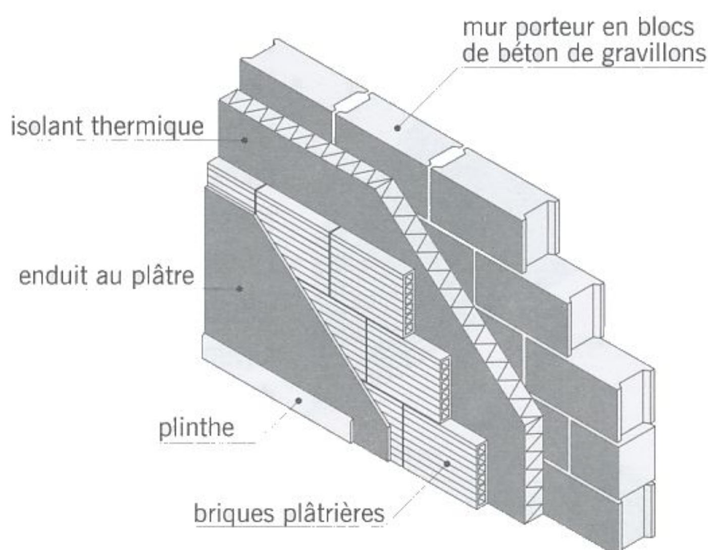
fig. 8.2 cloison de doublage
