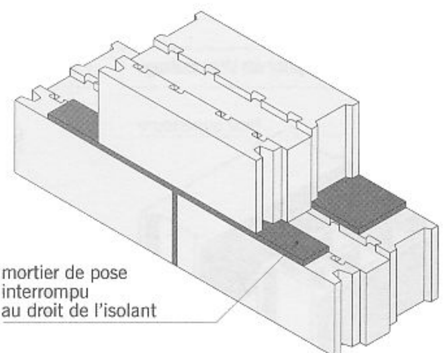
fig. 3.14 mise en place des blocs à isolation intégrée
