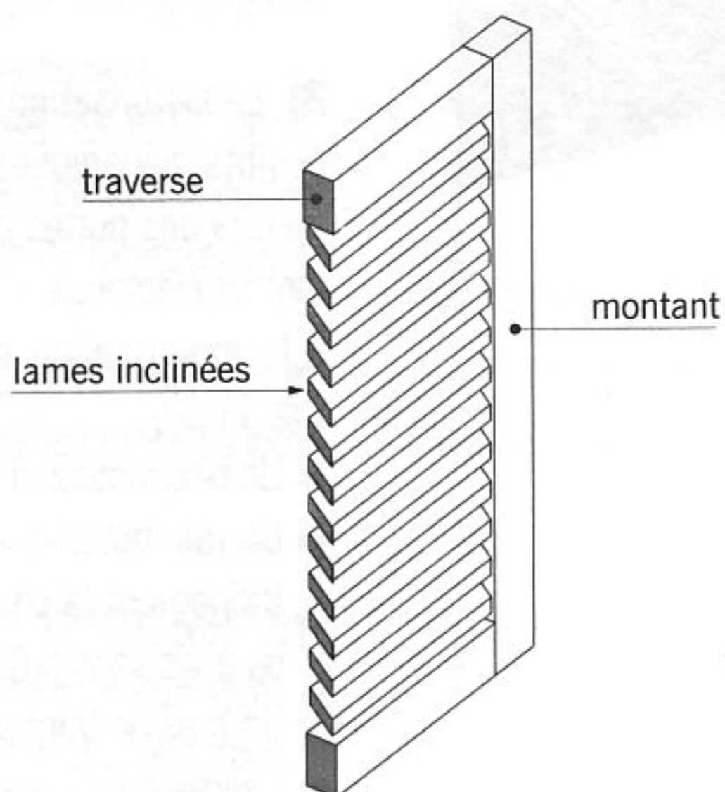
détail des lames d'un volet-persienne
