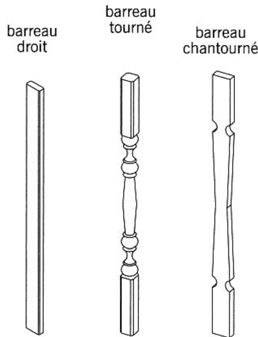
fig. 13.45 barreaux
