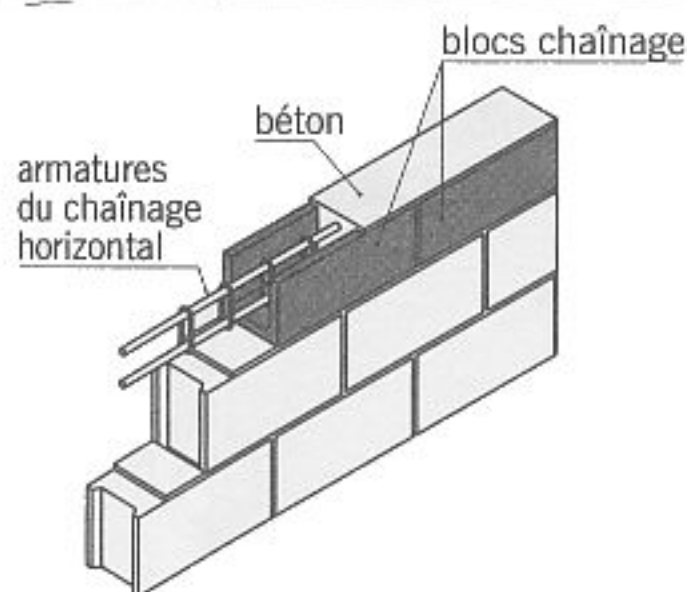
fig. 3.5 mise en place des blocs chaînage
