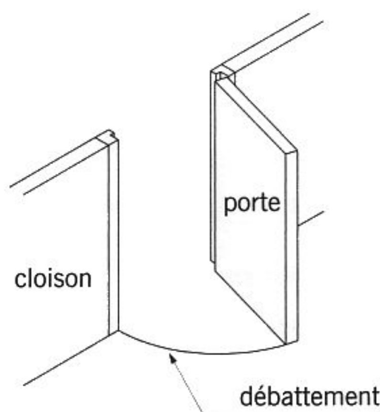
fig. 12.13 débattement
