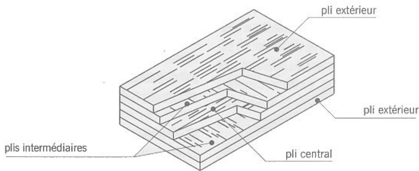
fig. 1.9 contreplaqué
