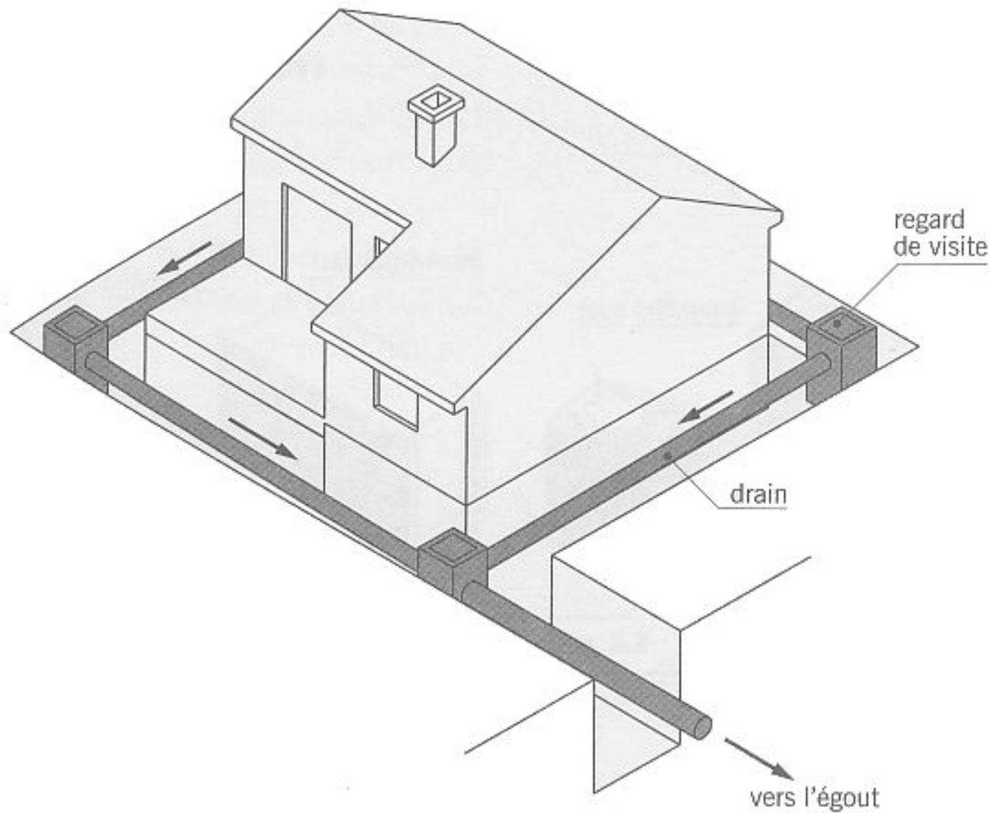
fig. 2.14 dispositif de drainage
