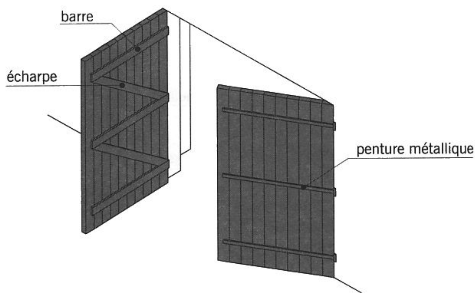
fig. 11.53 porte battante
