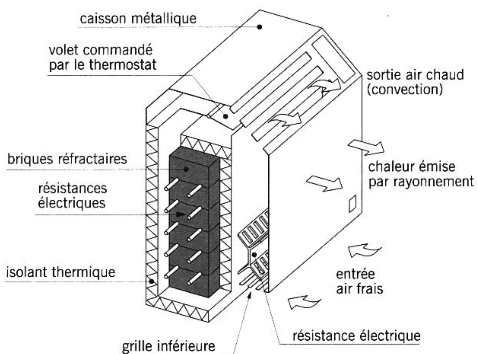
fig. 17.8 accumulateur statique compensé
