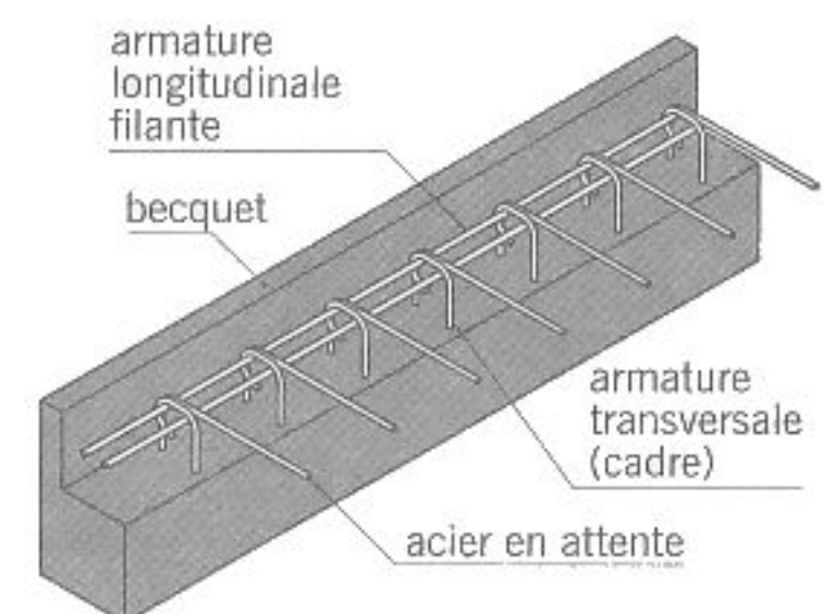
fig. 2.10 longrine de rive
