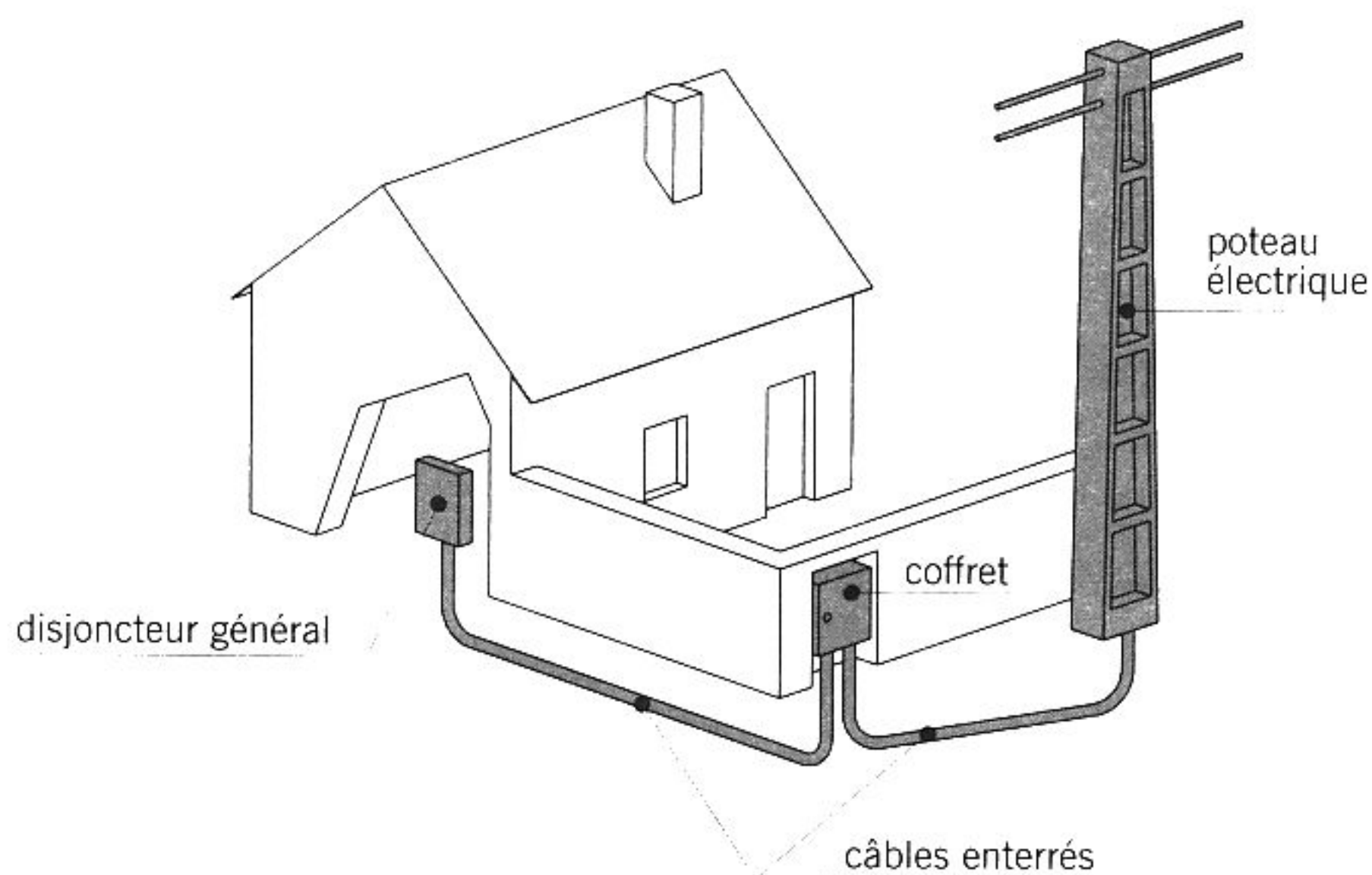
fig. 16.2 branchement aéro-souterrain
