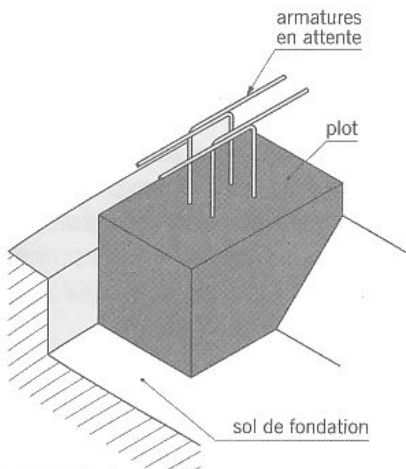
fig. 2.9 plot en béton
