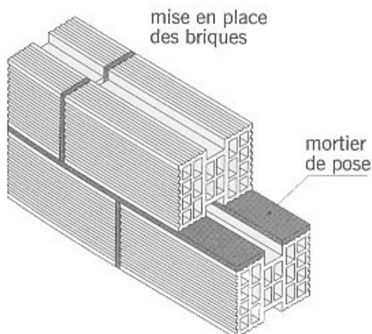
fig. 3.18 brique à rupture de joint
