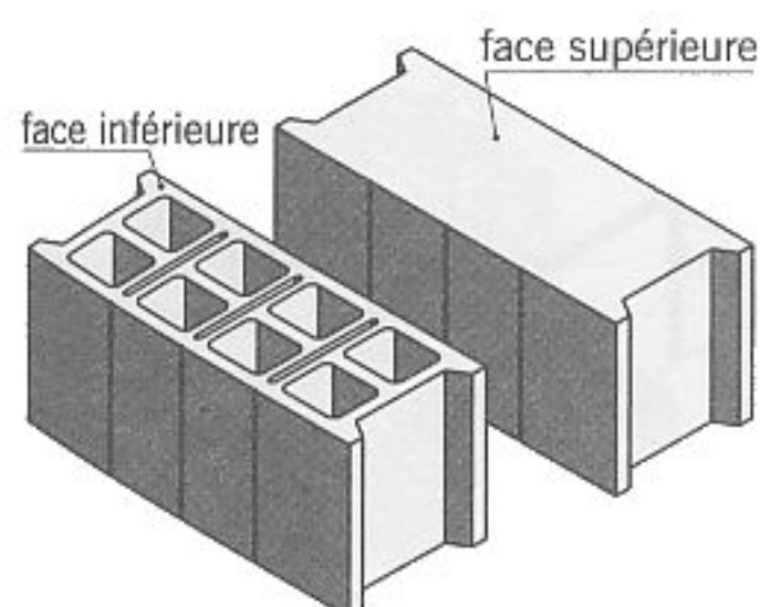
fig. 3.7 bloc de coupe
