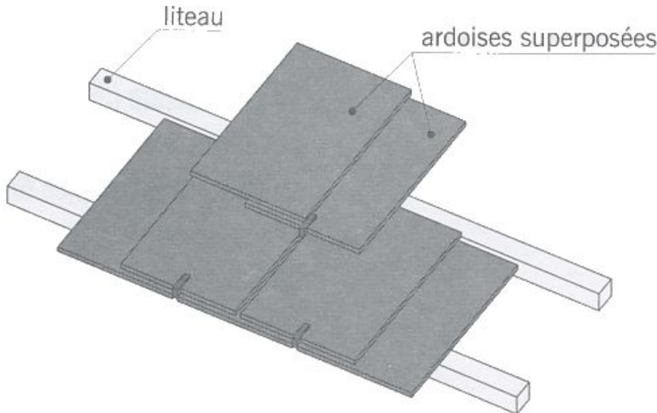
fig. 7.40 pose à pureau développé
