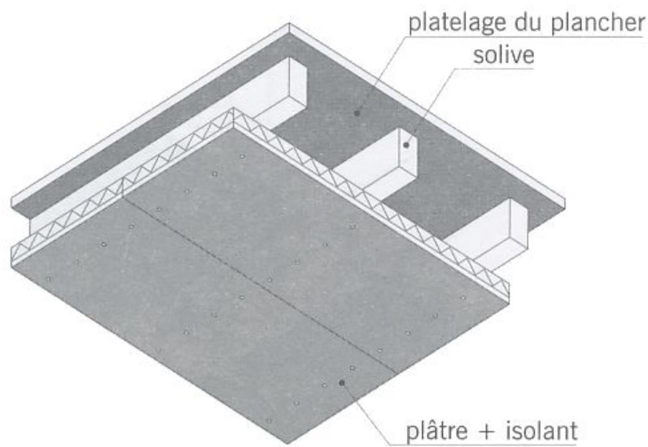
fig. 9.2 plafond fixe avec complexe isolant
