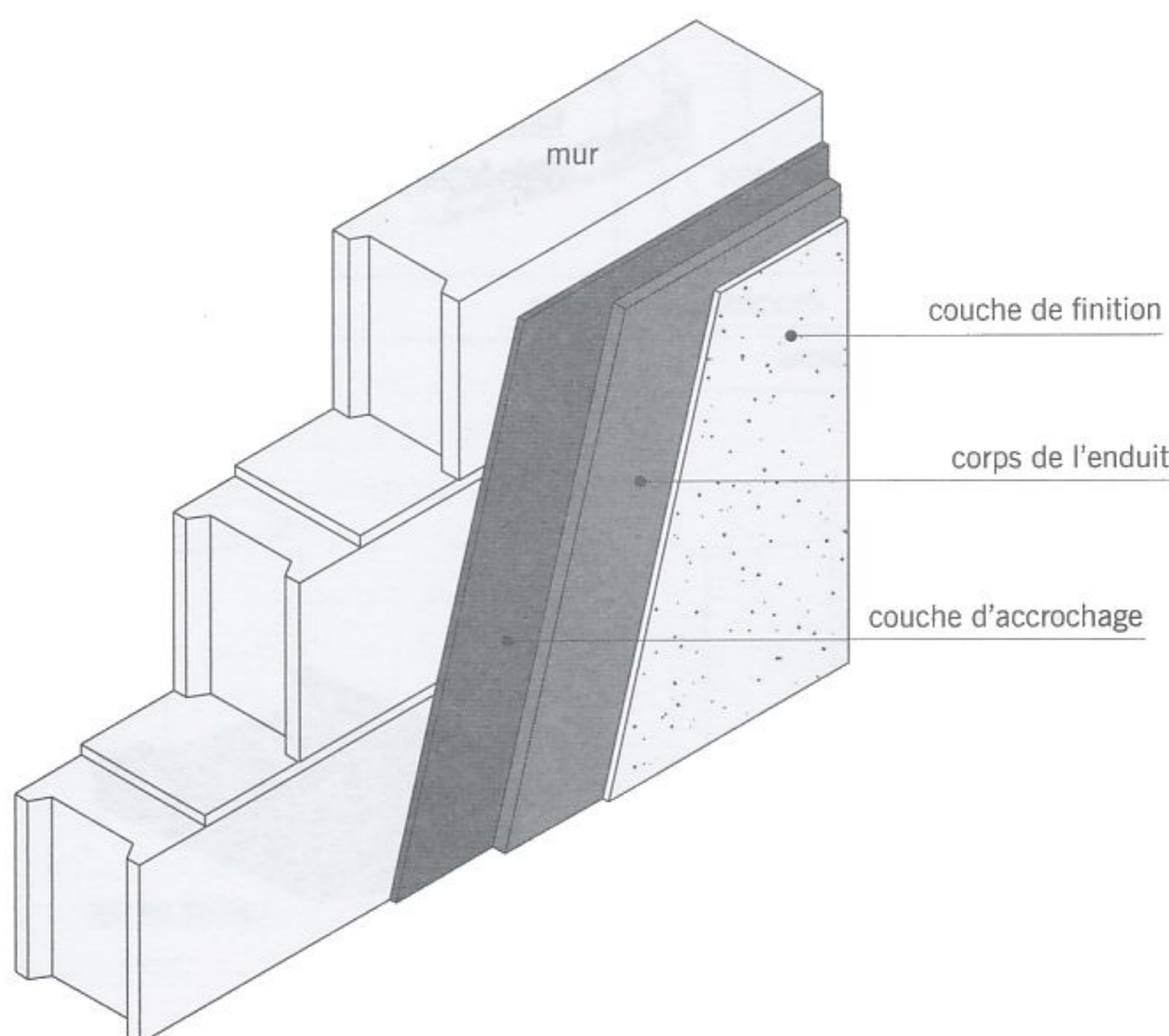
fig. 3.39 enduit traditionnel
