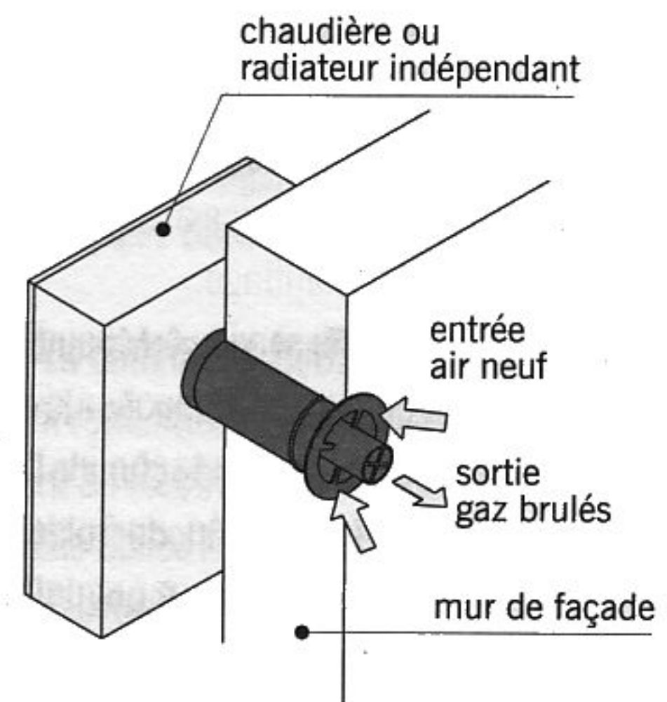
fig. 17.25 mise en place d'une ventouse
