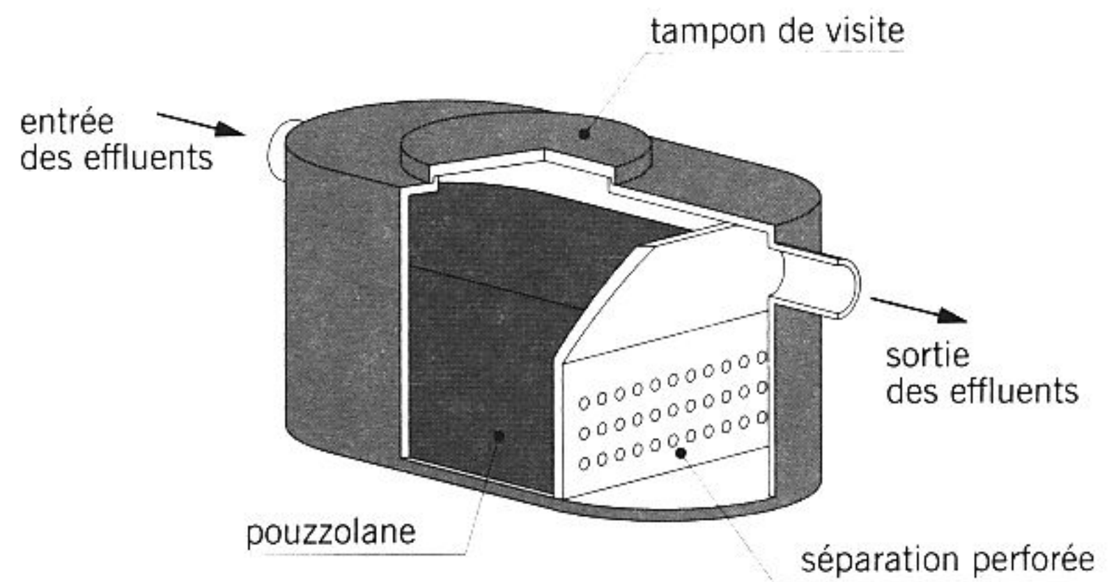
fig. 15.11 préfiltre
