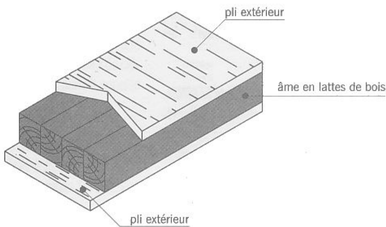
fig. 1.10 latté
