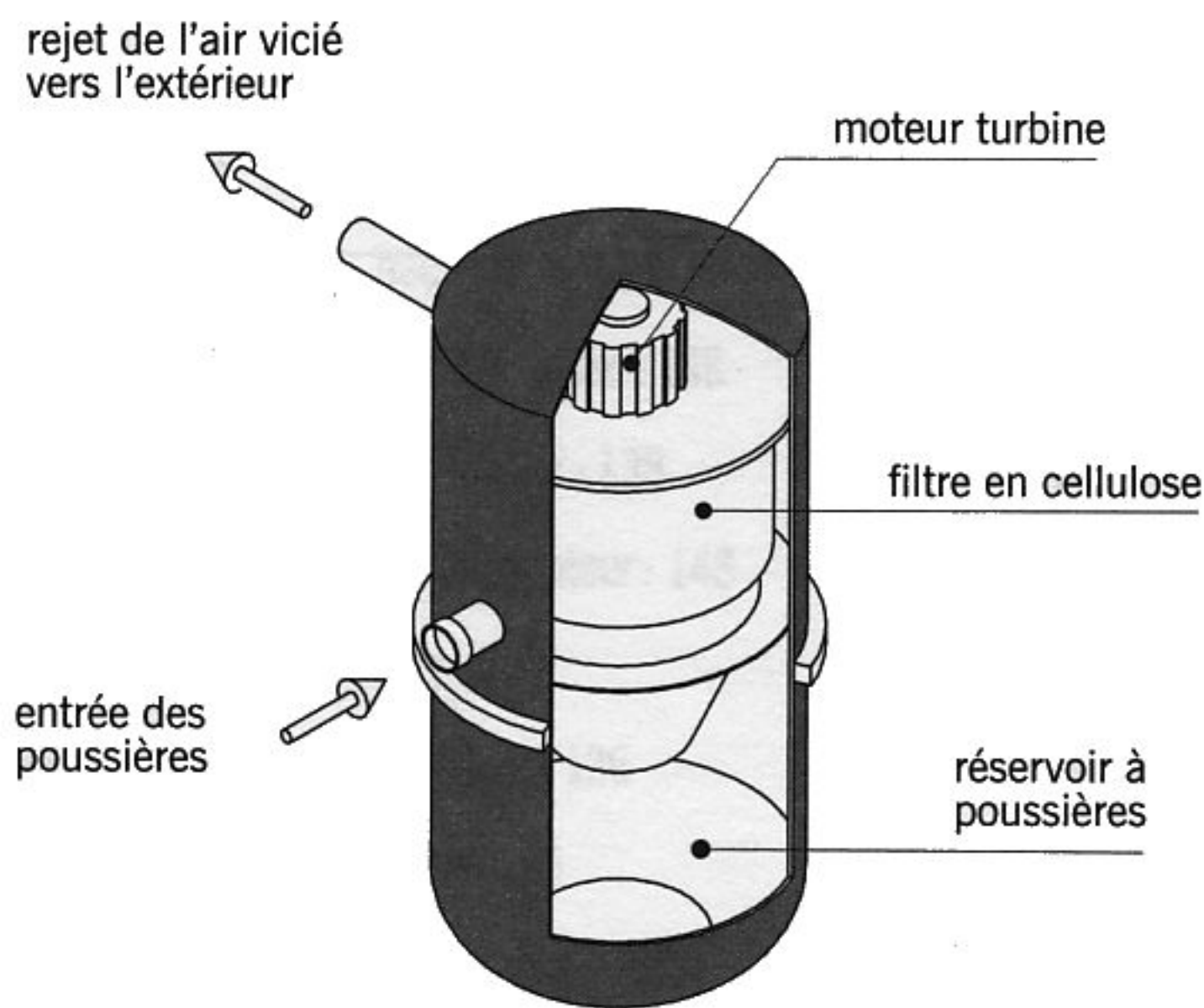
fig. 19.2 centrale d'aspiration
