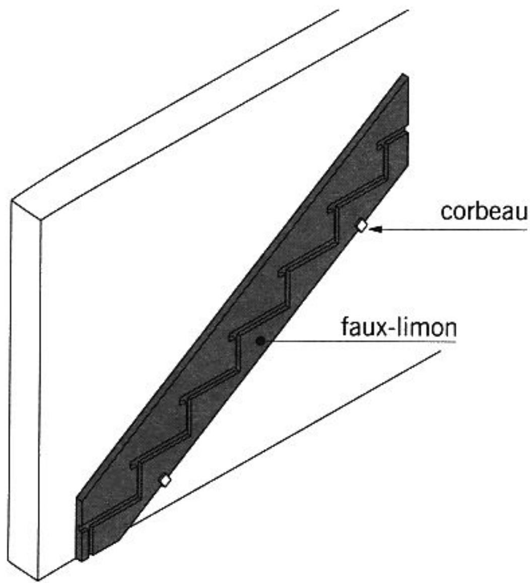
fig. 13.13 faux-limon
