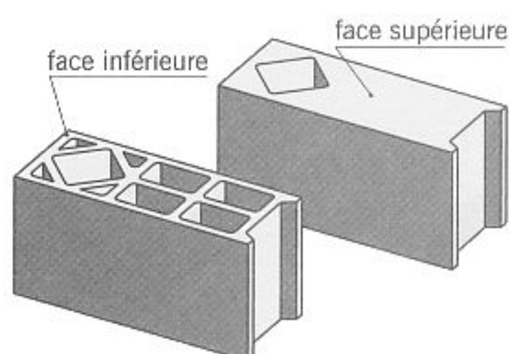
fig. 3.2 bloc d'angle
