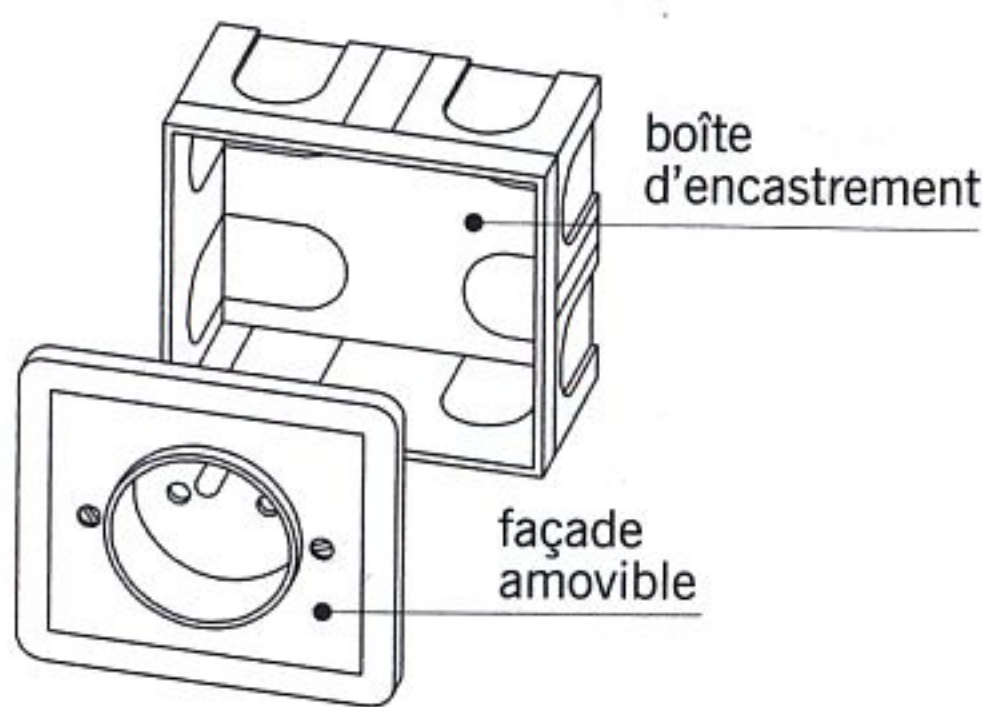
fig. 16.17 prise 2 P + T à encastrer
