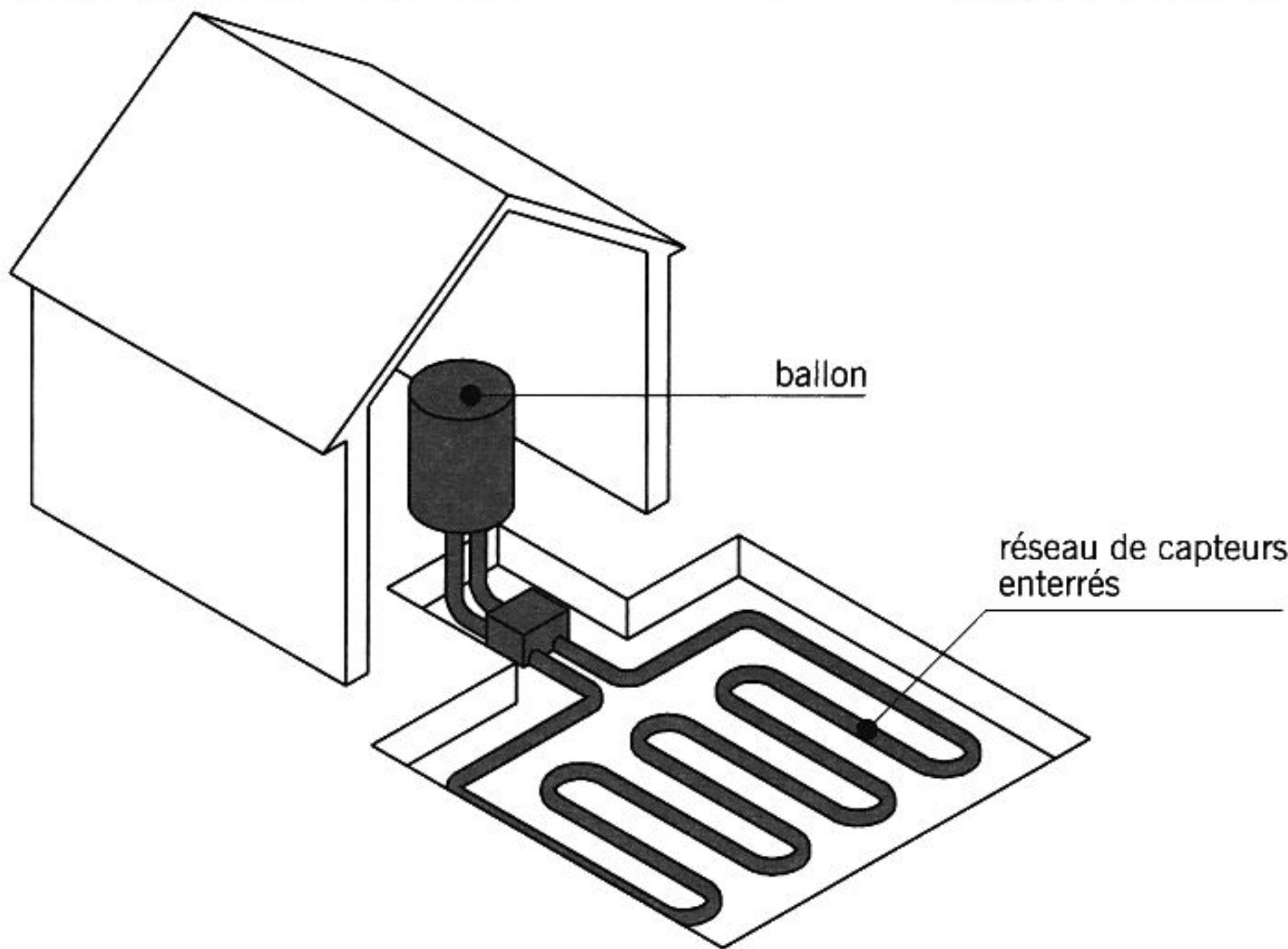
fig. 14.14 schéma d'une installation de chauffe-eau géothermique
