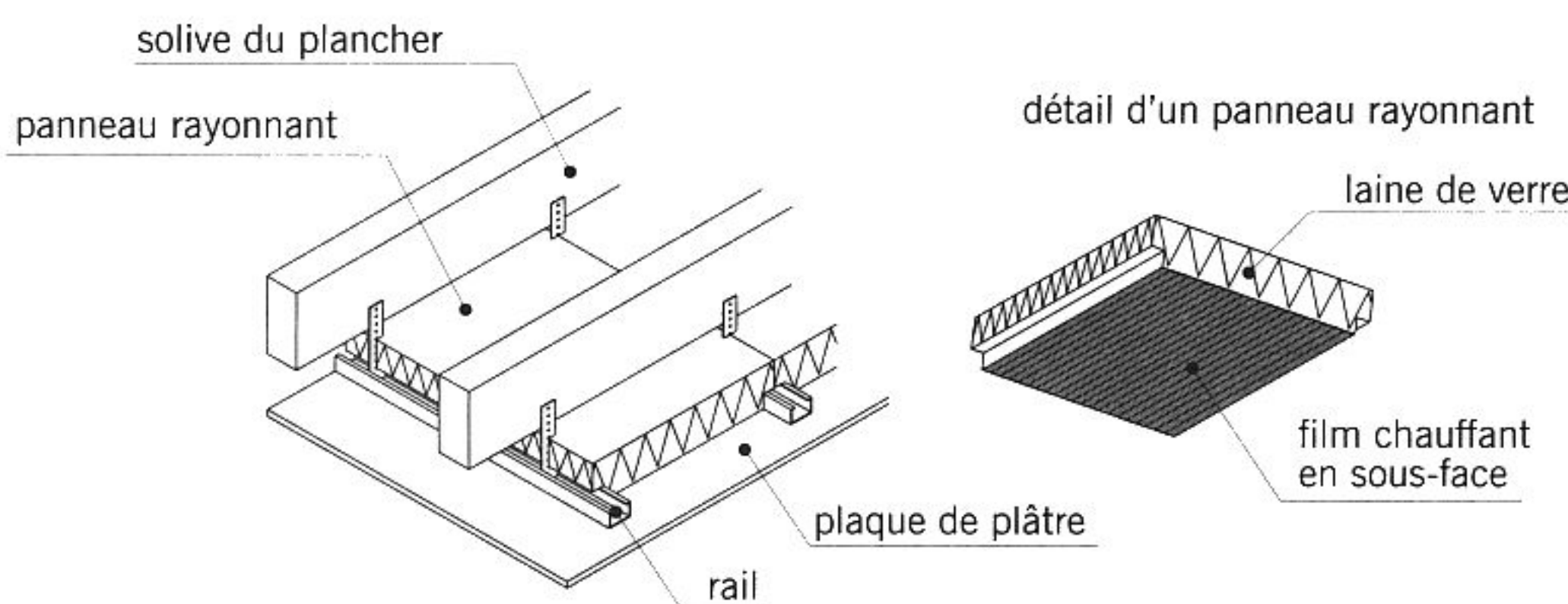
fig. 17.13 plafond avec panneau rayonnant
