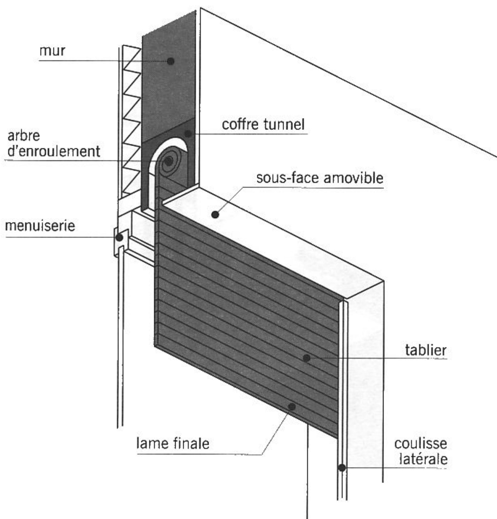
fig. 11.64 coffre placé dans l'épaisseur du mur
