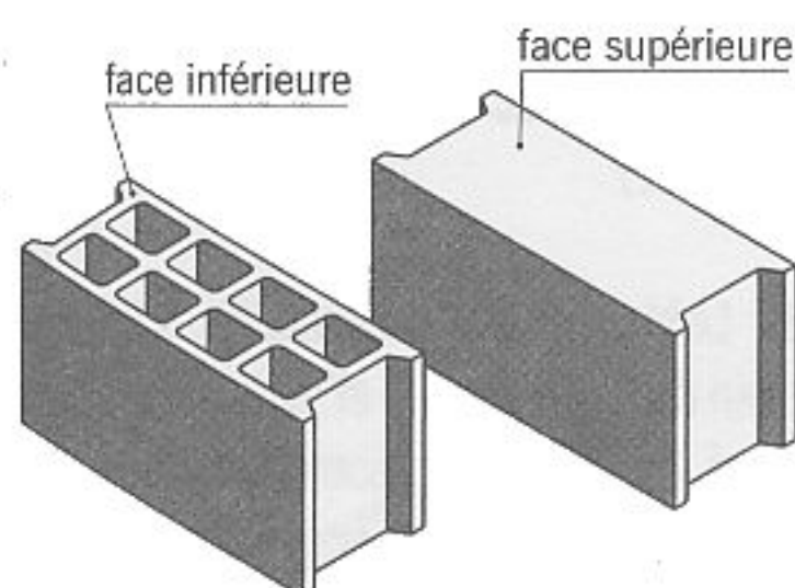
fig. 3.1 bloc creux en béton de granulats
