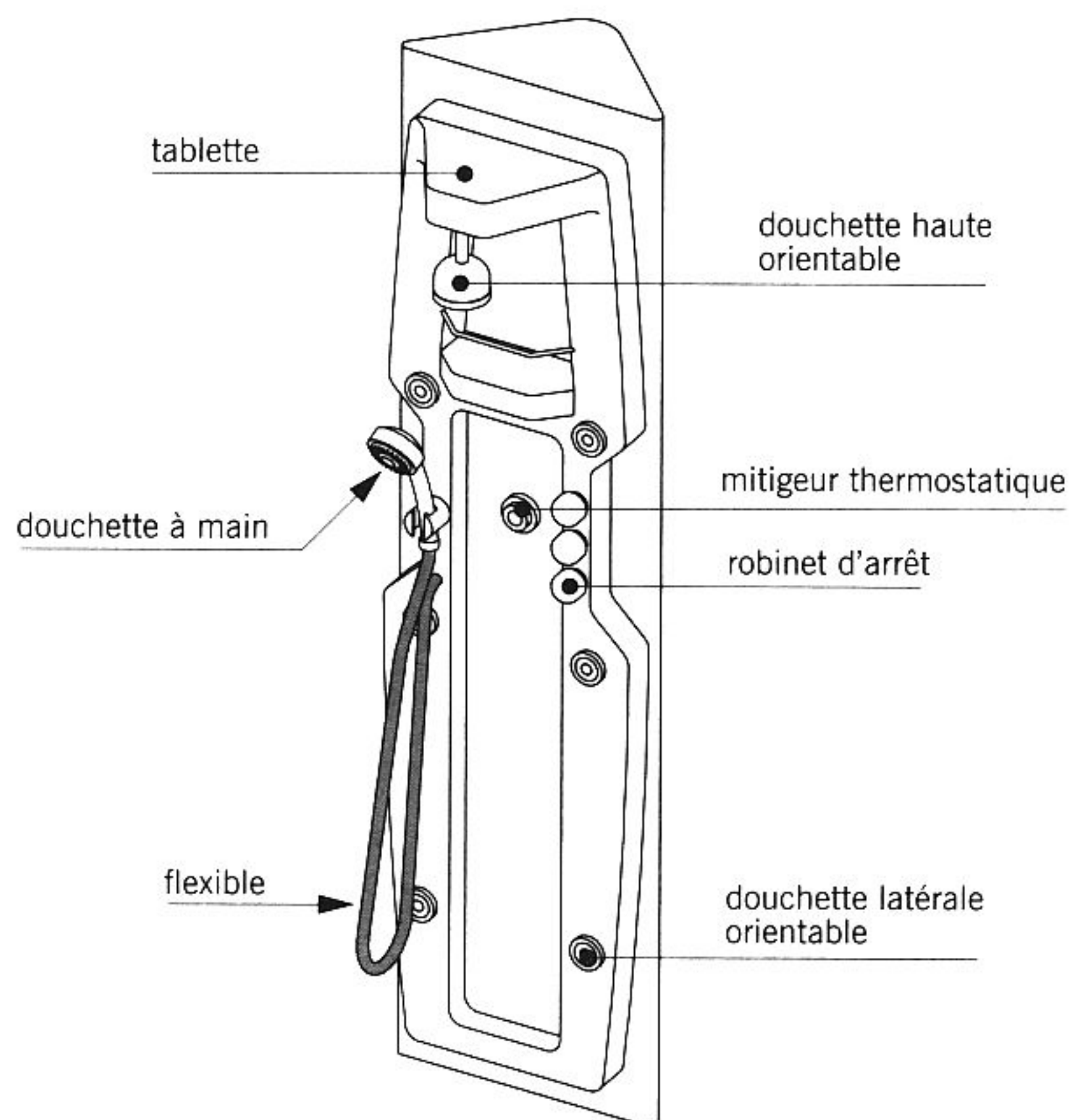
fig. 14.46 colonne de douche
