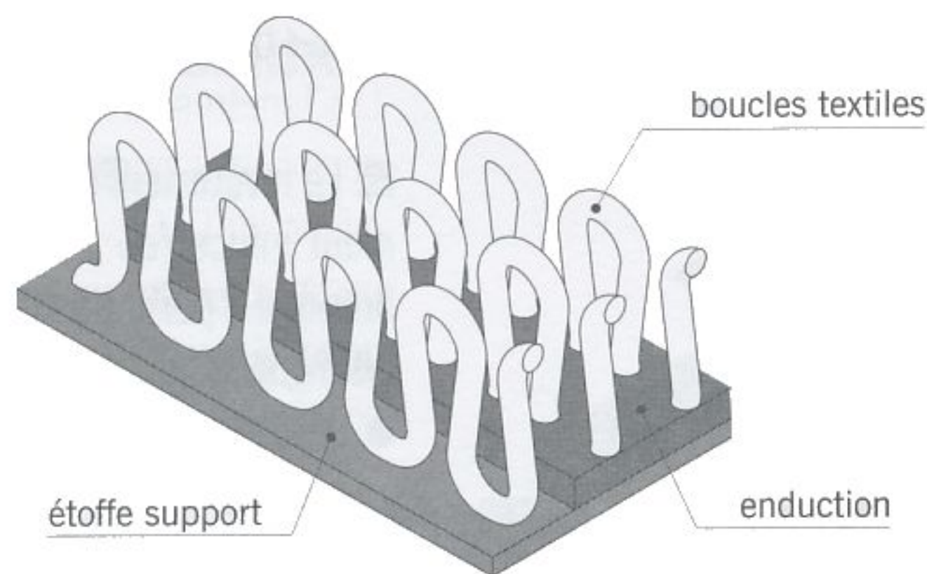
fig. 10.20 moquette tuftée
