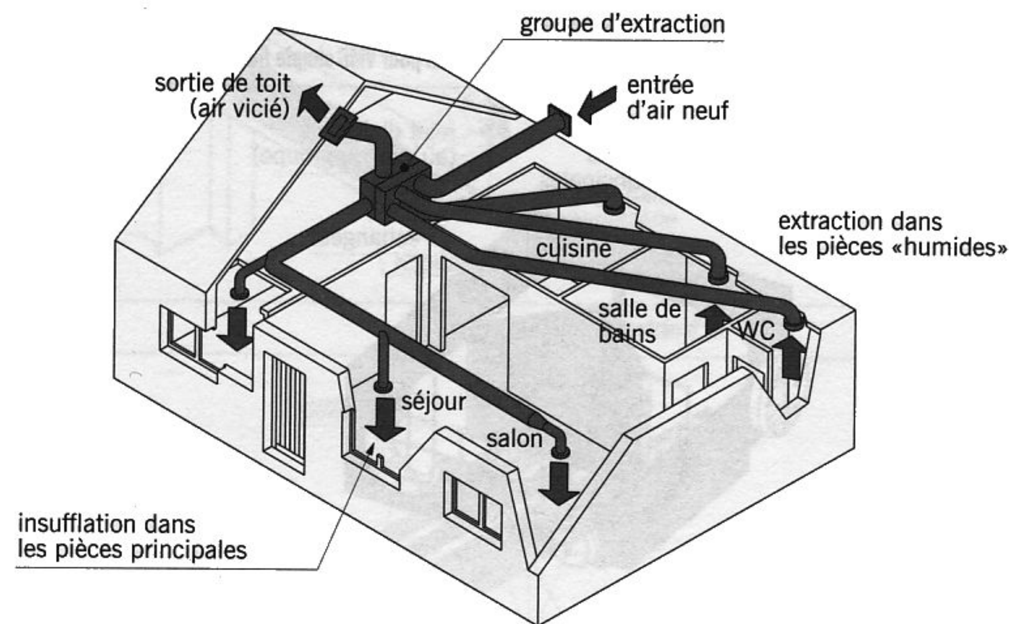
fig. 18.3 VMC à double flux
