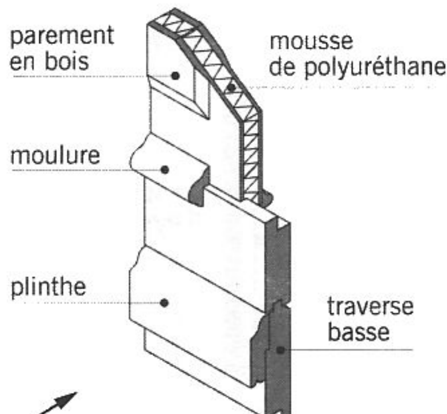
fig. 11.46 porte d'entrée isolante
