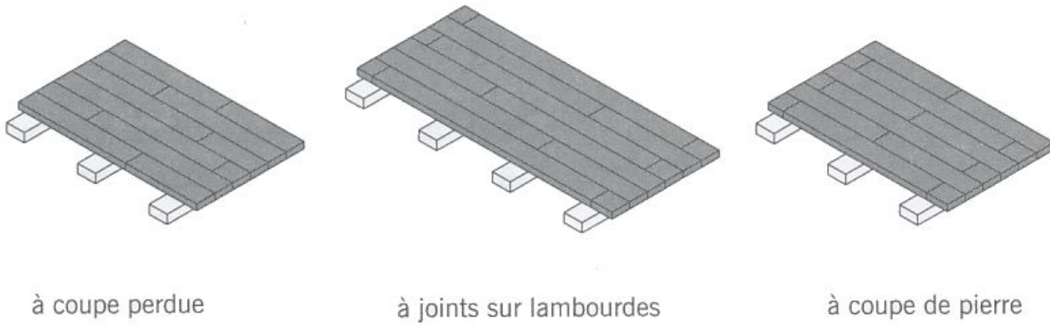
fig. 10.5 parquets à l'anglaise
