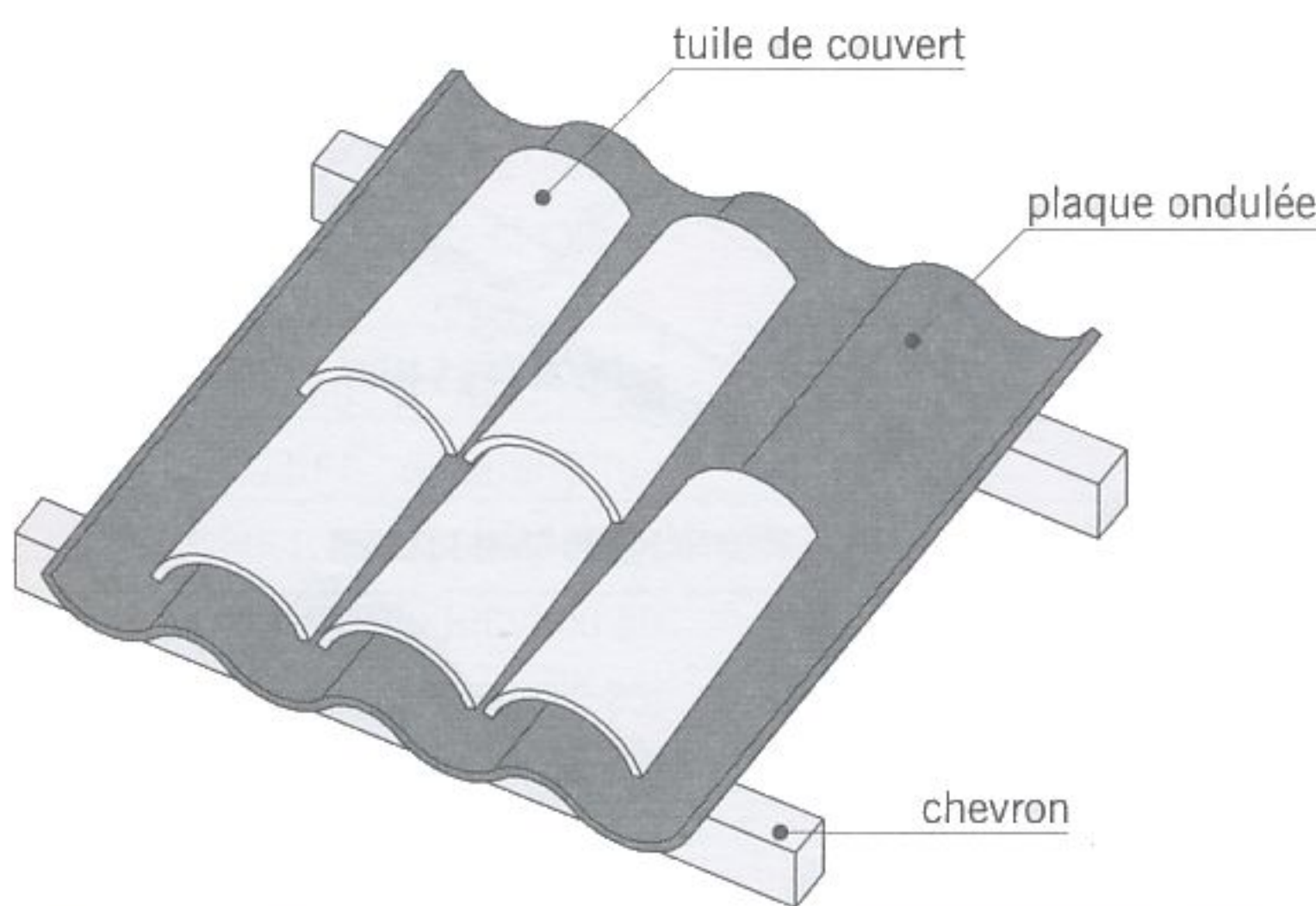
fig. 7.9 tuiles canal posées sur une plaque ondulée
