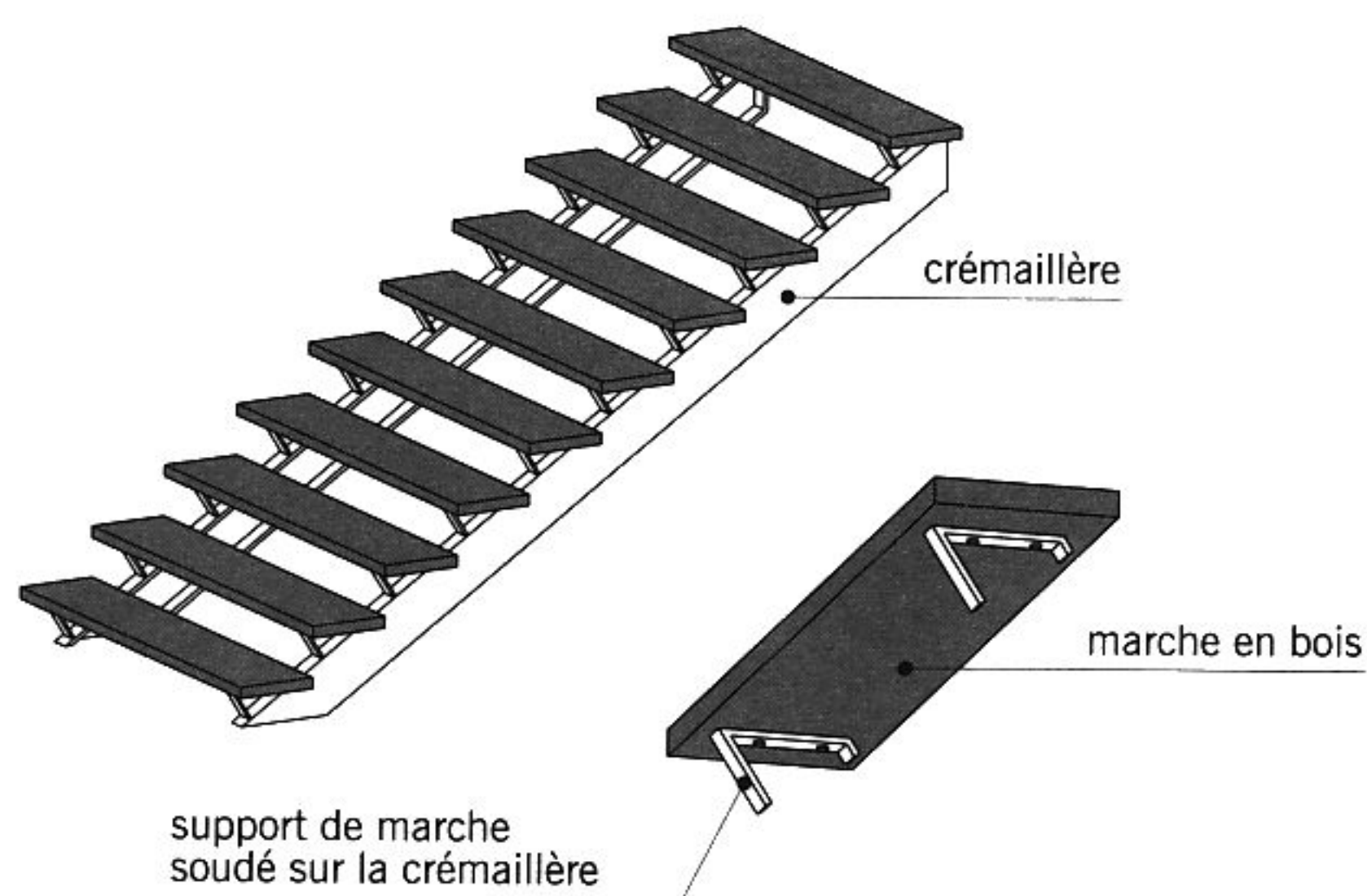
fig. 13.30 escalier à deux crémaillères métalliques
