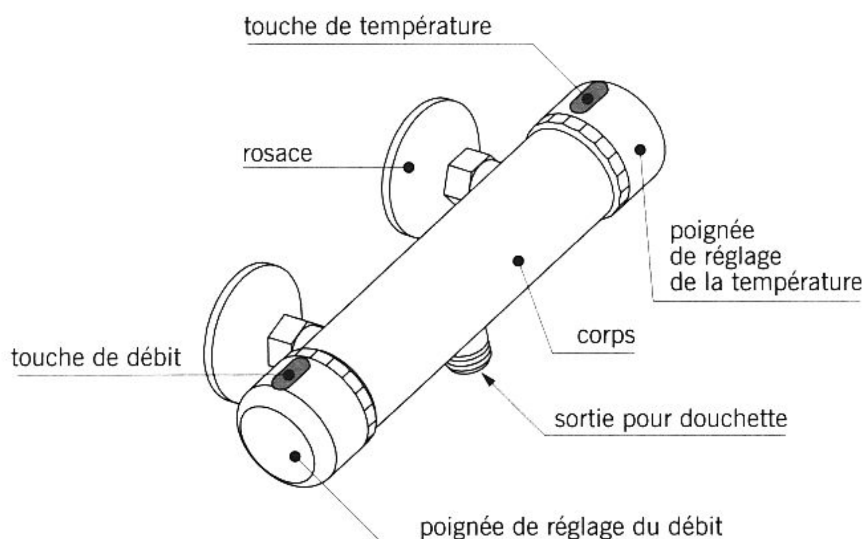
fig. 14.41 mitigeur thermostatique de douche
