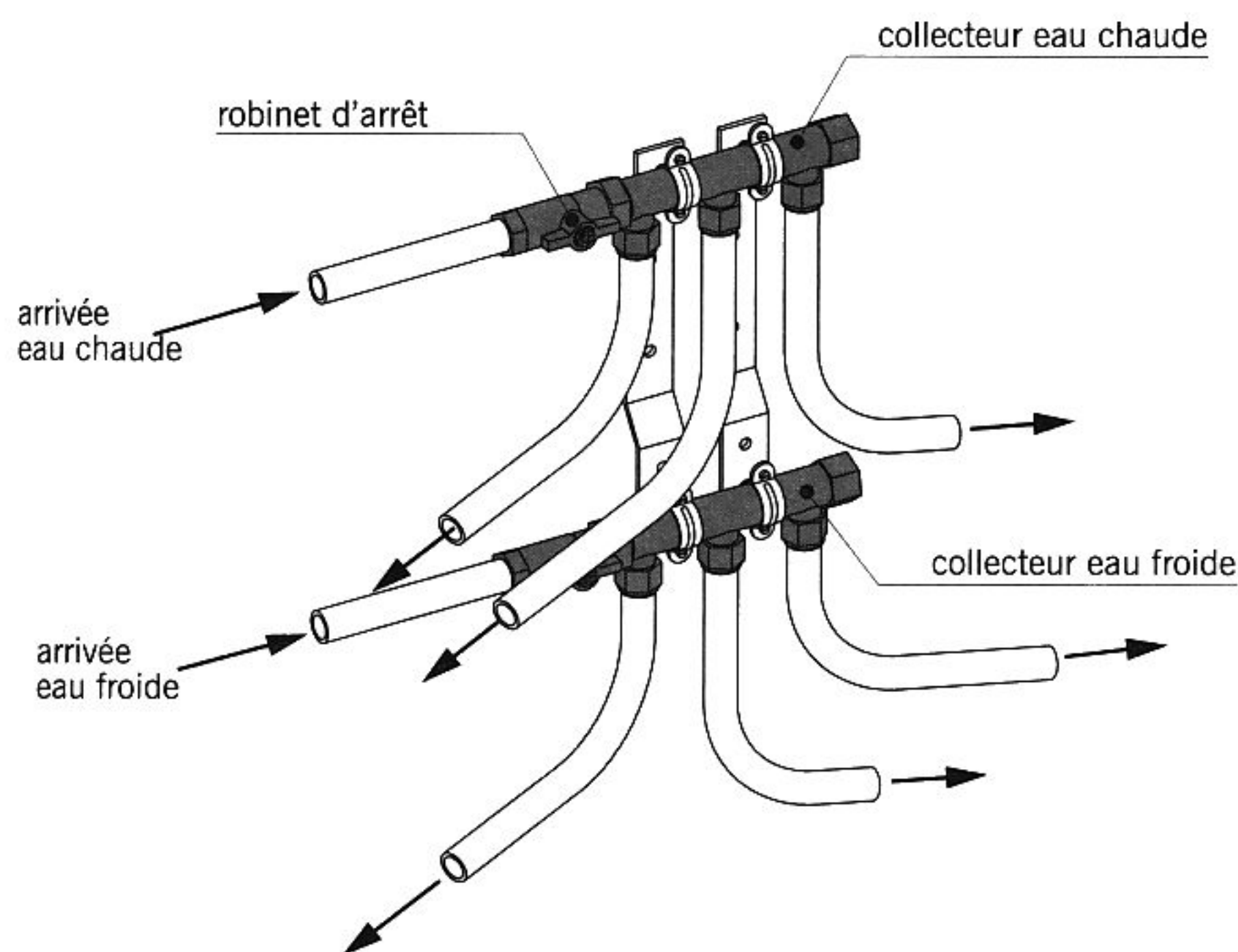
fig. 14.6 exemple de collecteurs pour tubes PER
