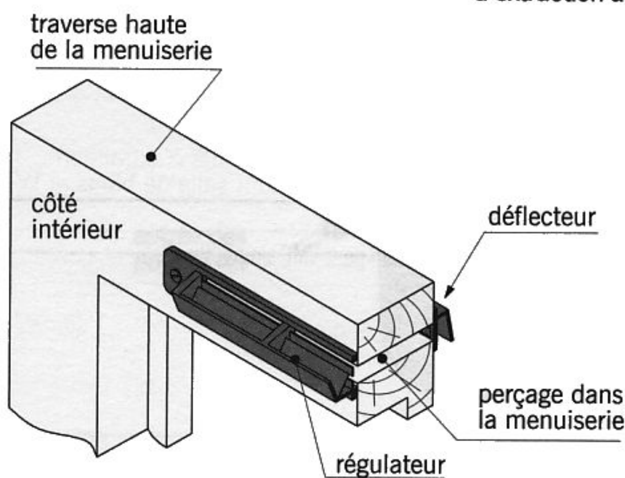
fig. 18.9 mise en place d'une entrée d'air
