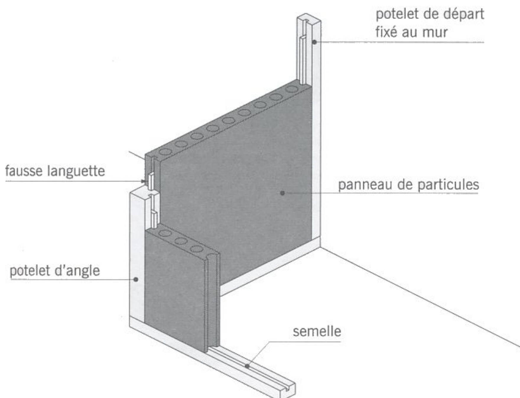
fig. 8.8 cloison sèche en panneaux de particules alvéolés
