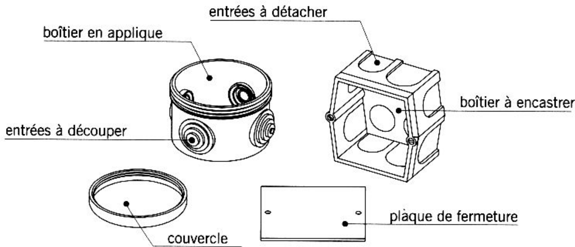
fig. 16.25 boîtes de dérivation
