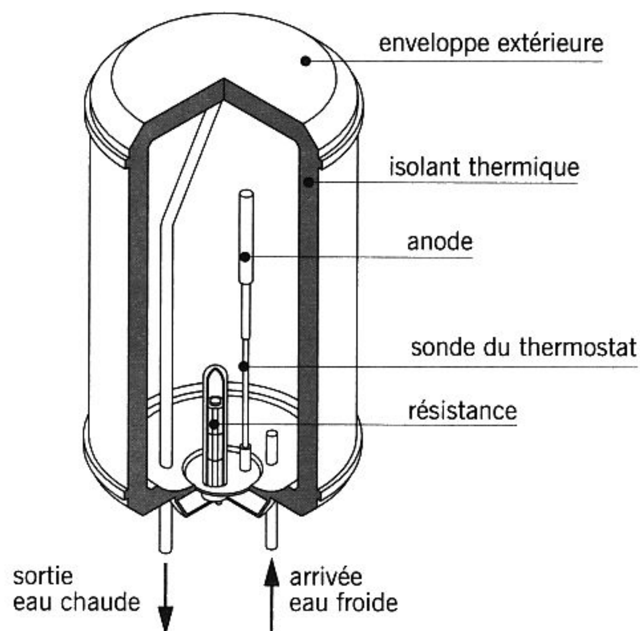
fig. 14.9 chauffe-eau électrique à accumulation
