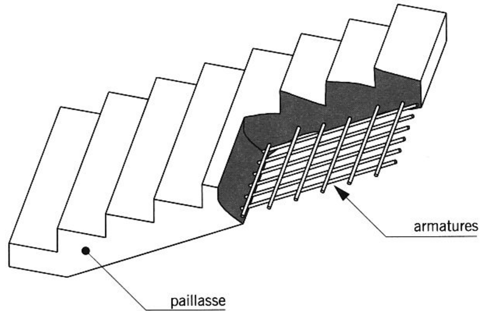
escalier coulé en place
