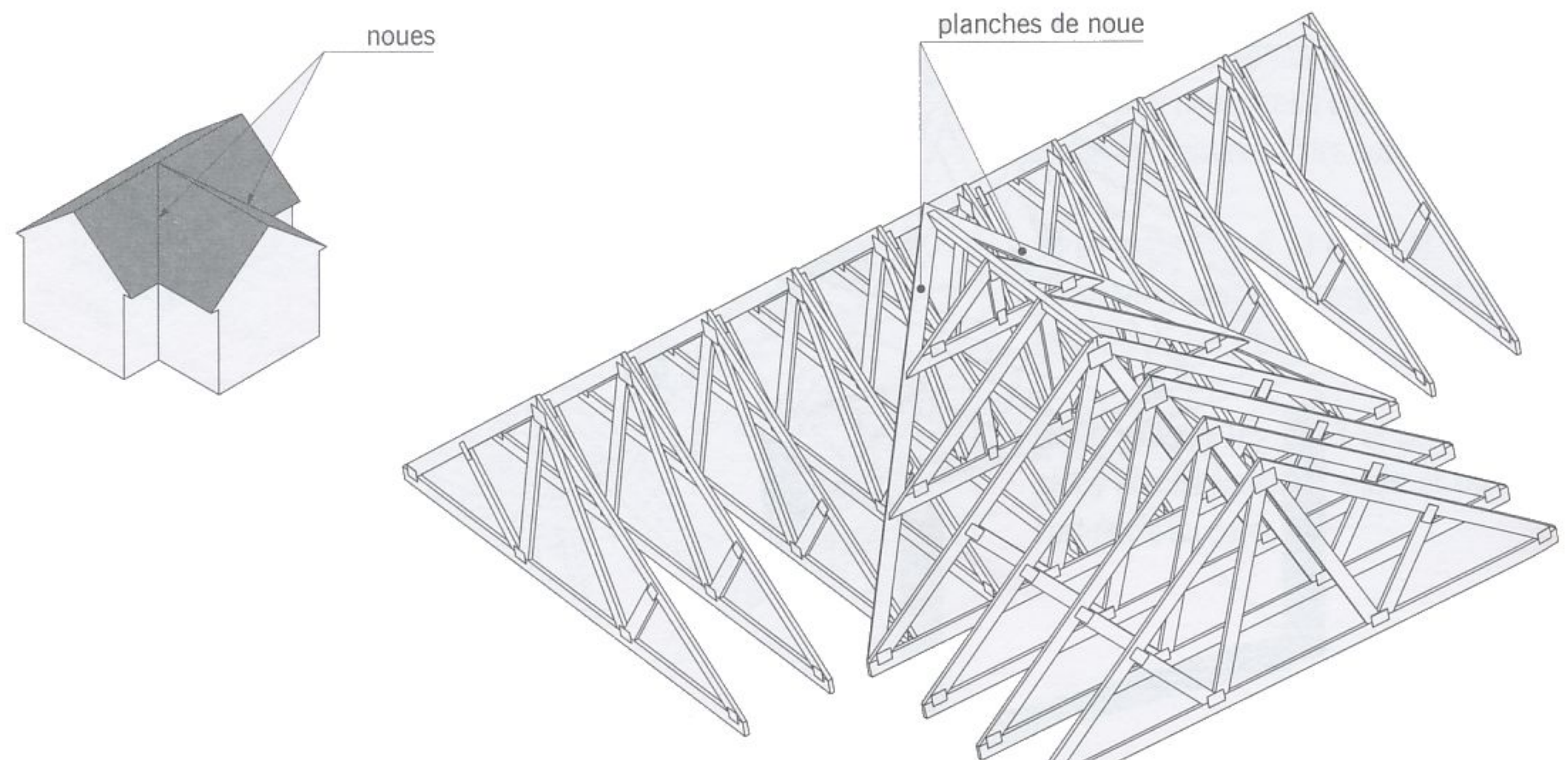
fig. 5.21 vue d'ensemble de la noe
