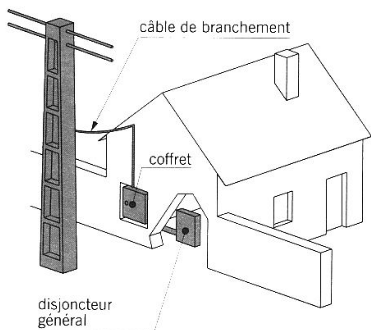
fig. 16.3 branchement aérien
