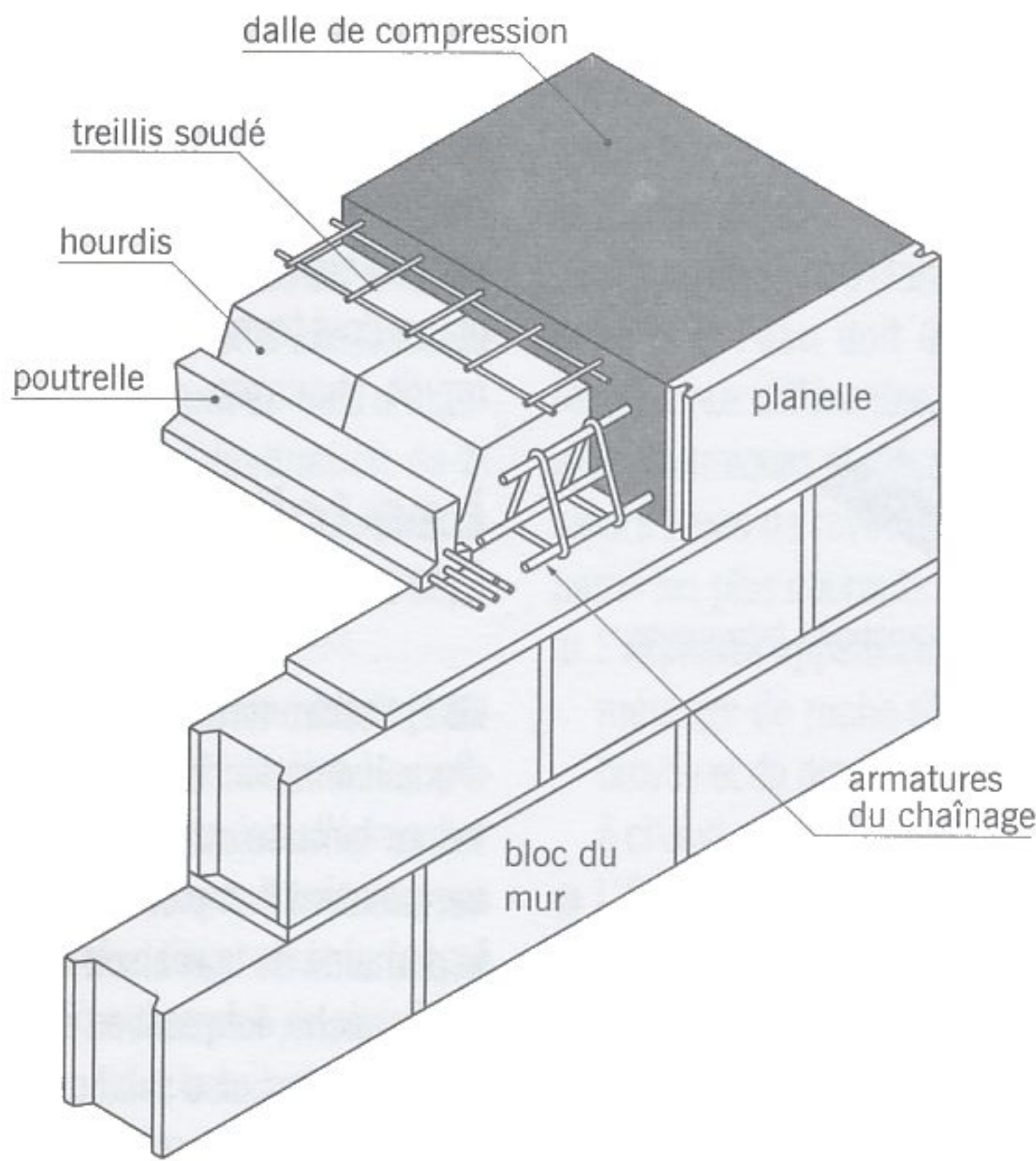
chaînage horizontal
