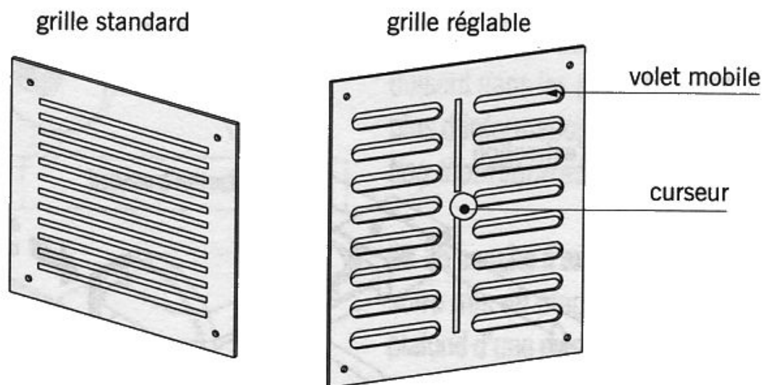
fig. 18.1 grilles de ventilation
