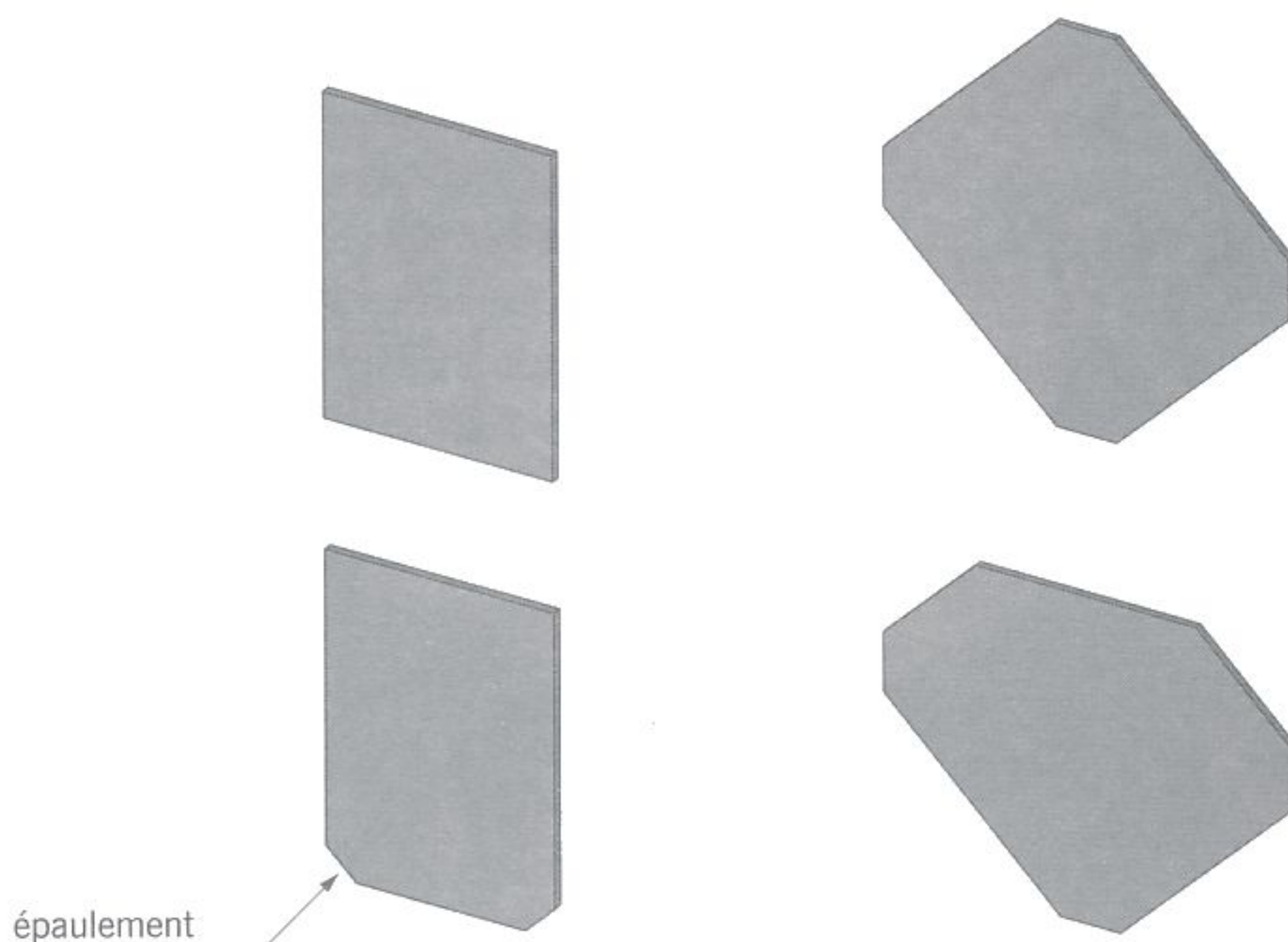
fig. 7.36 ardoises rectangulaires
