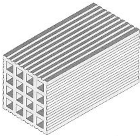
fig. 3.17 brique creuse ordinaire
