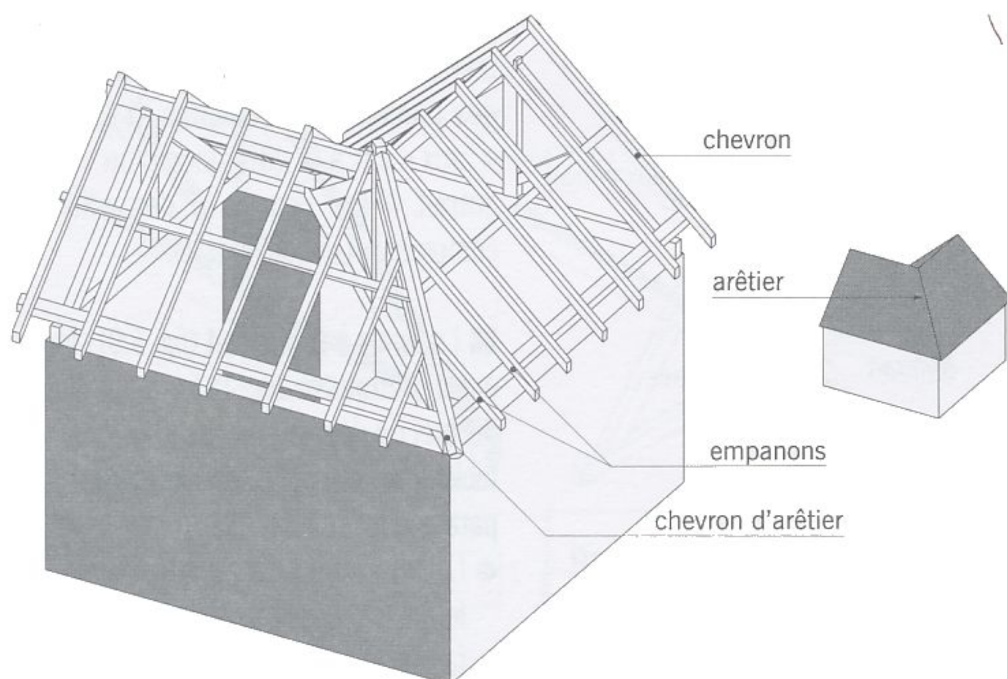
intersection de deux charpentes observée côté arêtier
