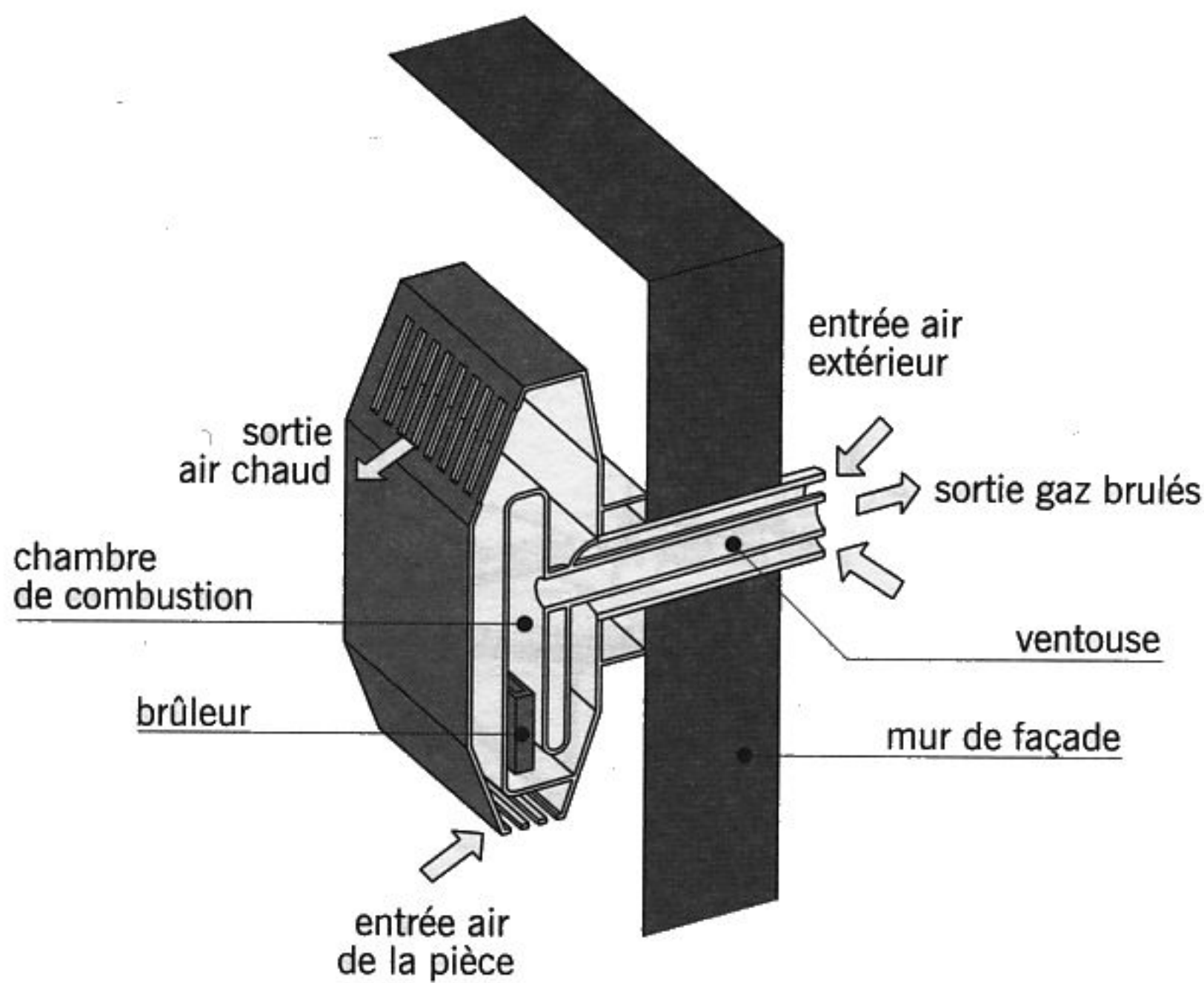
fig. 17.23 radiateur indépendant
