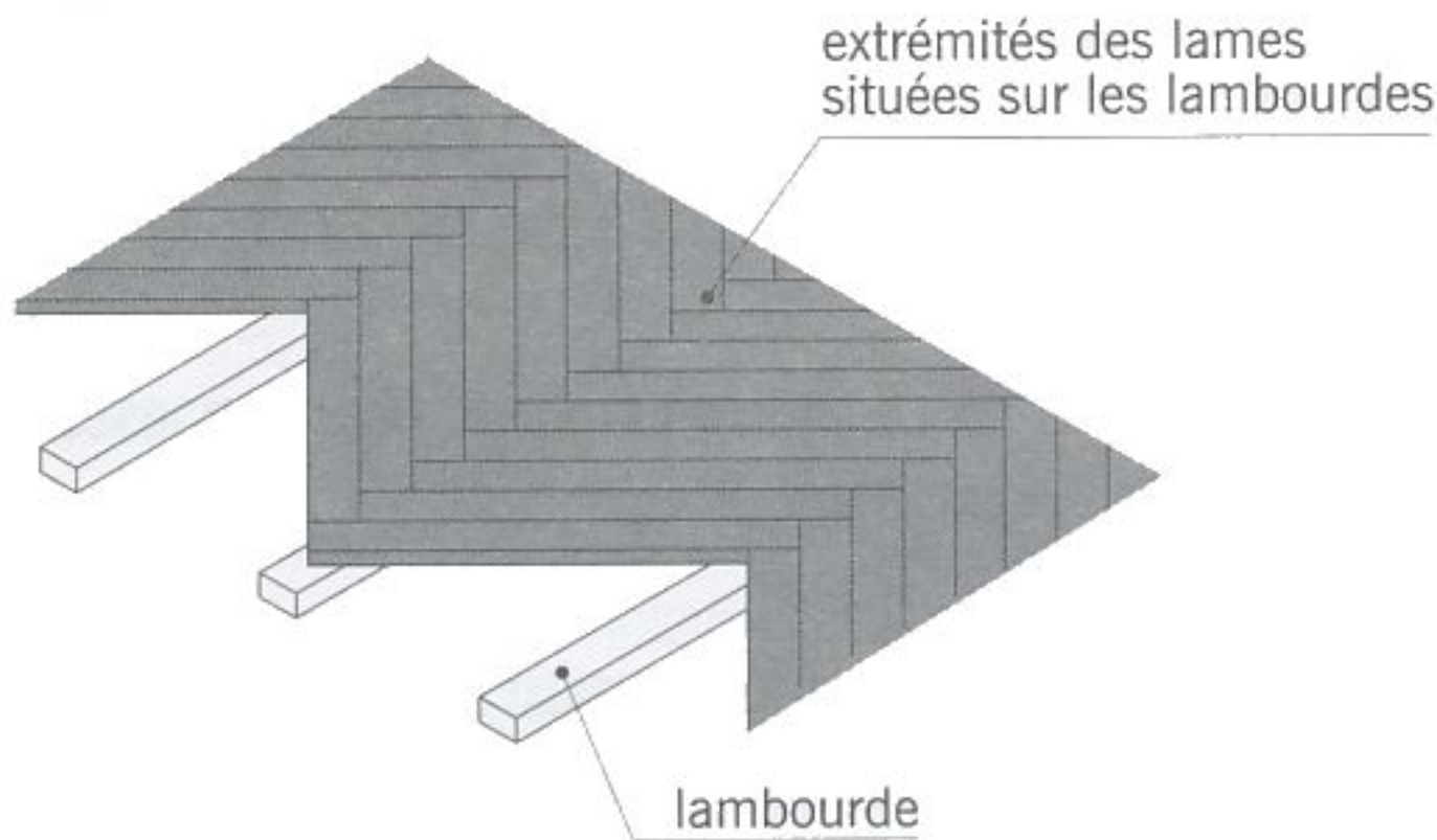
fig. 10.6 parquet à bâtons rompus
