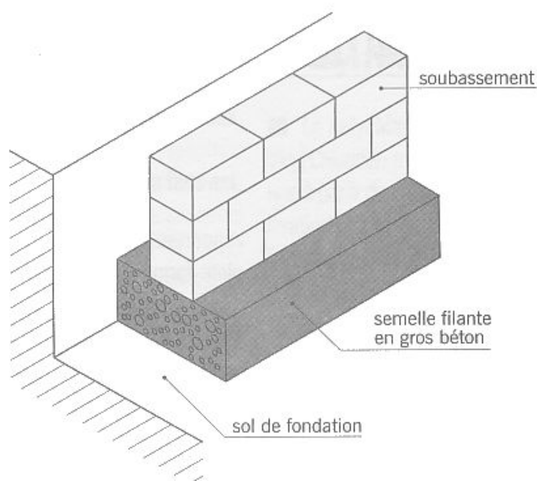
semelle filante non armée
