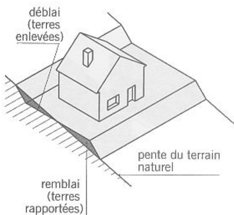
fig. 2.2 déblai et remblai
