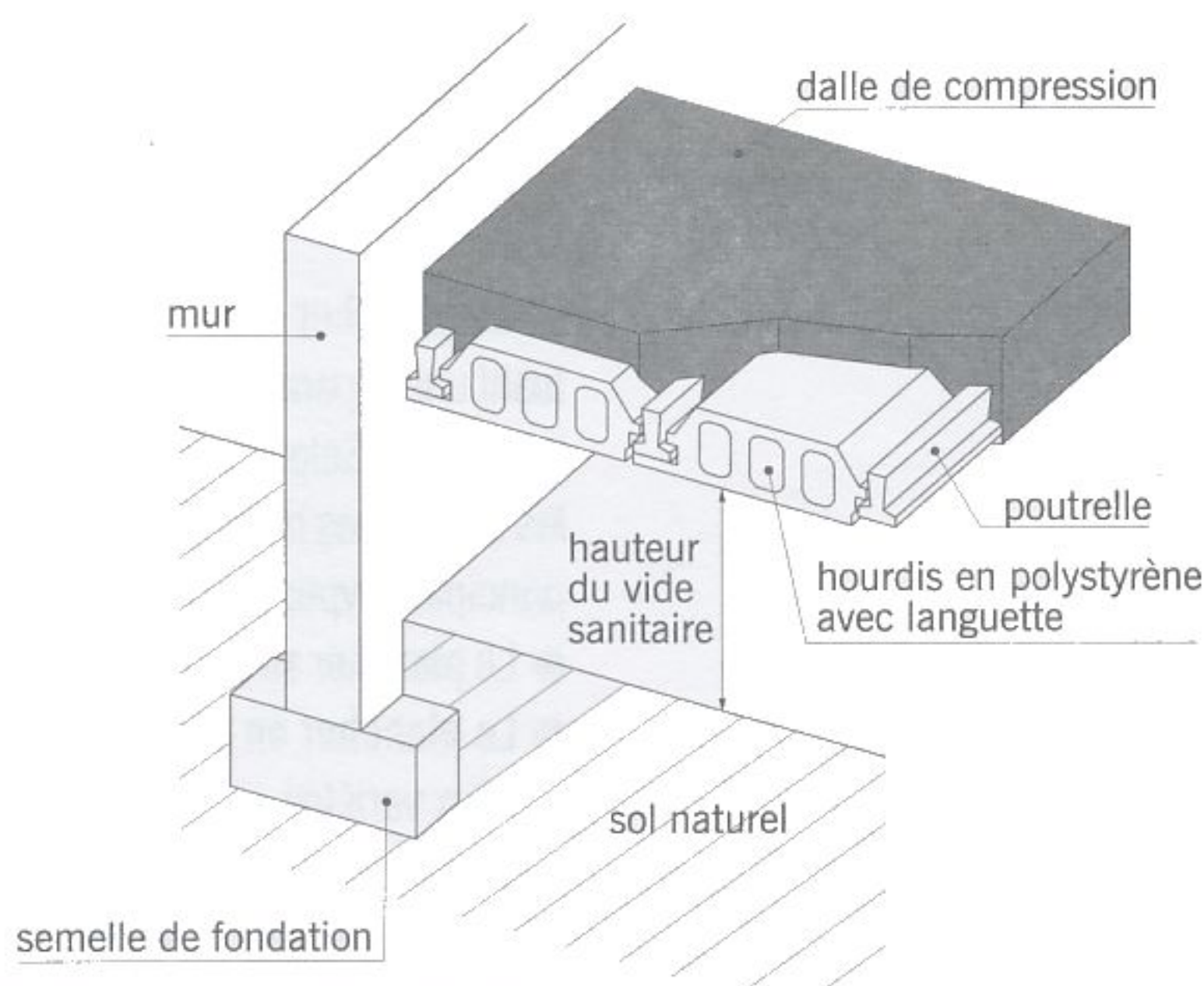
plancher sur vide sanitaire
