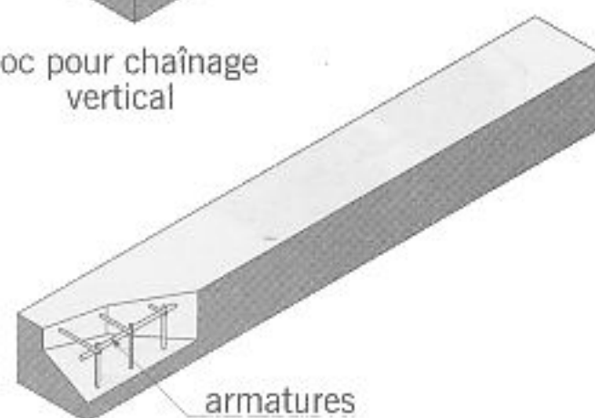
bloc linteau porteur
