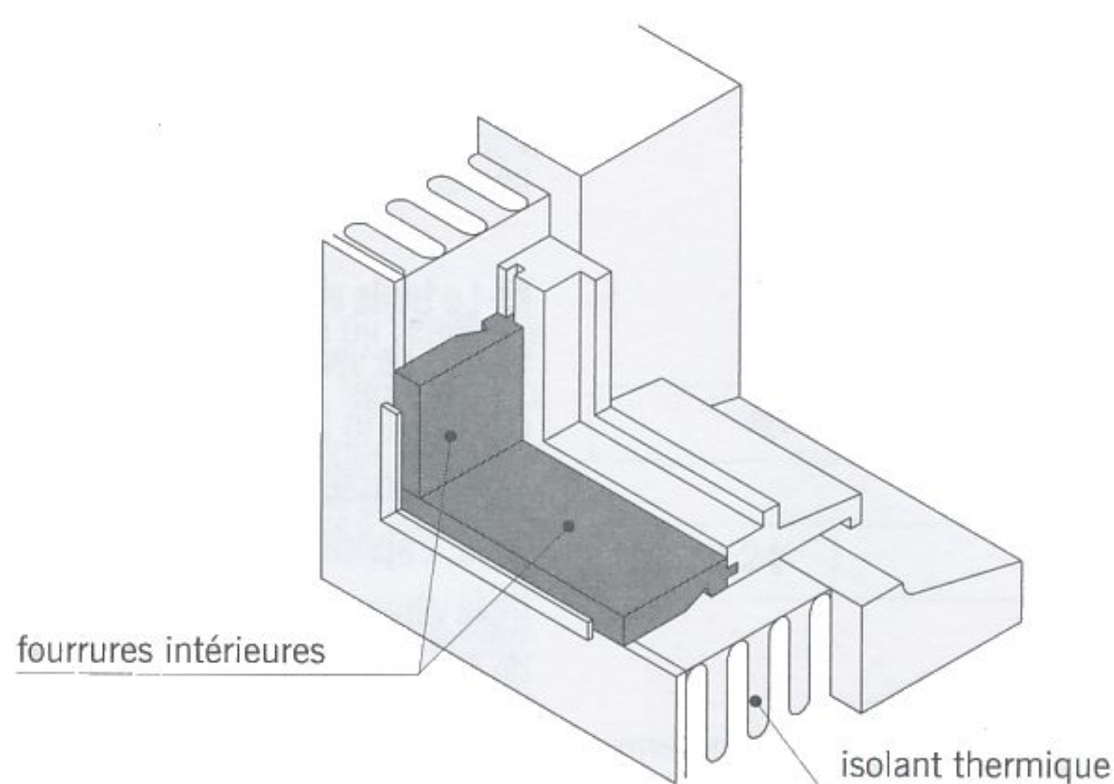
fig. 11.17 fourrure intérieure (cadre ouvrant non représenté)
