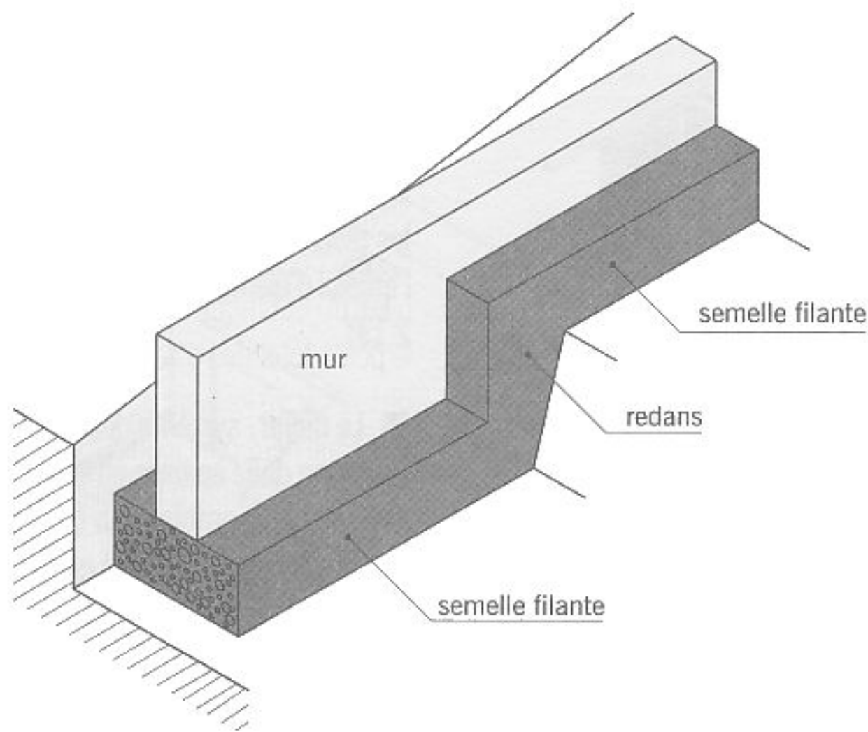
fig. 2.7 semelle à redans
