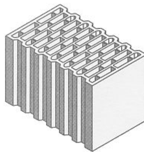
fig. 3.10 bloc perforé en terre cuite
