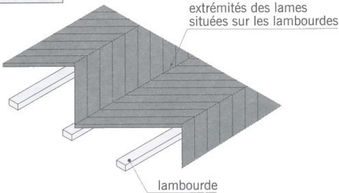
fig. 10.7 parquet en point de Hongrie
