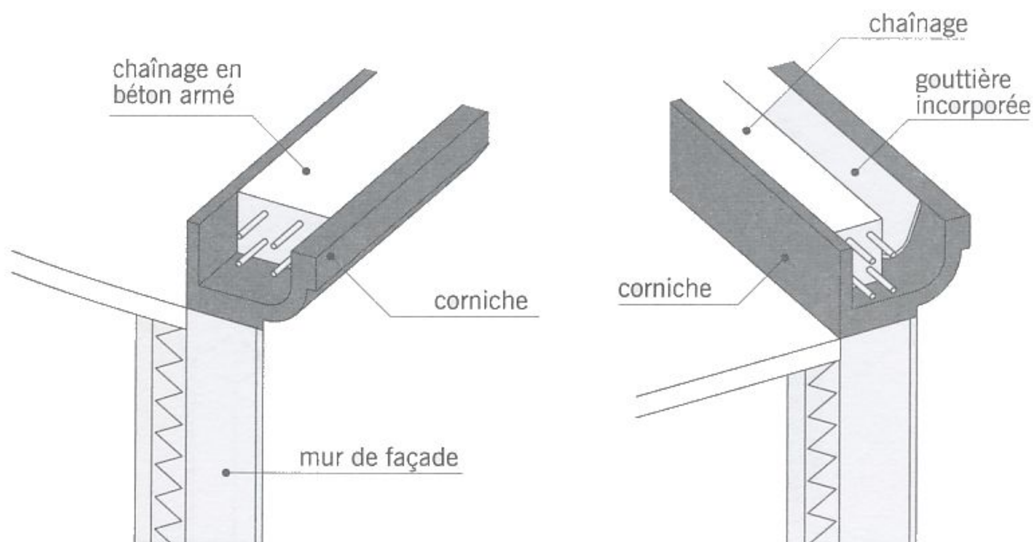
fig. 3.46 corniches
