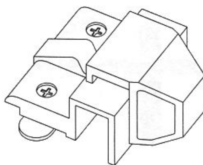
fig. 11.42 loqueteau pour menuiserie en aluminium
