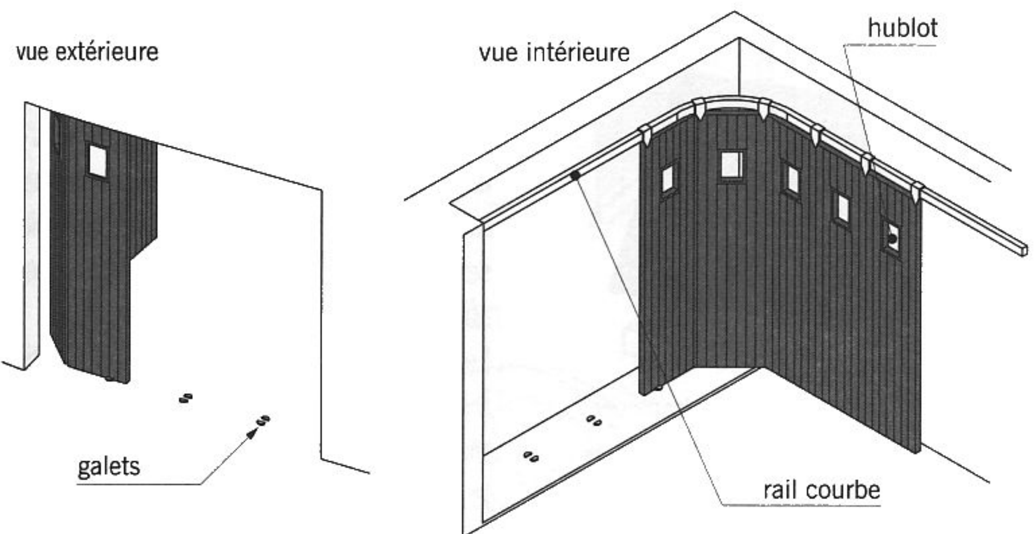
fig. 11.58 porte coulissante
