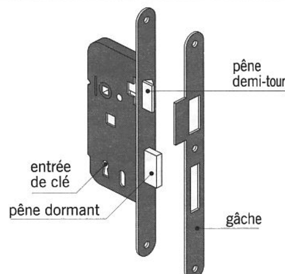
fig. 12.19 serrure à larder à deux pènes
