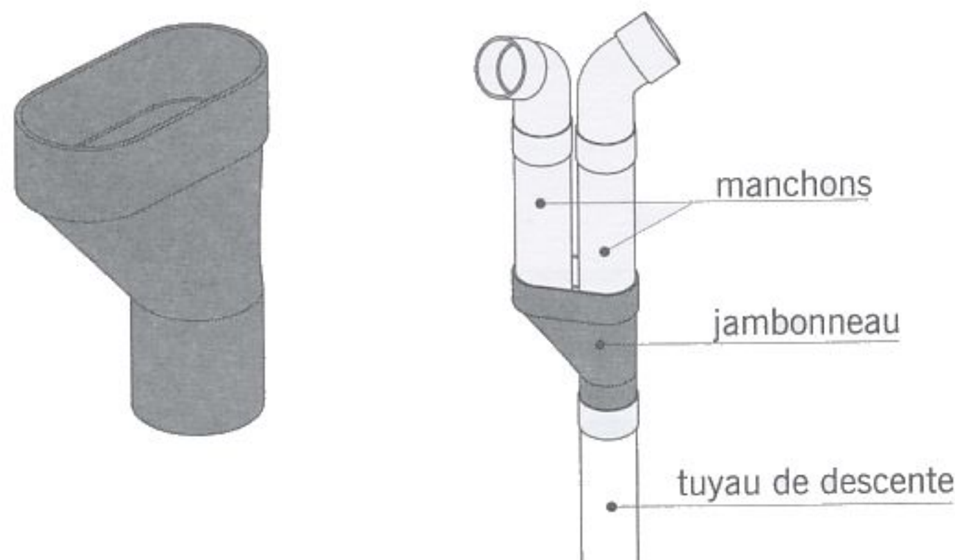
fig. 7.65 jambonneau
