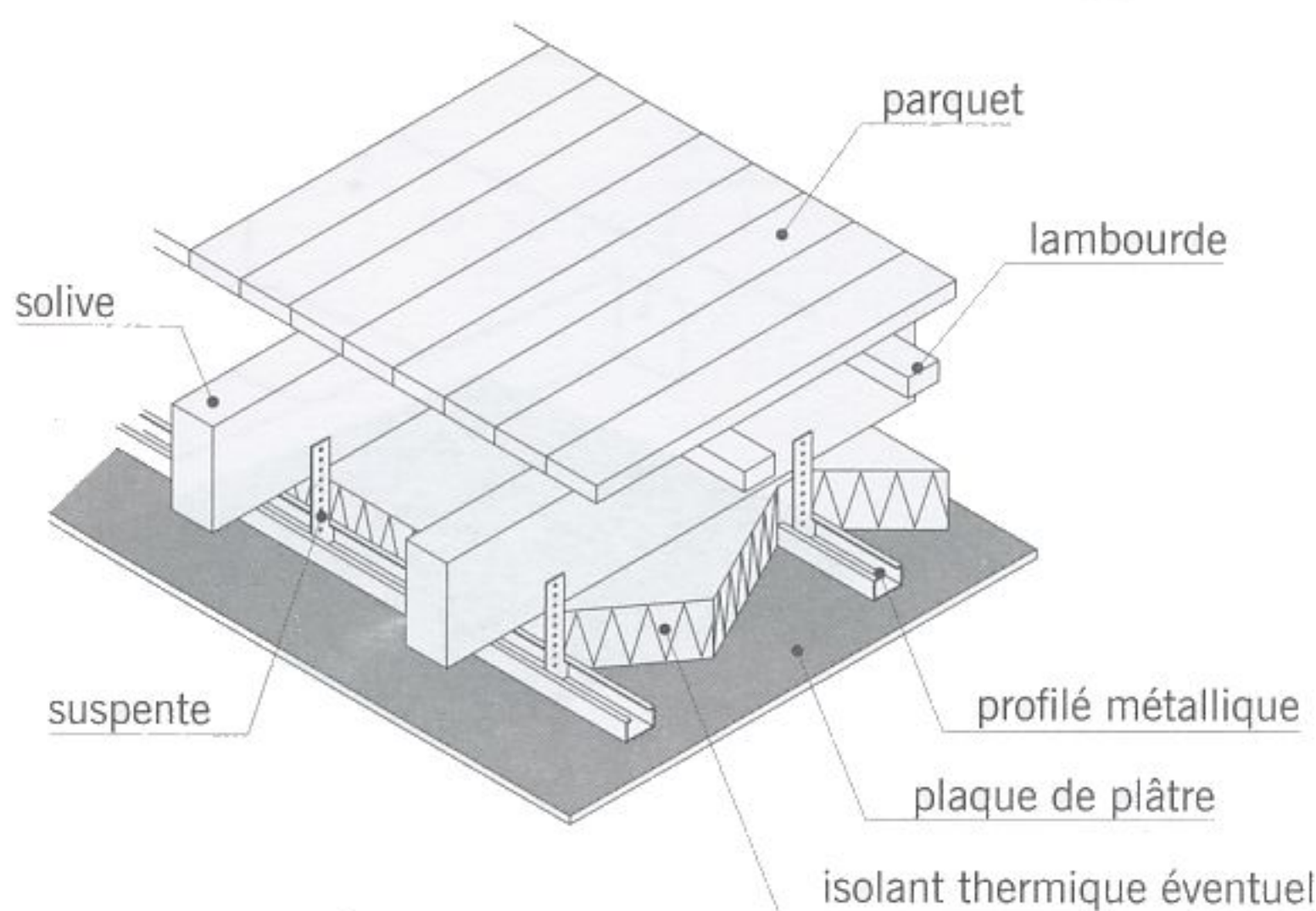
fig. 9.4 plafond suspendu sous plancher en bois
