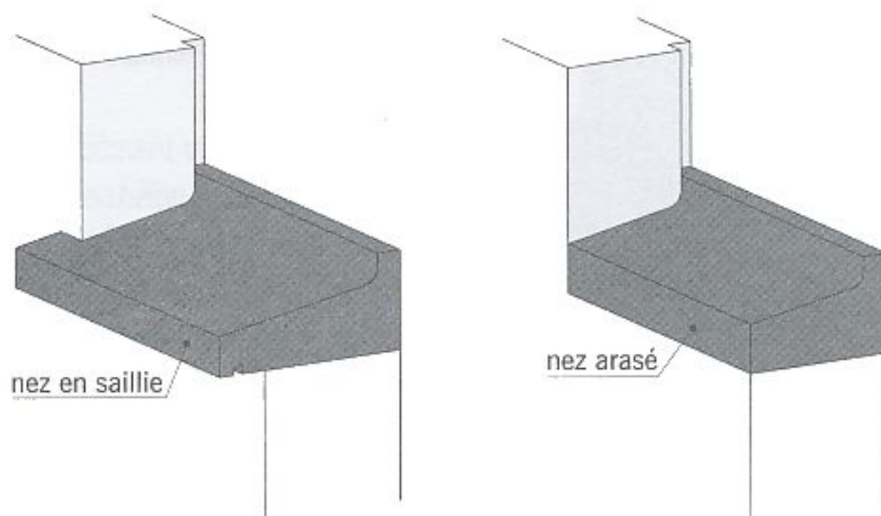
fig. 3.33 nez d'appui
