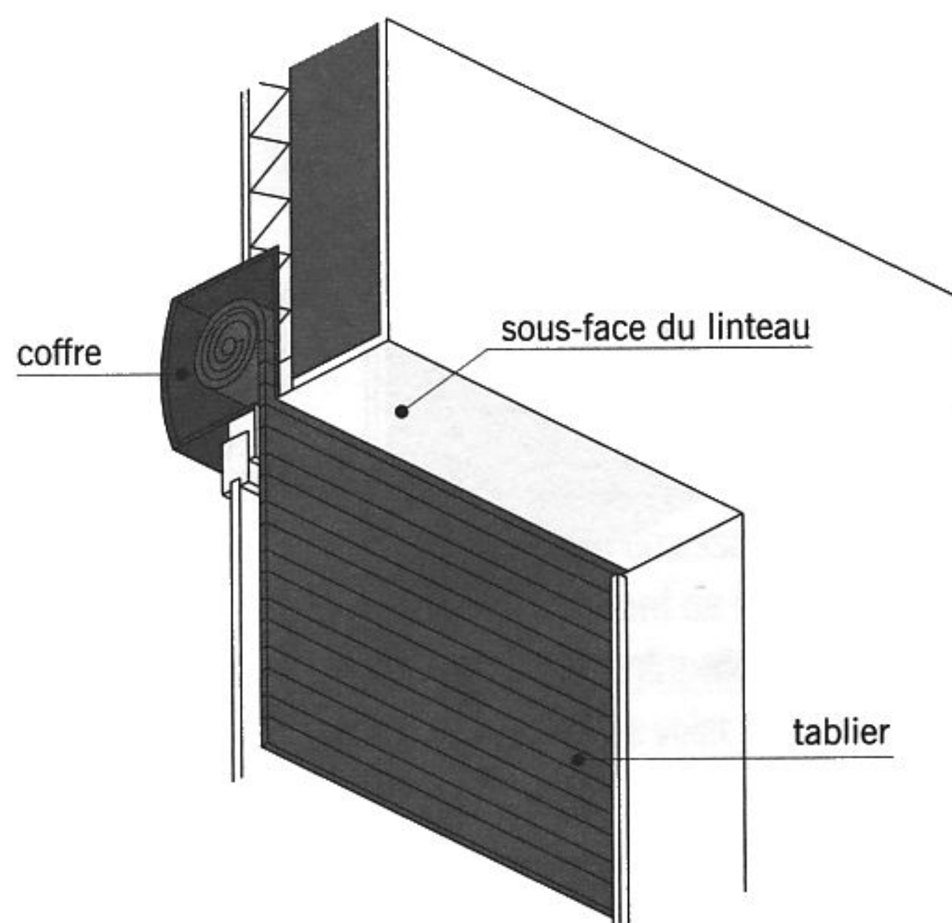
coffre apparent à l'intérieur
