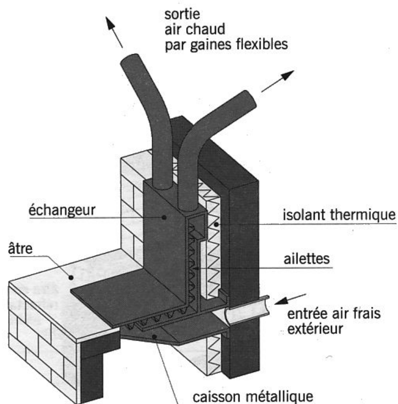
fig. 17.39 échangeur à ailettes
