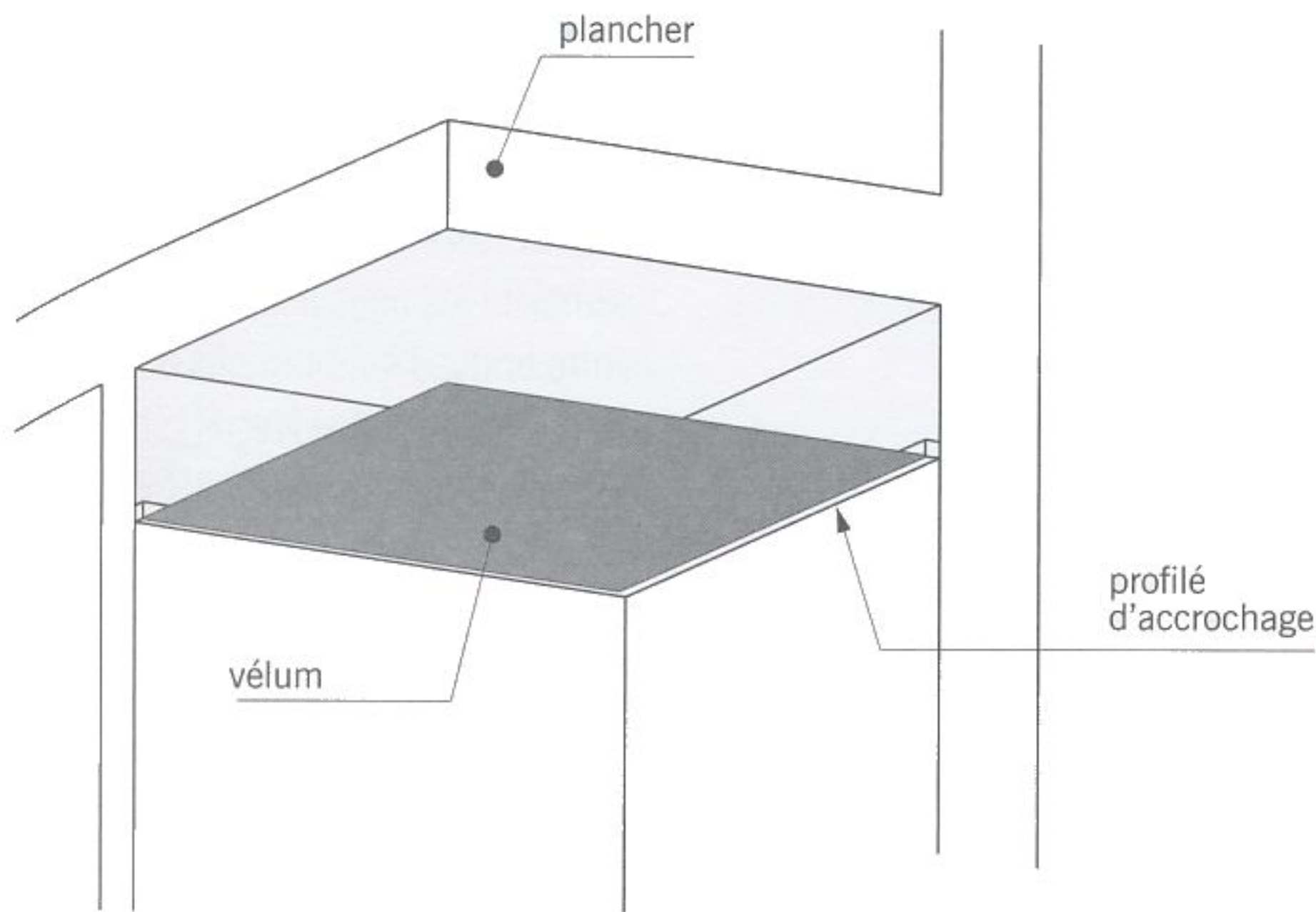
fig. 9.11 plafond tendu
