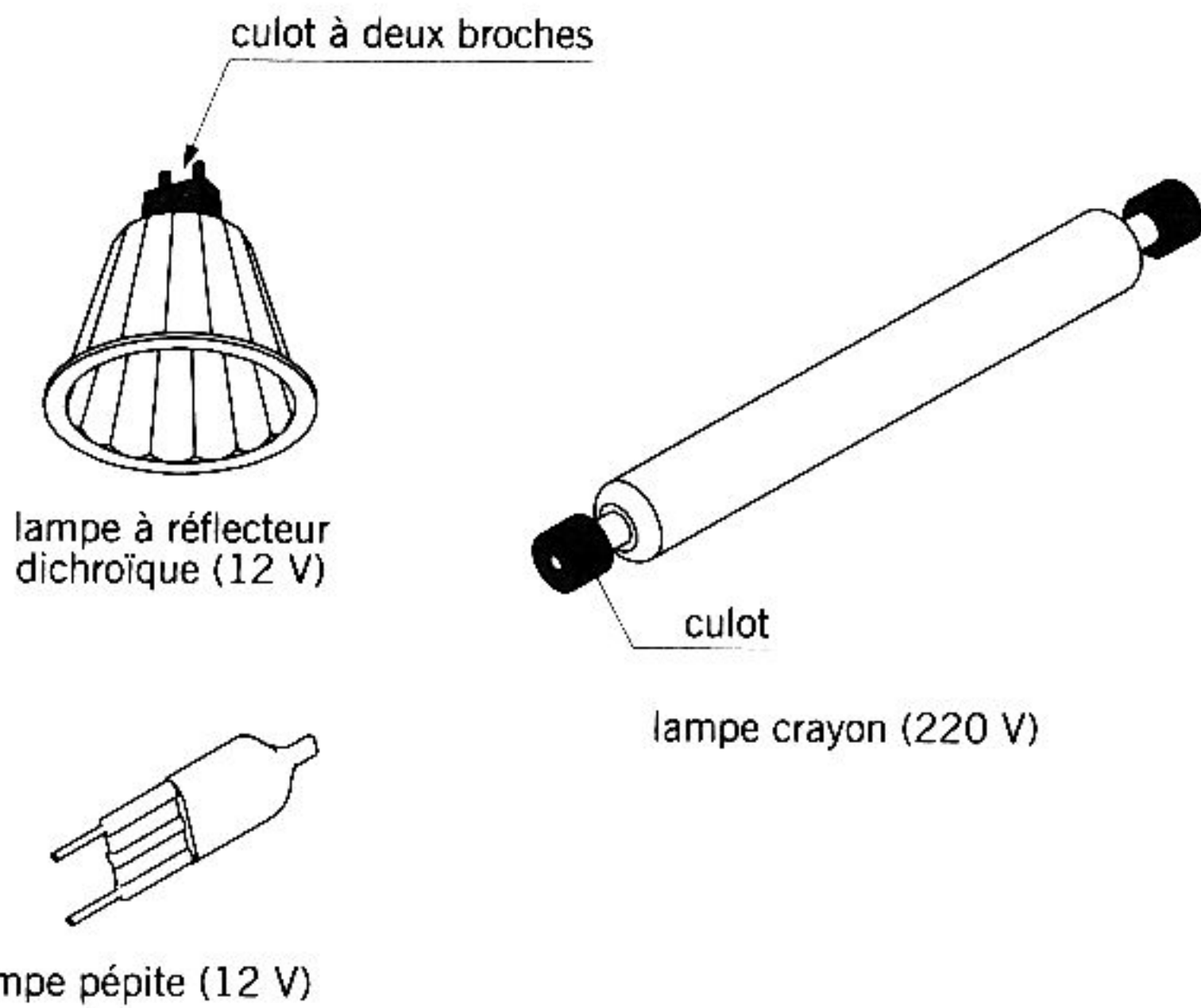
fig. 16.32 lampes halogènes
