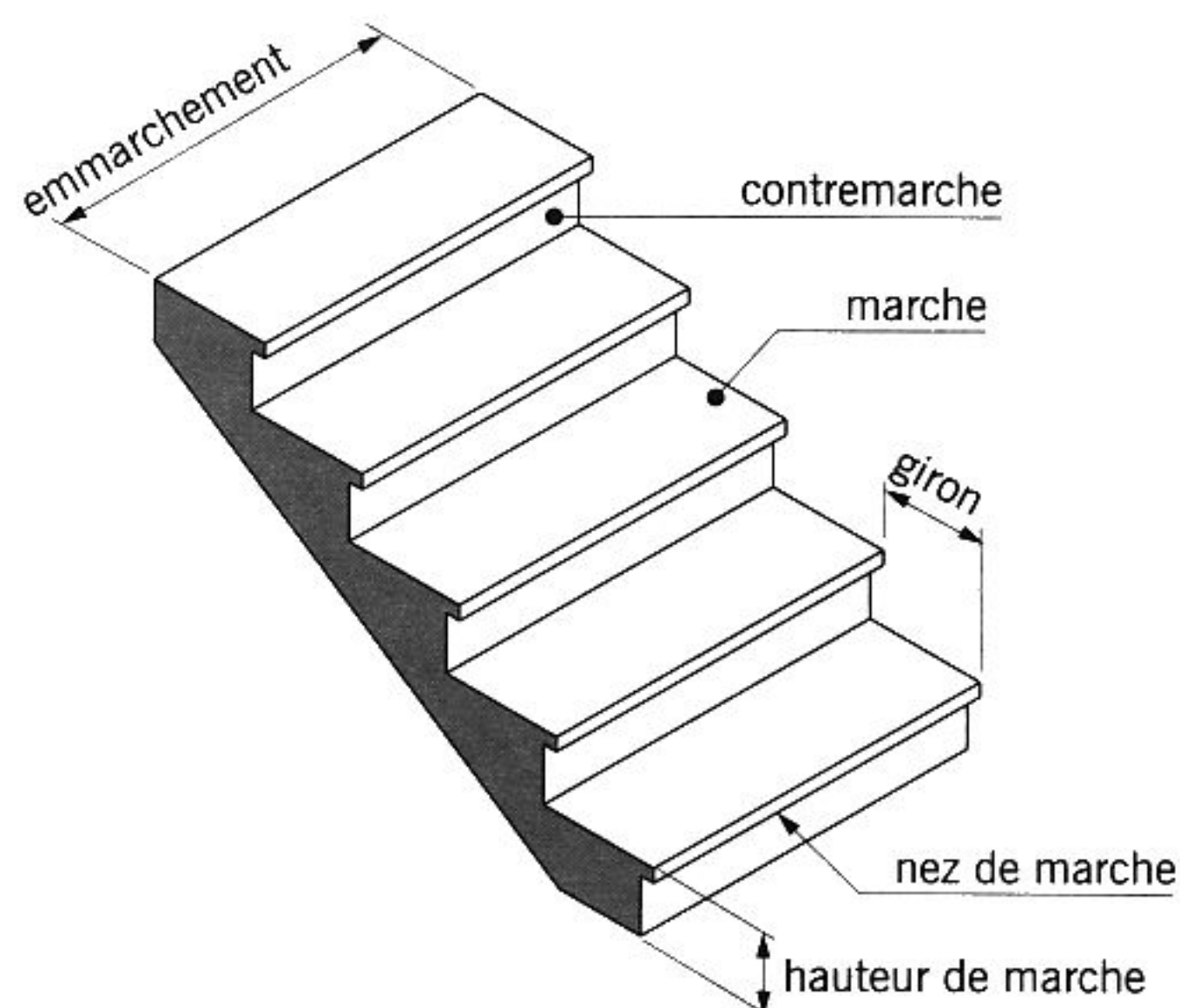
fig. 13.1 volée d'escalier
