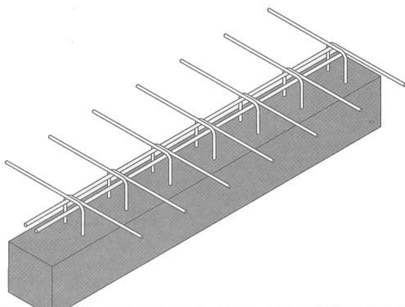
longrine intermédiaire
