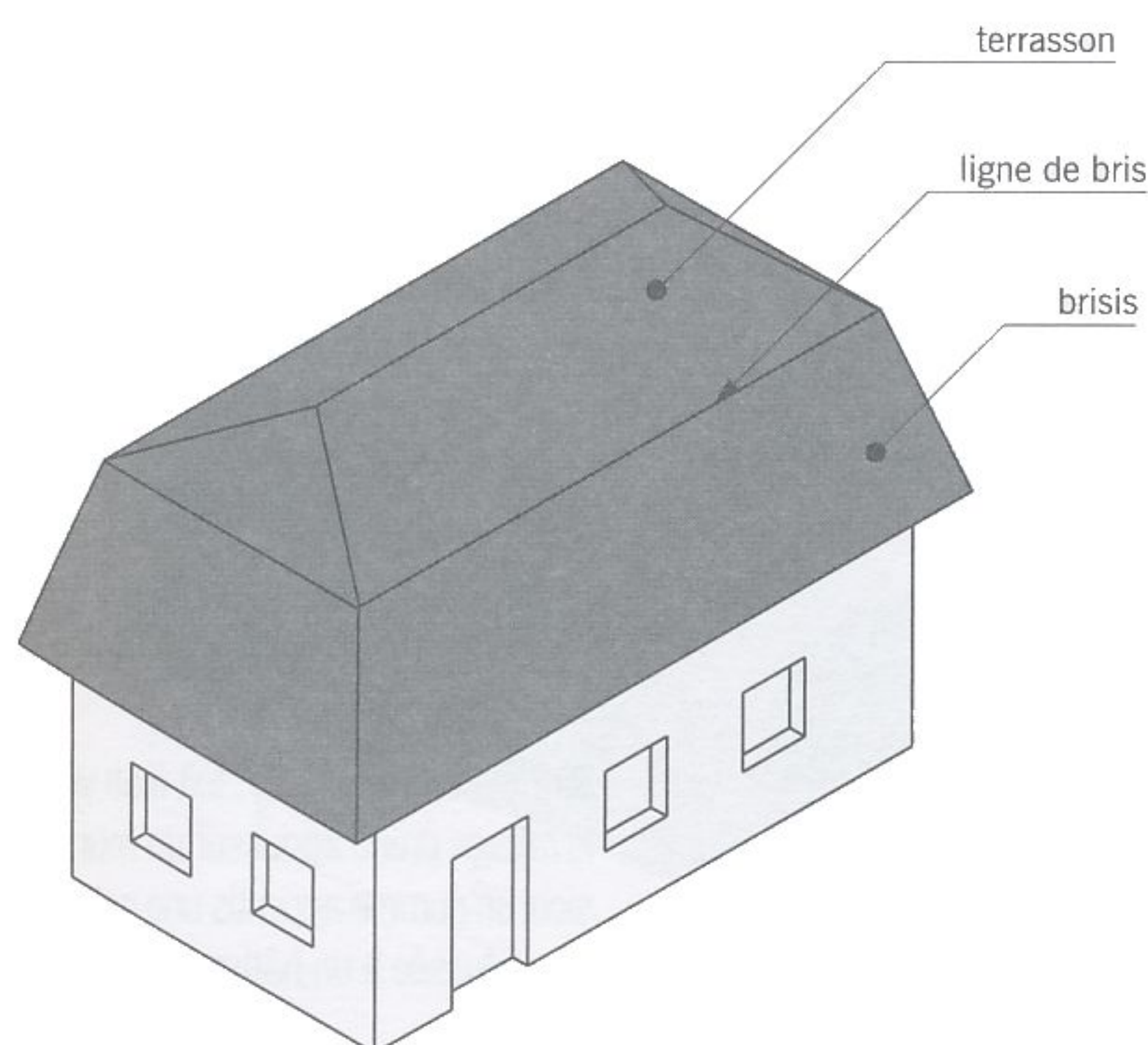
fig. 6.2 comble à la Mansart
