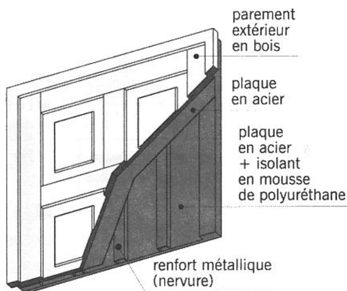
fig. 11.45 détail d'une porte blindée
