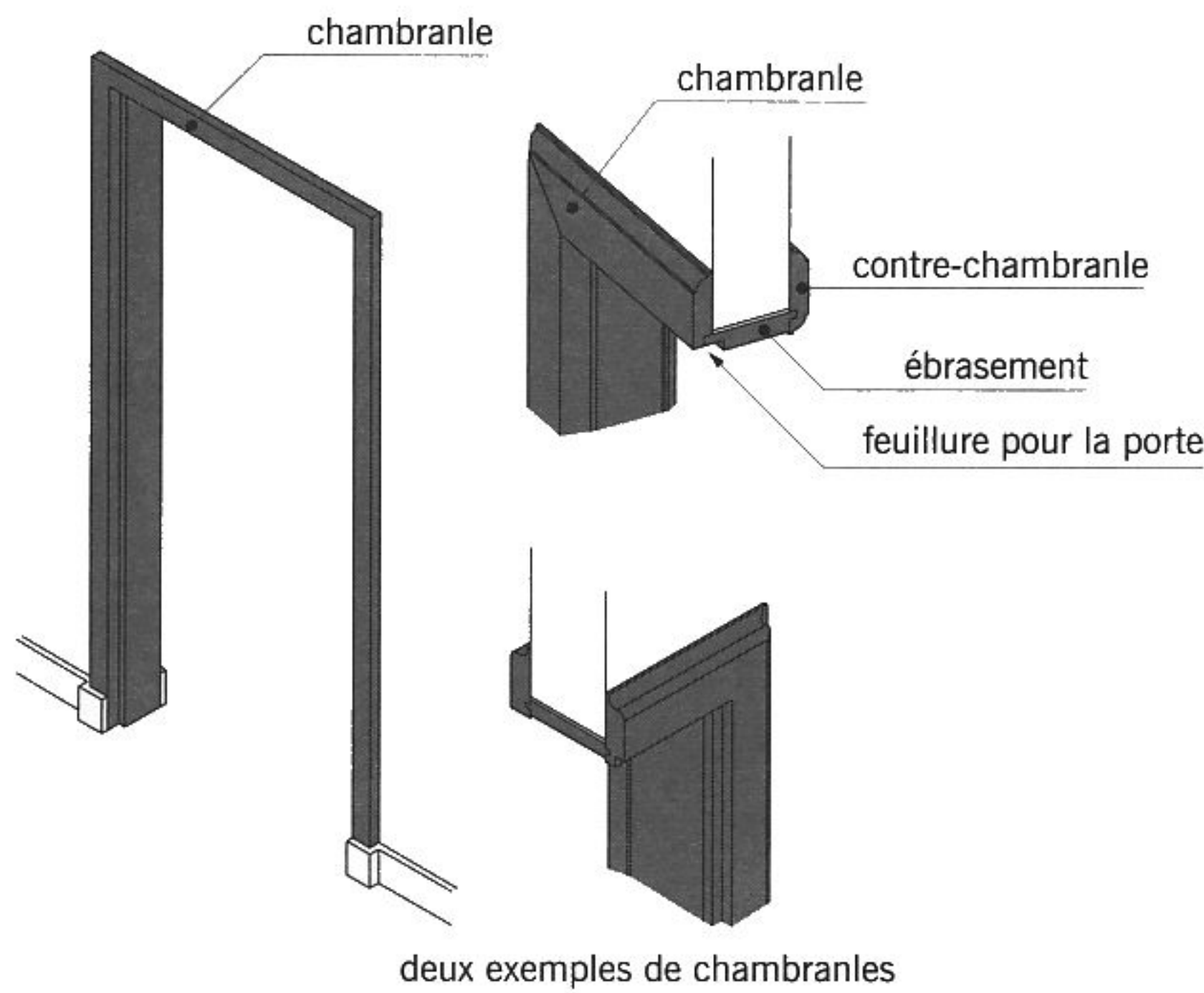
fig. 12.8 chambranles
