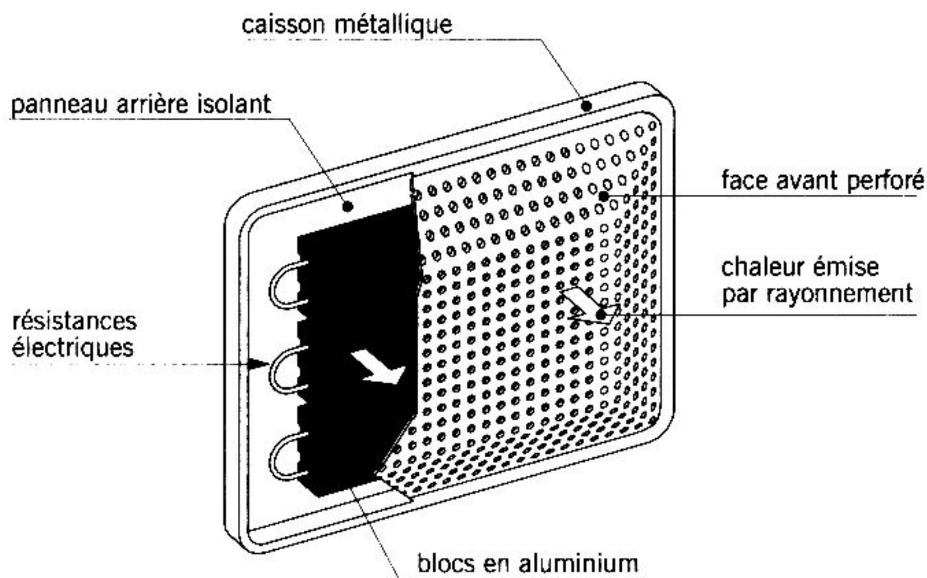
fig. 17.6 panneau radiant
