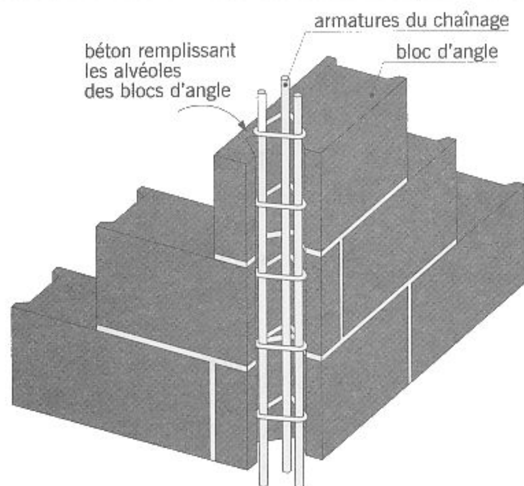
vue intérieure d'un chaînage vertical
