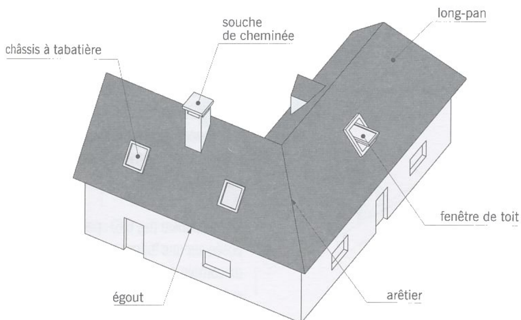
fig. 6.7 mots de la toiture (2)
