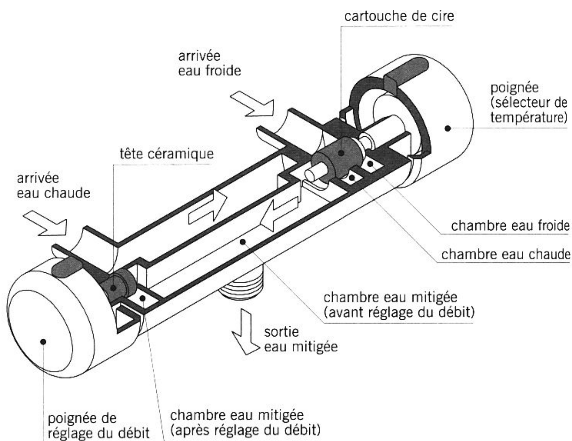
fig. 14.42 mitigeur thermostatique schéma de fonctionnement
