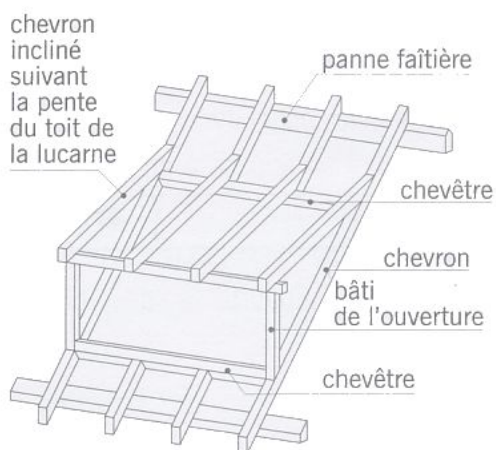
fig. 5.27 lucarne rampante
