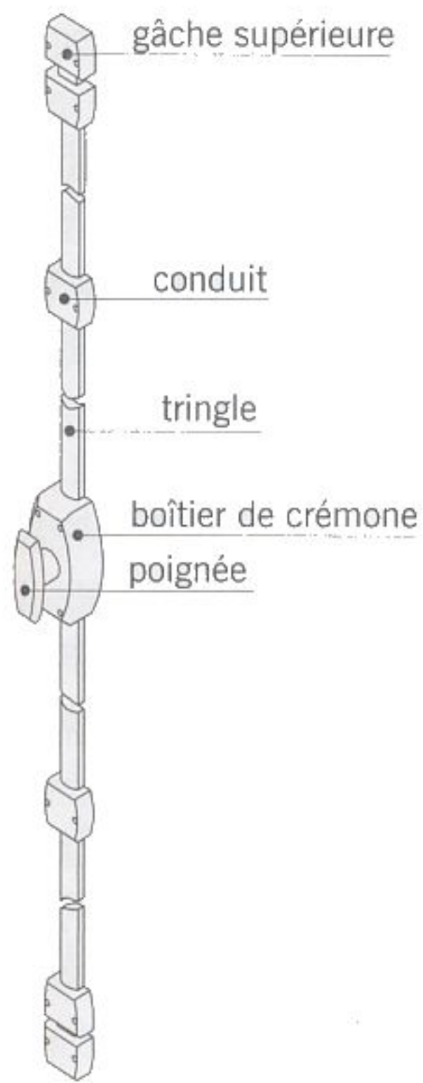
fig. 11.37 crémonne en applique pour menuiseries en bois
