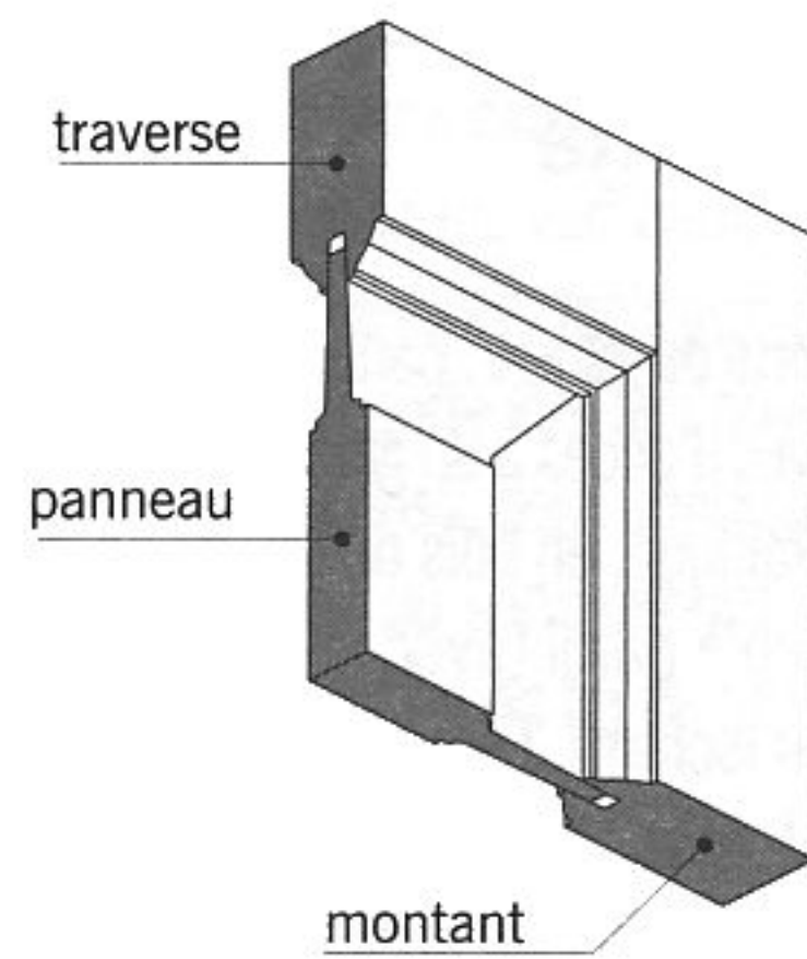
fig. 11.47 détail d'un angle de porte menuisée
