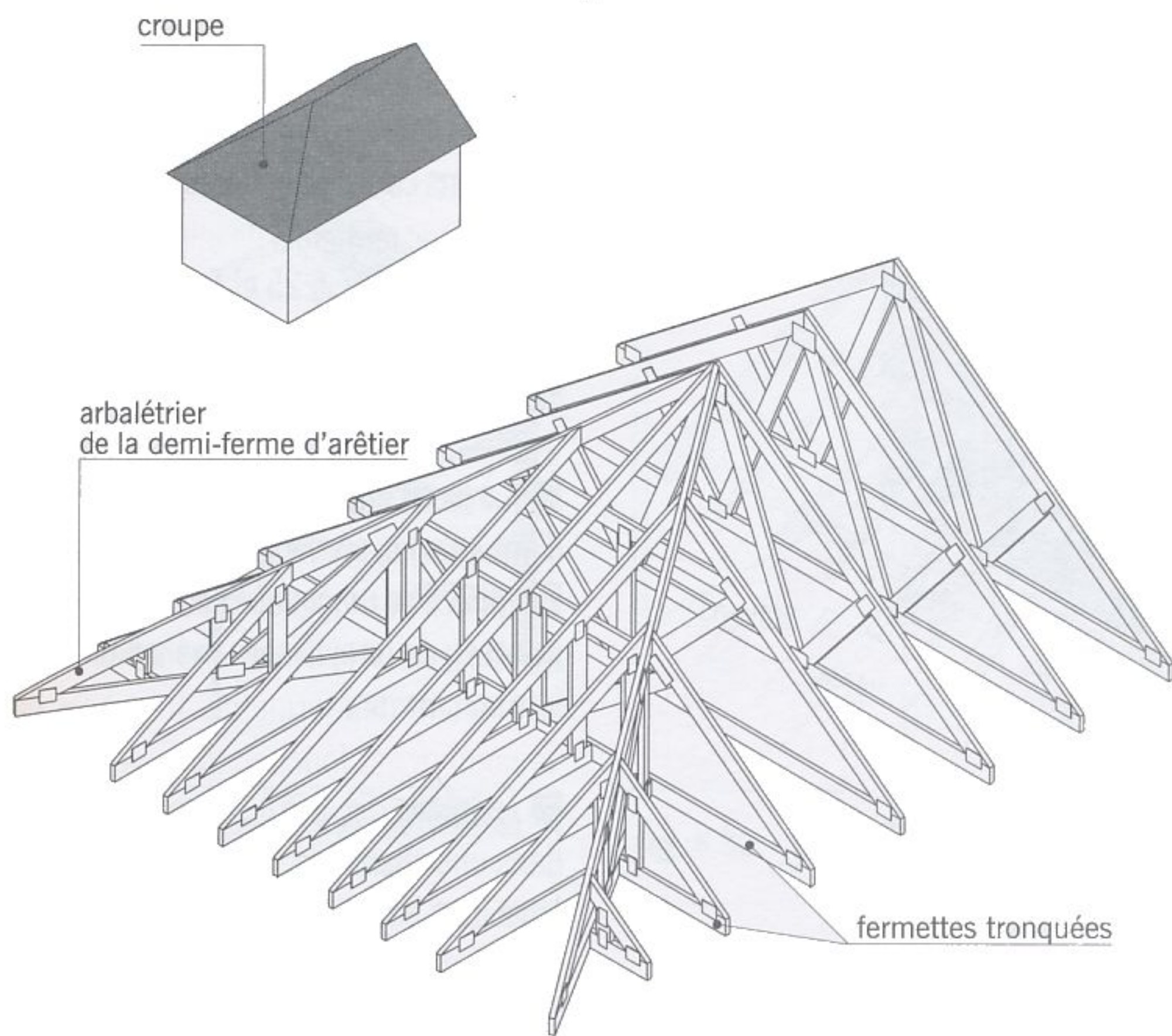
fig. 5.22 vue d'ensemble de la croupe
