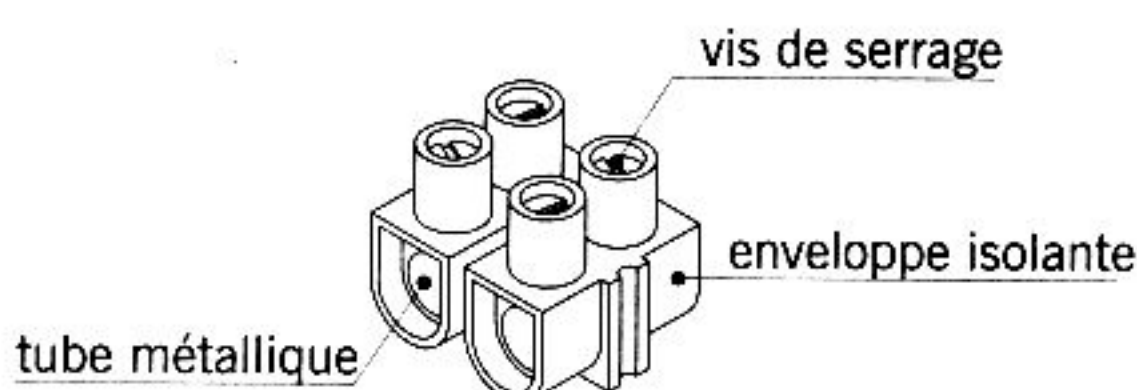
fig. 16.27 domino
