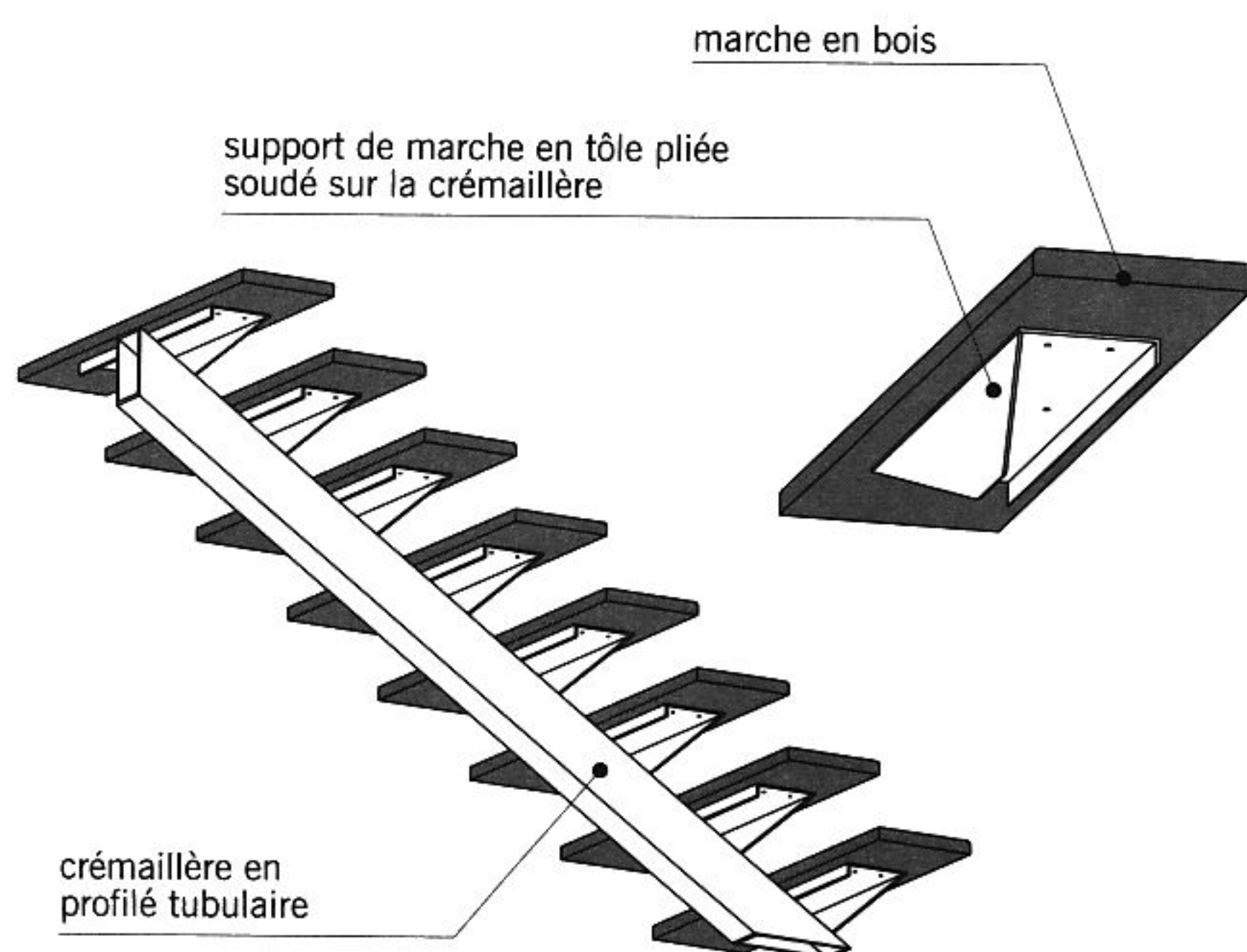
fig. 13.31 escalier à crémaillère métallique centrale
