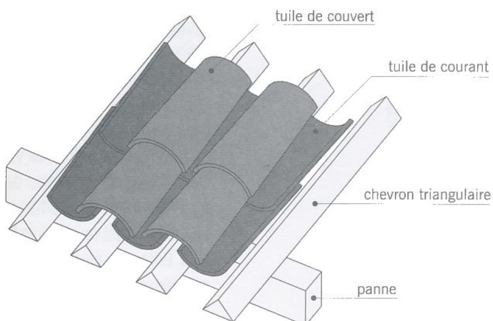
tuiles canal posées sur chevrons triangulaires
