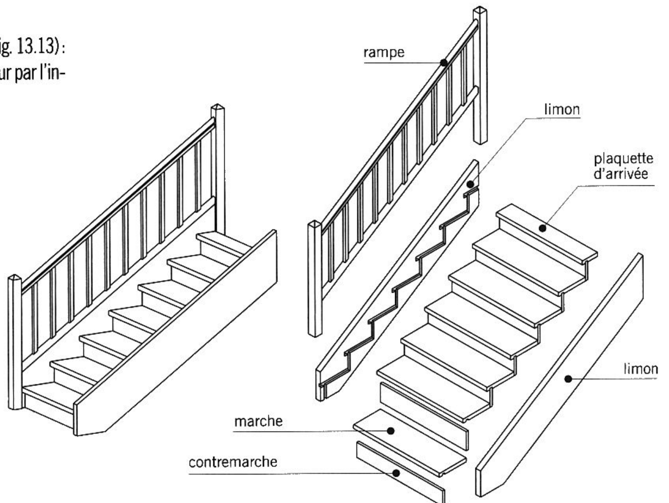
escalier à la française
