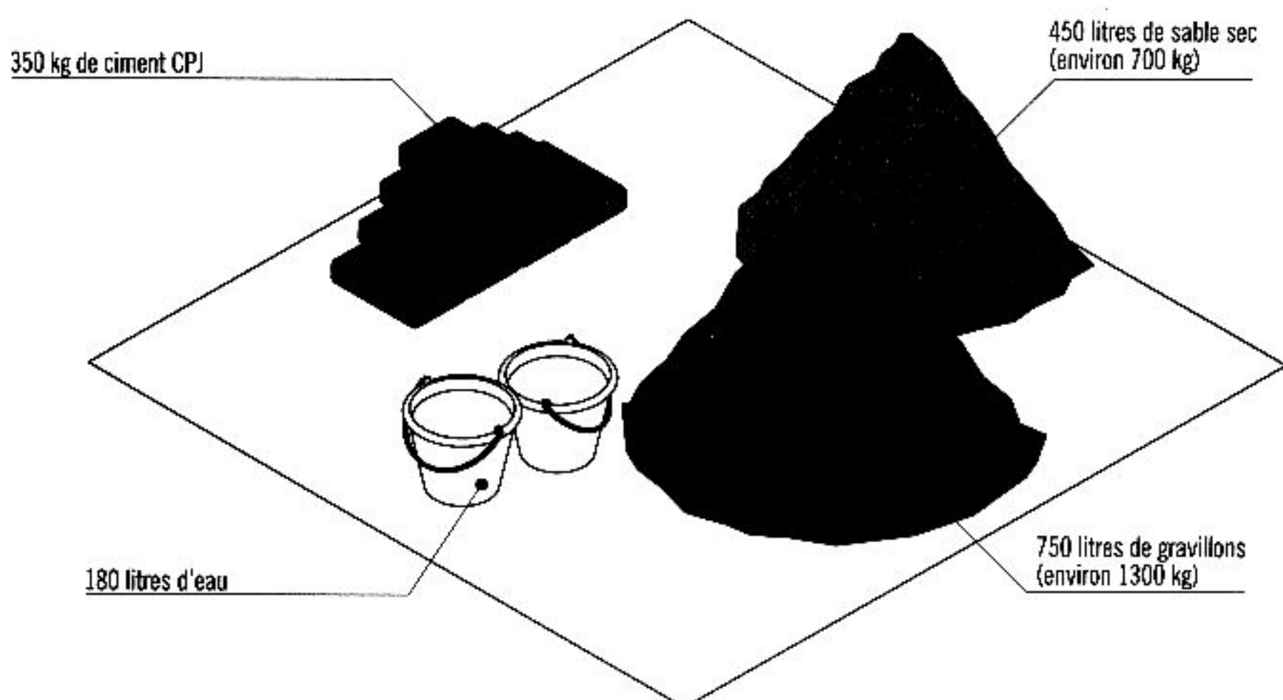
fig. 1.1 constituants d'1 \text{m}^3 de béton dosé à 350 kg de ciment (valeurs moyennes)
