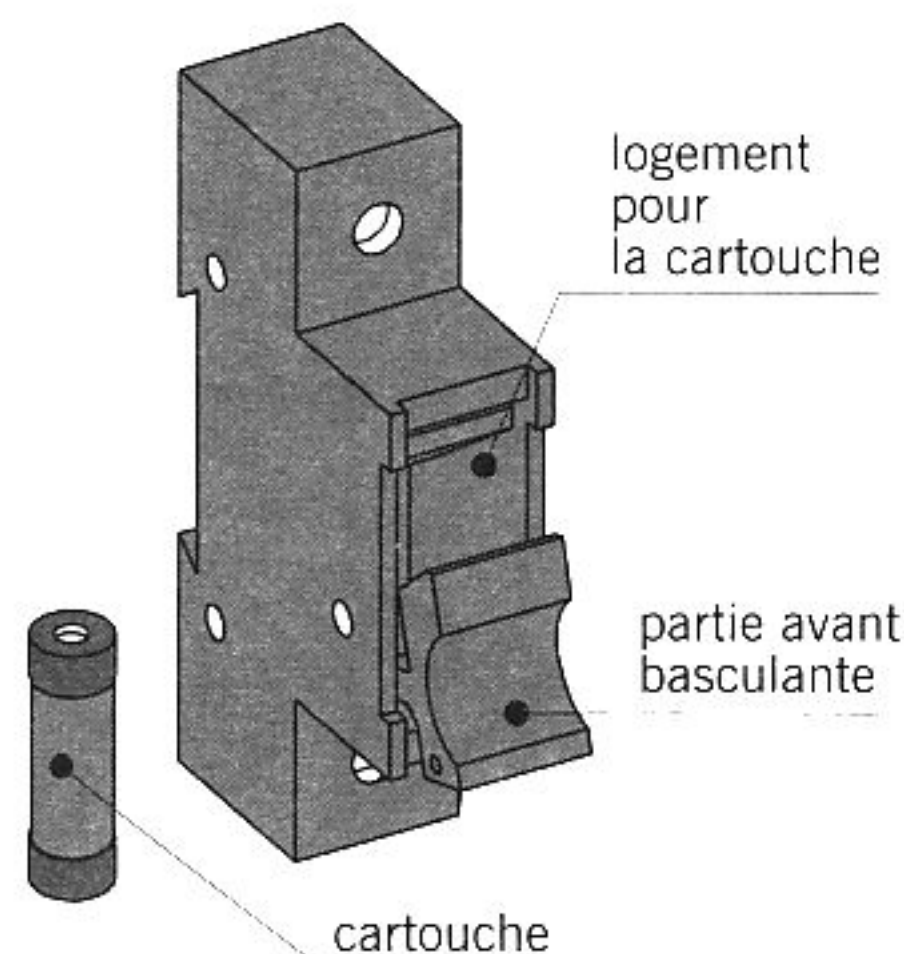
fig. 16.9 coupe-circuit à cartouche
