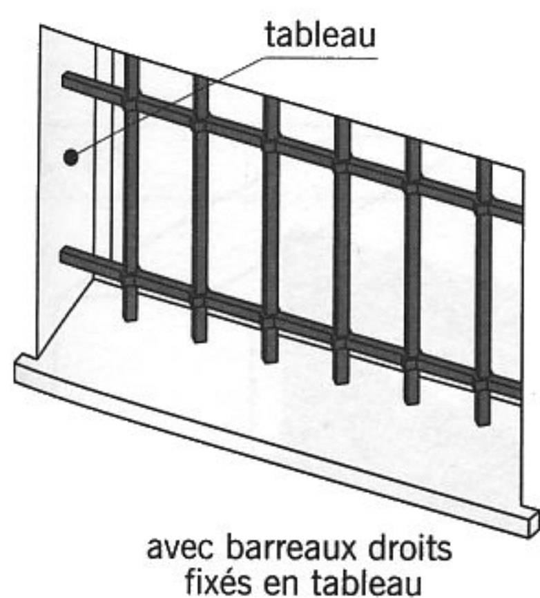
fig. 11.72 exemples de grilles de défense
