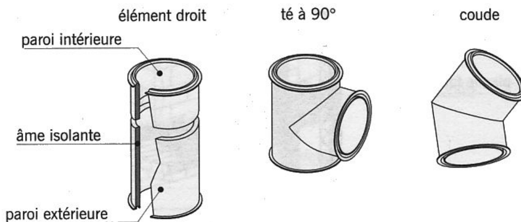
fig. 17.41 conduits métalliques à double paroi
