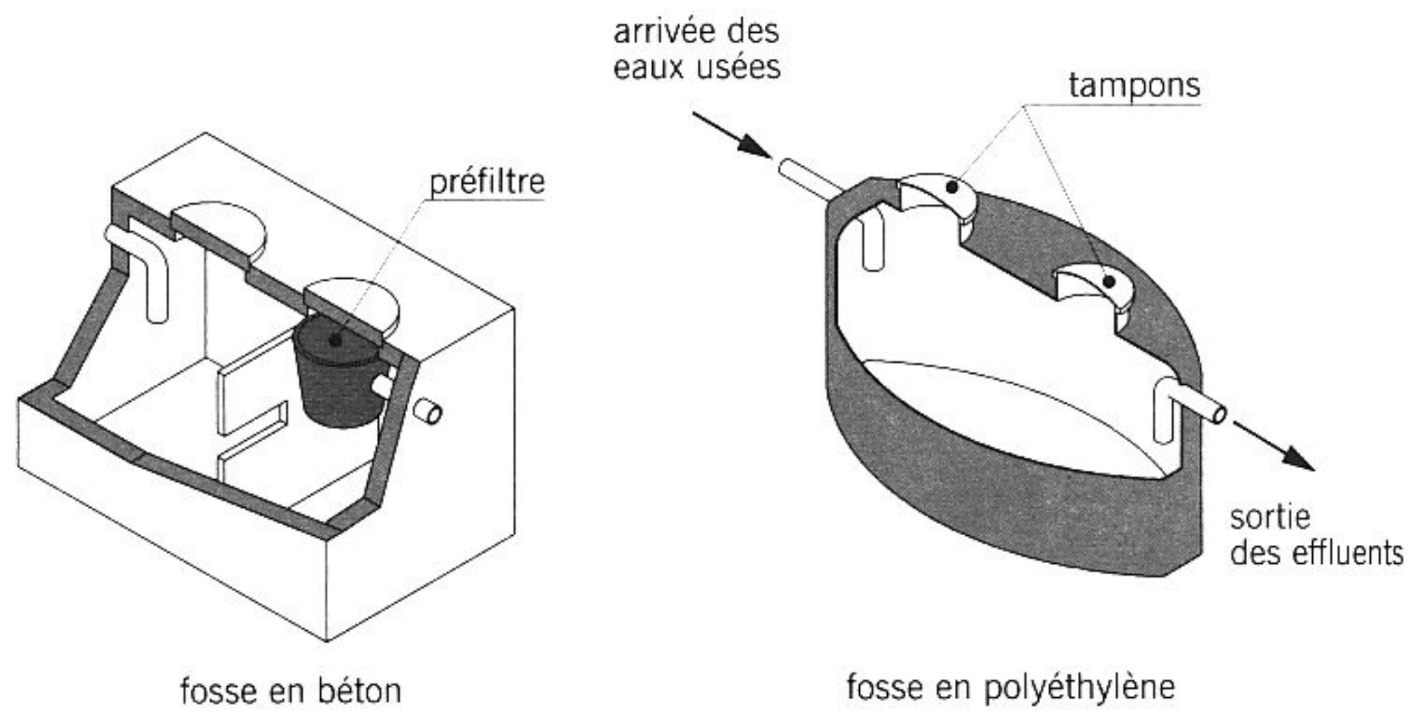
fig. 15.10 fosses toutes eaux
