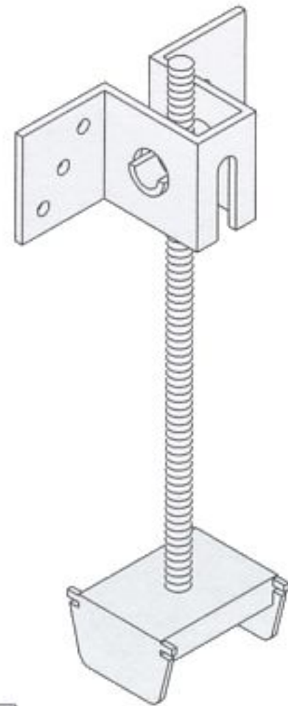
suspente articulée
