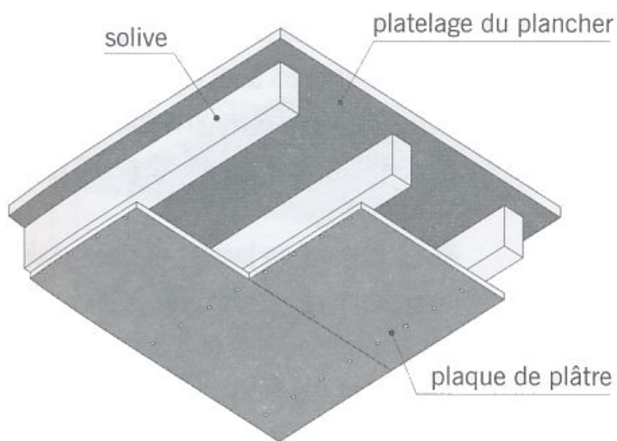
fig. 9.1 plafond fixe sous plancher en bois
