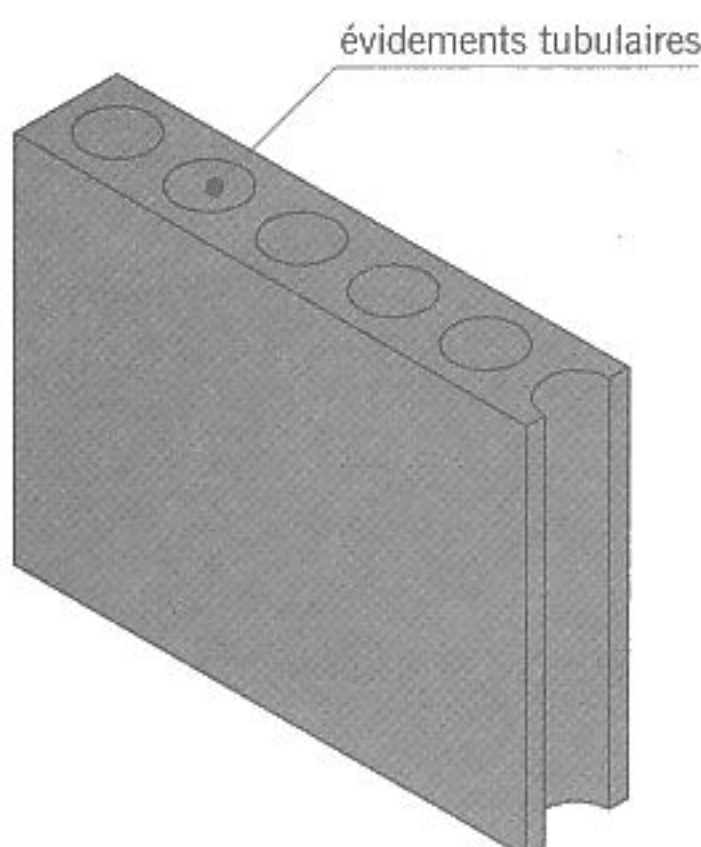
fig. 1.11 élément de cloison en panneau de particules
