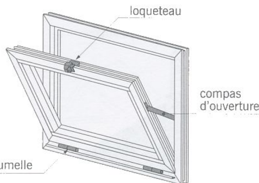
fig. 11.40 accessoires d'une fenêtre à soufflet en aluminium
