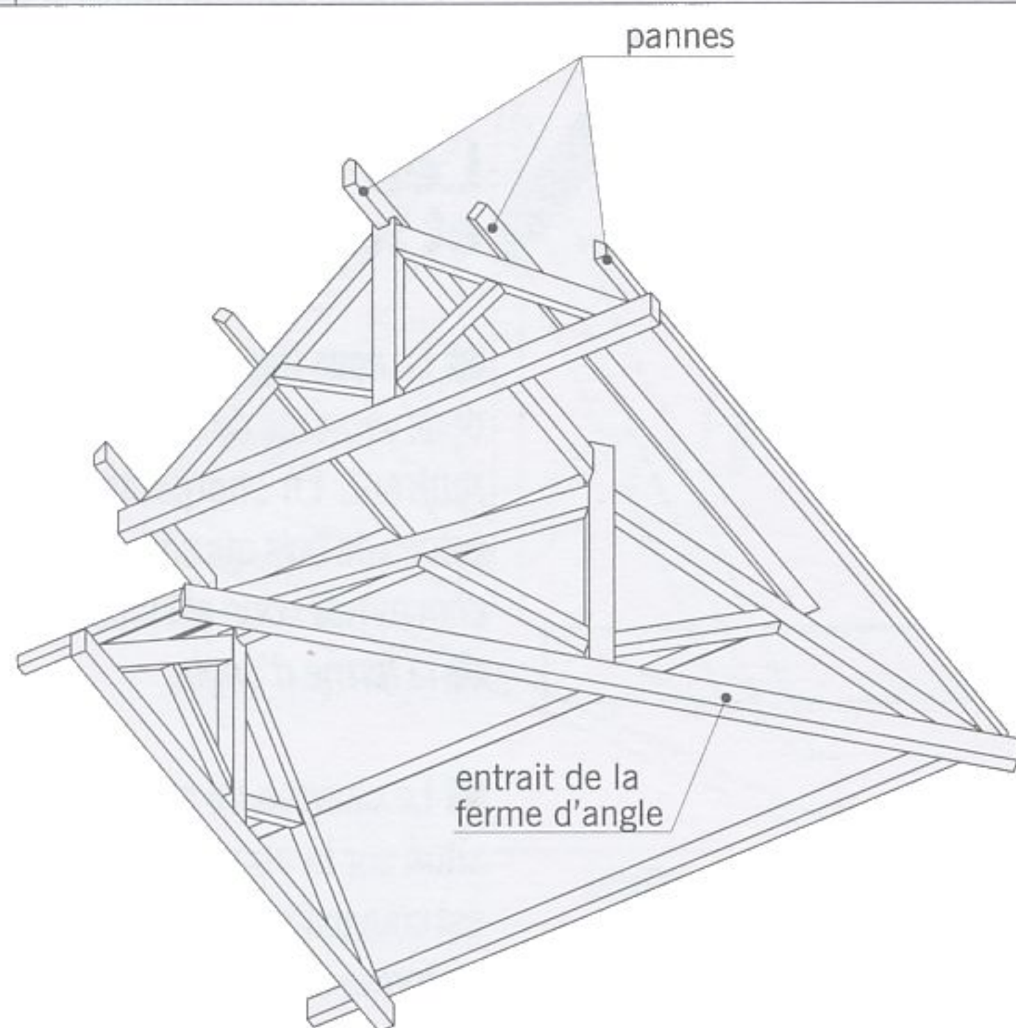
intersection de deux charpentes observée par dessous (chevrons non représentés)
