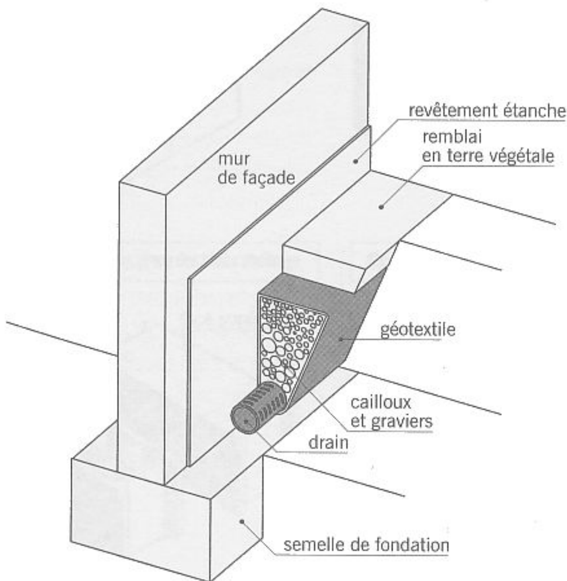
fig. 2.15 éléments constitutifs du drainage
