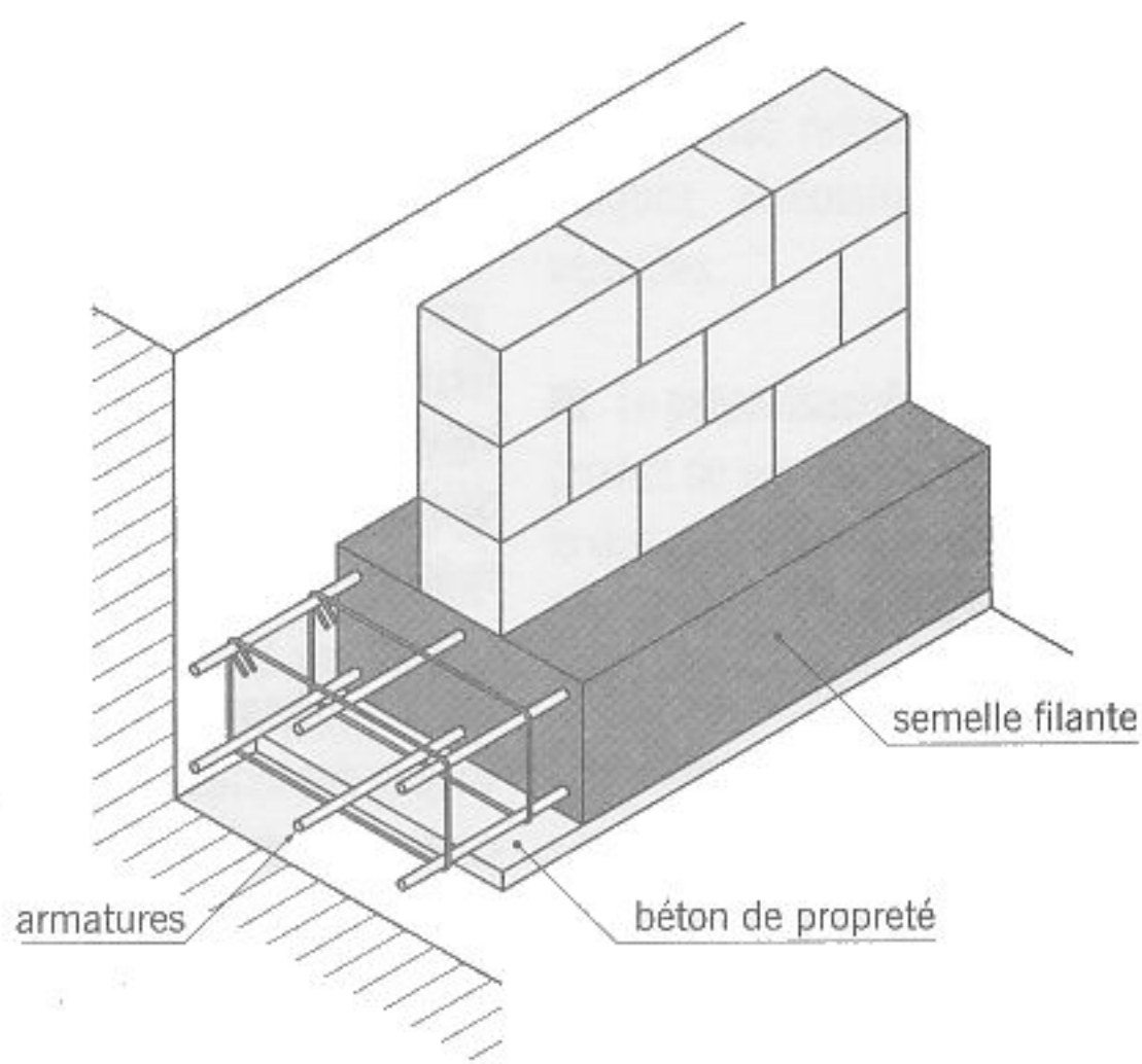
semelle filante armée
