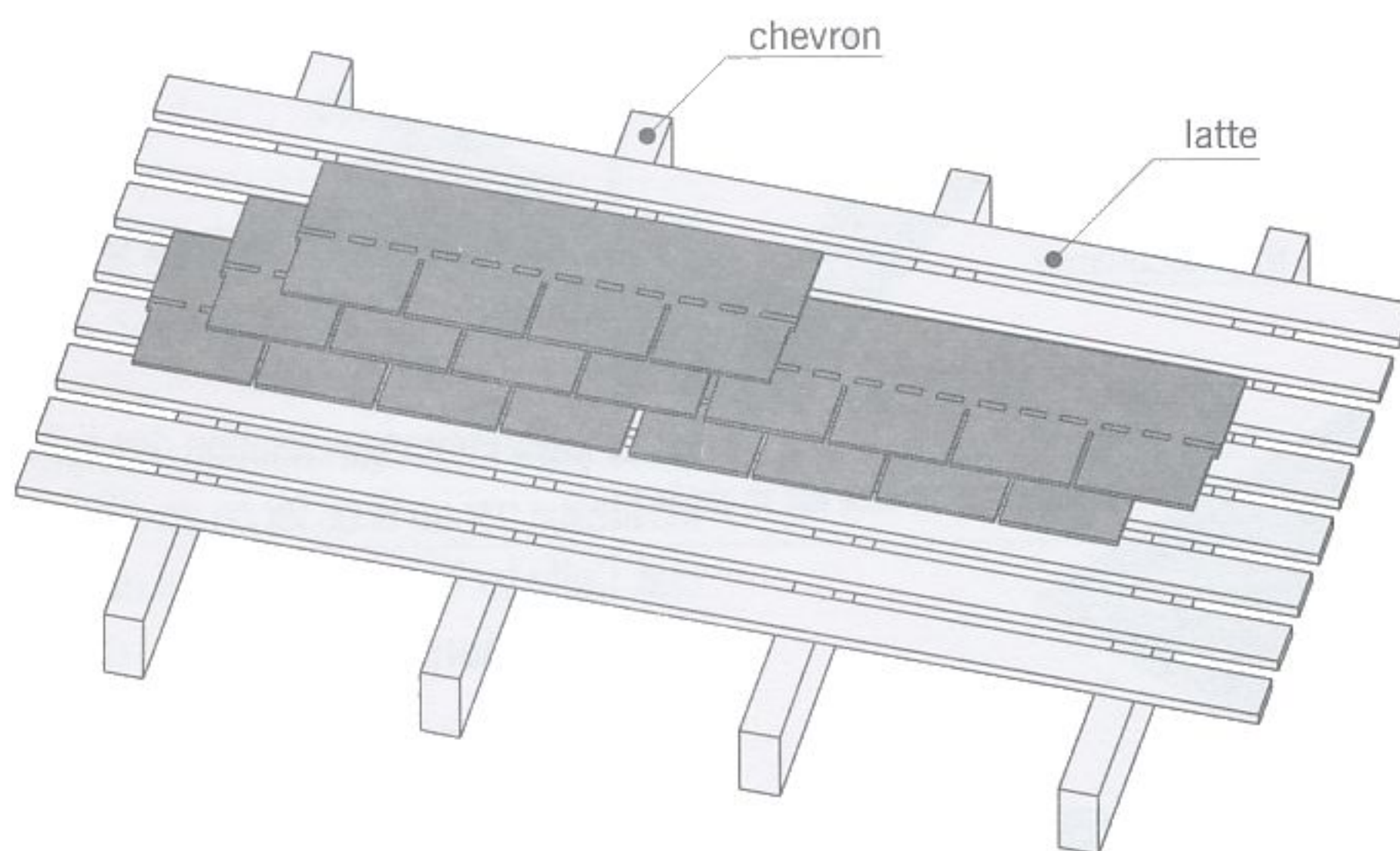
fig. 7.35 pose à la française
