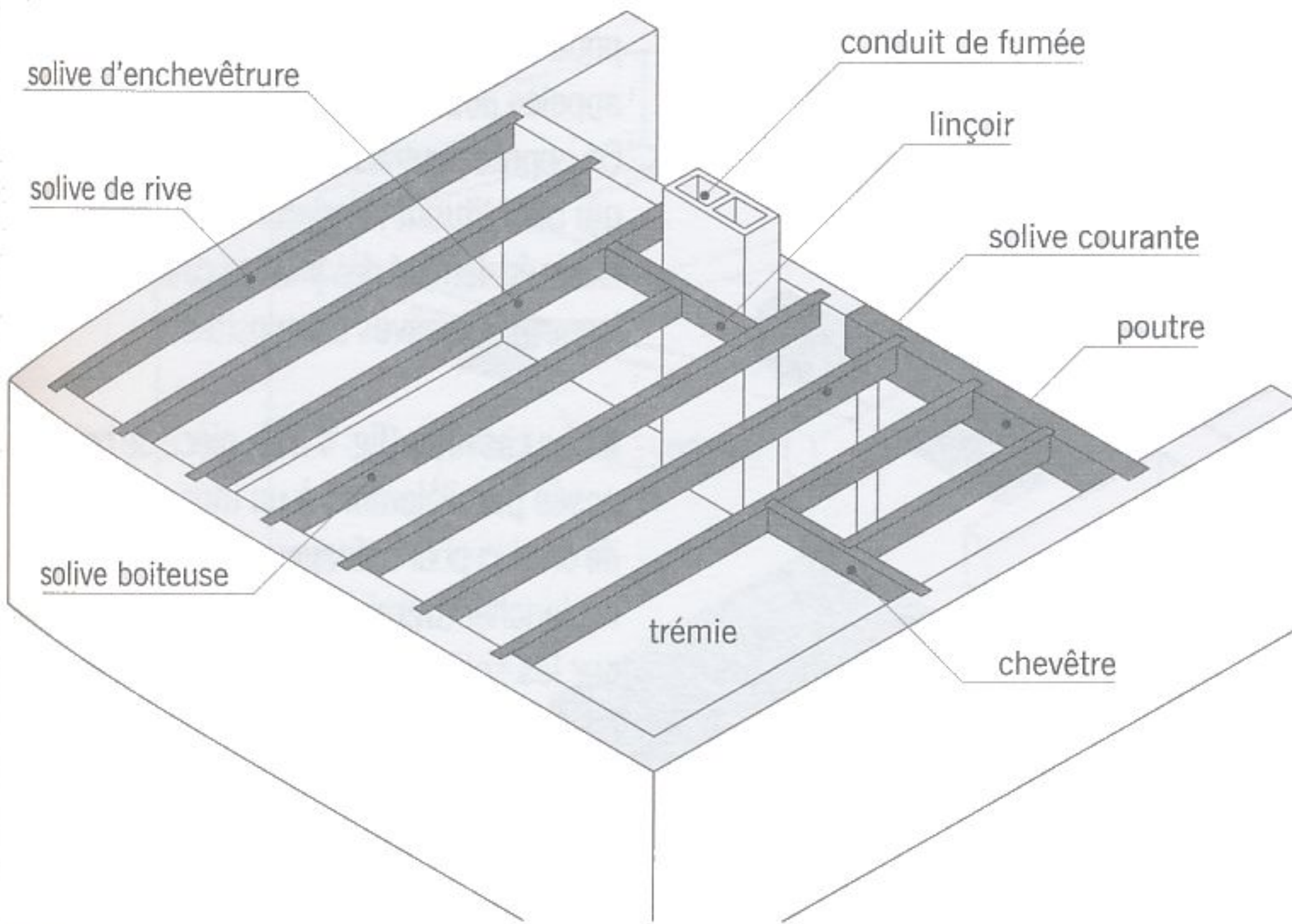
fig. 4.21 éléments porteurs d'un plancher en bois
