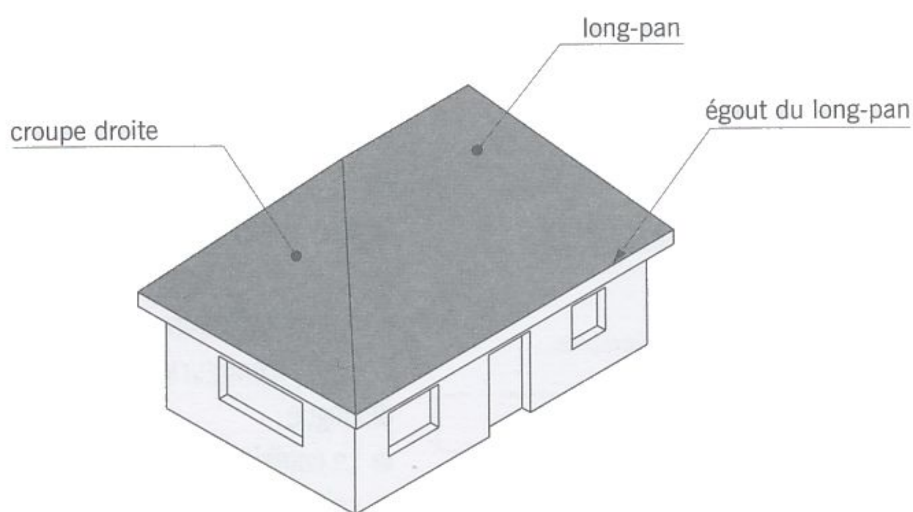
croupe droite
