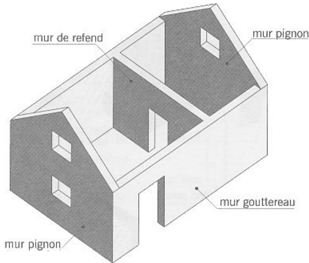
différents murs (1)
