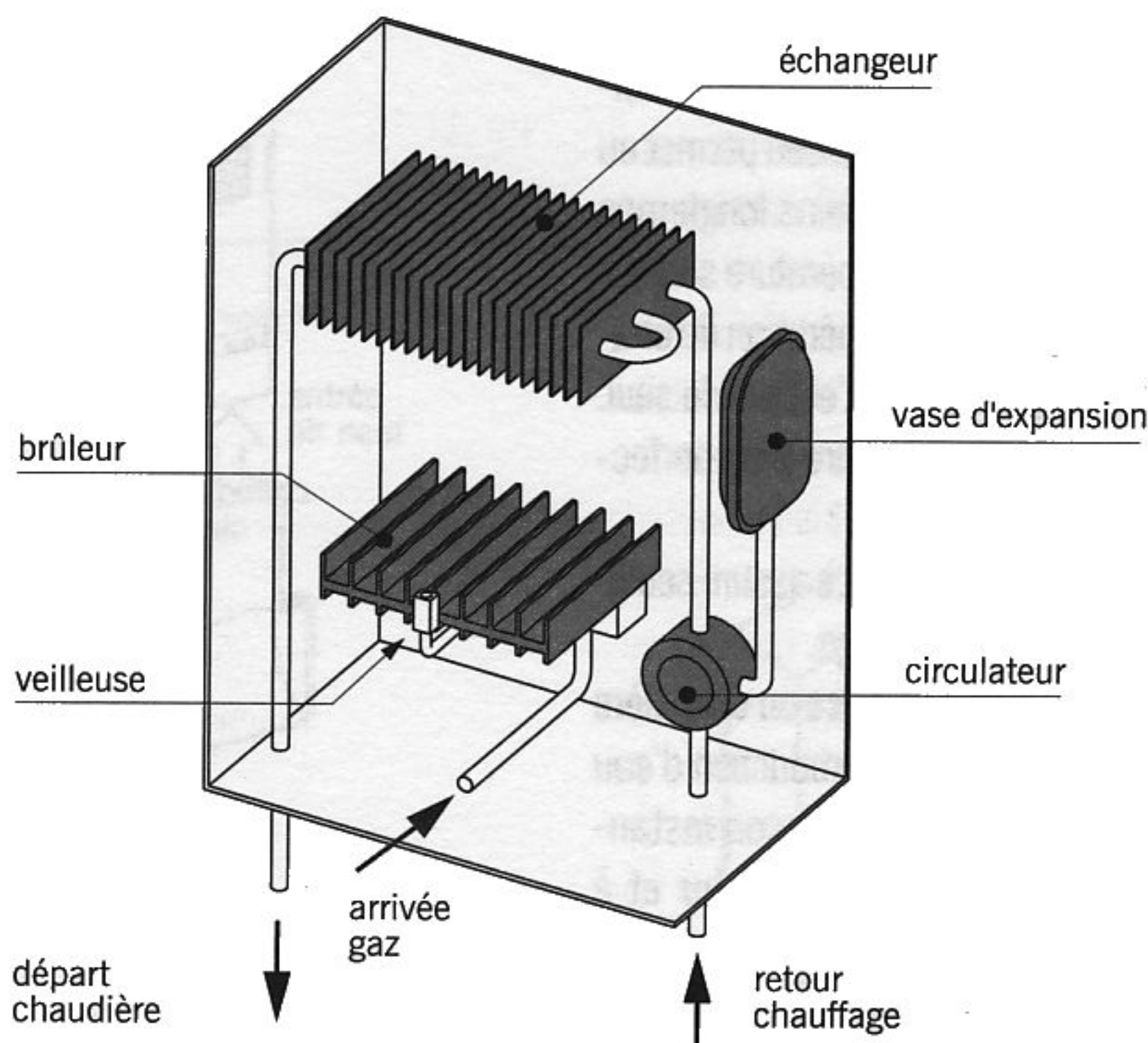
fig. 17.19 composants principaux d'une chaudière à gaz
