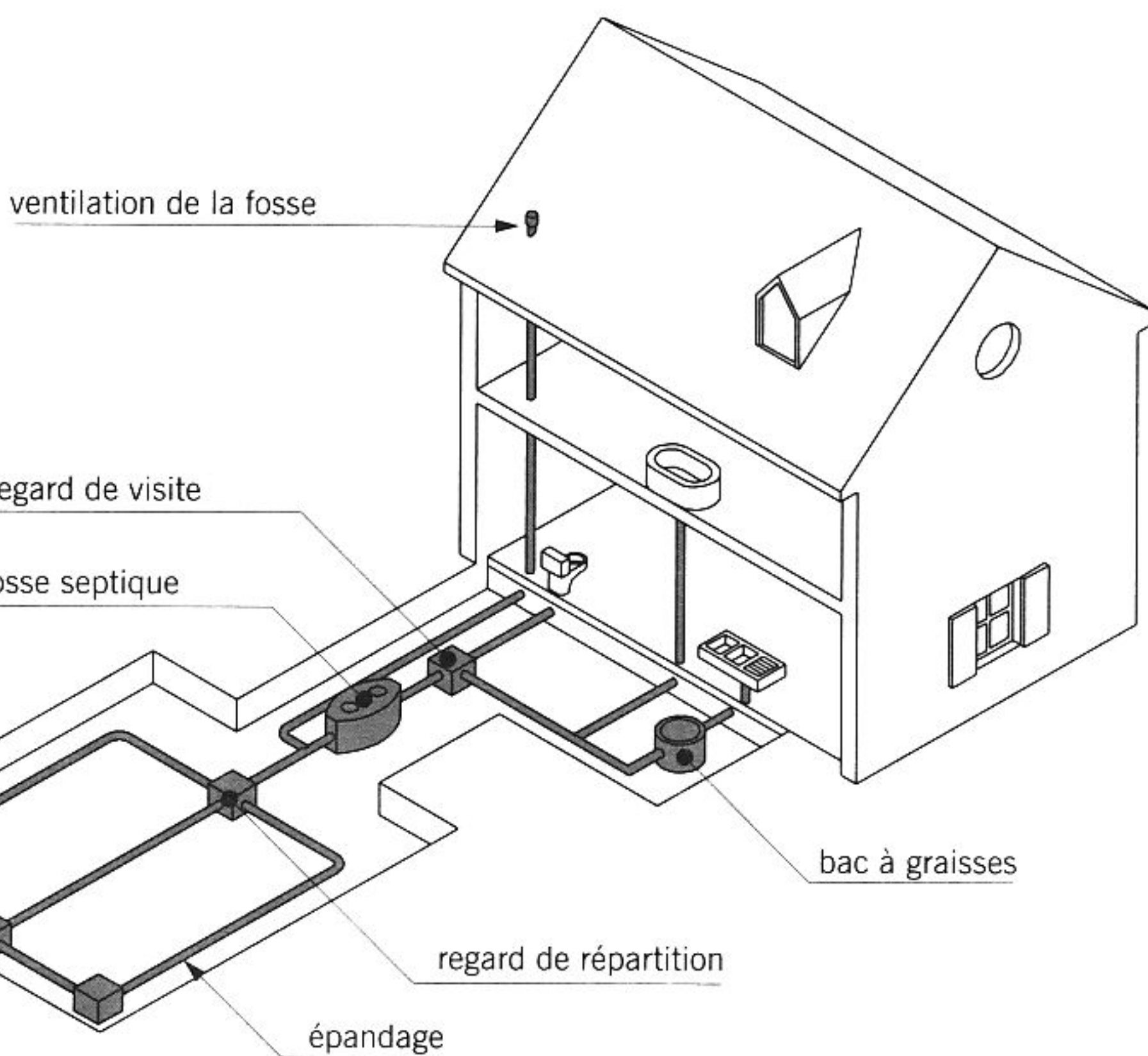
fig. 15.9 exemple d'une filière d'assainissement
