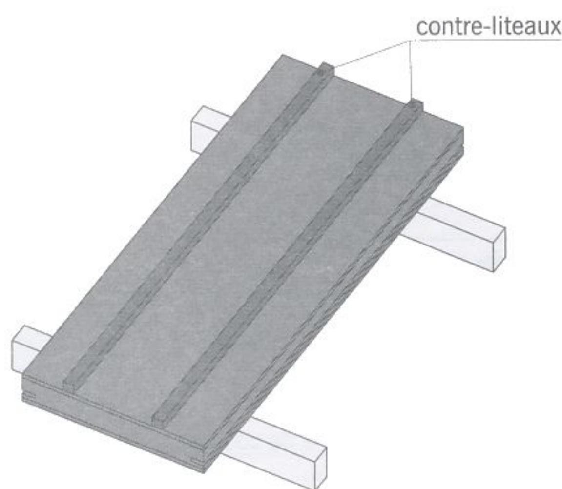
fig. 7.5 panneau sandwich avec contre-liteaux
