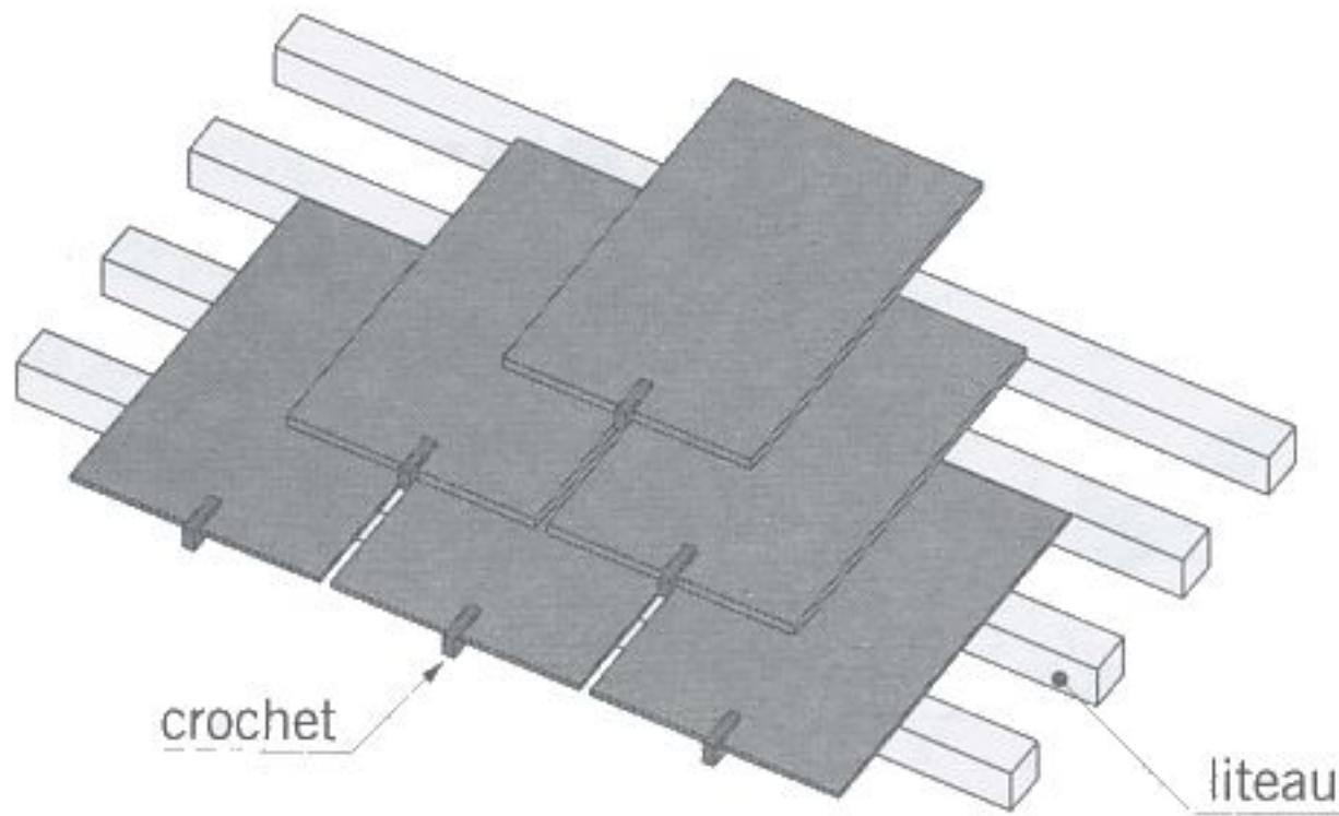
fig. 7.39 pose à pureau entier
