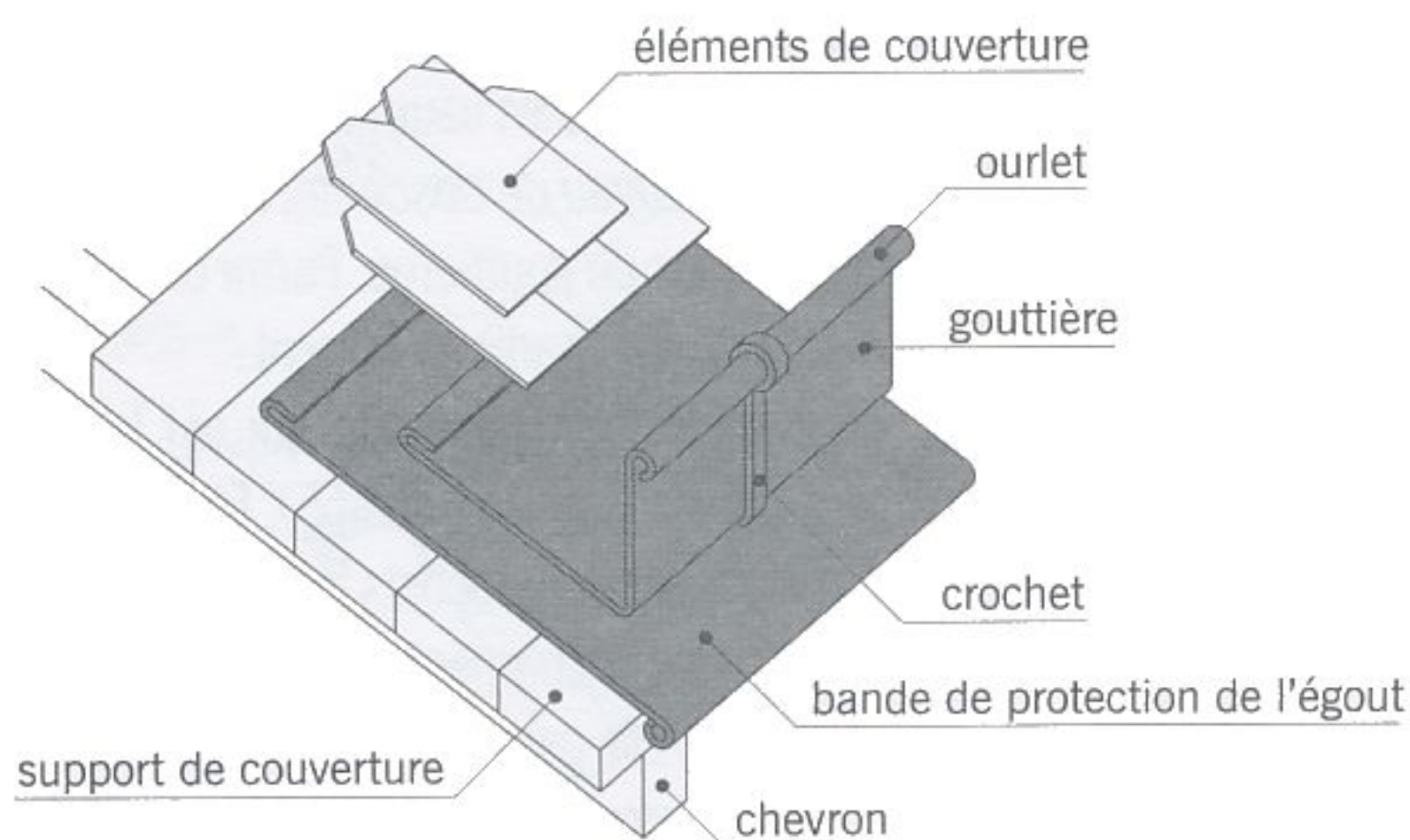
fig. 7.56 gouttière de Laval
