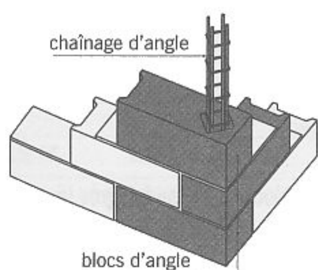
fig. 3.3 mise en place des blocs d'angle
