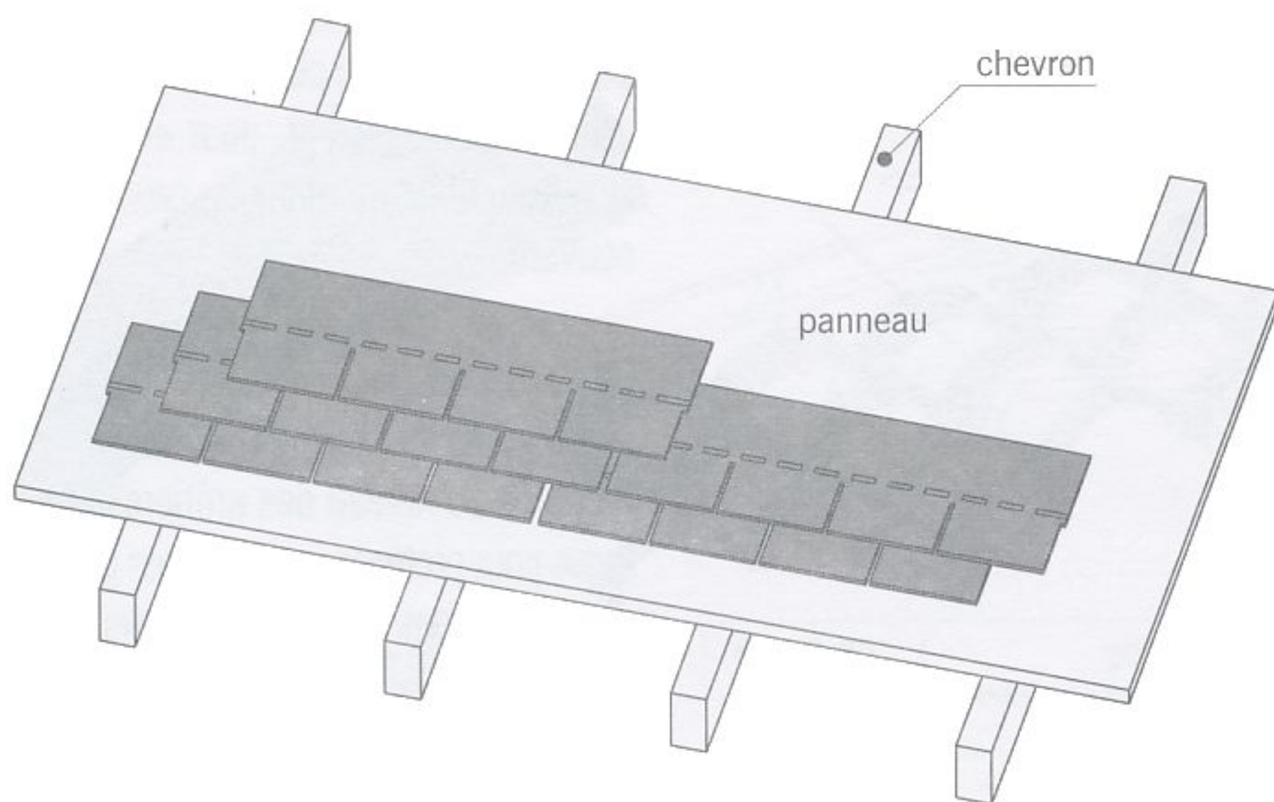
fig. 7.34 pose à l'américaine
