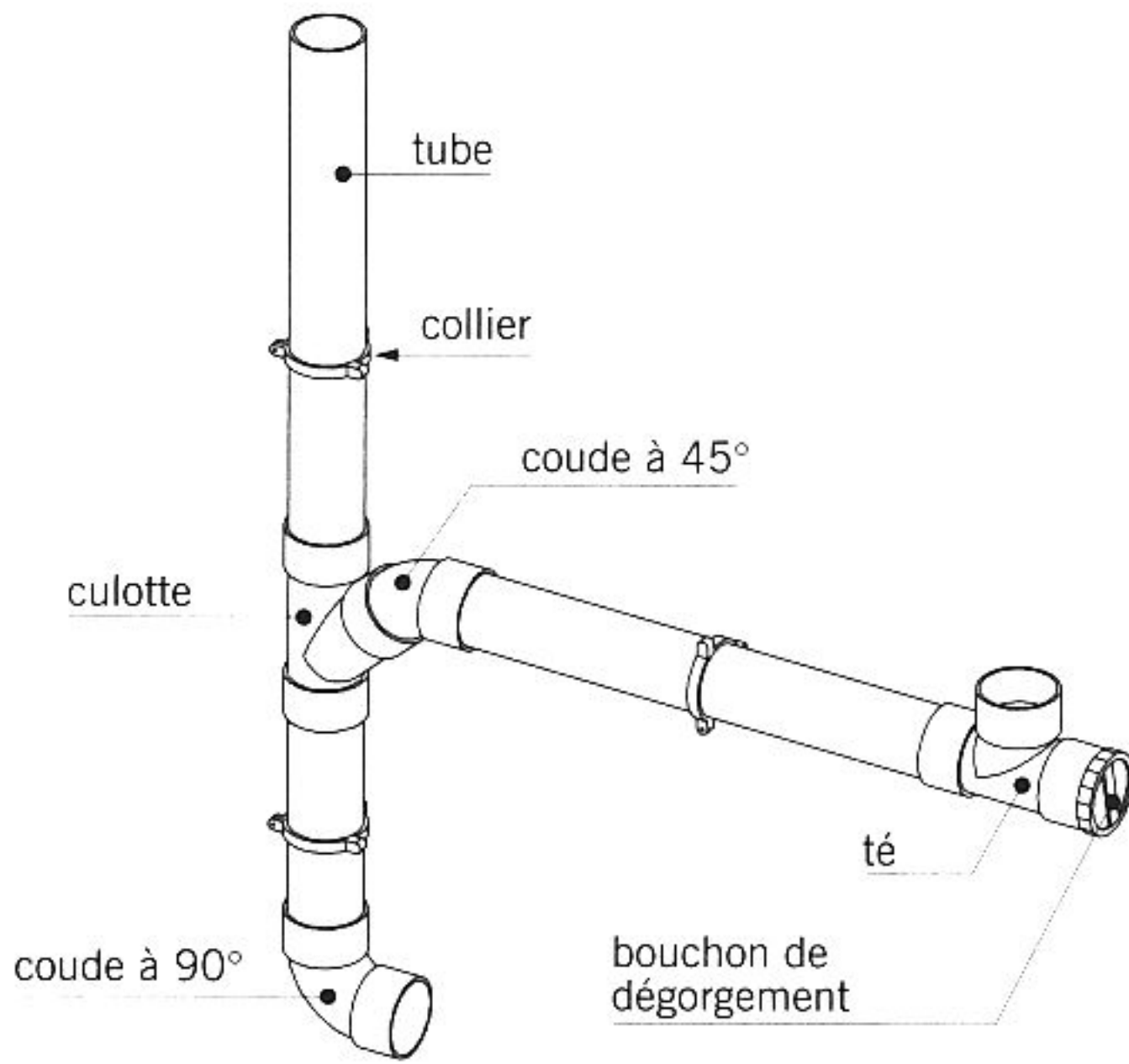
fig. 15.1 portion d'un réseau d'évacuation
