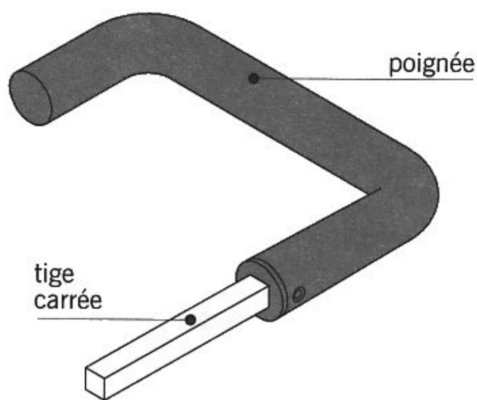
fig. 12.24 béquille
