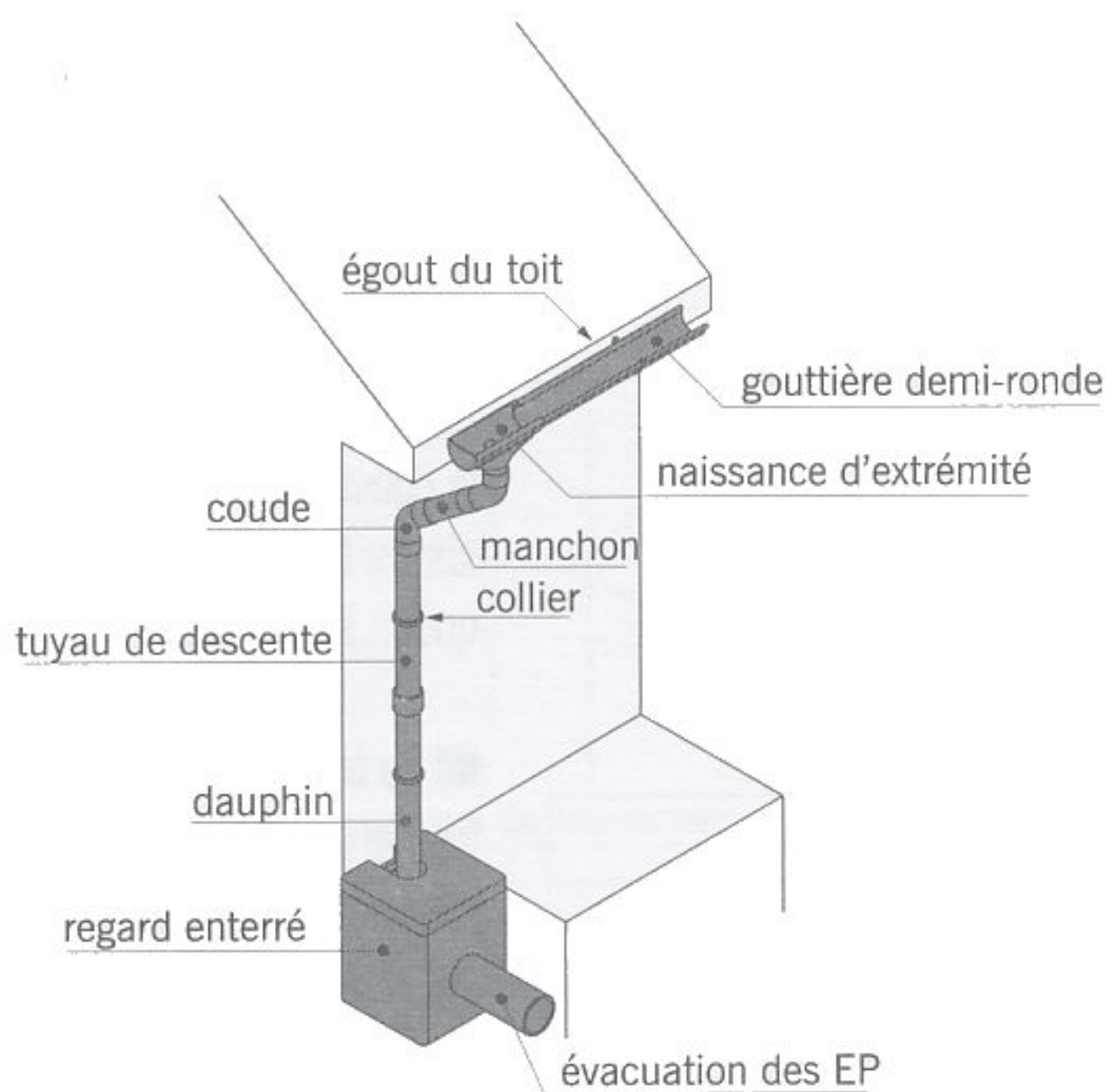
fig. 7.53 réseau d'évacuation des EP
