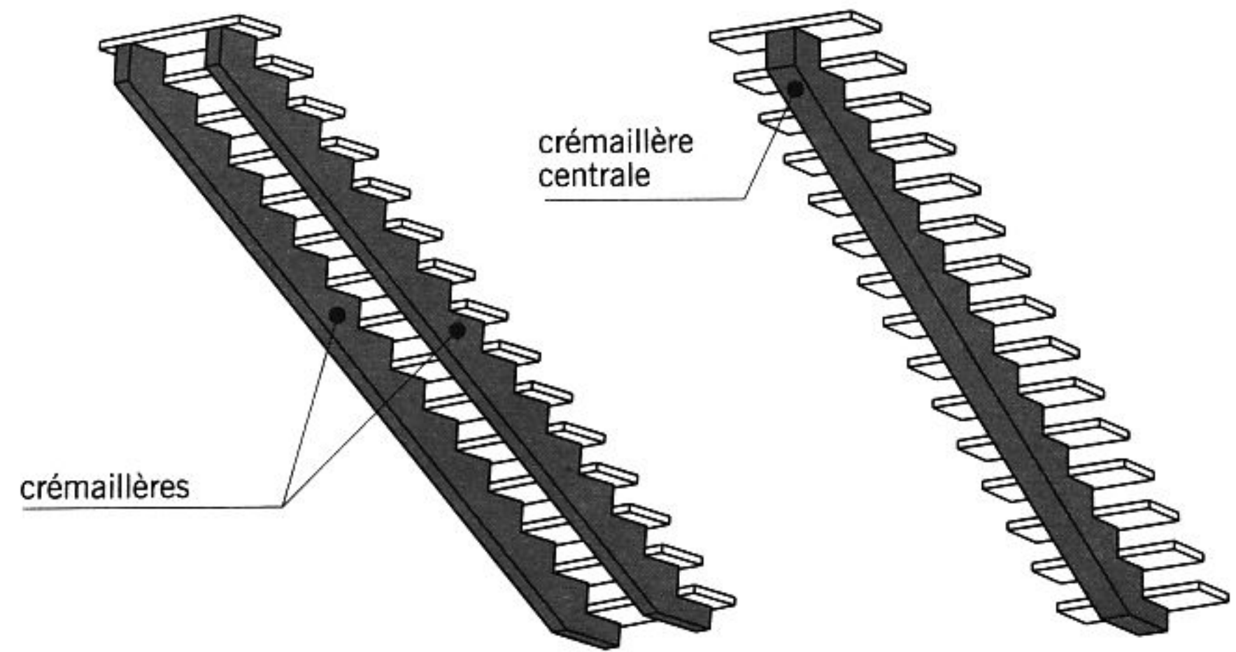
escaliers préfabriqués avec crémaillères en béton
