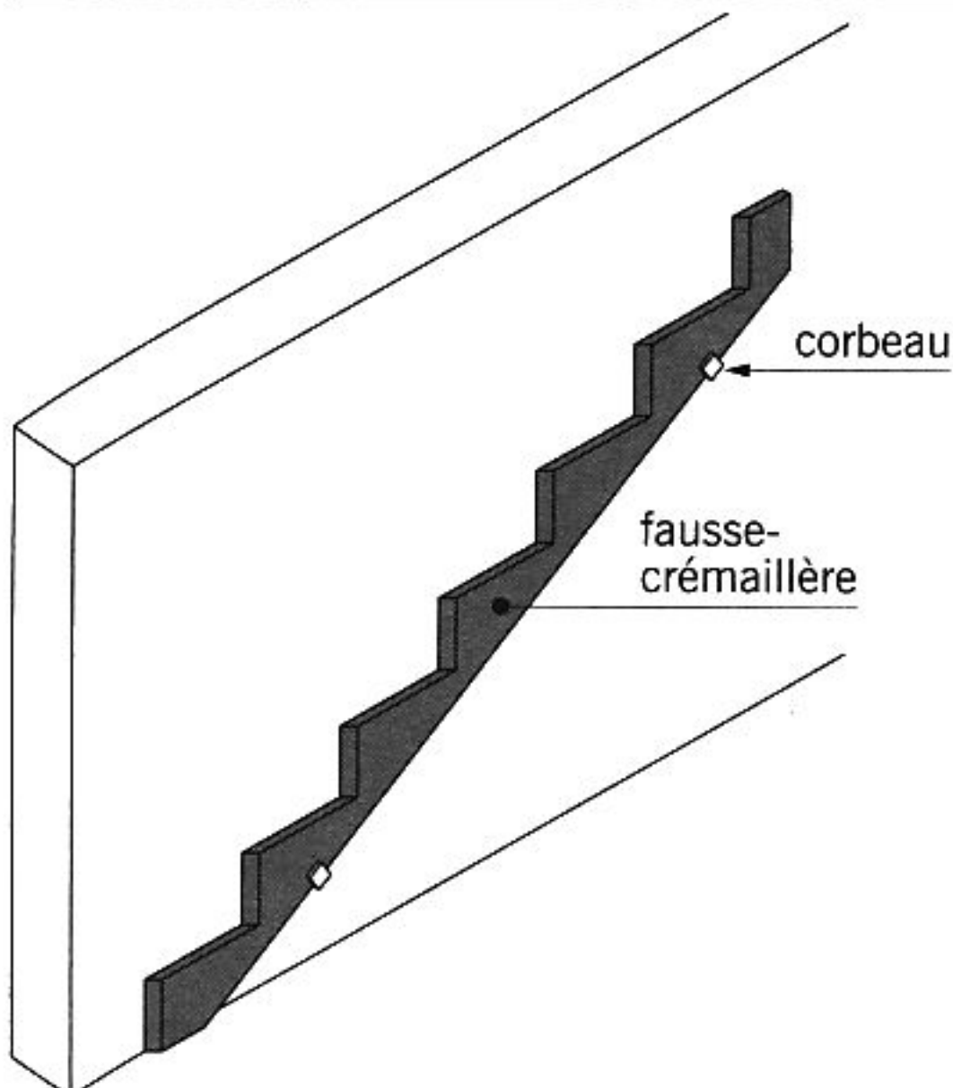
fig. 13.15 escaler à l'anglaise
