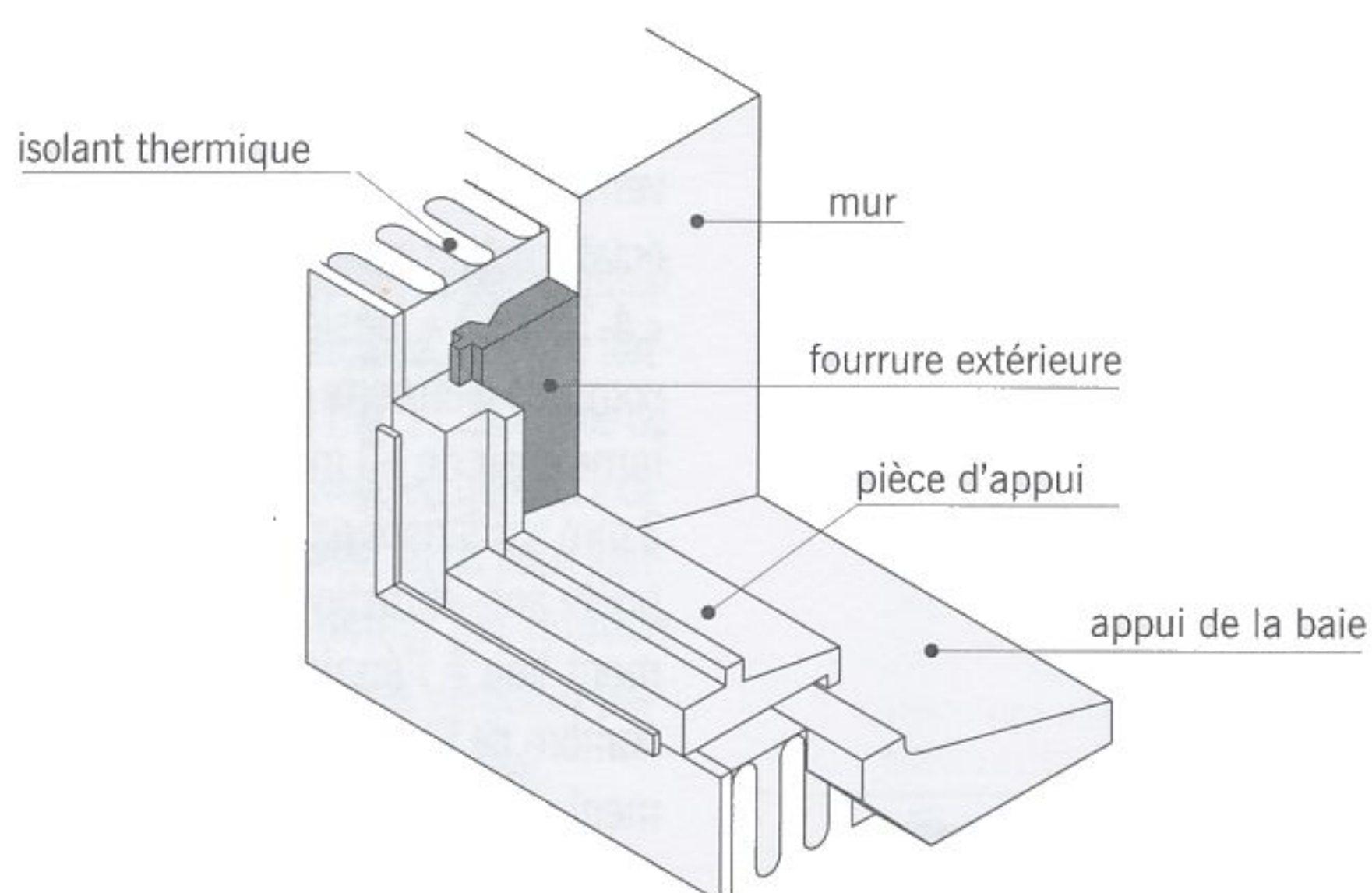
fig. 11.16 fourrure extérieure (cadre ouvrant non représenté)
