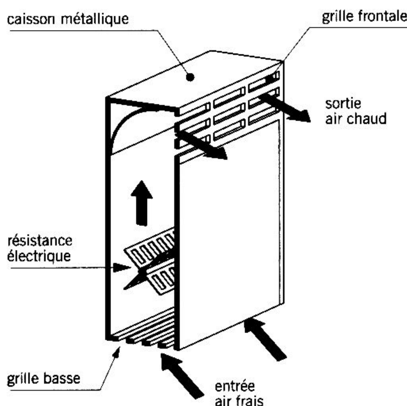
schéma de fonctionnement d'un convecteur
