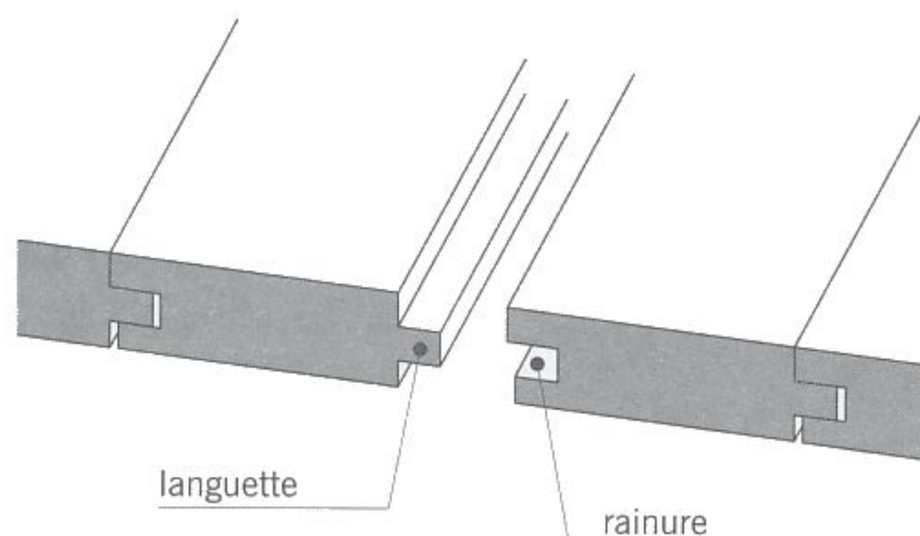
fig. 10.1 parquet à lames
