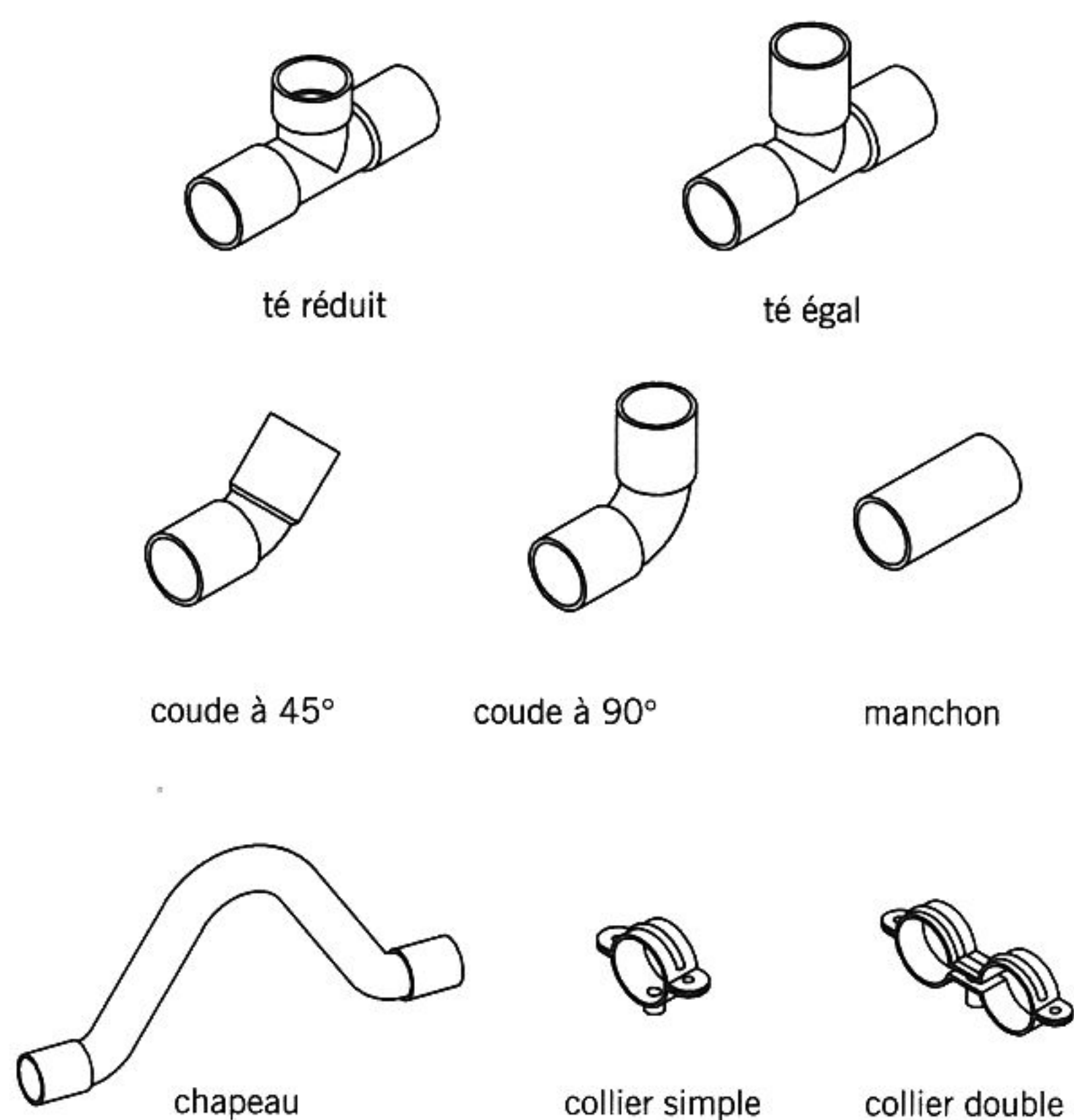
fig. 14.2 raccords à souder et accessoires en cuivre
