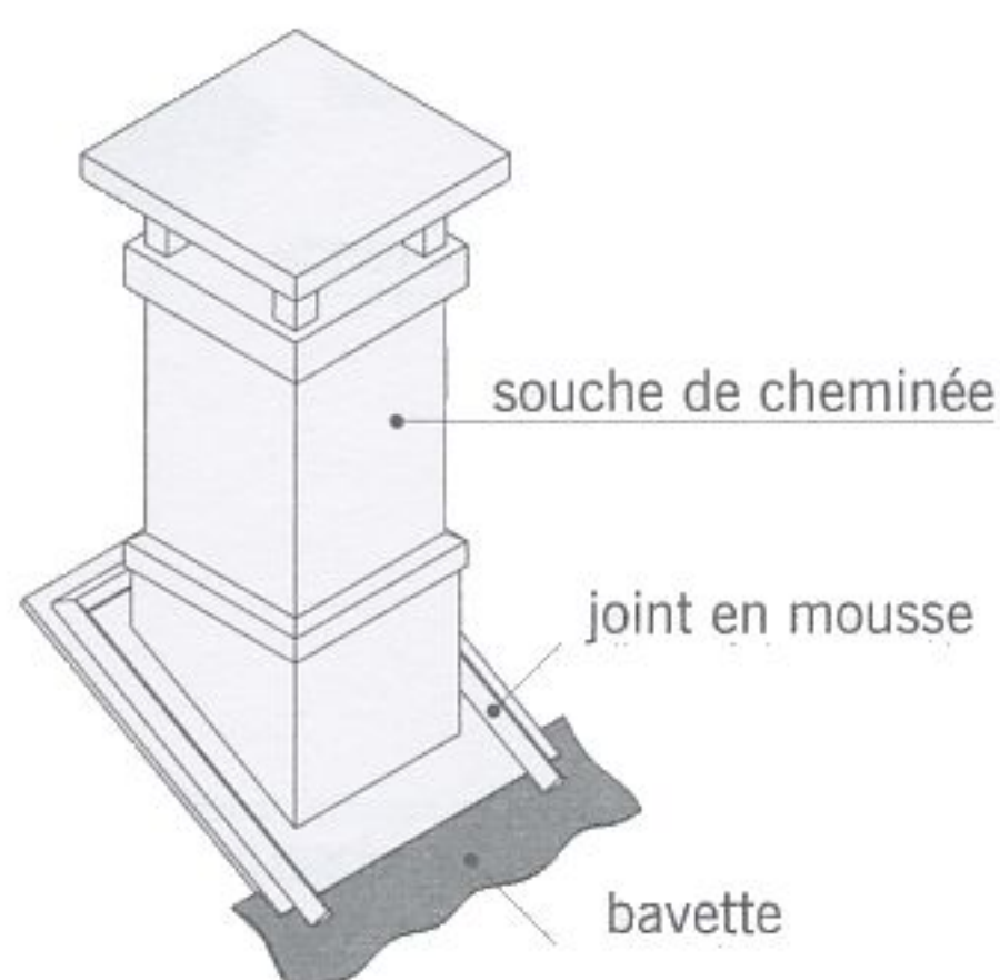
fig. 7.51 Bavette de souche de cheminée métallique
