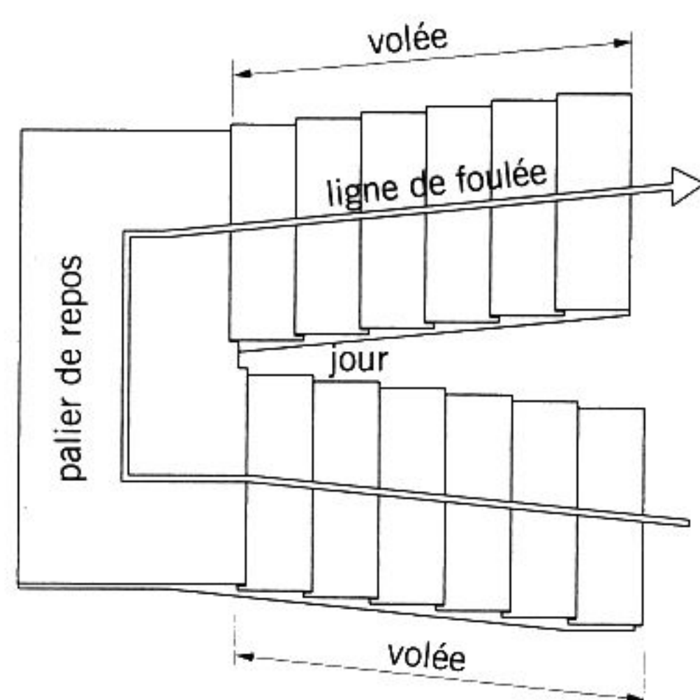
fig. 13.2 vue de dessus de deux volées d'escalier
