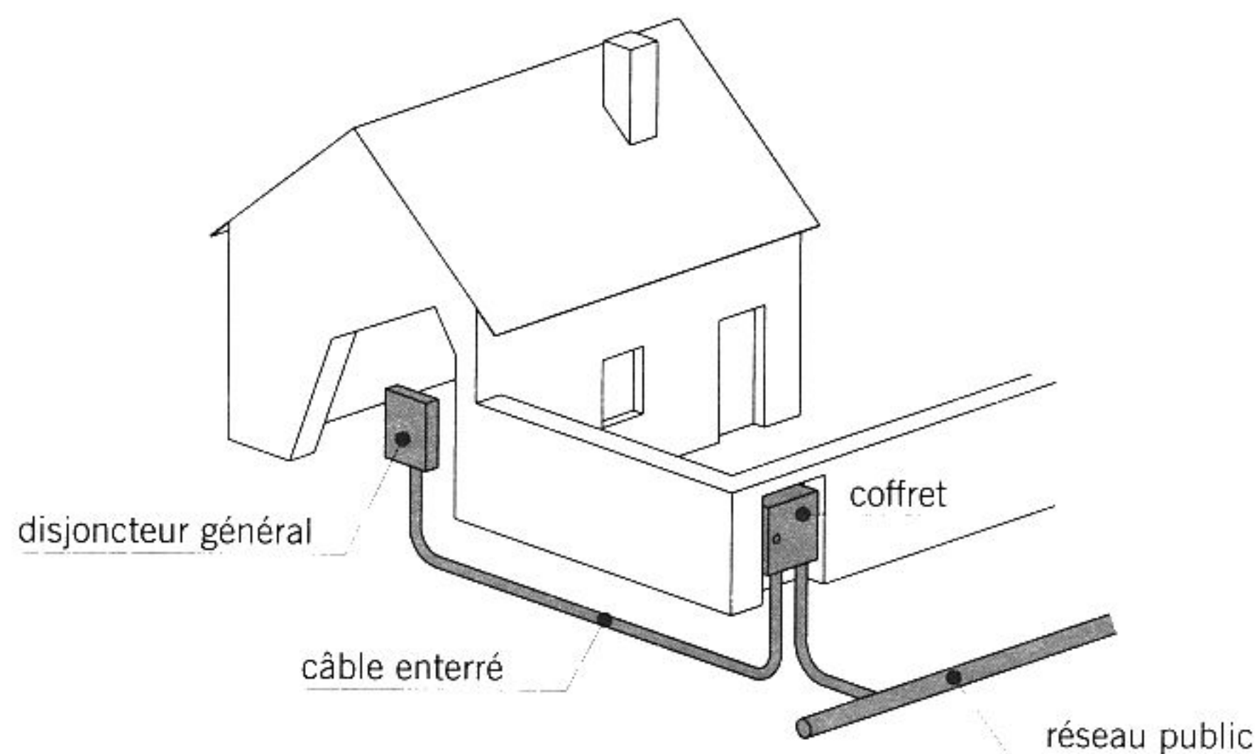
fig. 16.1 branchement souterrain
