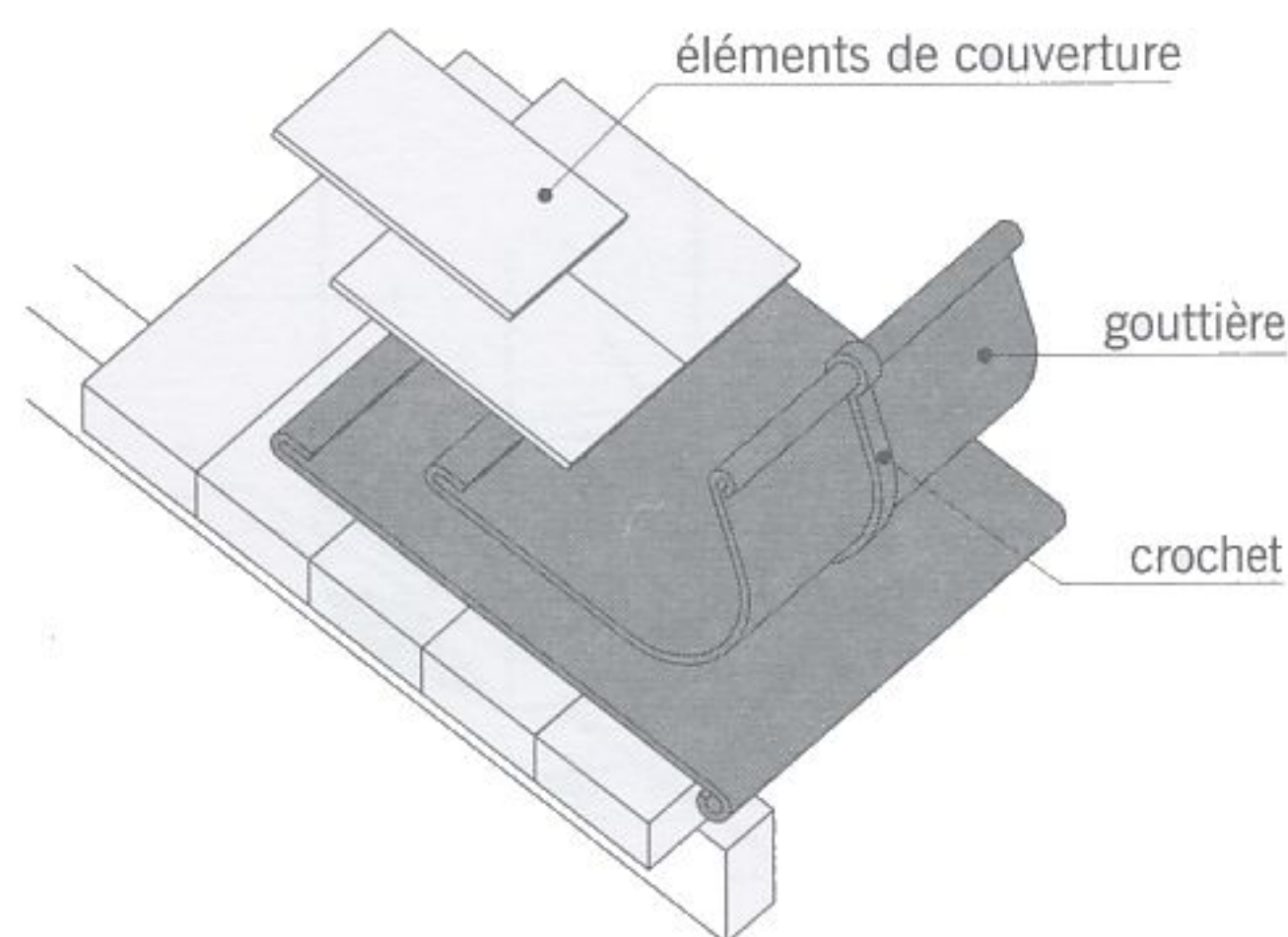
fig. 7.57 gouttière havraise
