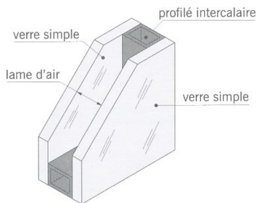
fig. 11.20 double vitrage
