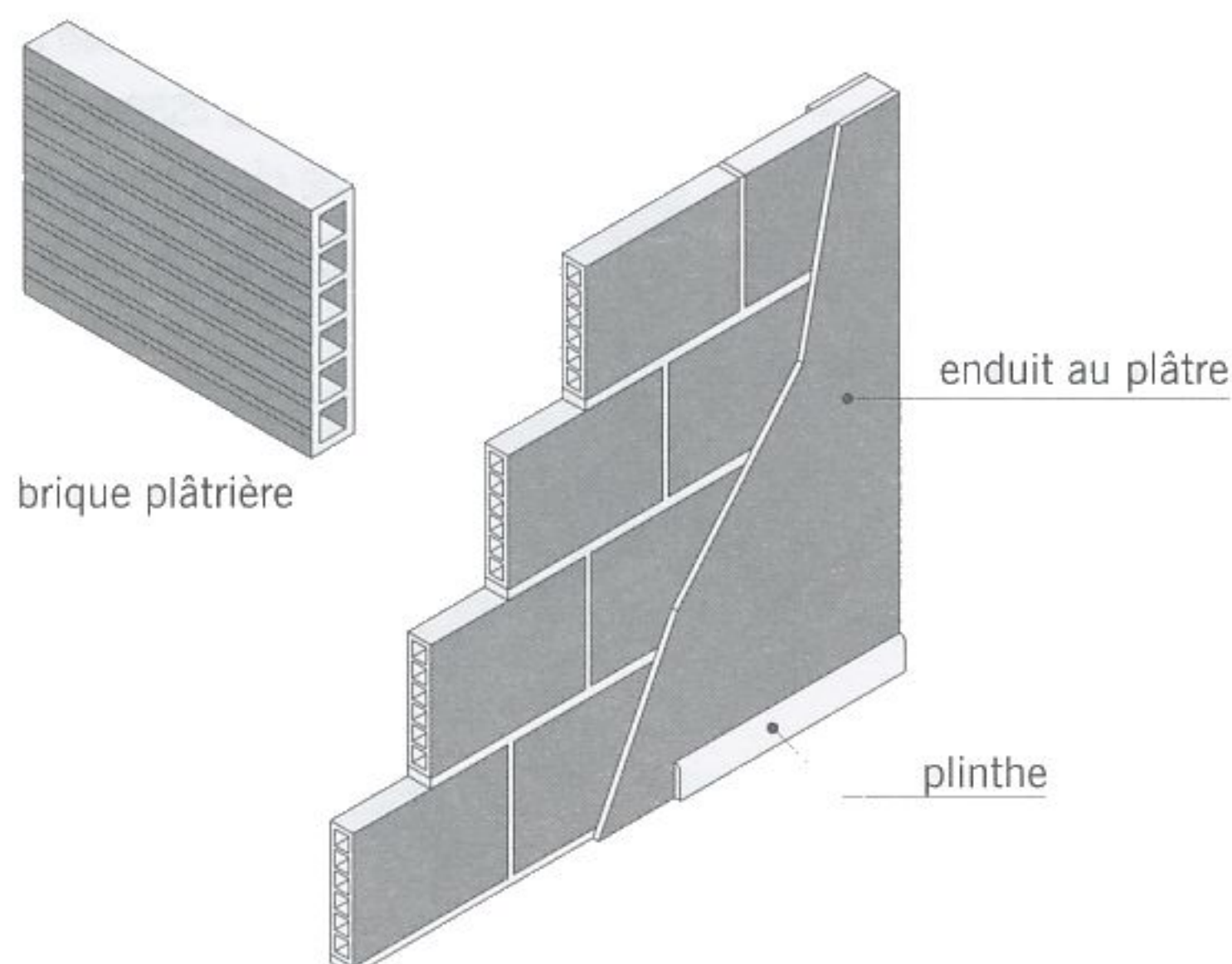
fig. 8.3 cloison pleine en briques plâtrières
