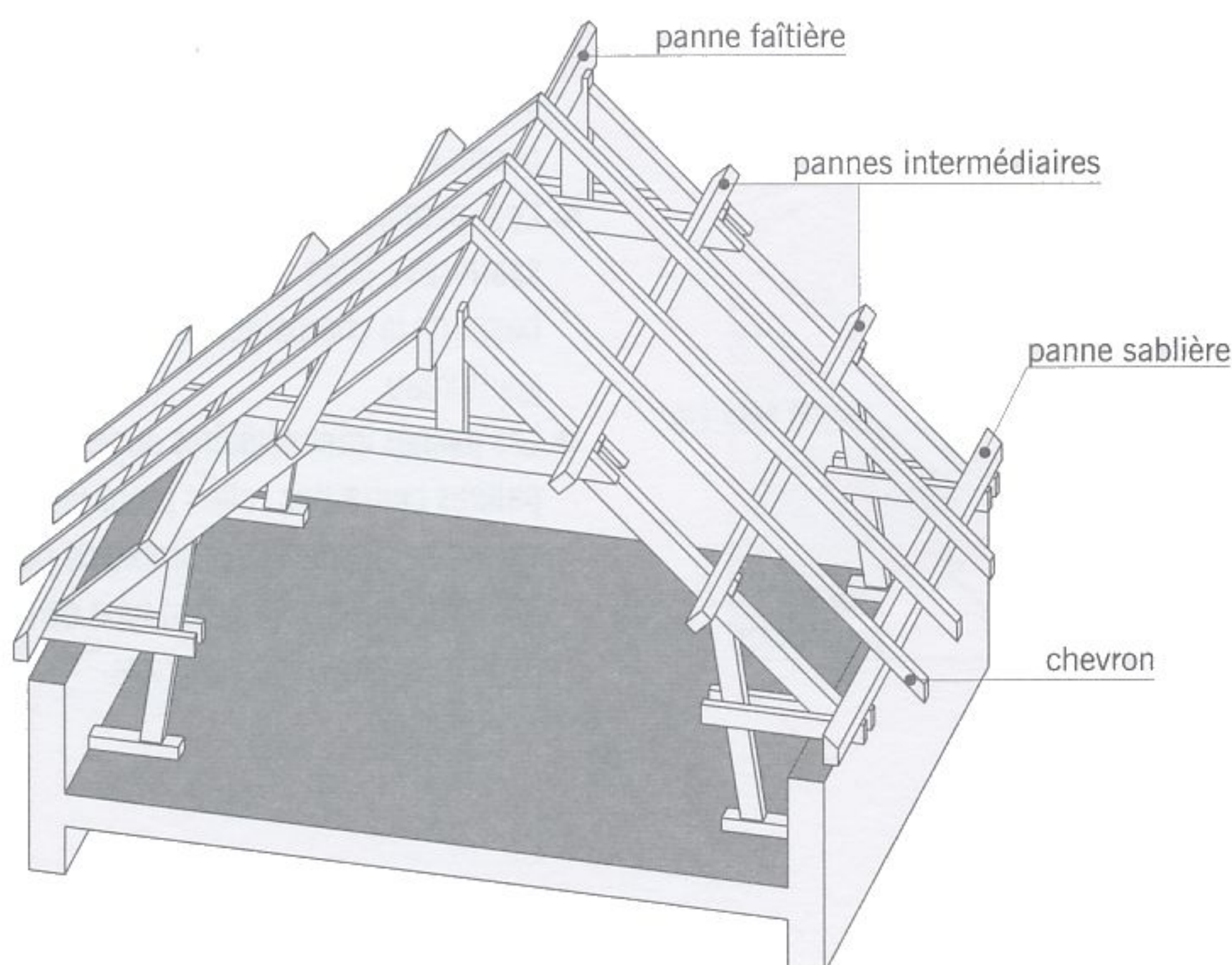
fig. 5.6 charpente avec fermes à entrait retroussé
