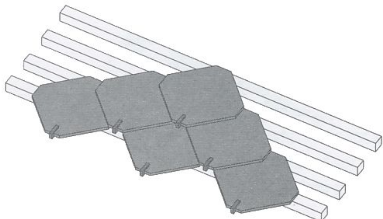
fig. 7.42 pose en diagonale
