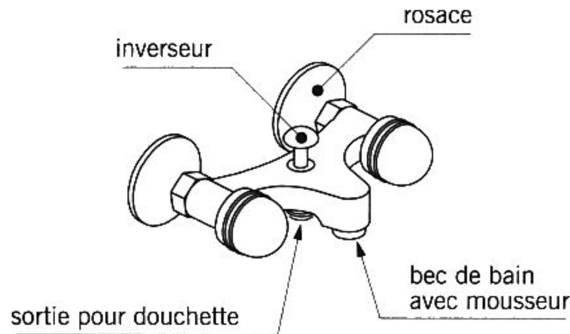
mélangeur de bains / douche
