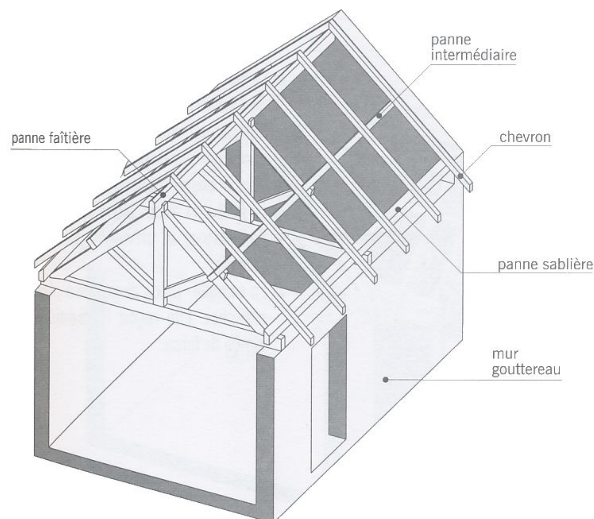
fig. 5.2 pannes reposant sur des fermes
