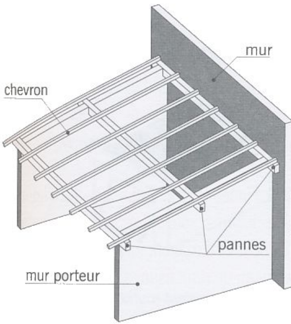
fig. 5.31 charpente d'appentis reposant sur des murs
