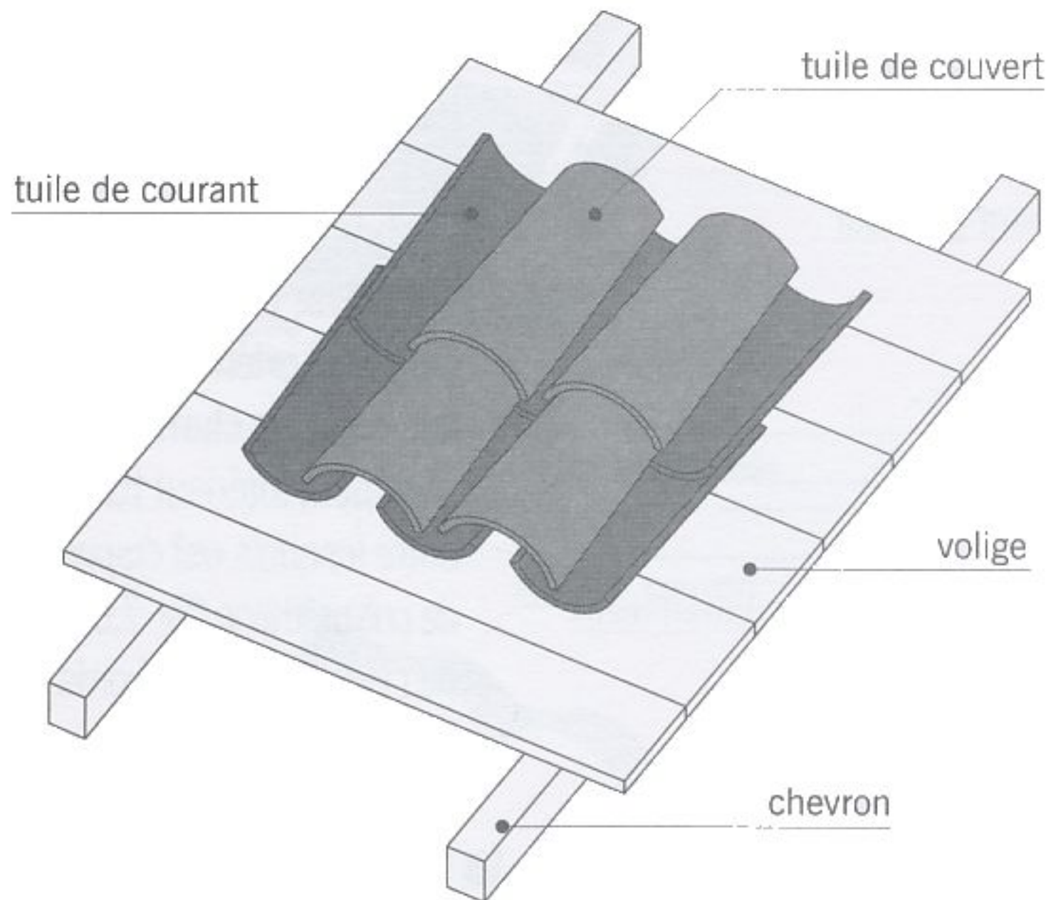
tuiles canal posées sur voliges
