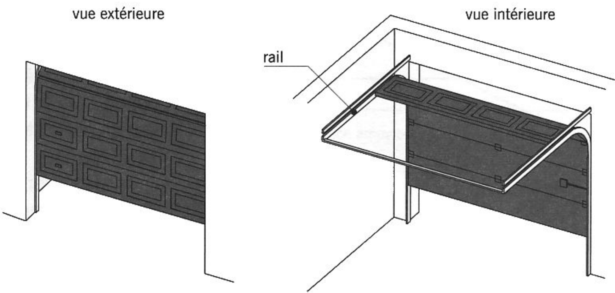
fig. 11.57 porte sectionnelle
