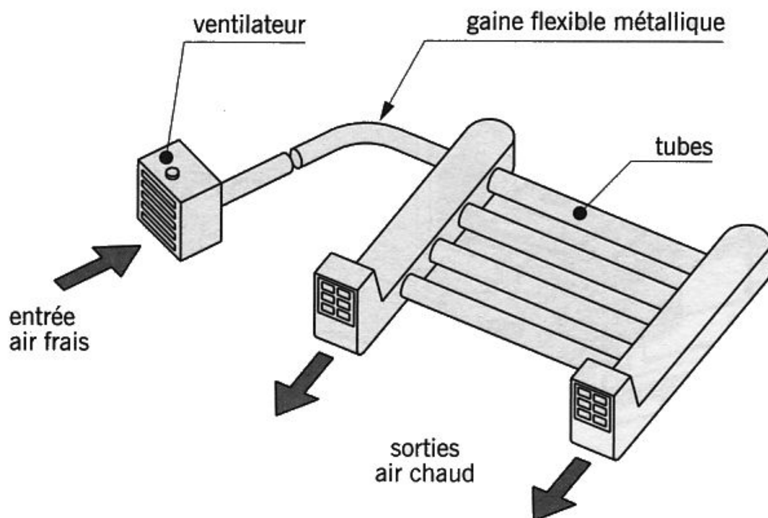
fig. 17.38 chenets soufflants
