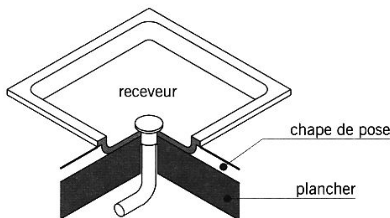
fig. 14.21 receveur à encastrer
