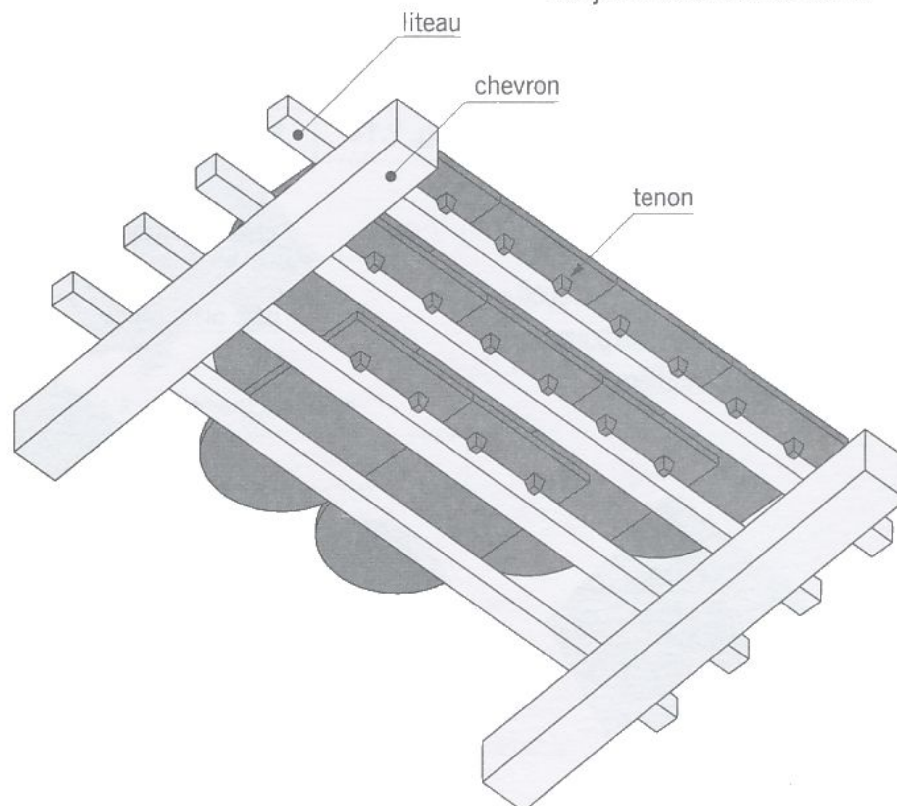
fig. 7.11 accrochage des tuiles plates
