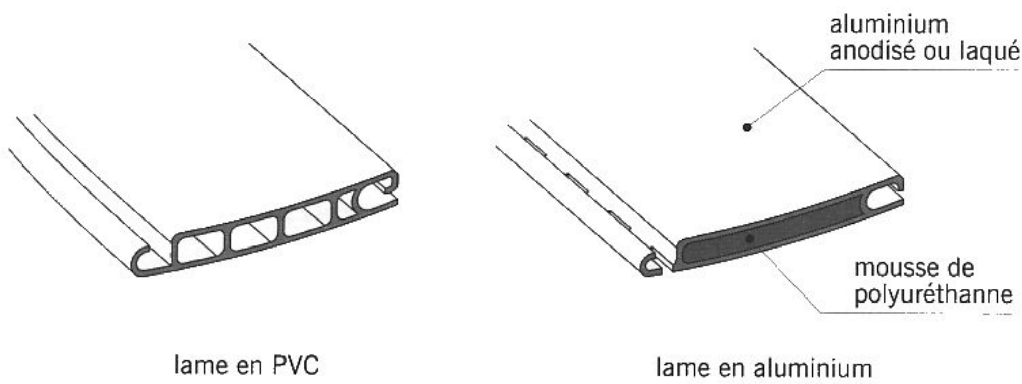
fig. 11.63 lames
