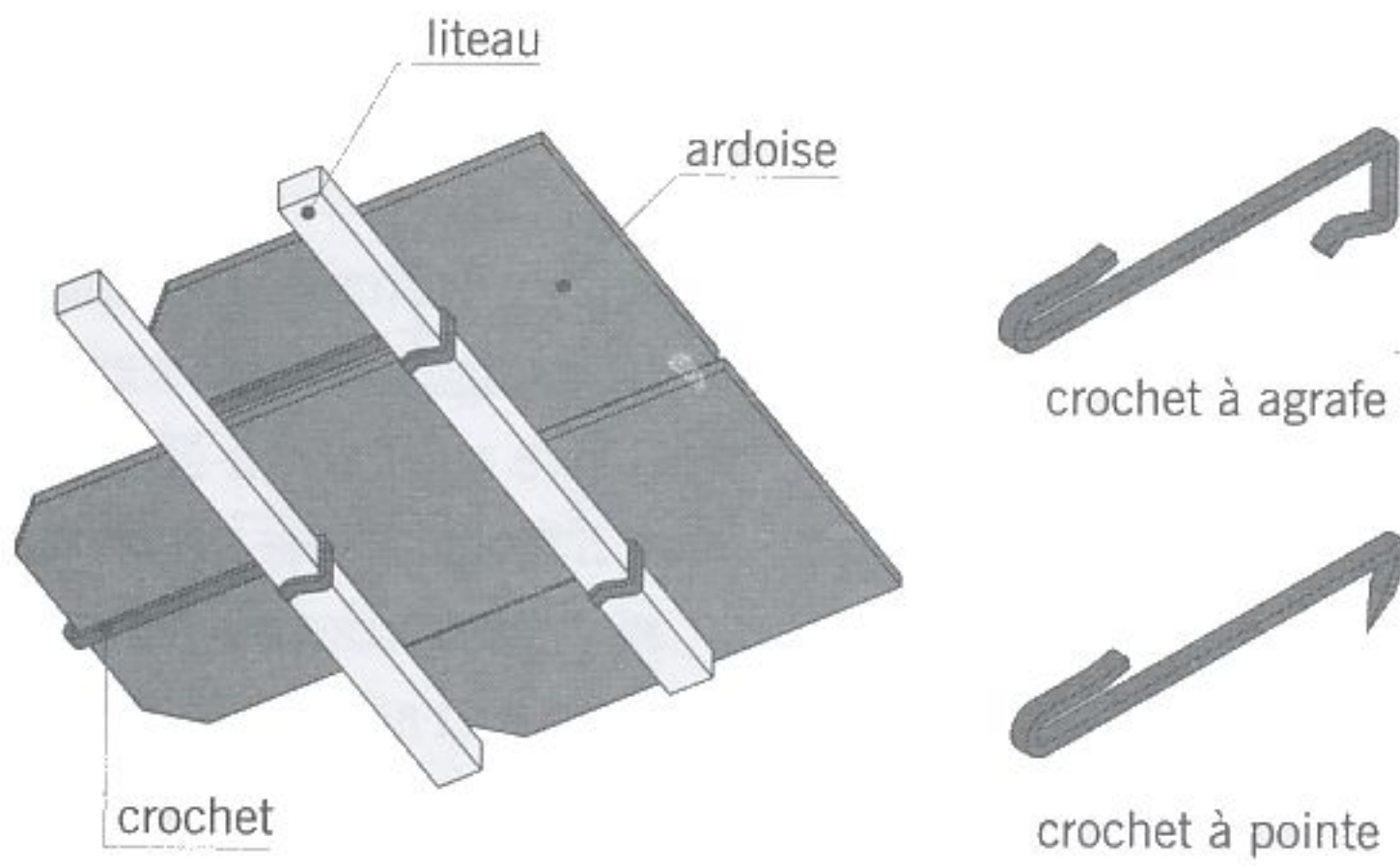
fig. 7.38 crochets pour ardoises
