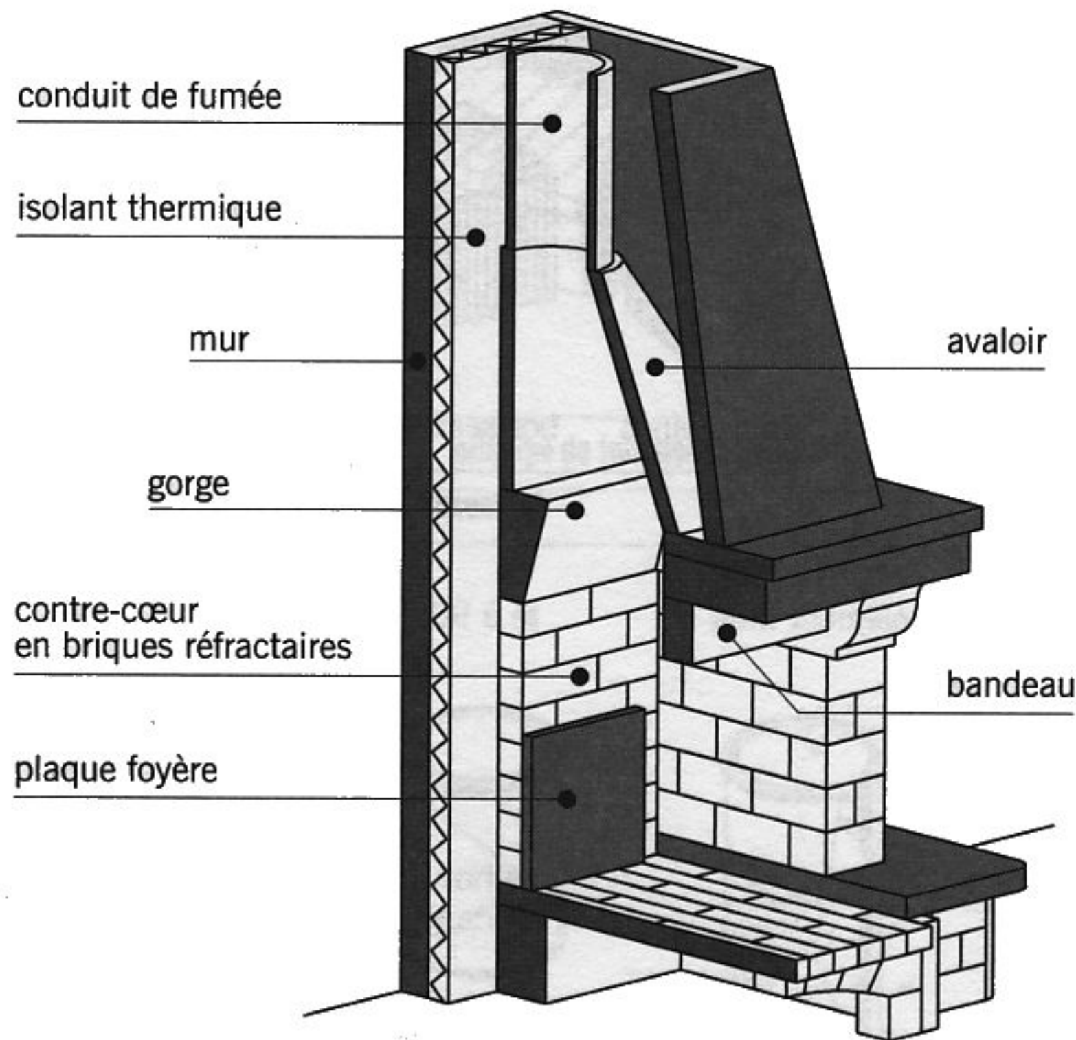
fig. 17.37 cheminée (2)
