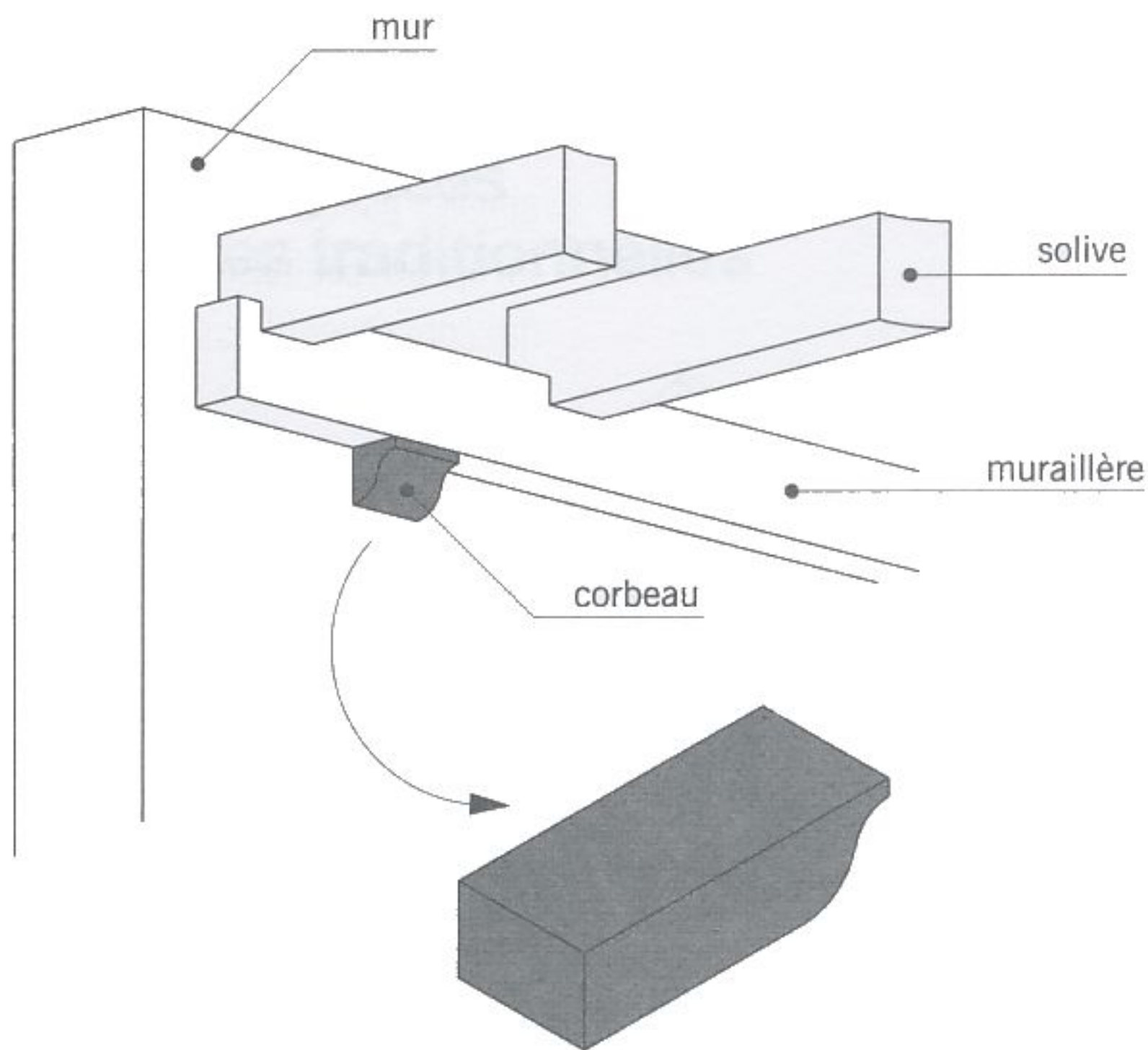
corbeau en pierre
