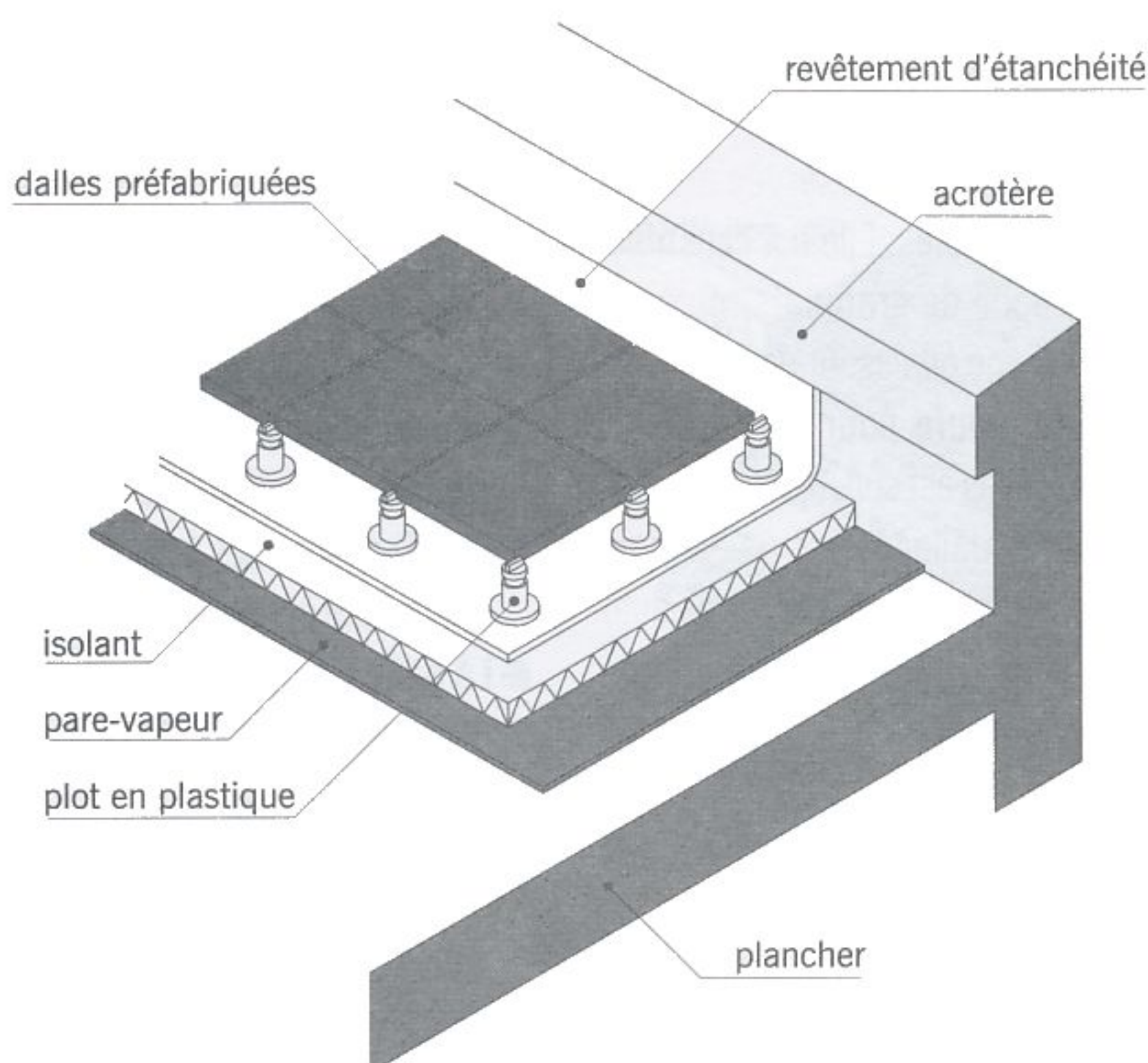
toiture-terrasse accessible aux piétons
