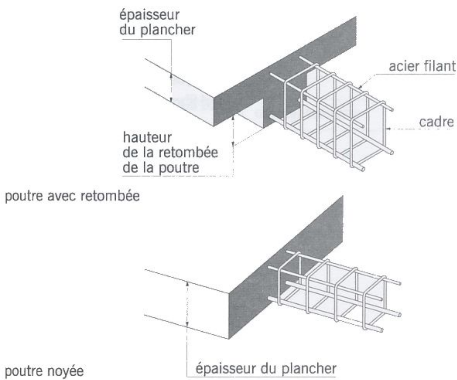
fig. 4.9 poutre
