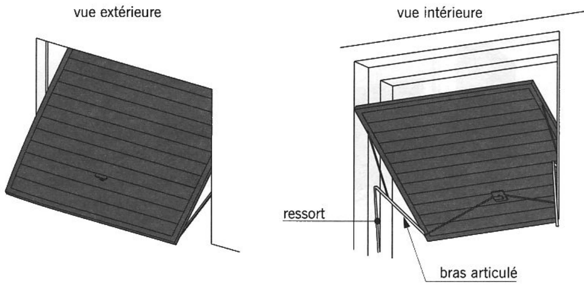
fig. 11.56 porte basculante
