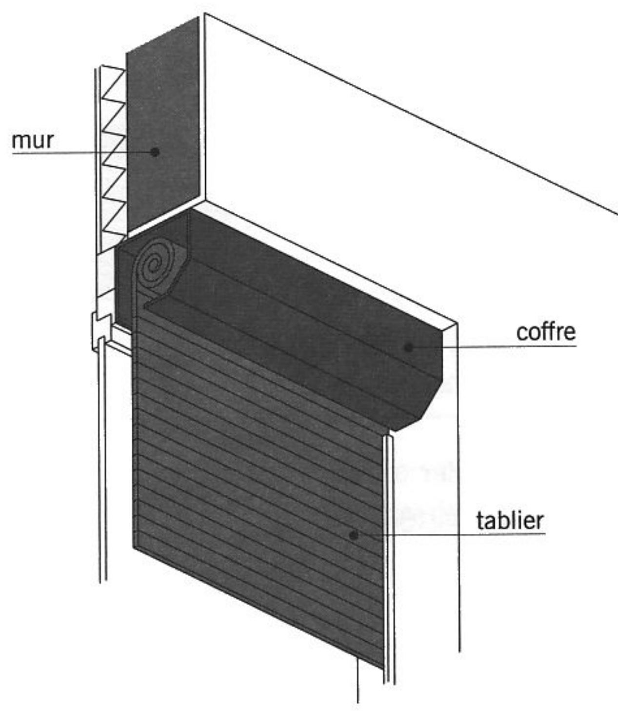
coffre apparent à l'extérieur
