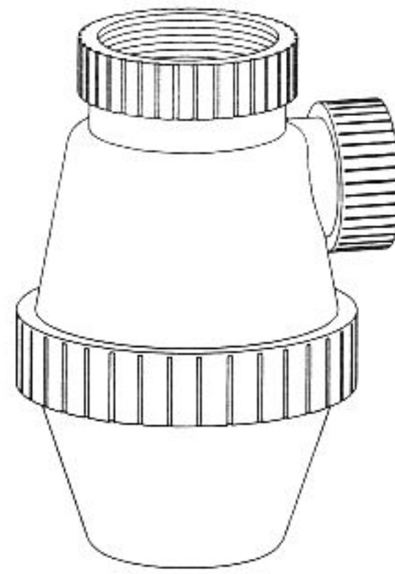
fig. 15.7 siphon de lavabo
