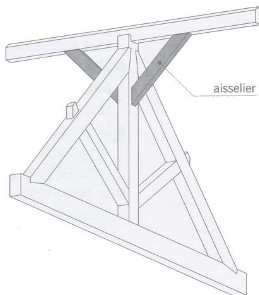
fig. 5.5 aisselier
