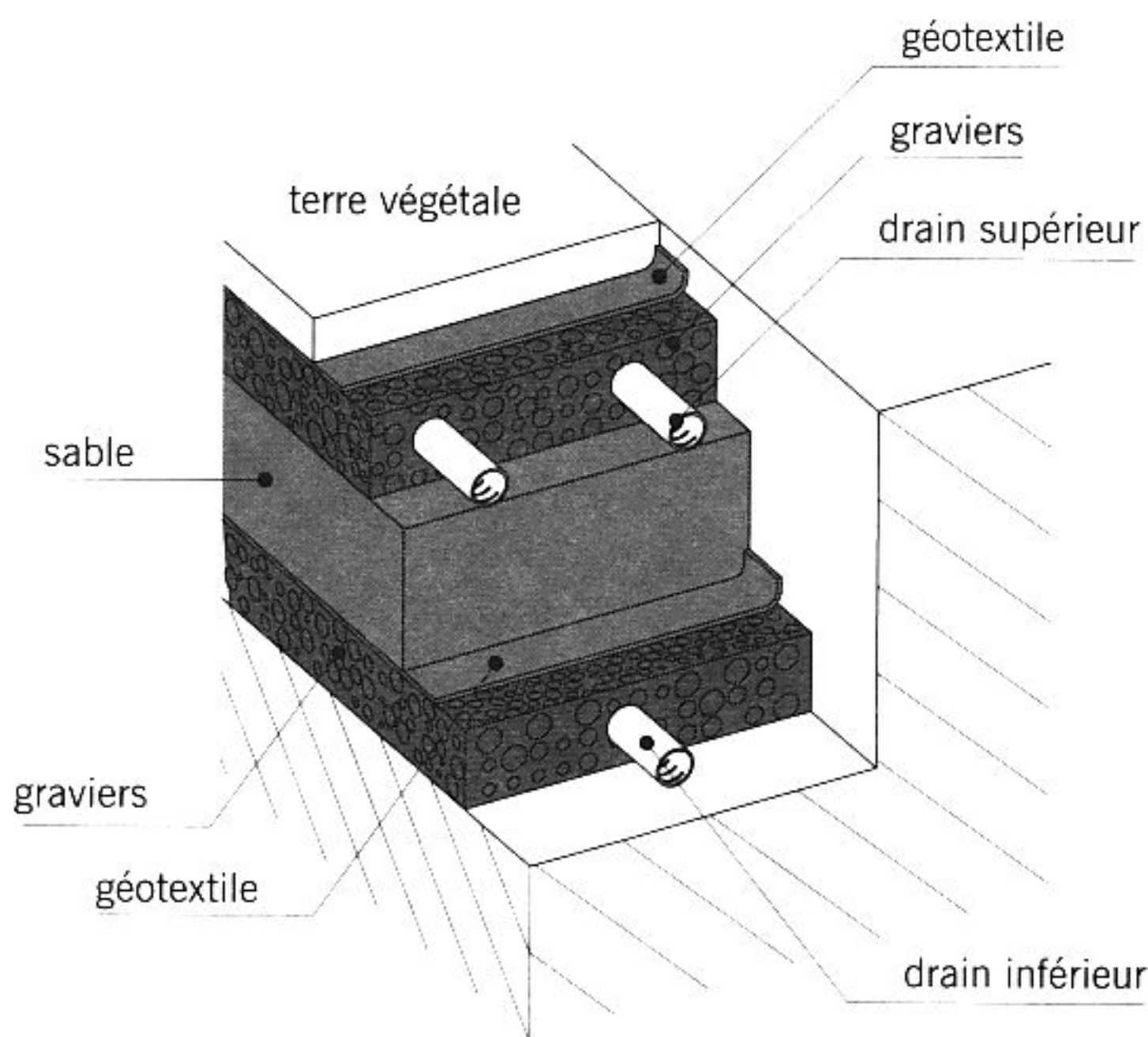
détail d'un filtre à sable vertical drainé
