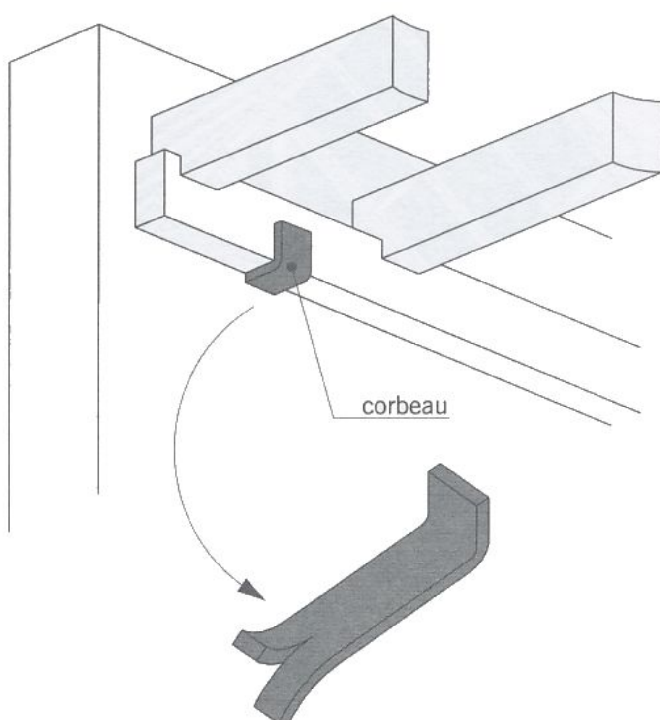
corbeau métallique
