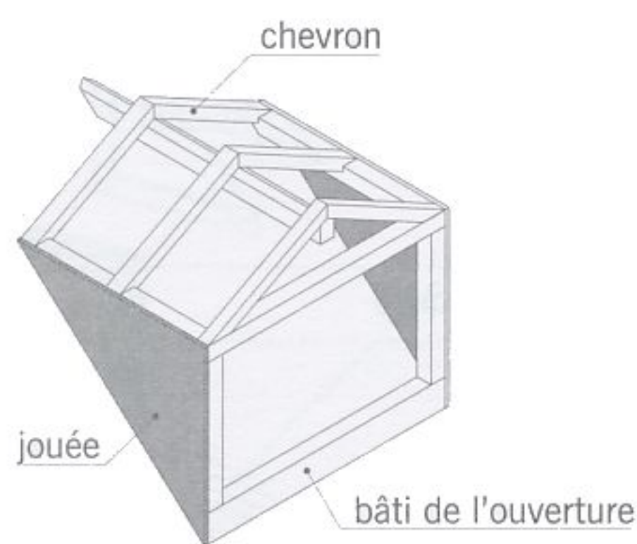
fig. 5.26 détail de la lucarne
