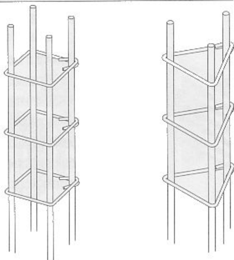
exemples d'armatures pour chaînages verticaux
