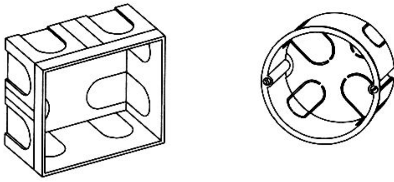
fig. 16.24 boîtiers d'encadrement
