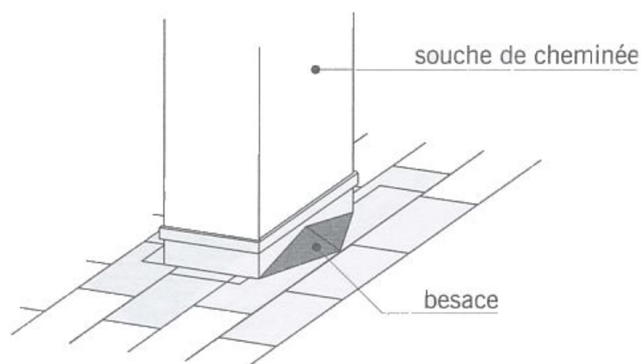
fig. 7.52 besace
