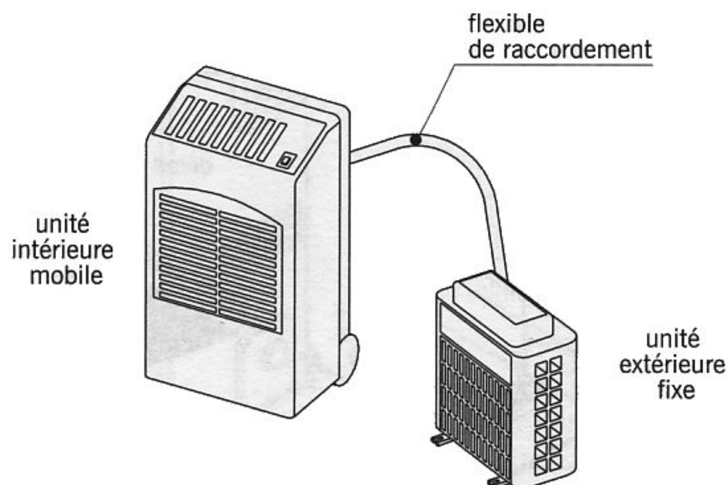
fig. 17.17 climatiseur bi-bloc
