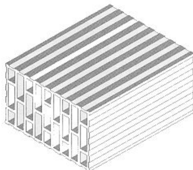
fig. 3.19 brique isolante
