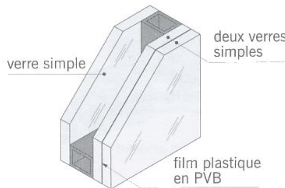
fig. 11.21 double vitrage de sécurité
