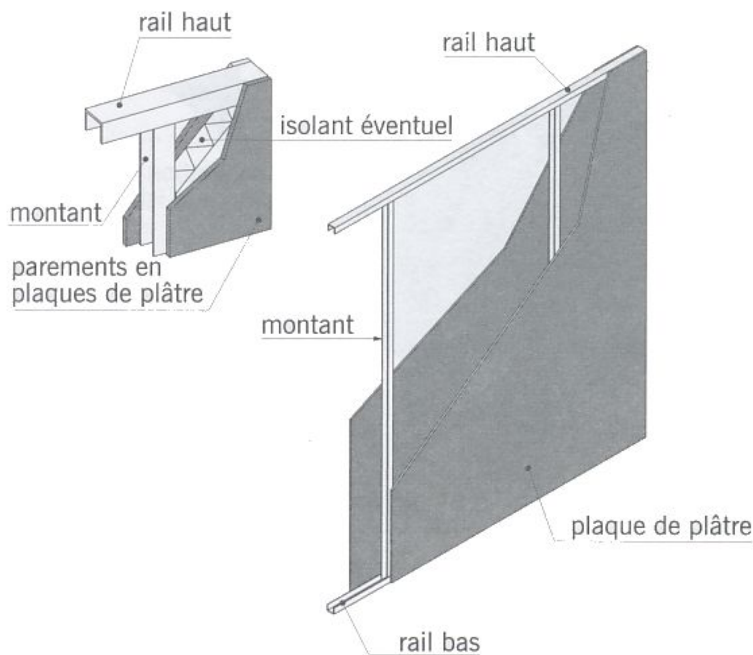
fig. 8.7 cloison sèche sur ossature métallique
