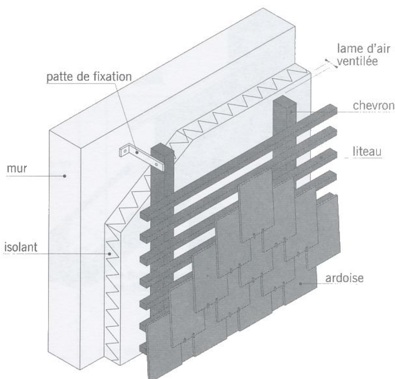
bardage d'ardoises
