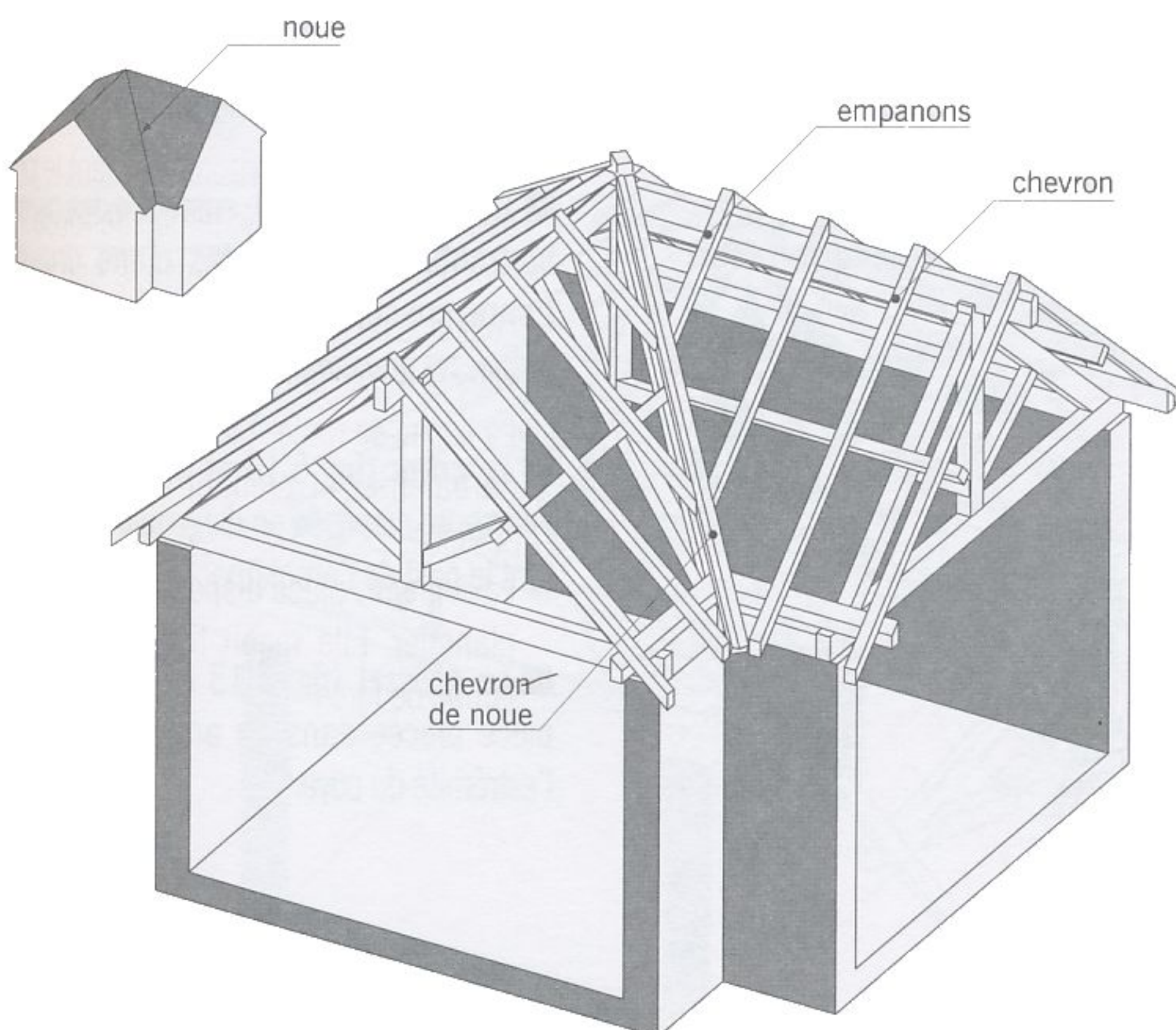
fig. 5.10 intersection de deux charpentes observée côté noue
