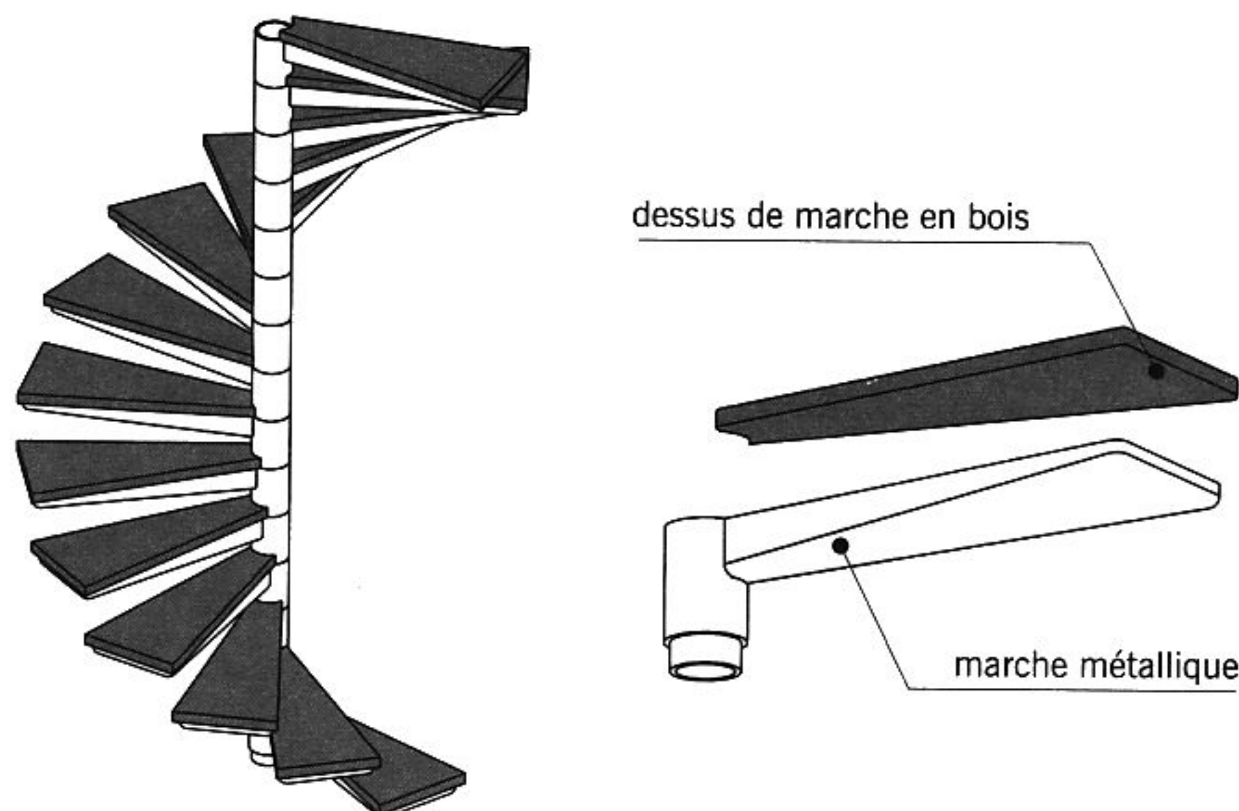
fig. 13.32 escalier métallique hélicoïdal
