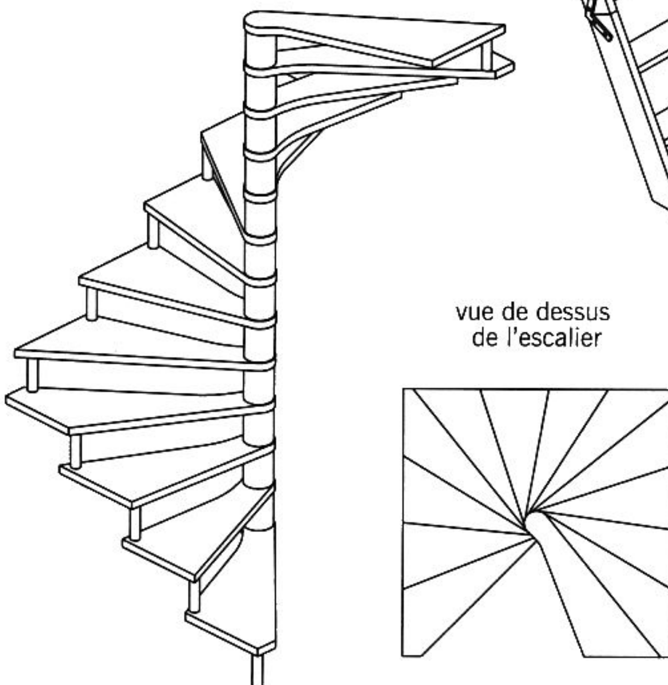
fig. 13.23 escalier hélicoïdal sur plan carré
