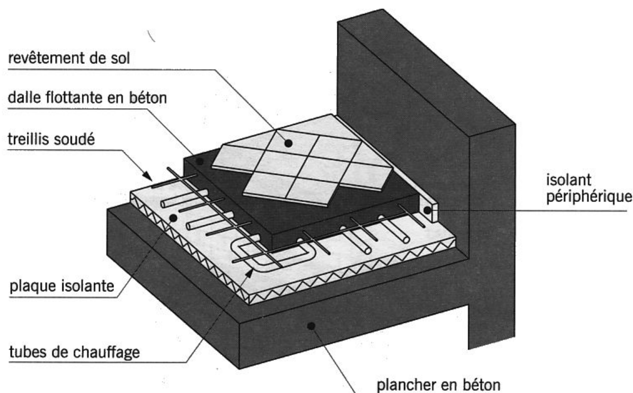
fig. 17.29 plancher chauffant à eau chaude
