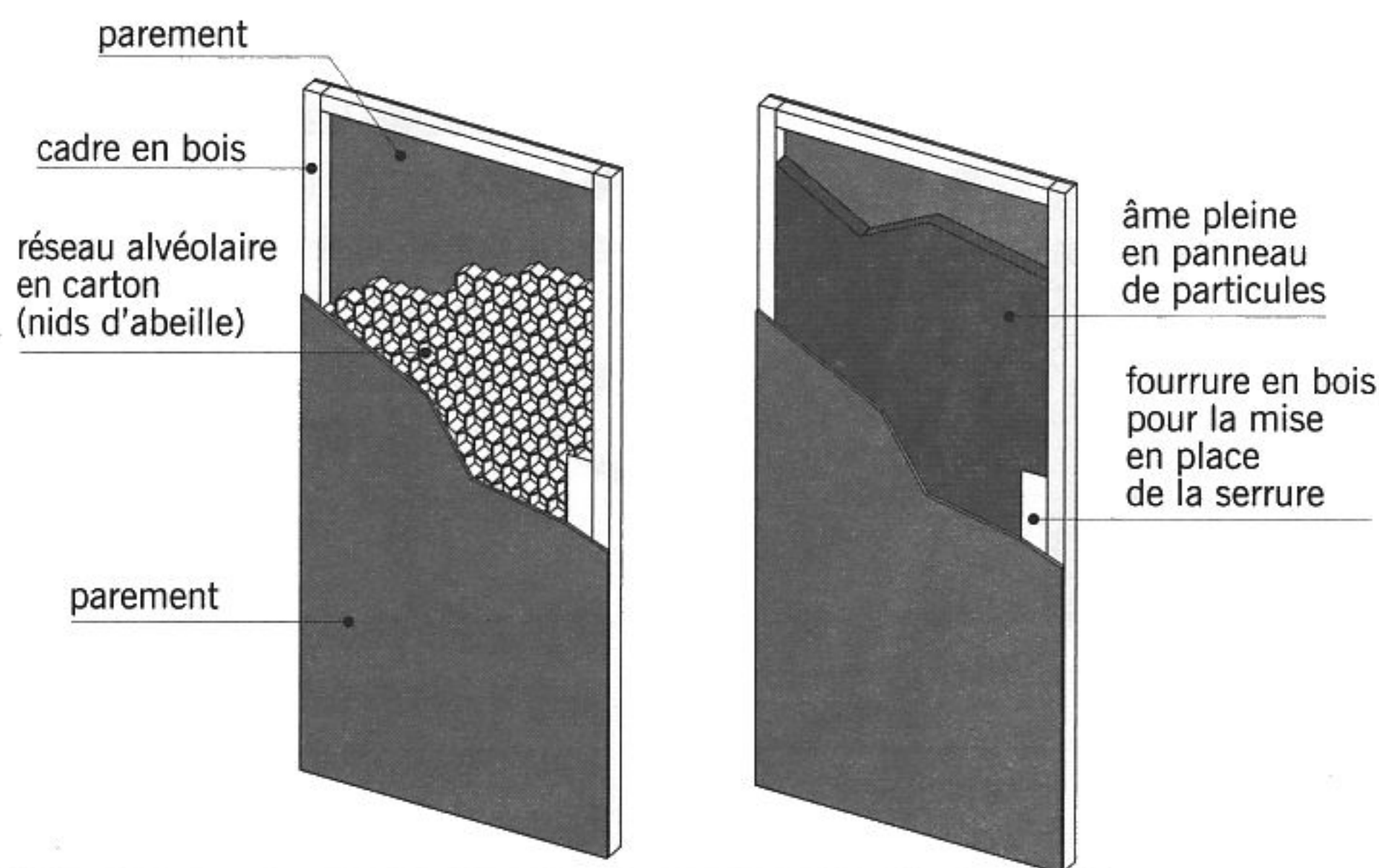
fig. 12.1 portes isoplanes
