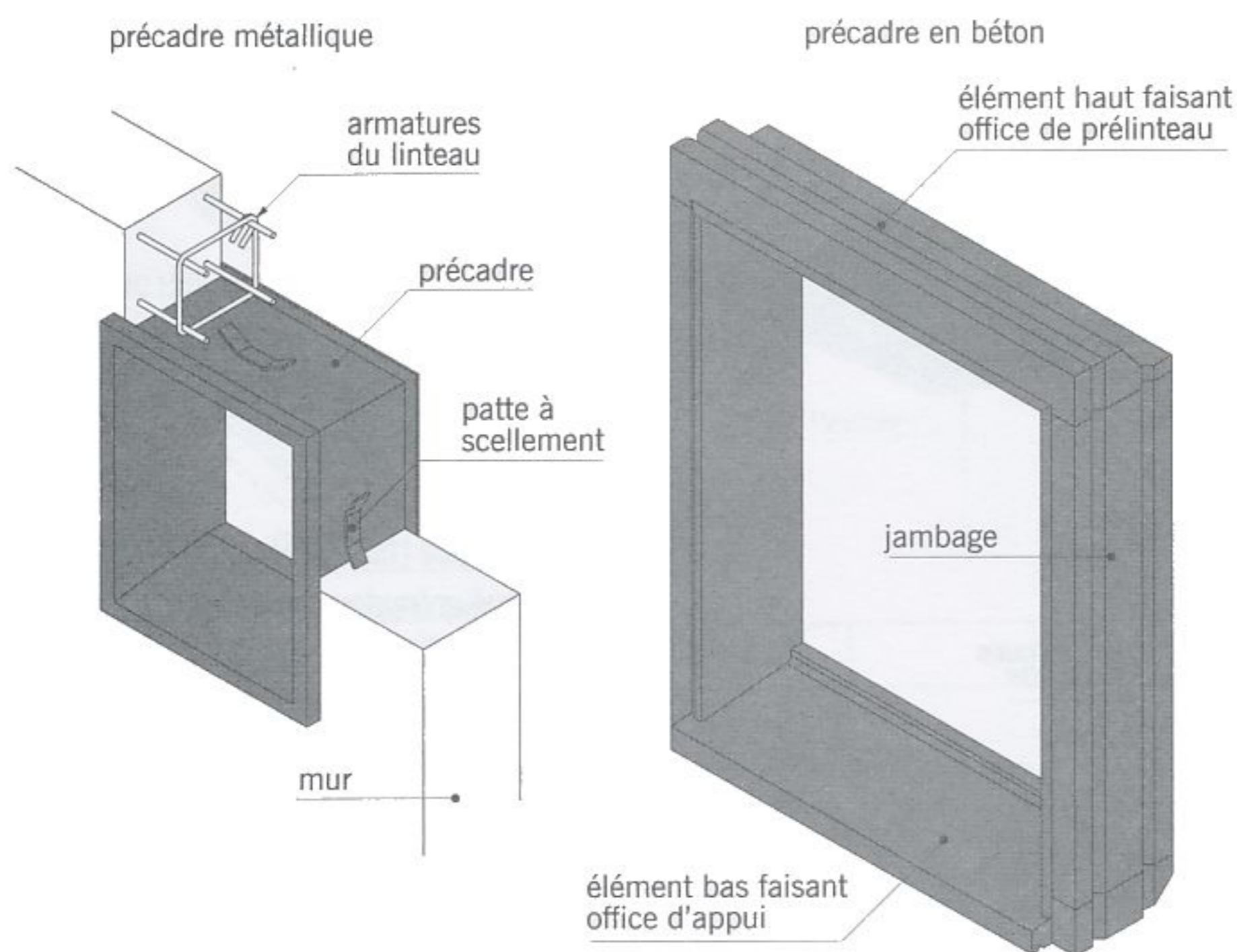
fig. 3.38 précadres
