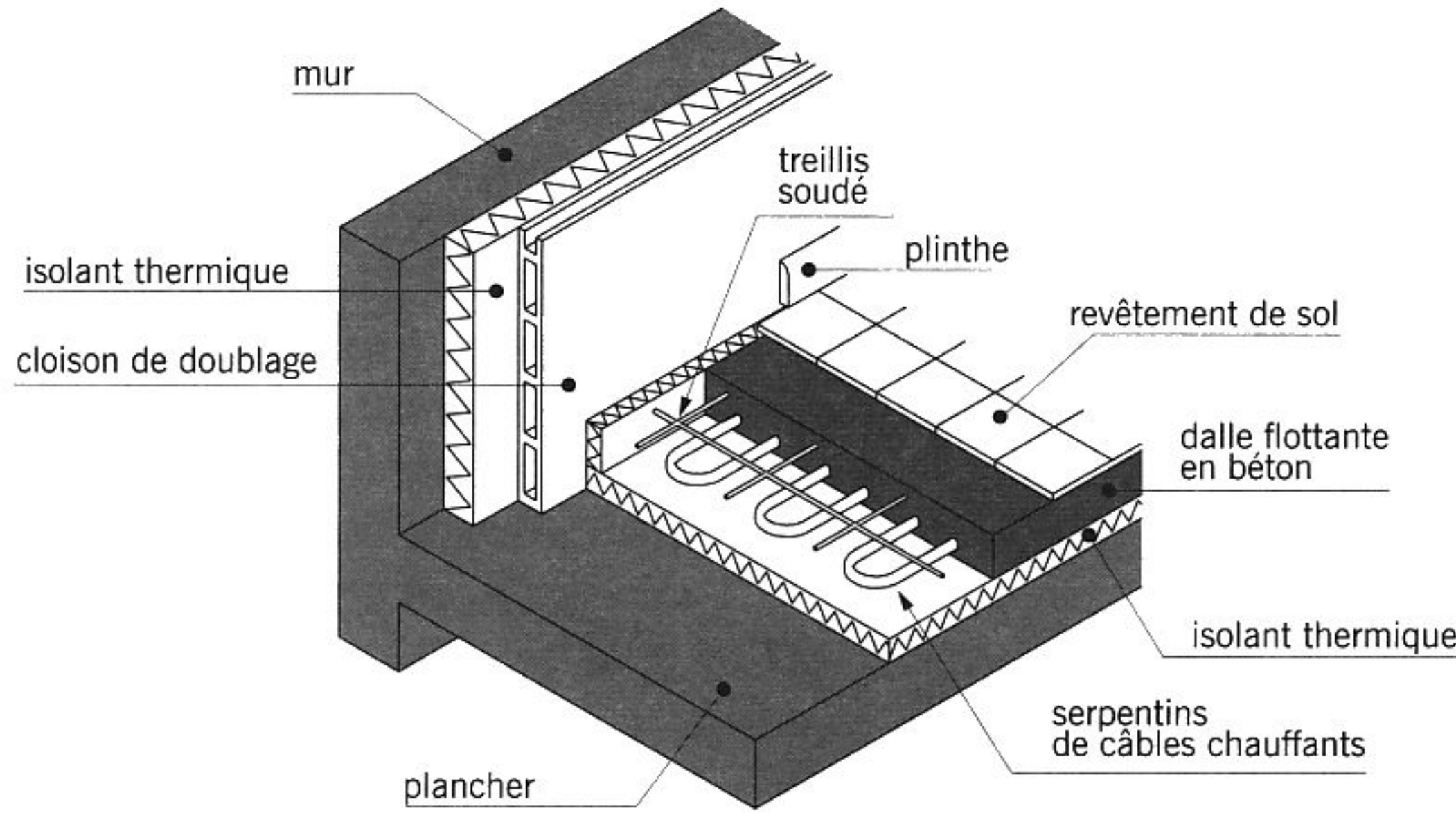
fig. 17.11 plancher chauffant à accumulation
