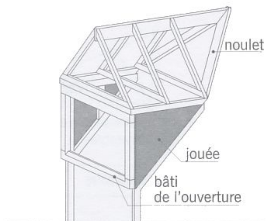
fig. 5.29 détail de la lucarne
