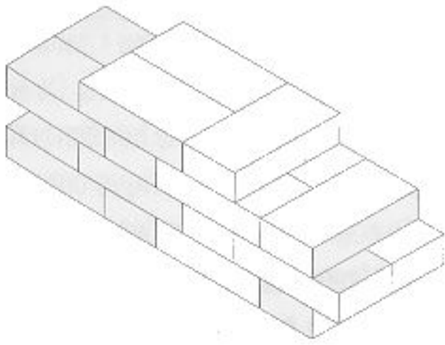
fig. 3.15 mur en briques pleines
