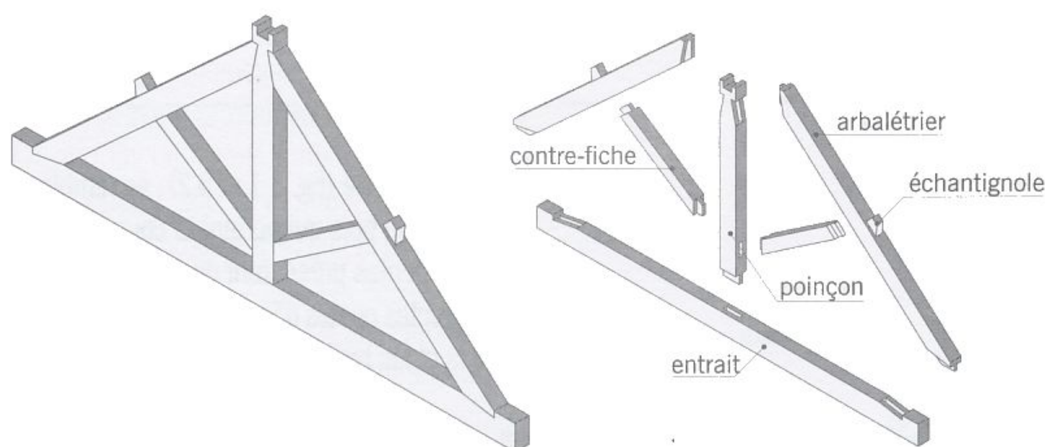
fig. 5.4 éléments constitutifs d'une ferme
