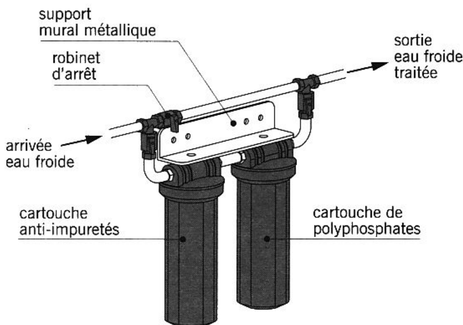
fig. 14.15 dispositif anti-tartre
