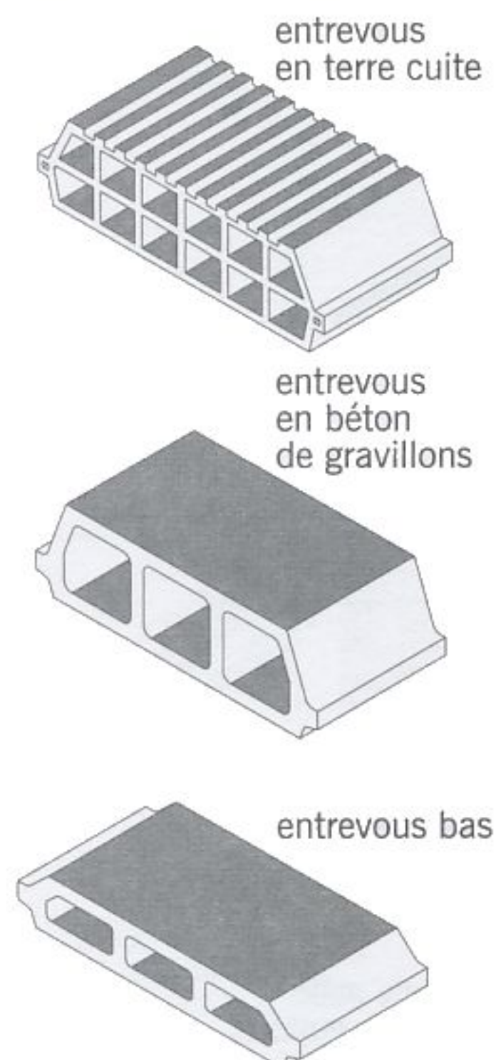
entrevous
