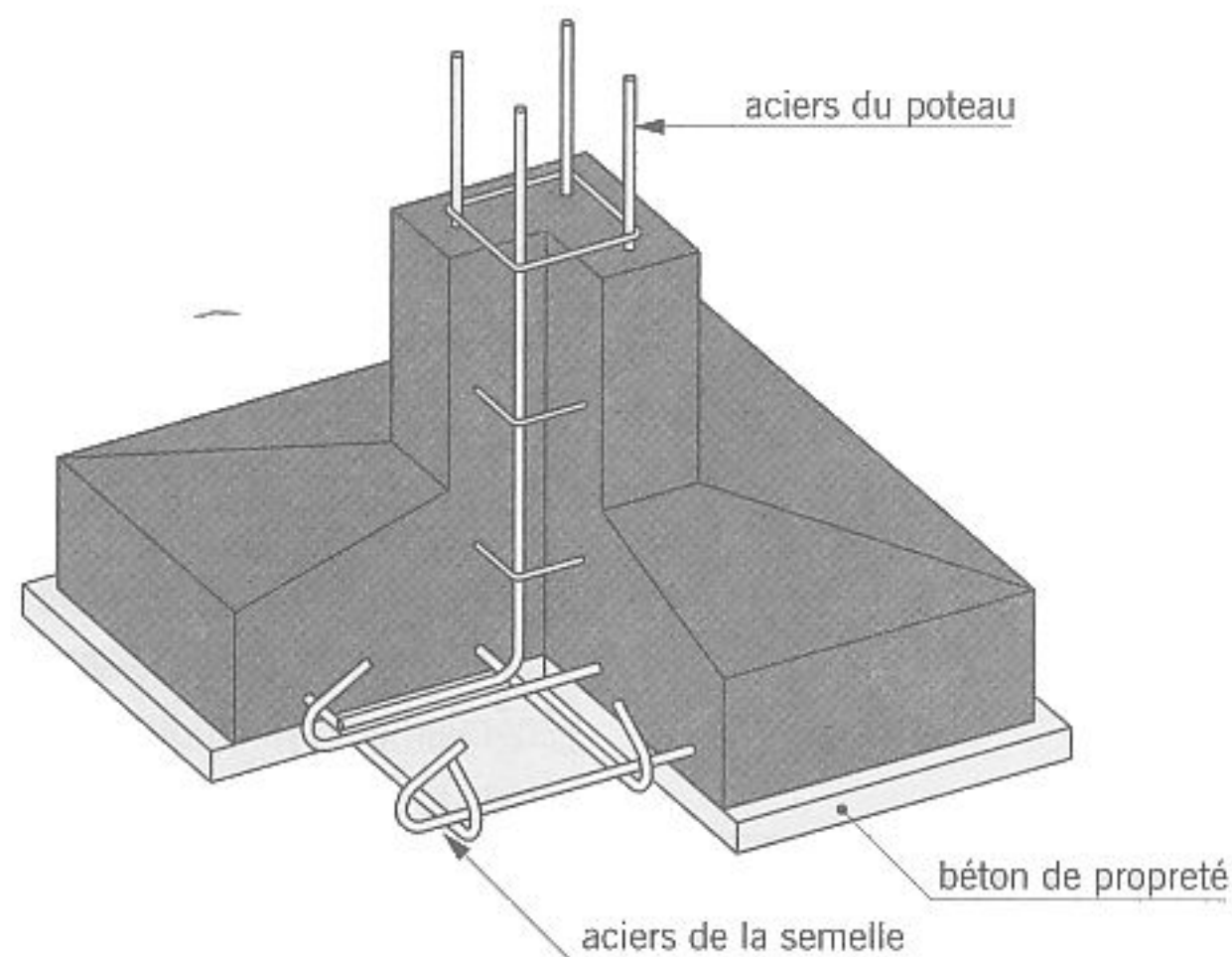
fig. 2.8 semelle isolée sous poteau
