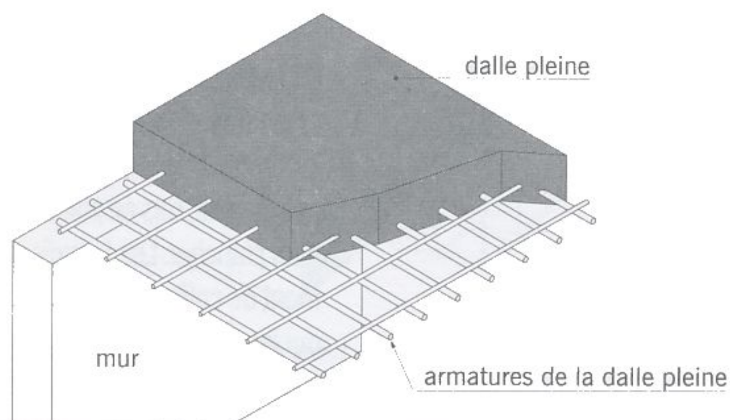
fig. 4.2 dalle pleine
