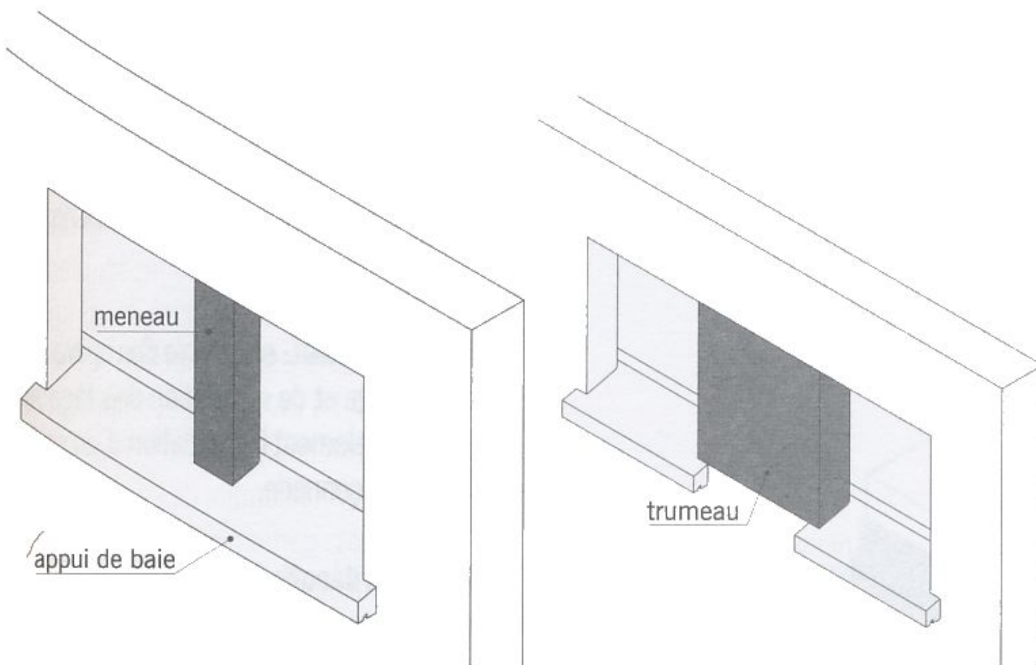
fig. 3.35 meneau
