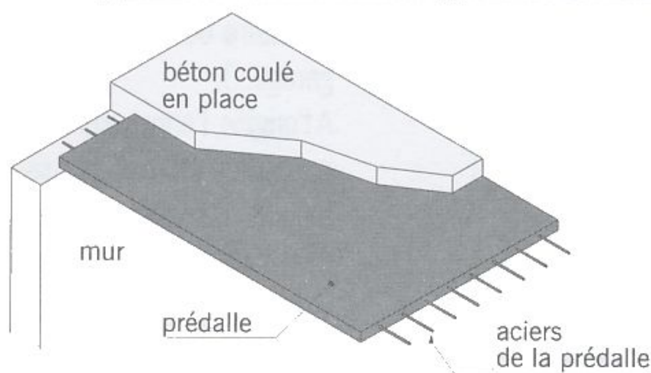
fig. 4.2 dalle pleine
