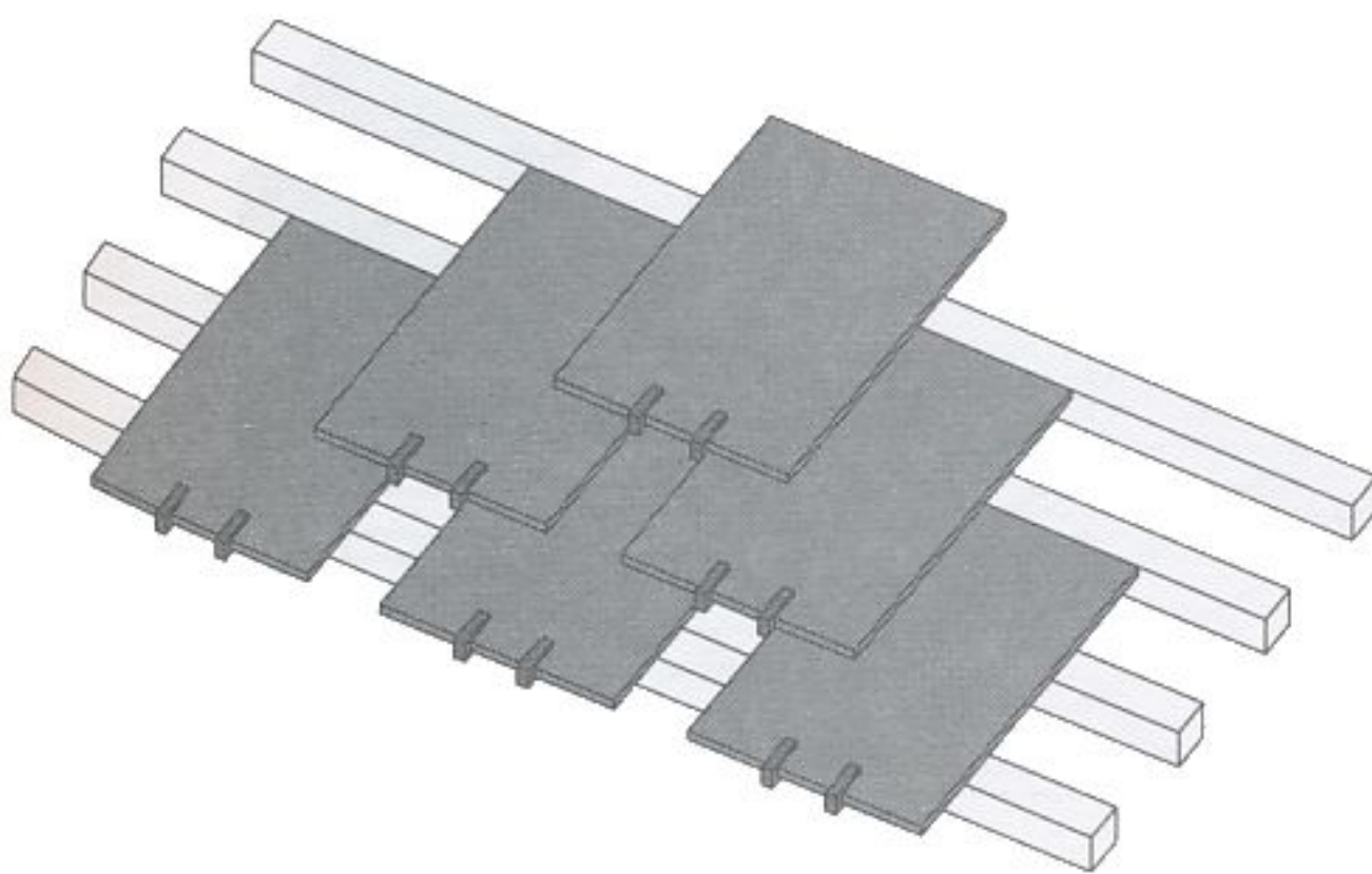
fig. 7.41 pose à claire-voie ordinaire
