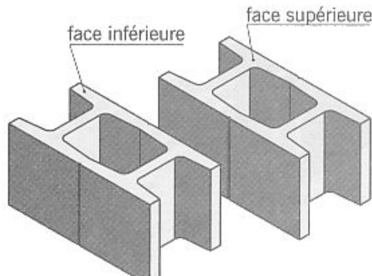
fig. 3.8 bloc à bancher
