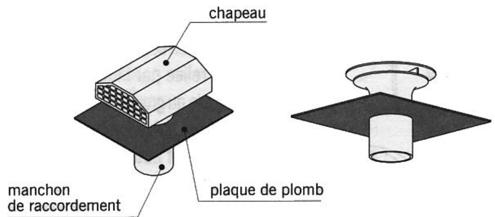
fig. 18.12 sorties de toit
