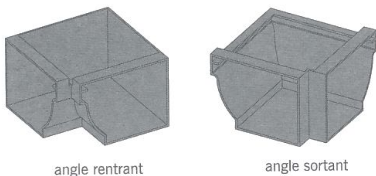
fig. 7.66 angles pour gouttière corniche
